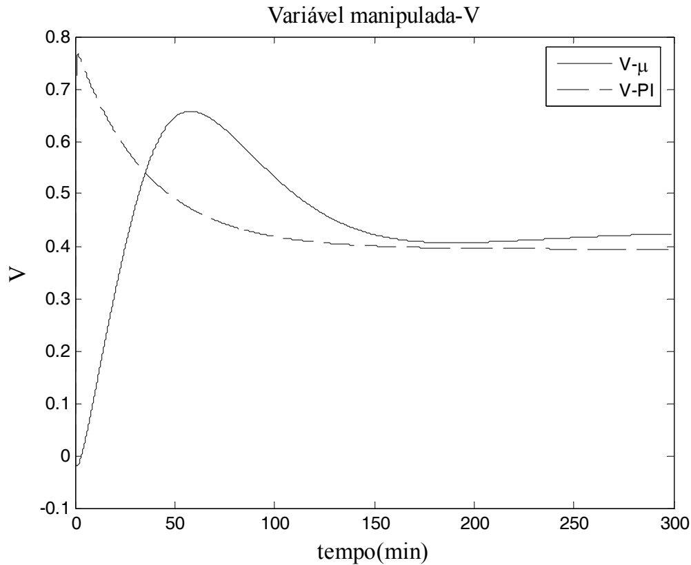
Figura 3. 12 – (a) Sistema em malha fechada com controladores \mu e PI.
