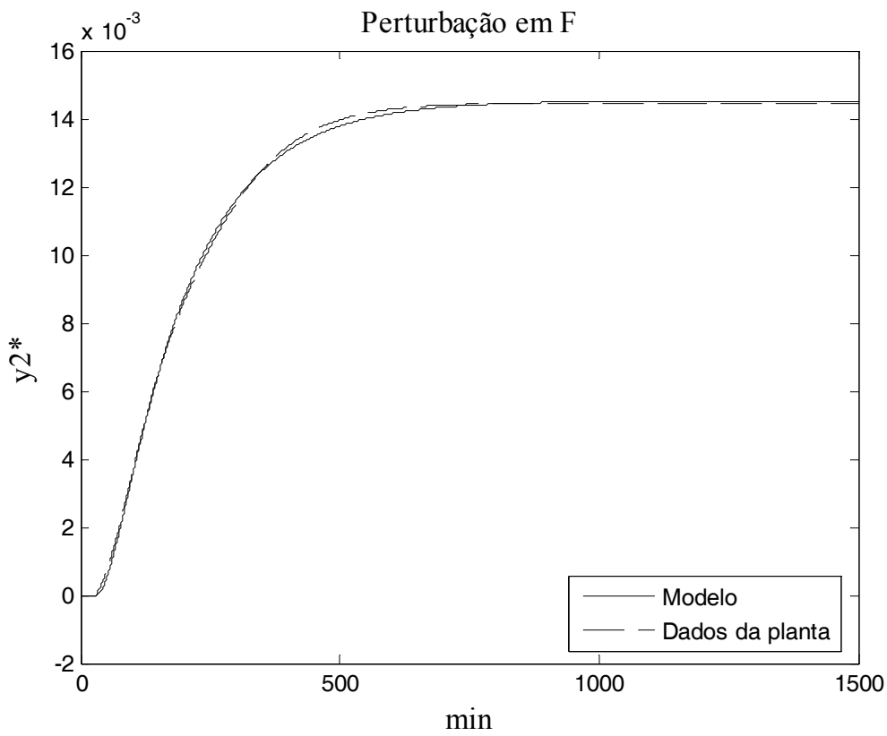
Figura III. 7 – Distúrbios aplicados à coluna com estrutura DV em malha aberta.
