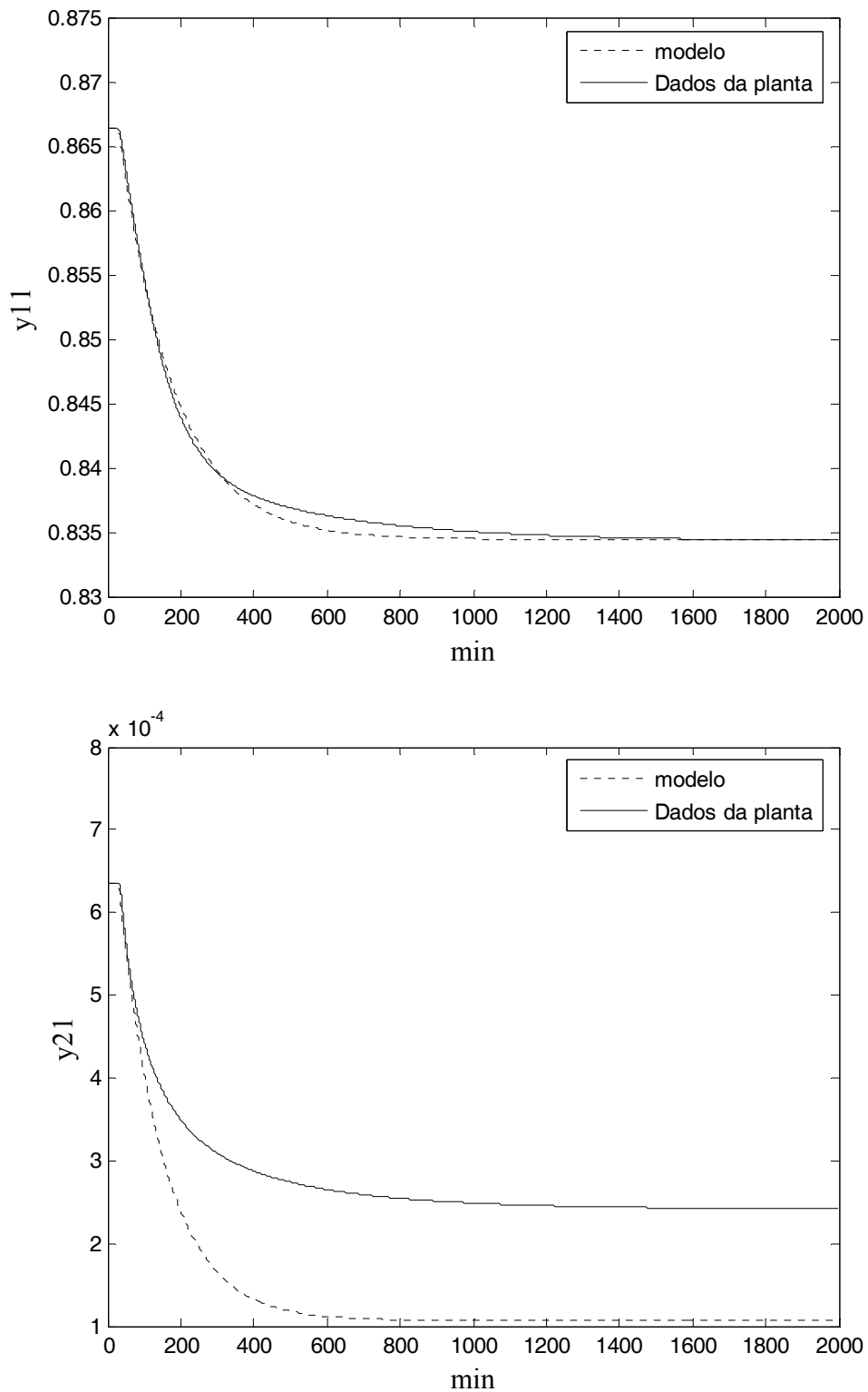
Figura II. 1 – Resposta do topo e do fundo a um degrau positivo em u_1(D) para a estrutura DV.
