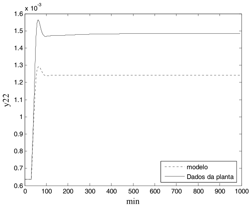
Figura II. 16 – Resposta do topo e do fundo a um degrau negativo em u_2 ( setpoint de T) para a estrutura LVCascata.
