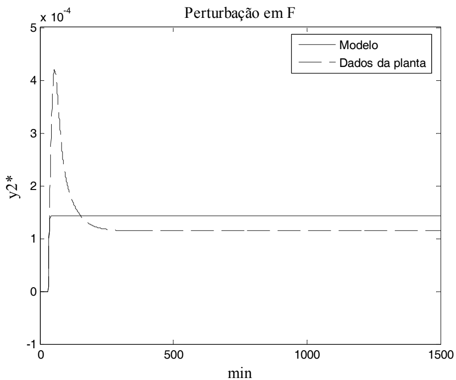
Figura III. 1 – Distúrbios aplicados à coluna com estrutura LVCascata em malha aberta.
