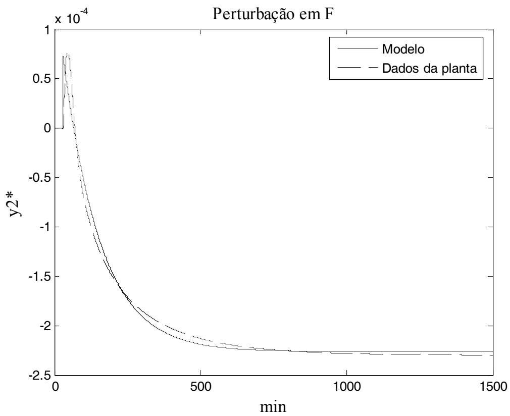
Figura III. 10 – Distúrbios aplicados à coluna com estrutura L/D_V/B em malha aberta.
