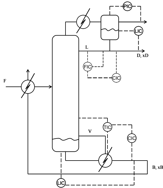
Figura 4. 4 – Estrutura de controle LVCascata
