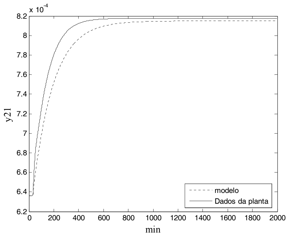
Figura II. 5 – Resposta do topo e do fundo a um degrau positivo em u_1(L/D) para a estrutura L/D_{V/B}
