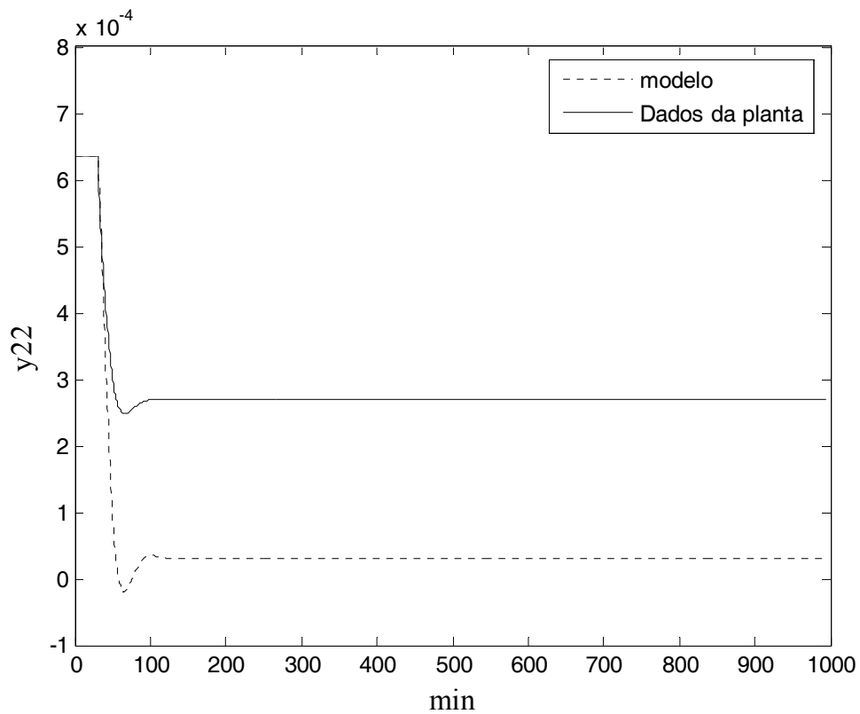
Figura II. 14 – Resposta do topo e do fundo a um degrau positivo em u_2 ( setpoint de T) para a estrutura LVCascata.
