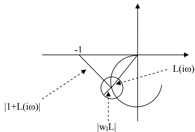
Figura 3. 4 – Diagrama de Nyquist para modelo nominal, mostrando a incerteza em um ponto.
