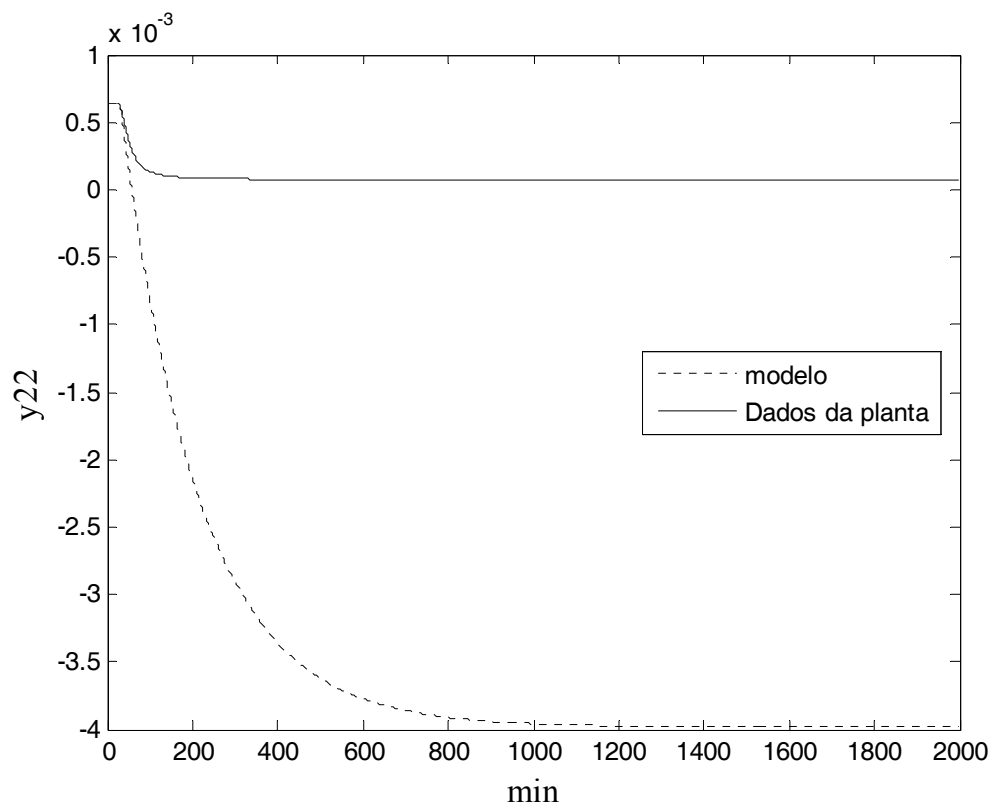
Figura II. 6 – Resposta do topo e do fundo a um degrau positivo em u_2(V/B) para a estrutura L/D_V/B .
