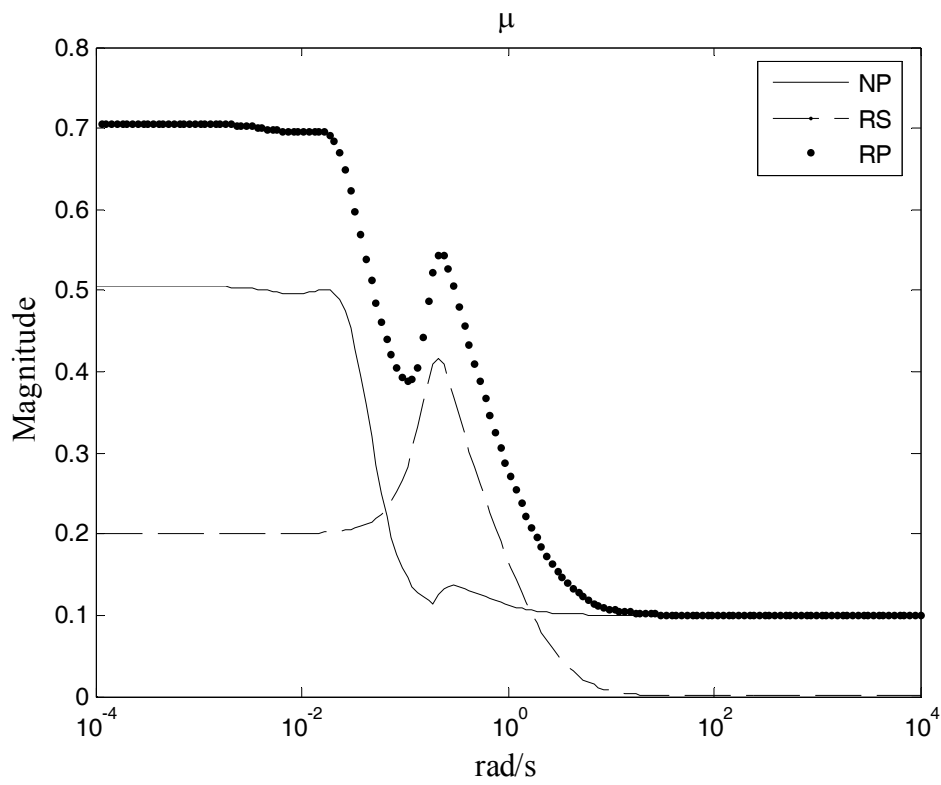
Figura 3. 10 – (a) Simulação do sistema 3.55 em malha fechada. (b) Análise de NP, RS e RP.
