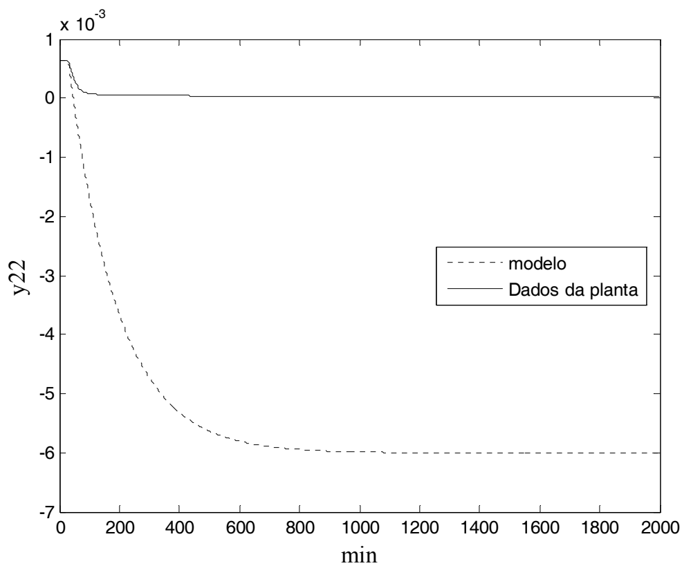
Figura II. 2 – Resposta do topo e do fundo a um degrau positivo em u_2(V) para a estrutura DV.
