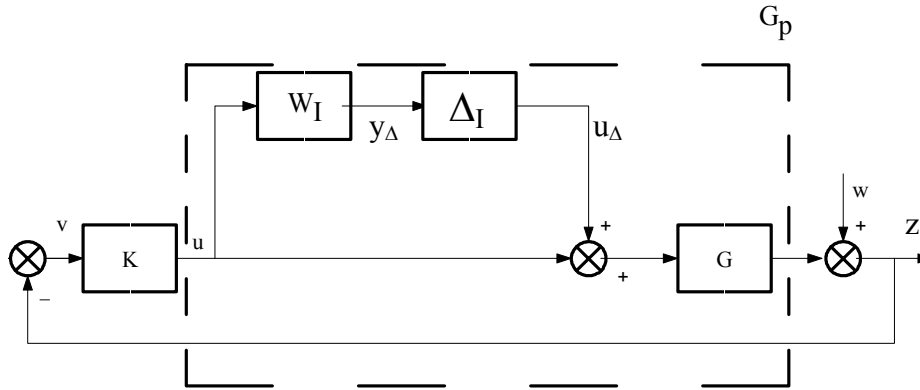
Figura 3. 3 – Planta G admitindo incertezas multiplicativas na entrada
