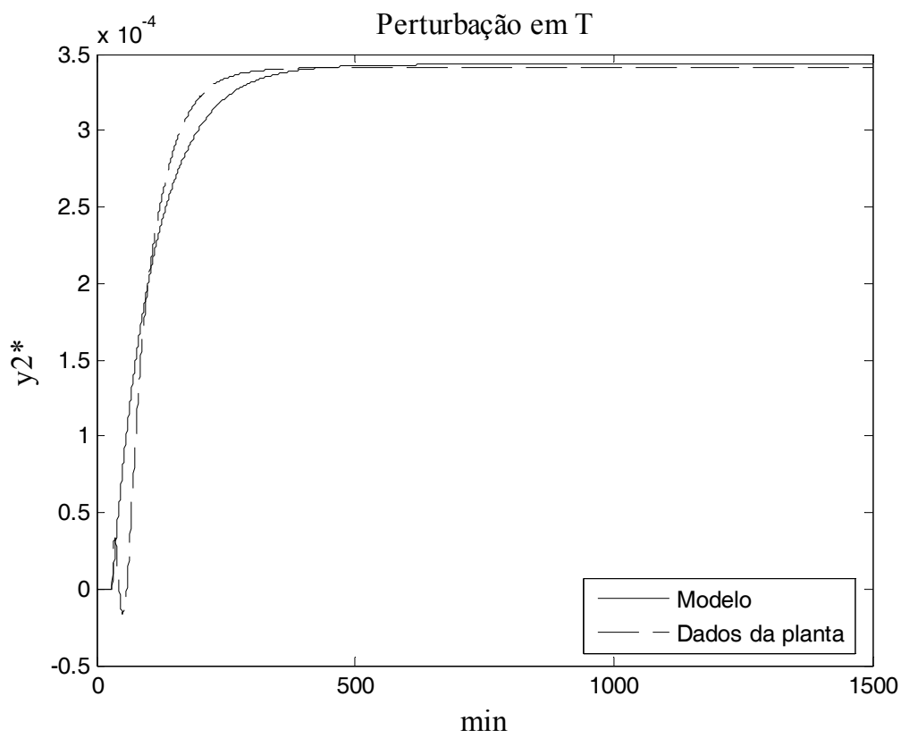
Figura III. 2 – Distúrbios aplicados à coluna com estrutura LVCascata em malha aberta.
