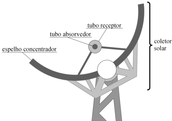
Figura 3.1: Estrutura do coletor solar de calha parabólica.
