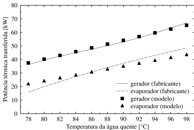
Figura 5.9: Comparação entre o modelo teórico e os dados do fabricante para a condição com água de resfriamento a 29,4^{\circ}\text{C} e água gelada a 9,0^{\circ}\text{C} na saída do evaporador.
