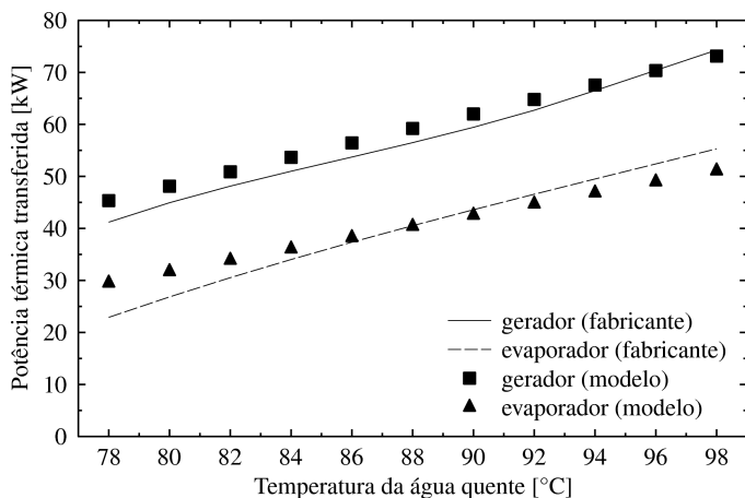
Figura 5.8: Comparação entre o modelo teórico e os dados do fabricante para a condição com água de resfriamento a 26,7^{\circ}\text{C} e água gelada a 9,0^{\circ}\text{C} na saída do evaporador.
