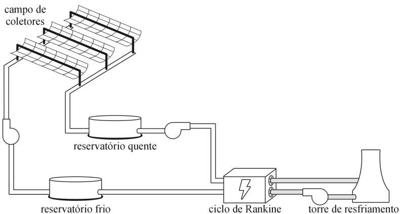
Figura 6.2: Disposição dos componentes na configuração B.
