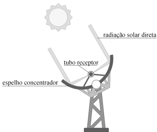
Figura 1.2: Concentração e absorção da radiação em uma calha parabólica.
