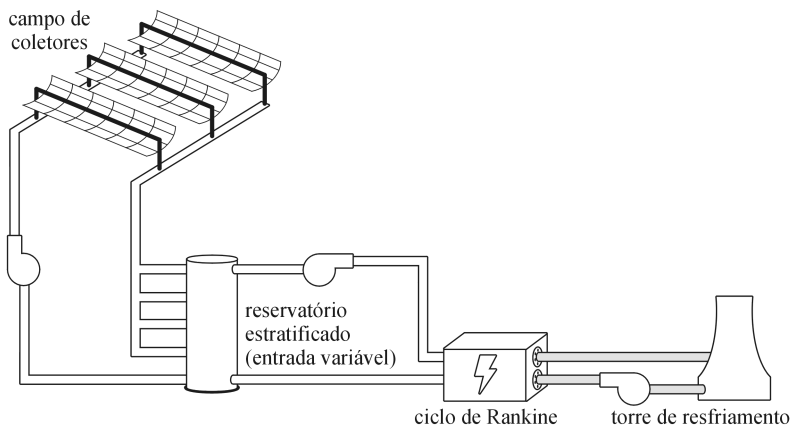
Figura 6.4: Disposição dos componentes na configuração D.
