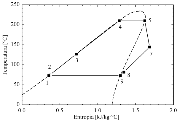
Figura 4.6: Representação do ciclo sem superaquecimento no diagrama T-s para o n-hexano como fluido de trabalho.
