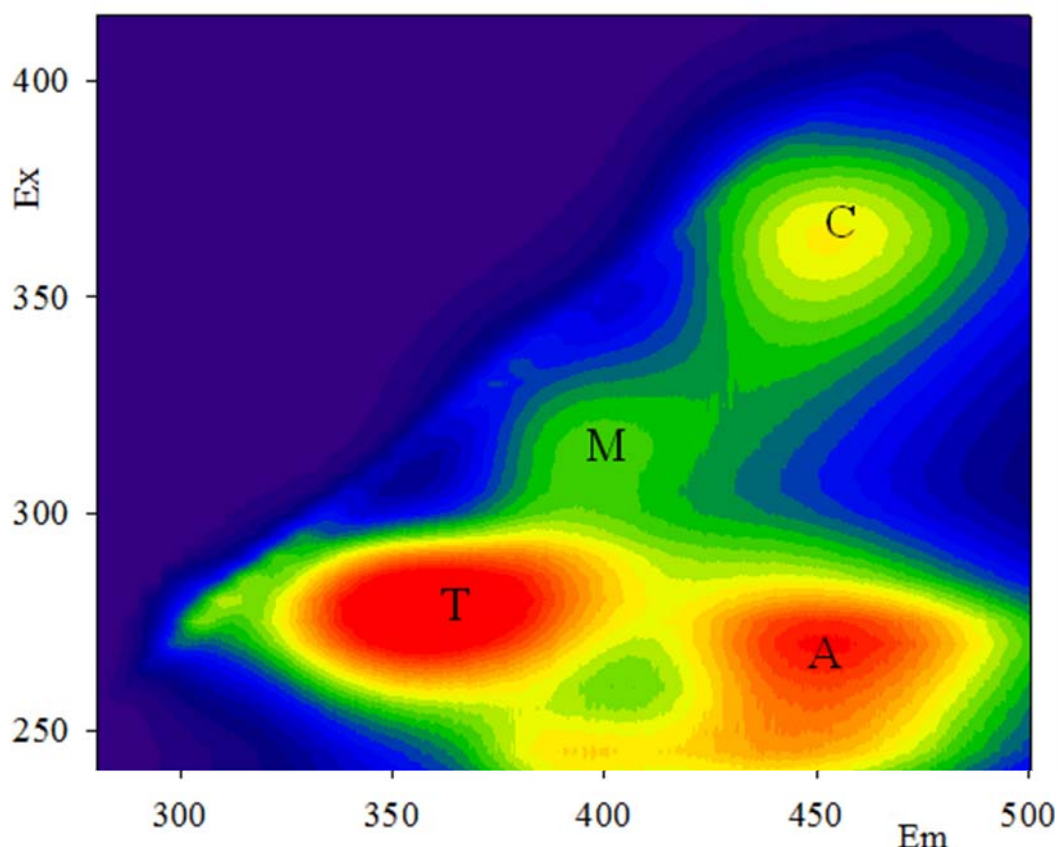
Figura 1. Exemplo de EEM (MOD-F extracelular da cultura de Microcystis aeruginosa ) e localização dos fluoróforos identificados neste estudo. T = material protéico; A = material húmico, C = material húmico de origem terrestre, e pico M.
