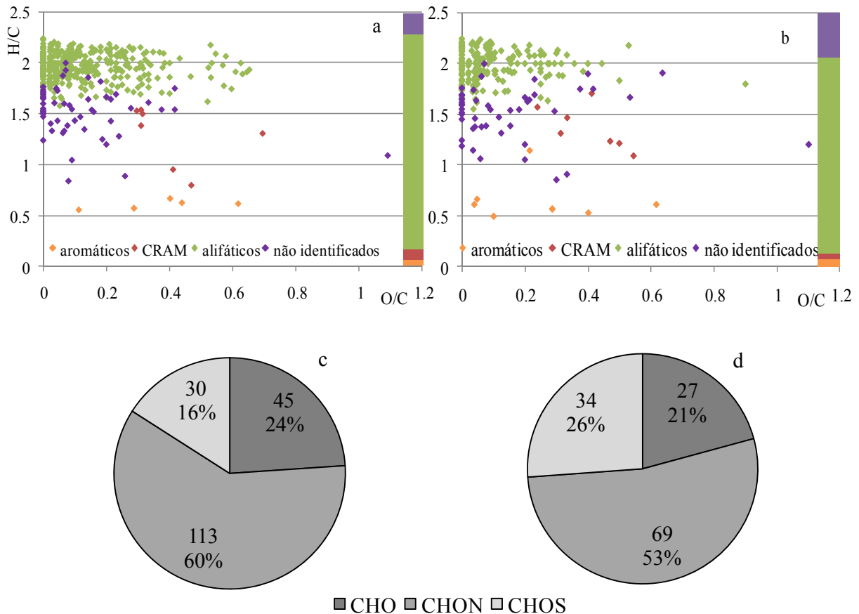
Figura 20. Composição química dos bioprodutos da atividade biológica sobre a MOD extracelular inicial (painéis a e c) e pré irradiada (painéis b e d) de Microcystis aeruginosa : (a e b) diagrama de Van Krevelen e classes estruturais, onde a barra representa a contribuição proporcional de cada classe, e (c e d) composição atômica em número e proporção (%).
