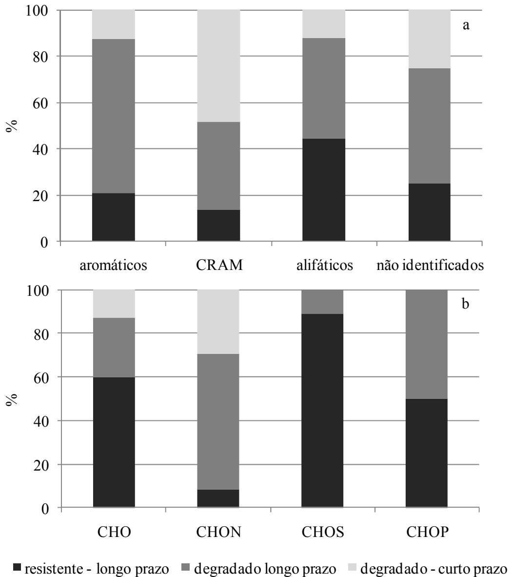
Figura 10. Proporção (%) de compostos resistentes a longo prazo (7 dias) e degradados em curto (0.5 dia) e longo prazo (7 dias), pertencentes às diversas classes (a) estruturais e (b) de composição atômica da MOD extracelular de Microcystis aeruginosa exposta à radiação UVB.
