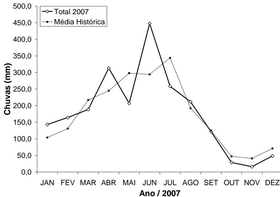
Figura 4. Total de chuvas (mm) observadas no período de janeiro a dezembro de 2007 e média histórica para região do município do Cabo de Santo Agostinho, estação meteorológica da Barragem de Suape (LAMEPE / ITEP, 2008).
