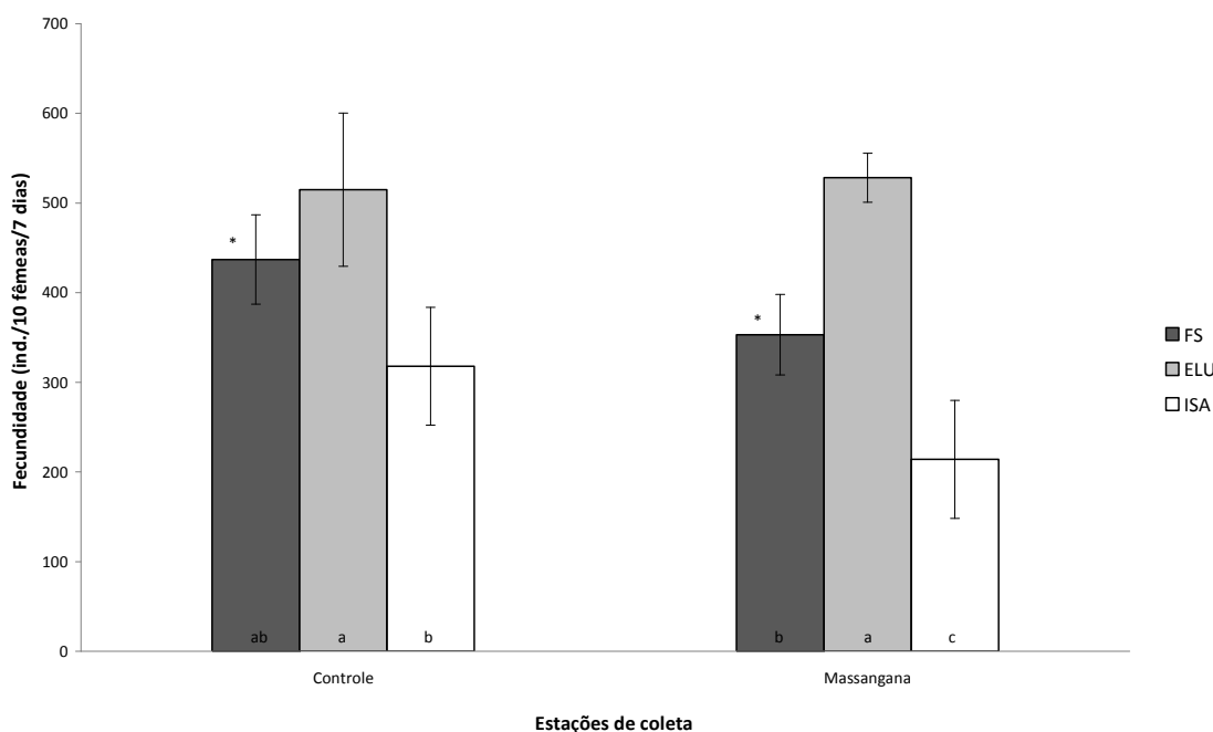
Figura 3. Média ( \pm desvio padrão) da fecundidade no experimento de outubro de 2007. a, b e c = diferenças encontradas pelo teste de Tukey entre as metodologias dentro de cada estação de coleta. * = diferenças encontradas pelo teste de Tukey entre as estações de coleta. FS = fase sólida; ELU = elutriato e ISA = interface sedimento/água.
