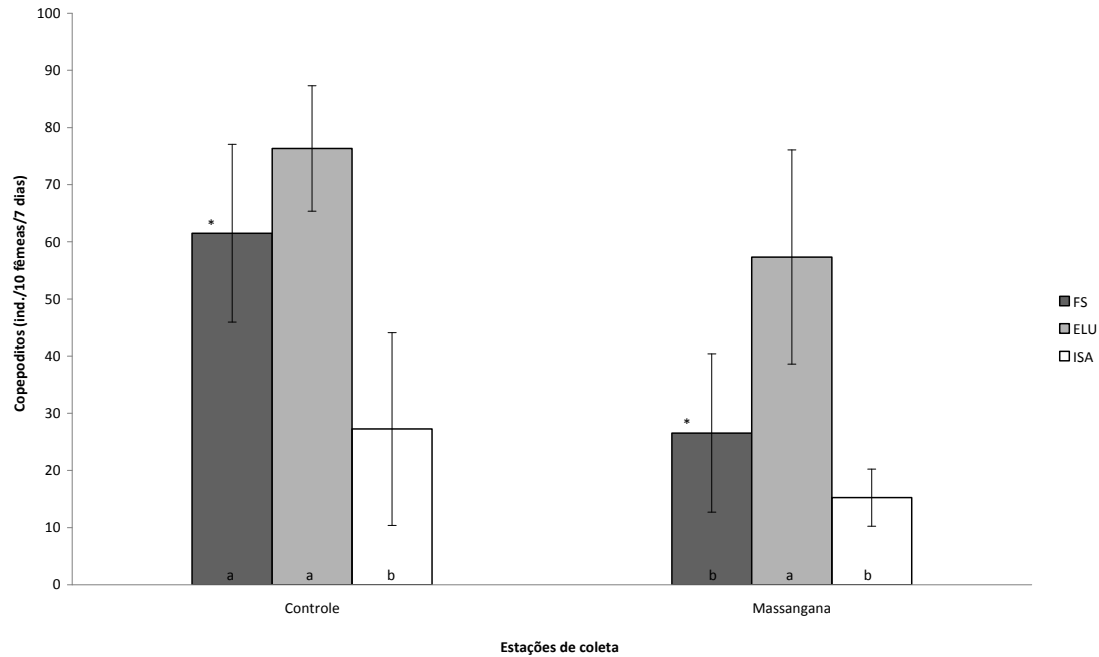
Figura 7. Média ( \pm desvio padrão) do número de copepoditos na prole no experimento de dezembro de 2007. a e b = diferenças encontradas pelo teste de Tukey dentro de cada estação de coleta. * = diferenças encontradas pelo teste de Tukey entre as estações de coleta. FS = fase sólida; ELU = elutriato e ISA = interface sedimento/água.
