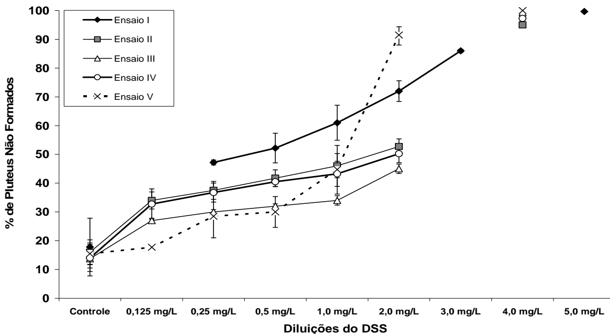
Figura 5. Média ( \pm desvio padrão) do percentual de pluteus não formados de L. variegatus em função da concentração de Dodecil Sulfato de Sódio - C_{12}H_{25}NaO_4S (DSS) em cada um dos 5 bioensaios realizados. Ensaio I = Ensaio Preliminar; Ensaio II = Maio/2007; Ensaio III = Agosto/2007; Ensaio IV = Outubro/2007 e Ensaio V = Dezembro/2007.
