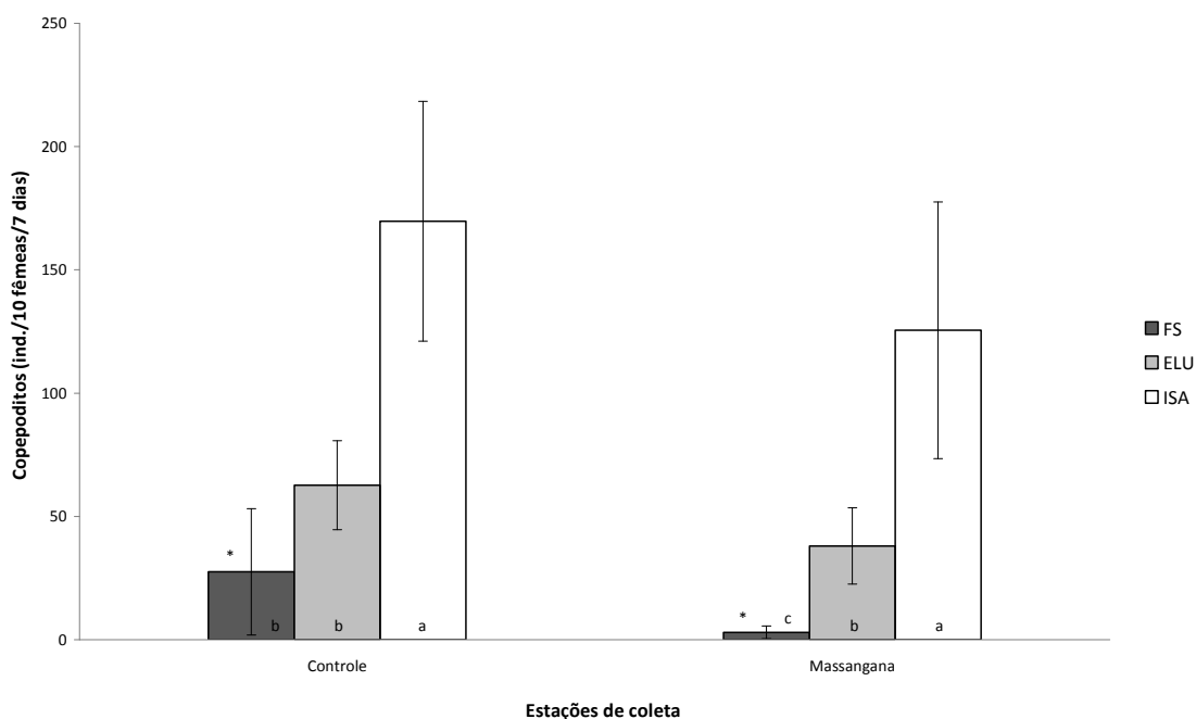
Figura 4. Média ( \pm desvio padrão) do número de copepoditos na prole no experimento de outubro de 2007. a, b e c = diferenças encontradas pelo teste de Tukey dentro de cada estação de coleta. * = diferenças encontradas pelo teste de Tukey entre as estações de coleta. FS = fase sólida; ELU = elutriato e ISA = interface sedimento/água.
