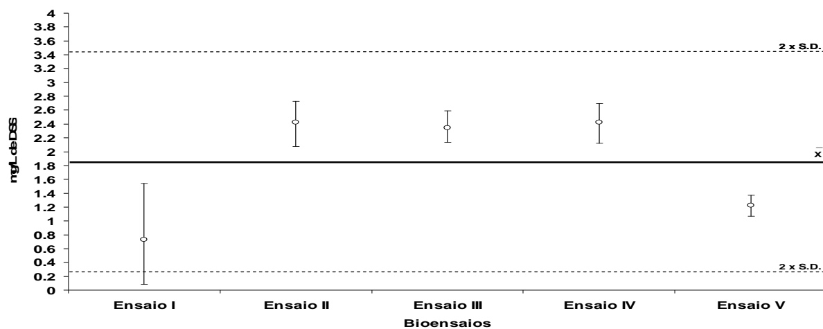
Figura 6. Valores ( \pm desvio padrão) da CE_{50} em mg/L do Dodecil Sulfato de Sódio - C_{12}H_{25}NaO_4S (DSS) após 28 horas em cada um dos 5 bioensaios com L. variegatus coletados em Muro Alto – PE, Brasil.
