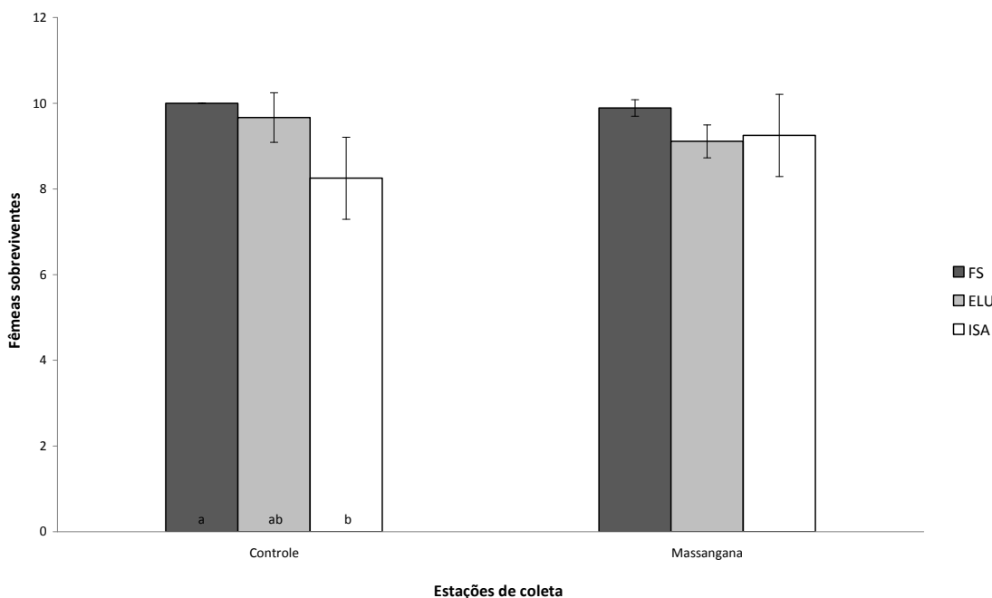
Figura 2. Média ( \pm desvio padrão) do total de fêmeas vivas ao final do experimento de outubro de 2007. a e b = diferenças encontradas pelo teste de Tukey na estação controle. FS = fase sólida; ELU = elutriato e ISA = interface sedimento/água.
