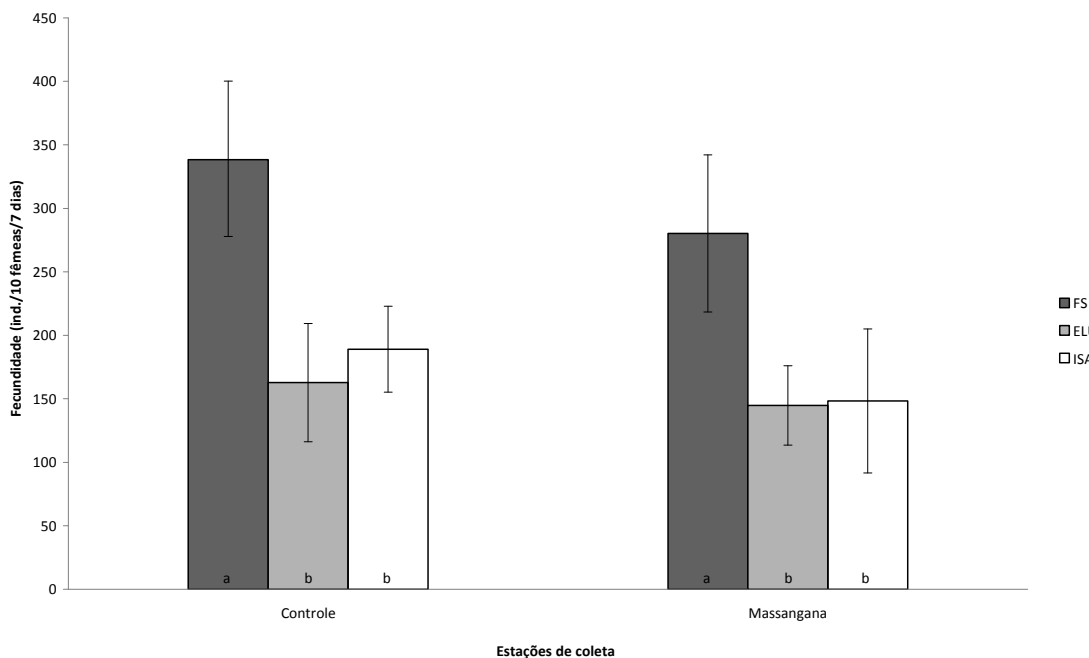
Figura 6. Média ( \pm desvio padrão) da fecundidade no experimento de dezembro de 2007. a e b = diferenças encontradas pelo teste de Tukey entre as metodologias dentro de cada estação de coleta. FS = fase sólida; ELU = elutriato e ISA = interface sedimento/água.
