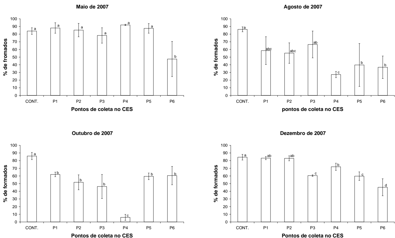
Figura 7. Média ( \pm desvio padrão) do percentual de pluteus formados de L. variegatus no controle e nos pontos de coleta em cada um dos meses de ensaios. As letras a, b e c mostram as diferenças significativas ( p < 0,05 ) no teste de Tukey.
