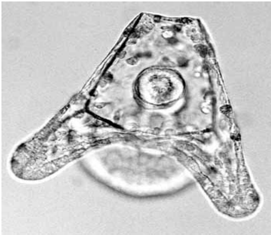
Figura 3. Pluteus recém formado no momento do encerramento do teste (CETESB, 1999).
