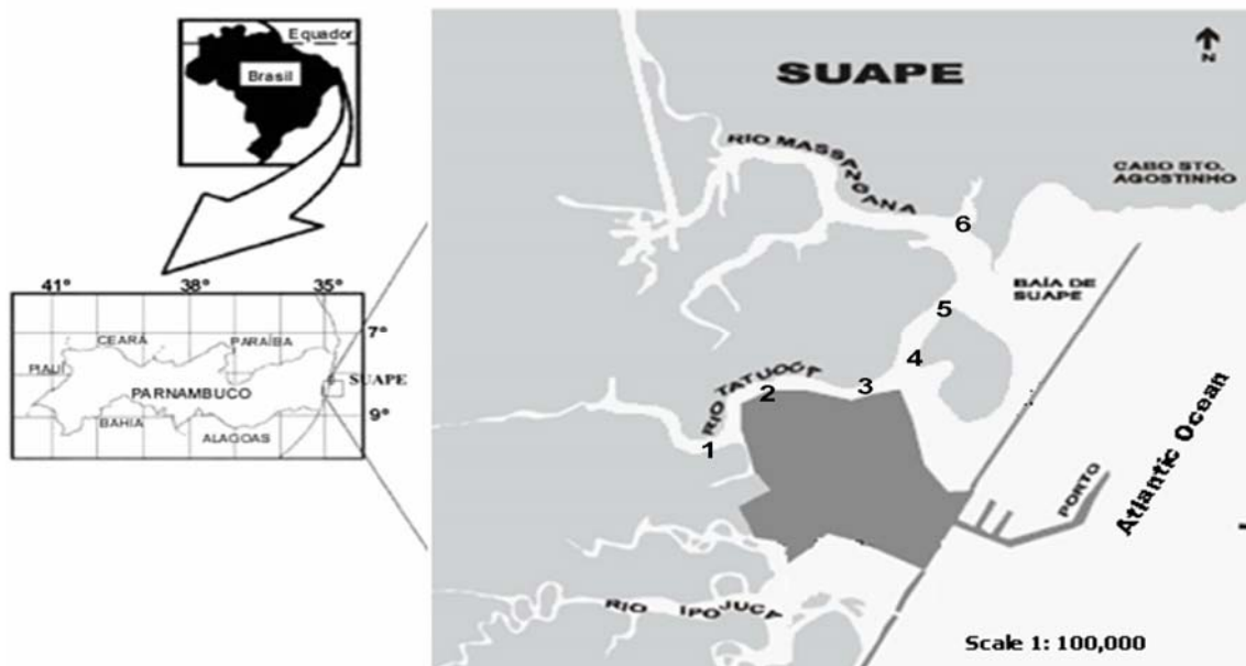
Figura 1. Área estudada e pontos de coleta. Estuários dos rios Tatuoca e Massangana. Adaptado de Koenig et al. , 2003.
