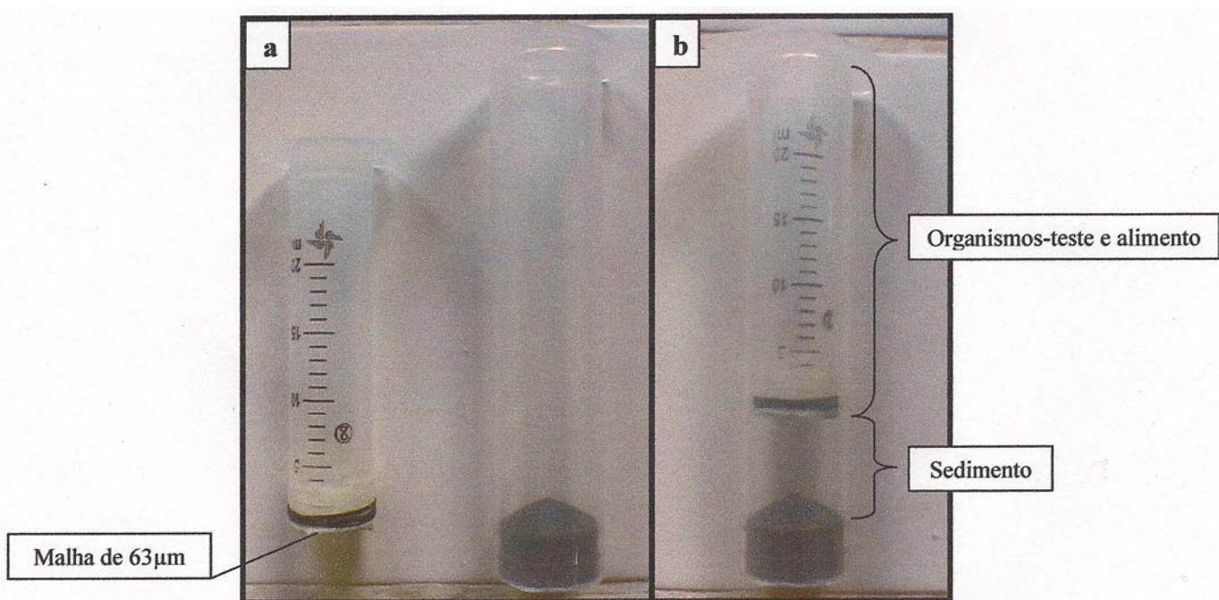
Figura 1. Foto dos recipientes utilizados na metodologia da interface sedimento/água. a) Recipientes de 20 e 60 ml e b) Recipiente de 20 ml, inserido no de 60 ml.
