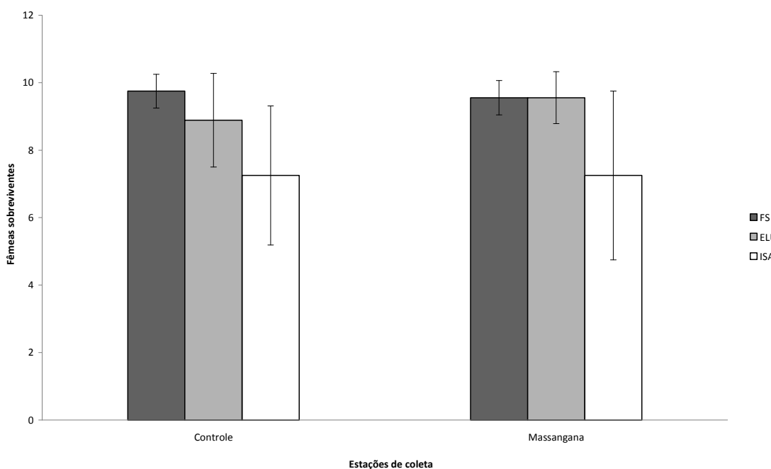
Figura 5. Média ( \pm desvio padrão) do total de fêmeas vivas ao final do experimento de dezembro de 2007. FS = fase sólida; ELU = elutriato e ISA = interface sedimento/água.
