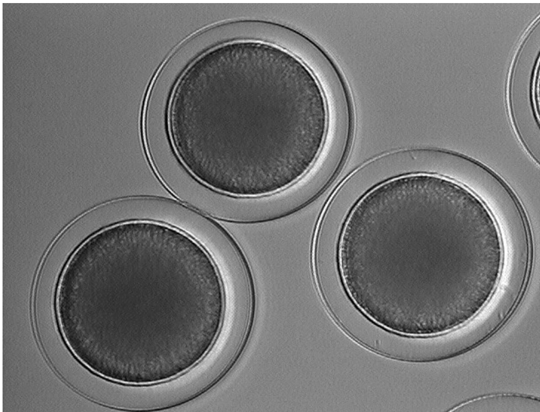
Figura 2. Ovos fertilizados, com destaque da membrana de fertilização (ABNT, 2006).
