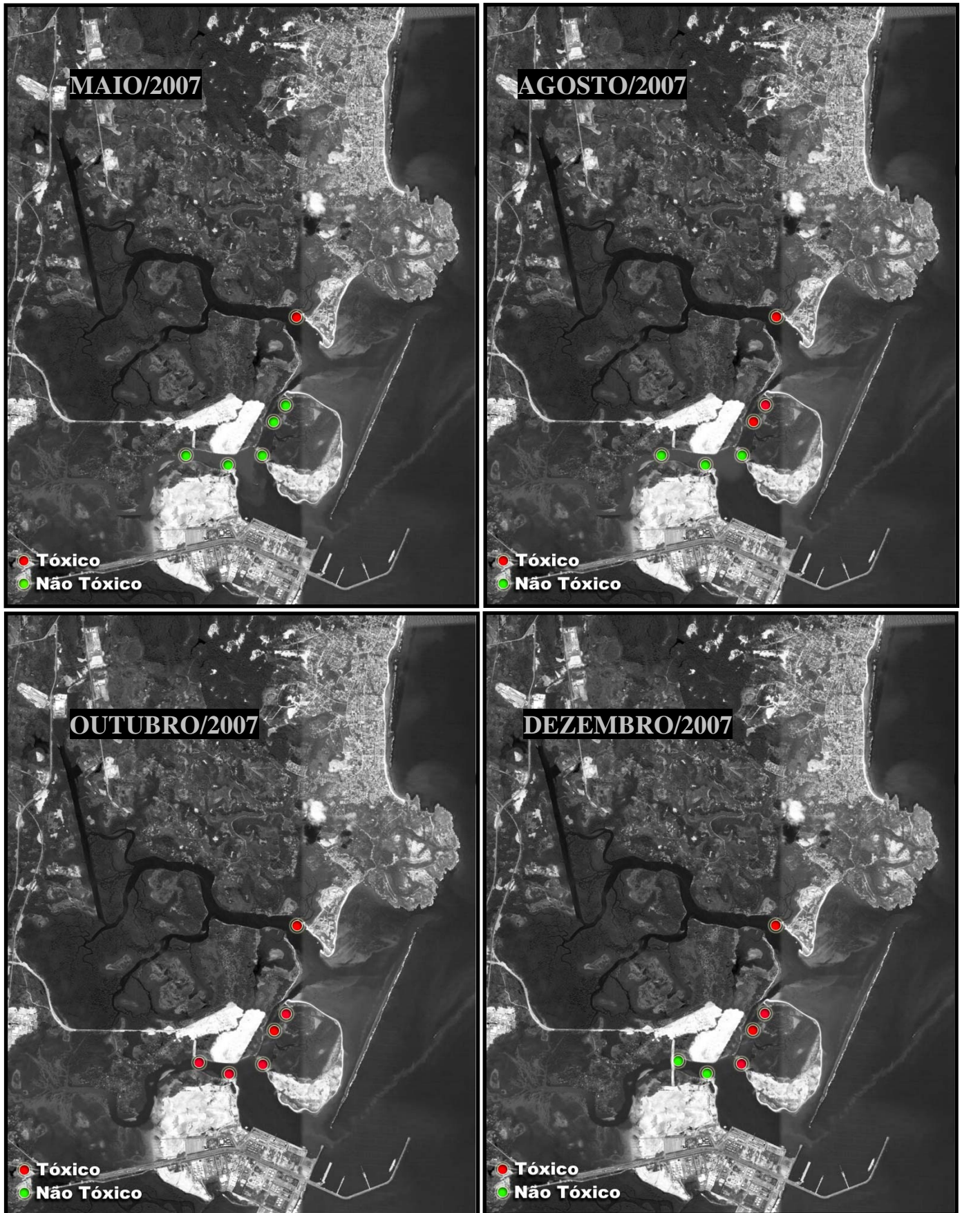
Figura 8. Imagem aérea da região mostrando a variação da toxicidade no mês de maio; agosto; outubro e dezembro de 2007. Pontos vermelhos = Tóxico; Pontos verdes = Não Tóxico.
