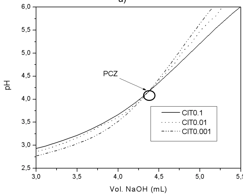
Figura 9: a) curvas de titulação do CIT com três concentrações de eletrólito; b) ampliação das curvas evidenciando o ponto de cruzamento entre elas.
