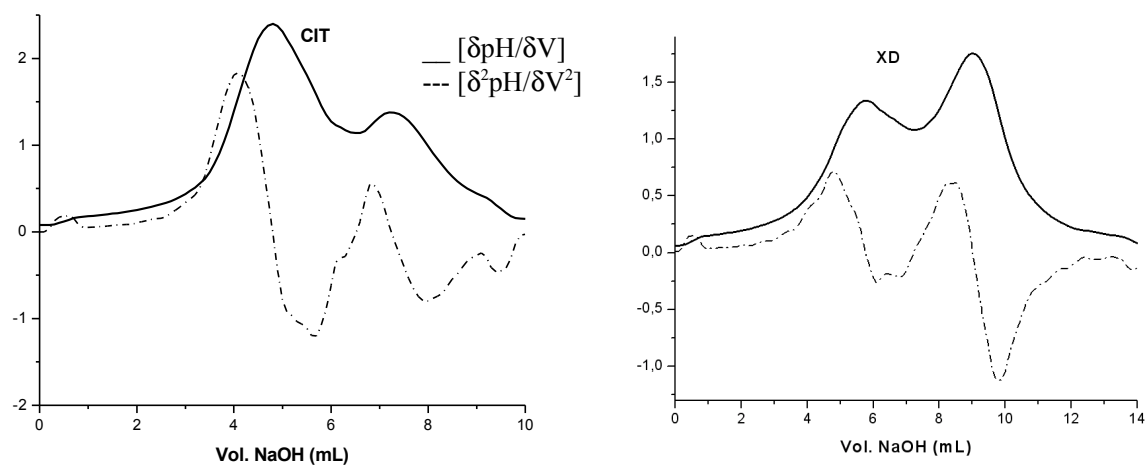
Figura 7: a) curvas de titulação dos materiais CIT e XD; b) curvas da primeira derivada (linha cheia) e segunda derivada (linha tracejada) de ambas as titulações de ambos os materiais.
