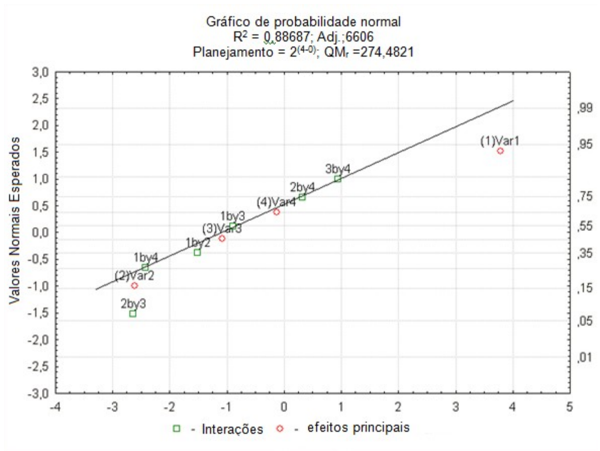
Figura 16: gráfico de probabilidade normal
