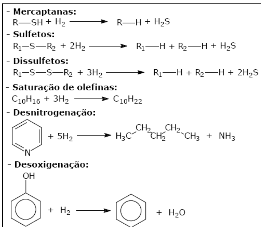
Figura 3: Processos comuns de hidrogenação em processo de hidrotreatamento
