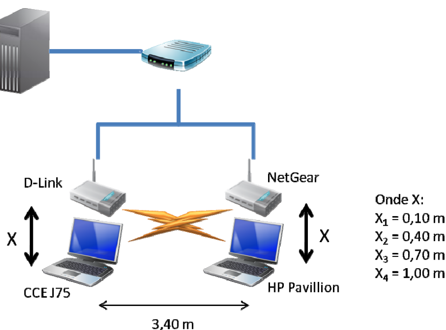
Figura 4.6 - Diagrama da medida com variação de distância.
