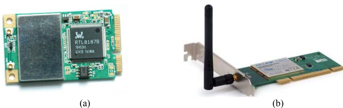
Figura 1.3 - (a) Placa para comunicação WiFi com chip RTL8187, sem antena, com 48x30mm, e interface USB. (b) Placa TP-Link TL-WN353GD, com antena, interface PCI.
