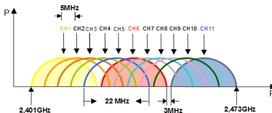
Figura 2.6 - Distribuição dos canais de transmissão para o padrão 802.11g, de acordo com a FCC (Modificado de [11]).
