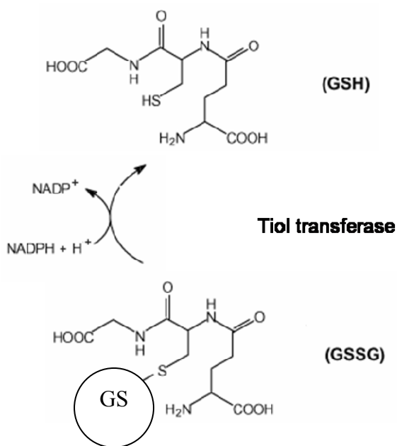
Figura 3: Reação catalizada pela enzima Tiol transferase.
