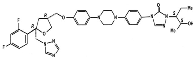
Figura 6 – Estrutura química do Posaconazol.
