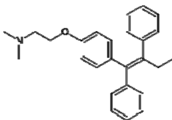
Figura 9: Estrutura química do Tamoxifeno.
