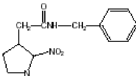
Figura 2 – Estrutura química do Benznidazol.
