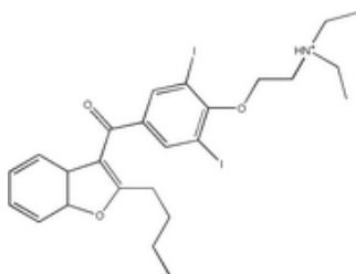
Figura 8 – Estrutura química da Amiodarona.
