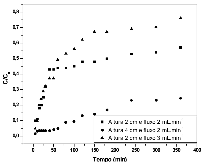
Figura 18: Curva de ruptura para adsorção dos TTHM em humina imobilizada em silicato de sódio. Condições: (razão do fluxo = 2 e 3 mL.min -1 , altura do leito = 2 e 4 cm respectivamente, temperatura = 25 \pm 0, 1^\circ\text{C} ).
