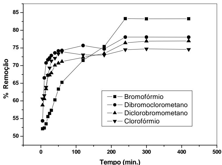
Figura 12: Efeito do tempo de contato na adsorção dos THM. Condições: Concentração inicial de 250,0 \mu\text{g. L}^{-1} , 0,1\text{g} de humina, temperatura de 25 \pm 0,2^\circ\text{C} e tempo de contato de 420 \text{ min} .
