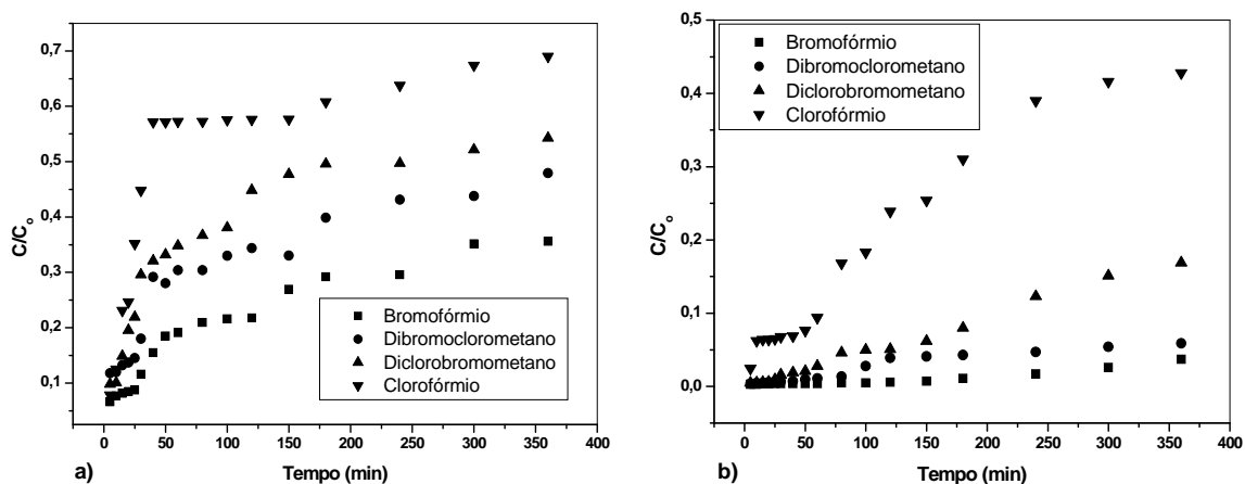
Figura 17: Curva de ruptura para adsorção dos THM em humina immobilizada em sílicato de sódio. Condições: (razão do fluxo = 2 \text{ mL}\cdot\text{min}^{-1} , altura do leito (a e b) = 2 e 4 cm respectivamente, T = 25 \pm 0,1^\circ\text{C} ).
