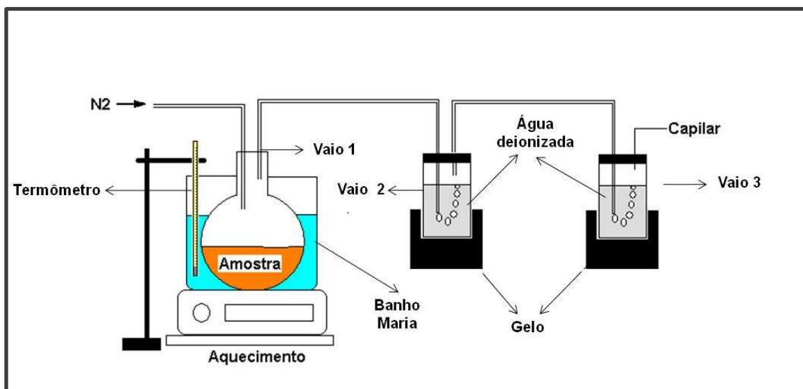
Figura 7: Esquema do sistema de dessorção térmica.
