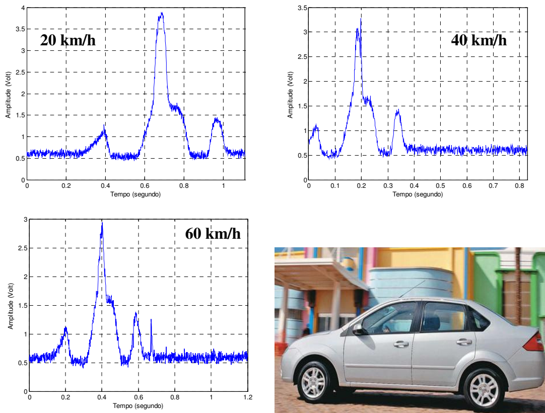
Figura 5.8. Perfis de veículo de passeio nas velocidades 20, 40 e 60 km/h (Ford Fiesta).
