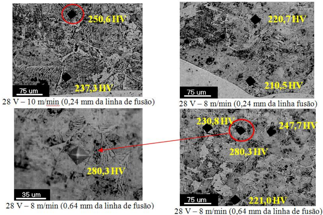
Figura 35. Microestrutura da ZTA com valores de dureza máxima.
