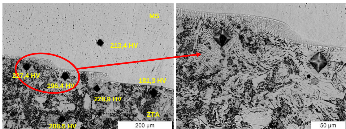
Figura 62. Microestrutura da ZTA próximo a região do 3º passe do revestimento na condição 24 V, 7 m/min, com pré-aquecimento de 423 K (150 °C) e H = 6,0 \text{ kJ/cm} .
