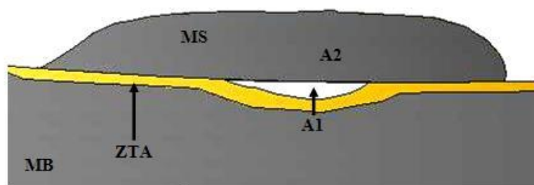
Figura 8. Apresentação esquemática da zona fundida e/ou metal de solda (A1+A2), zona termicamente afetada (ZTA), metal de base (MB) e metal de solda (MS).
