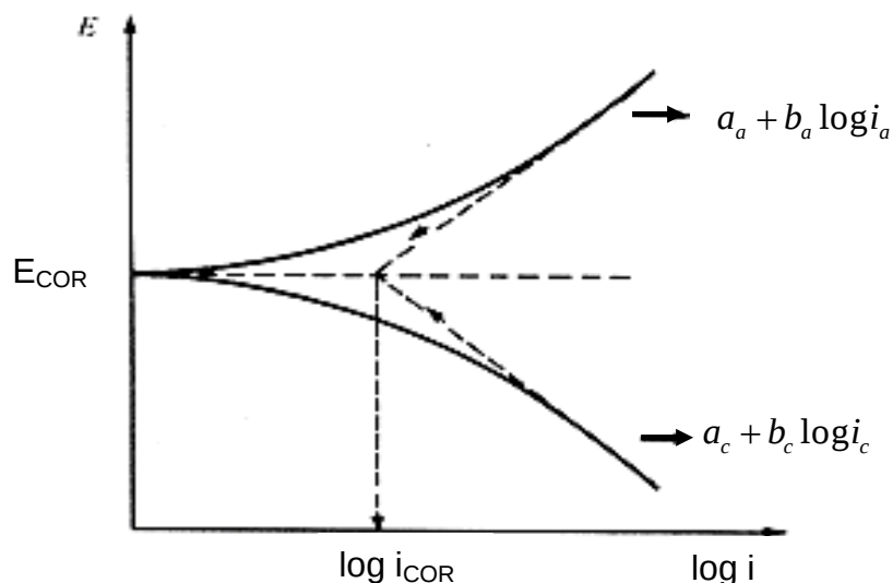
Figura 2. Representação gráfica da lei de Tafel.
