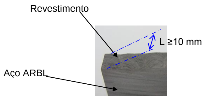
Figura 20. Corte de uma seção transversal do corpo de prova da região da solda, com largura superior a 10 mm.
