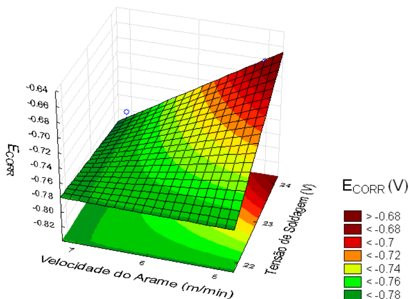
Figura 73: Superfície de resposta da tensão de soldagem vs. velocidade de alimentação do arame tendo como resposta o potencial de corrosão.
