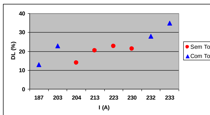
Figura 31. Relação entre a diluição longitudinal (DL), corrente de soldagem (I) e temperatura de pré-aquecimento.
