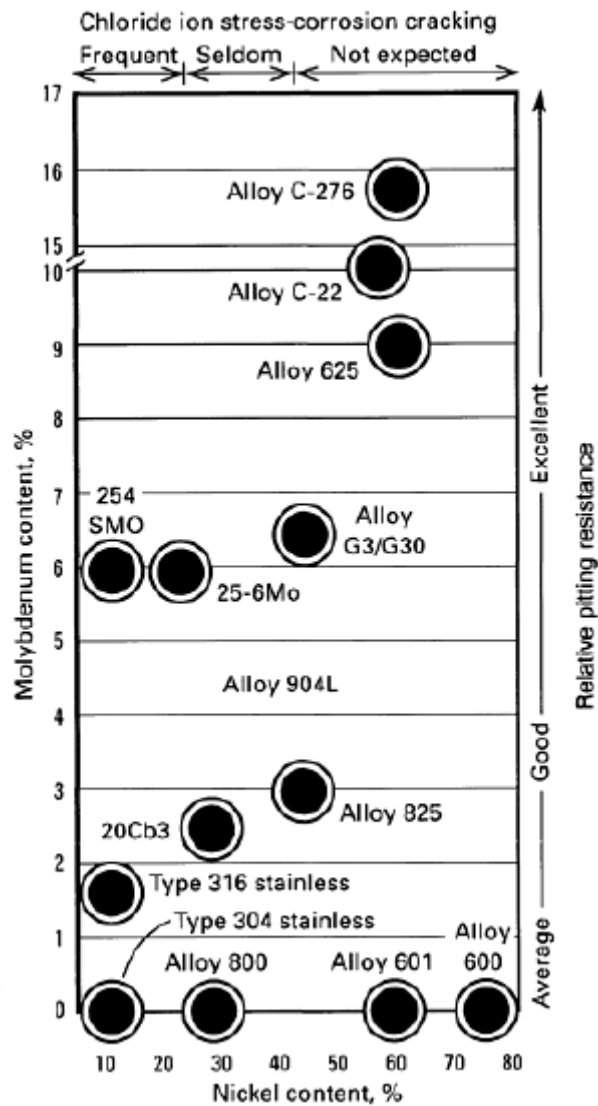
Figura 5. Efeito da porcentagem de molibdênio e níquel na resistência a corrosão de ligas comerciais selecionadas.
