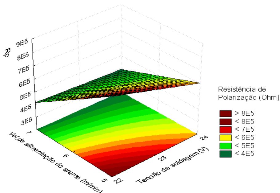
Figura 74: Superfície de resposta da tensão de soldagem vs. velocidade de alimentação do arame tendo como resposta a resistência de polarização.
