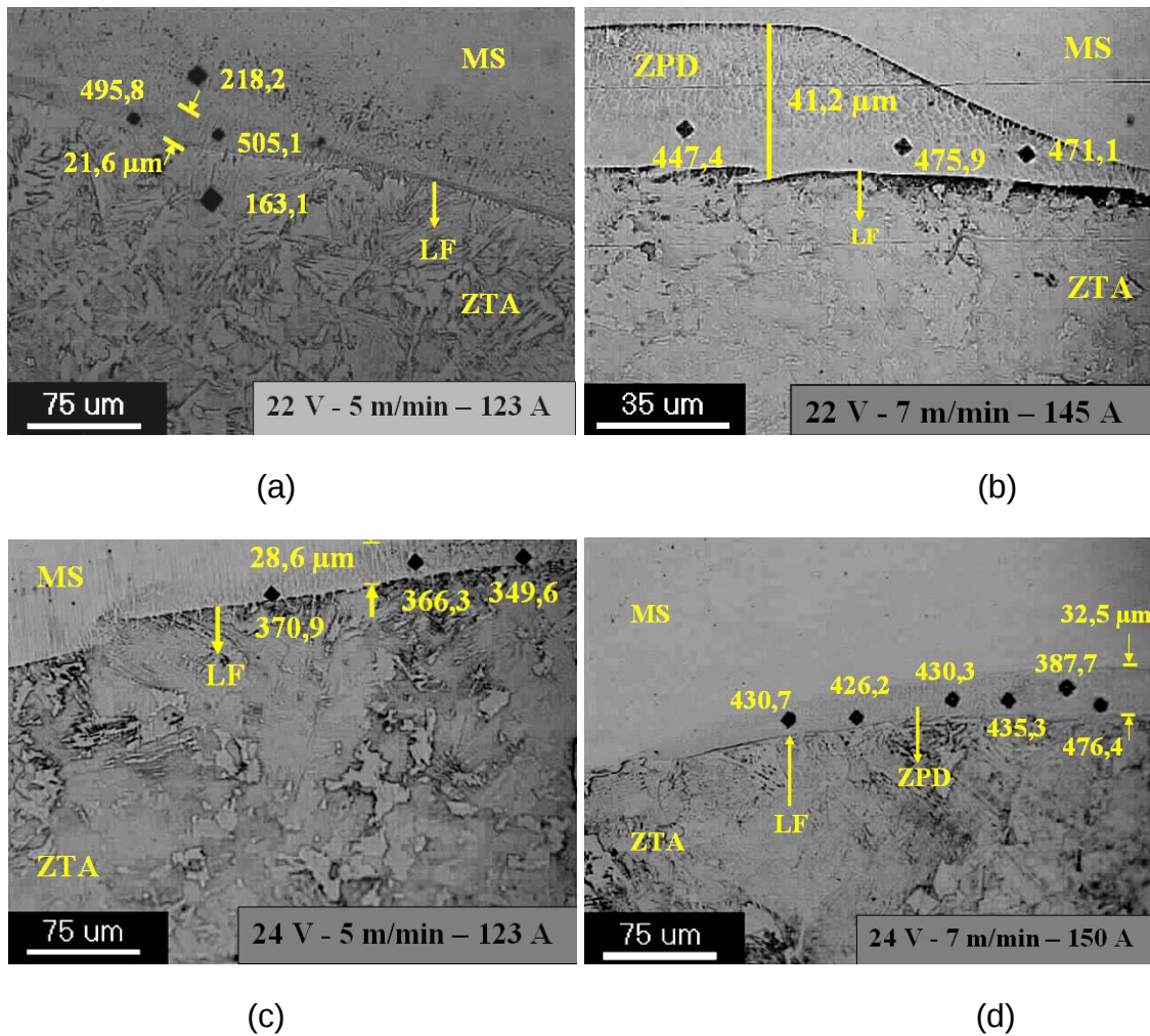
Figura 63. Interface da linha de fusão de soldas dissimilares depositadas em diferentes condições de tensão e velocidade de alimentação e sem pré-aquecimento para (a) H = 6,52 \text{ kJ/cm} , (b) H = 6,37 \text{ kJ/cm} , (c) H = 7,18 \text{ kJ/cm} e (d) H = 6,43 \text{ kJ/cm} .
