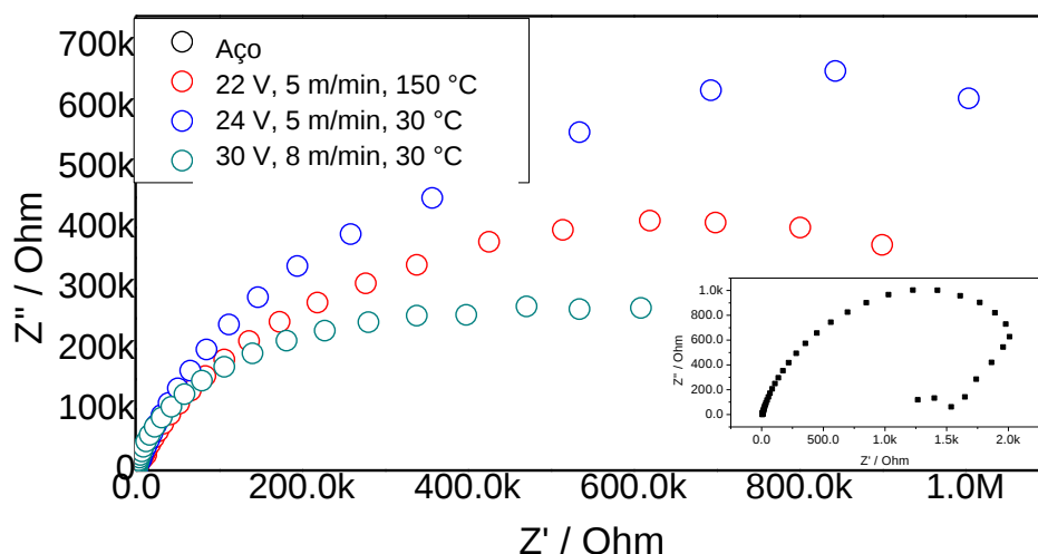
Figura 83: Diagrama de impedância relacionado aos revestimos otimizados obtidos sem e com pré-aquecimento de 423 K (150 °C), comparados com o substrato de aço carbono.
