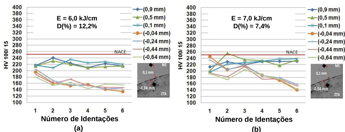
Figura 57: Perfil de microdureza ao longo do revestimento próximo a linha de fusão (interface) com tensão de 24 V, velocidade de alimentação de 5 m/mim. (a) com pré-aquecimento 423 K (150 °C) e (b) sem pré-aquecimento.
