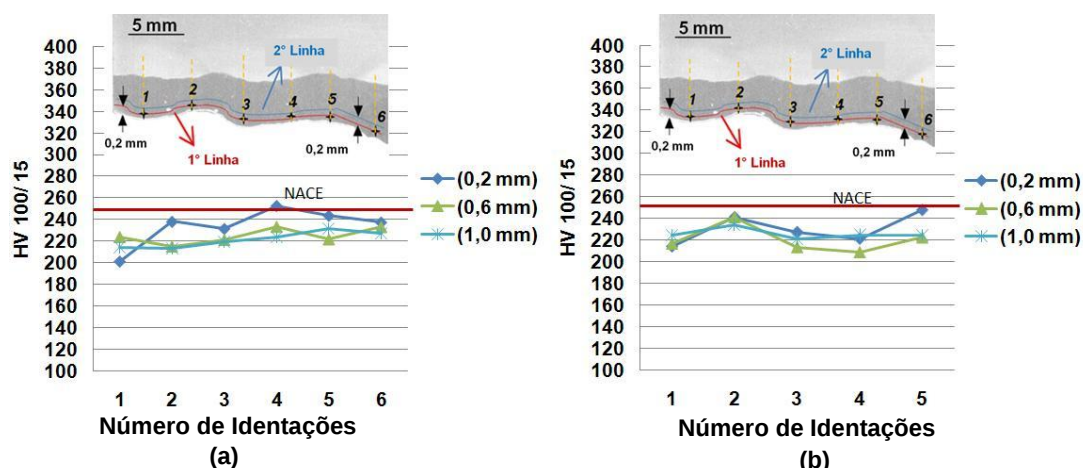
Figura 53: Perfil de microdureza próximo à superfície do revestimento com pré-aquecimento 423 K (150 °C). (a) condição 24 V, 5 m/mim. (b) condição 22 V, 5 m/min.
