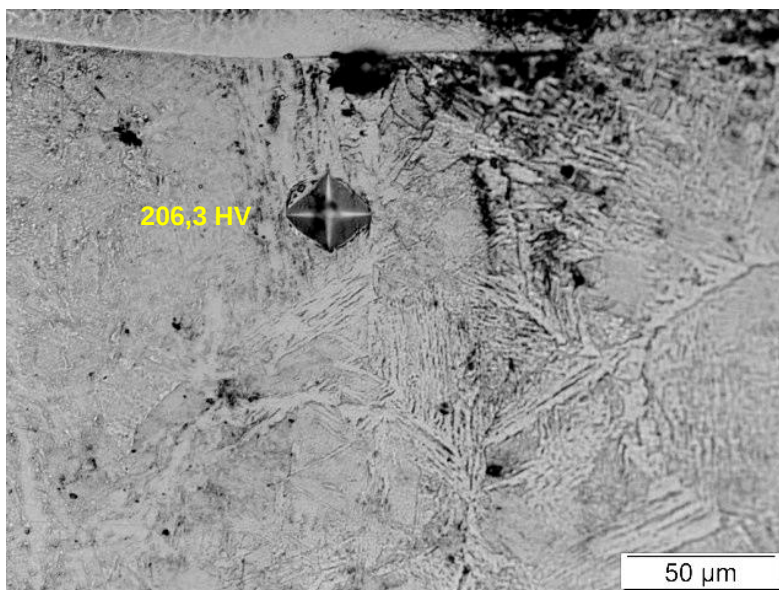
Figura 46. Microestrutura da ZTA com valores de dureza máximos. Identação número 1 a 0,04 mm da linha de fusão com pré-aquecimento na condição 22 V e 5 m/min, H = 5,6 kJ/cm.
