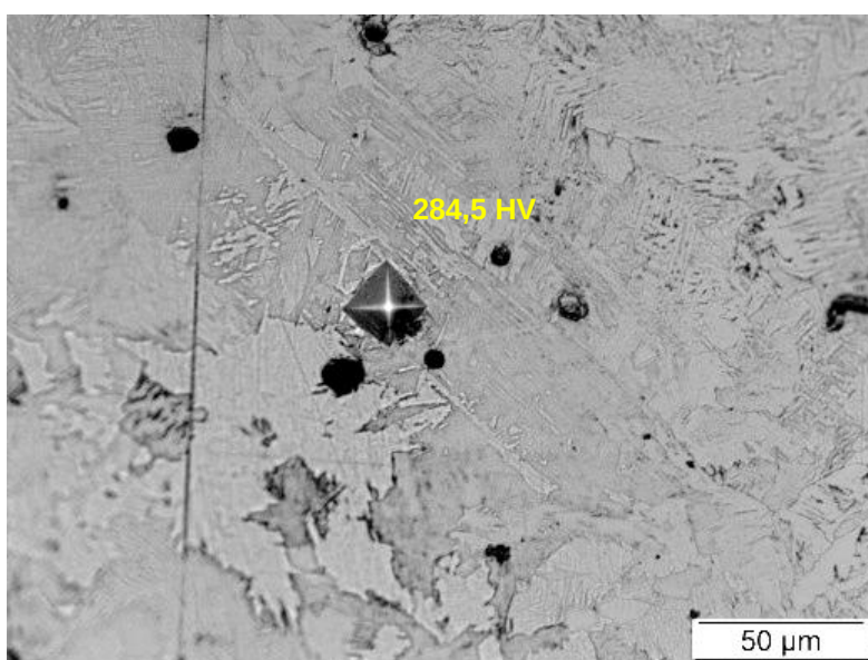
Figura 47. Microestrutura da ZTA com valores de dureza máximos. Identação número 1 com 0,24 mm da linha de fusão sem pré-aquecimento na condição 22 V e 5 m/min, H = 6,3 kJ/cm.
