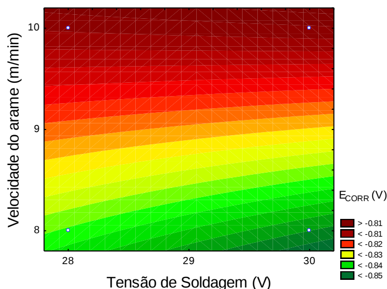
Figura 80: Superfície de resposta da tensão de soldagem vs. velocidade de alimentação do arame tendo como resposta o potencial de corrosão.
