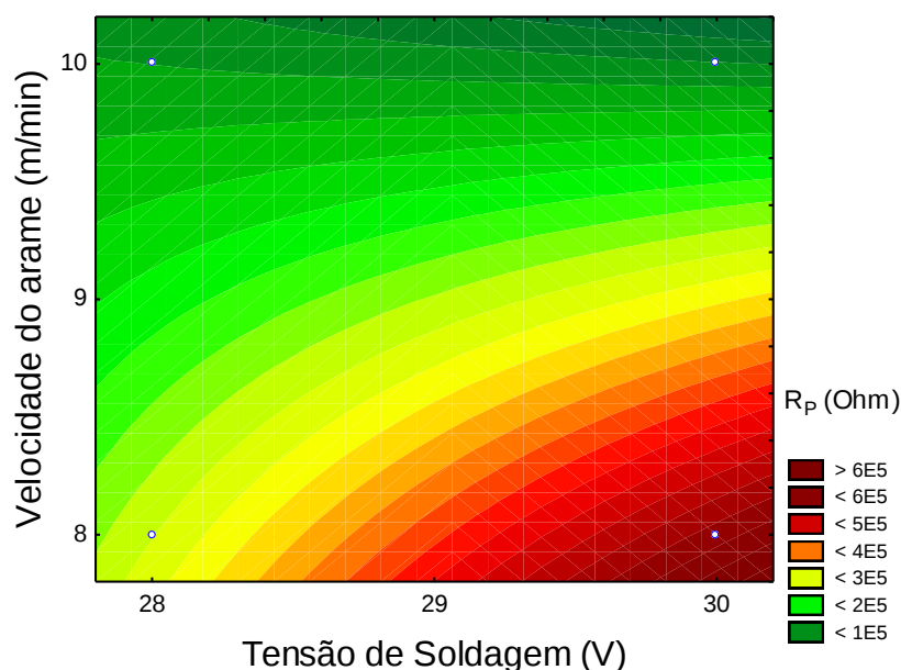
Figura 81: Superfície de resposta da tensão de soldagem vs. velocidade de alimentação do arame tendo como resposta a resistência de polarização.
