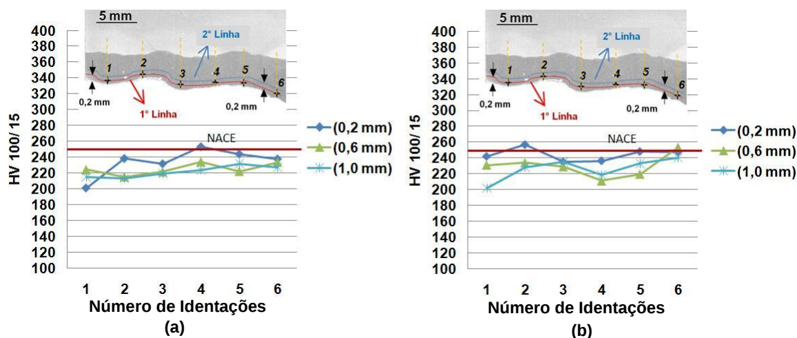
Figura 56: Perfil de microdureza próximo à superfície do revestimento com tensão de 24 V, velocidade de alimentação de 5 m/mim. (a) com pré-aquecimento 423 K (150 °C) e (b) sem pré-aquecimento.
