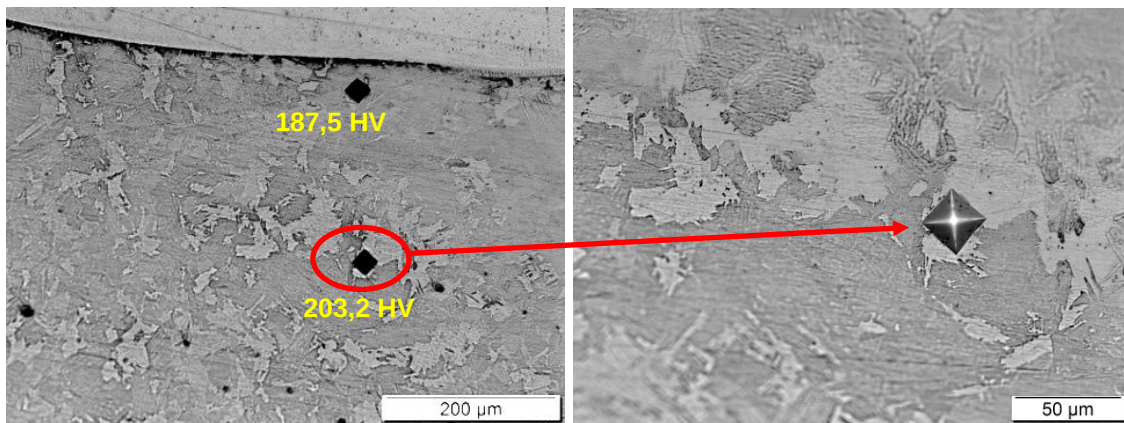
Figura 52. Microestrutura da ZTA próximo a região do 3º passe do revestimento na condição 22 V, 7 m/min e com pré-aquecimento com indentação a 0,24 mm da linha de fusão com 5,6 kJ/cm. (a).
