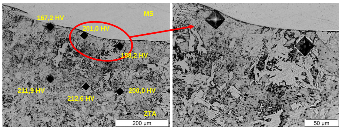
Figura 61. Microestrutura da ZTA próximo a região do 3º passe do revestimento na condição 24 V, 7 m/min, sem pré-aquecimento com H = 6,5 \text{ kJ/cm} .
