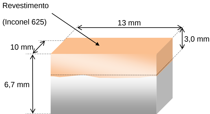
Figura 21. Desenho em perspectiva da amostra após o processo de usinagem.
