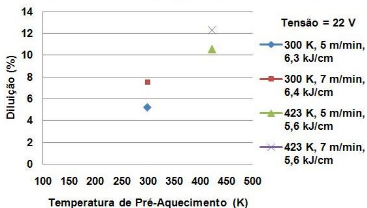
Figura 42 - Efeito do pré-aquecimento e da velocidade do arame para a condição 22 V.
