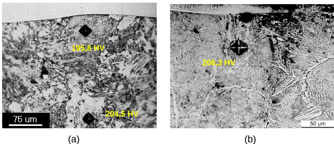
Figura 55. Microestruturas a 0,04 mm de distância da linha de fusão com pré-aquecimento de 423 K (150 °C). (a) na condição 24 V, 5 m/min, H = 6,0 kJ/cm e (b) 22 V, 5 m/min, H = 5,6 kJ/cm.
