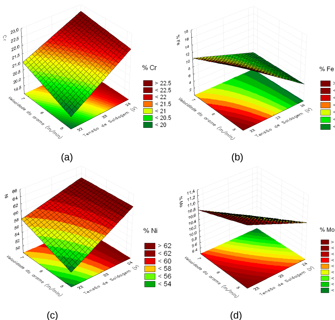
Figura 65 - Superfícies de resposta da tensão de soldagem vs. velocidade de alimentação do arame nas amostras soldadas com pré-aquecimento de 150 °C.
