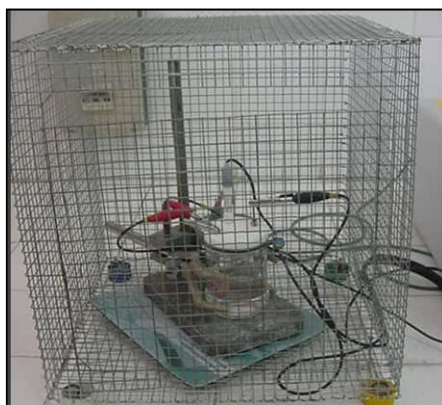
Figura 26. Gaiola de Faraday
