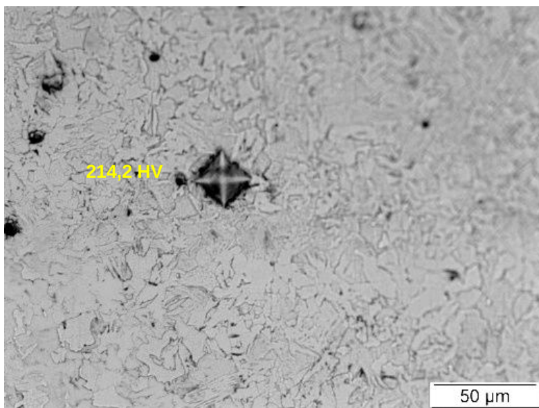
Figura 48. Microestrutura da ZTA com valores de dureza máximos. Identação número 2 com 0,24 mm da linha de fusão sem pré-aquecimento na condição 22 V e 5 m/min, H = 6,3 kJ/cm.
