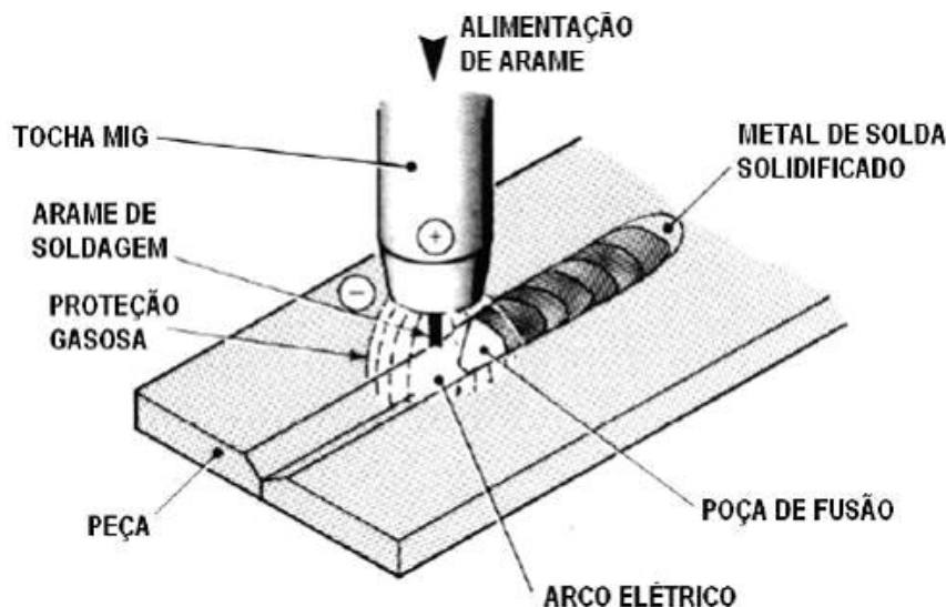
Figura 7. Processo básico de soldagem MIG/MAG.
