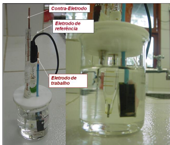
Figura 24. Célula eletroquímica de três eletrodos utilizada
