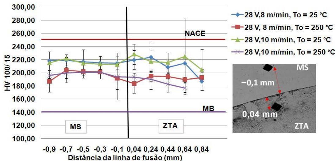
Figura 34. Perfil de microdureza ao longo do MS e ZTA na seção longitudinal.
