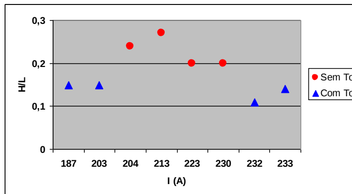
Figura 33. Relação entre altura (H) e largura (L) do cordão de solda, corrente de soldagem e temperatura de pré-aquecimento.
