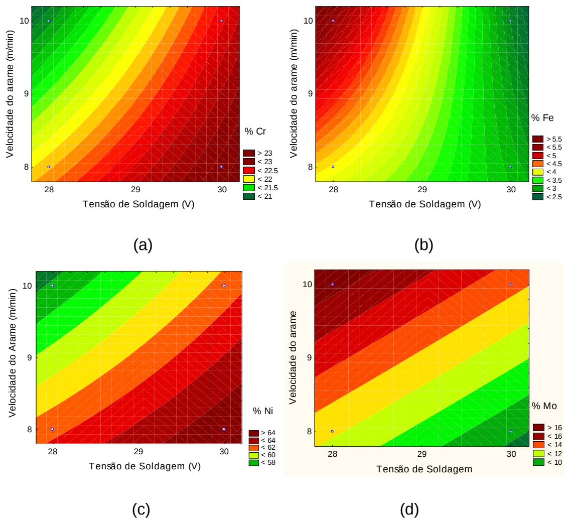
Figura 79 - Superfícies de resposta da tensão de soldagem vs. velocidade de alimentação do arame nas amostras soldadas sem pré-aquecimento. Tendo como respostas os teores de: (a) Cr (b) Fe (c) Ni (d) Mo.
