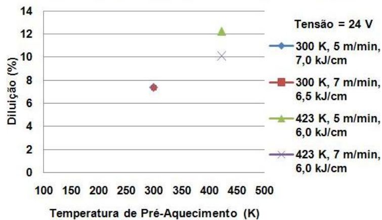
Figura 43 - Efeito do pré-aquecimento e da velocidade do arame para a condição 24 V.
