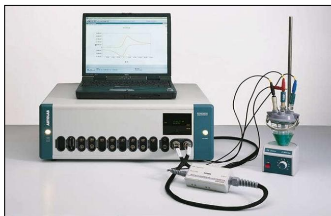
Figura 25. Potenciostato/Galvanostato PG STATE30 da Autolab
