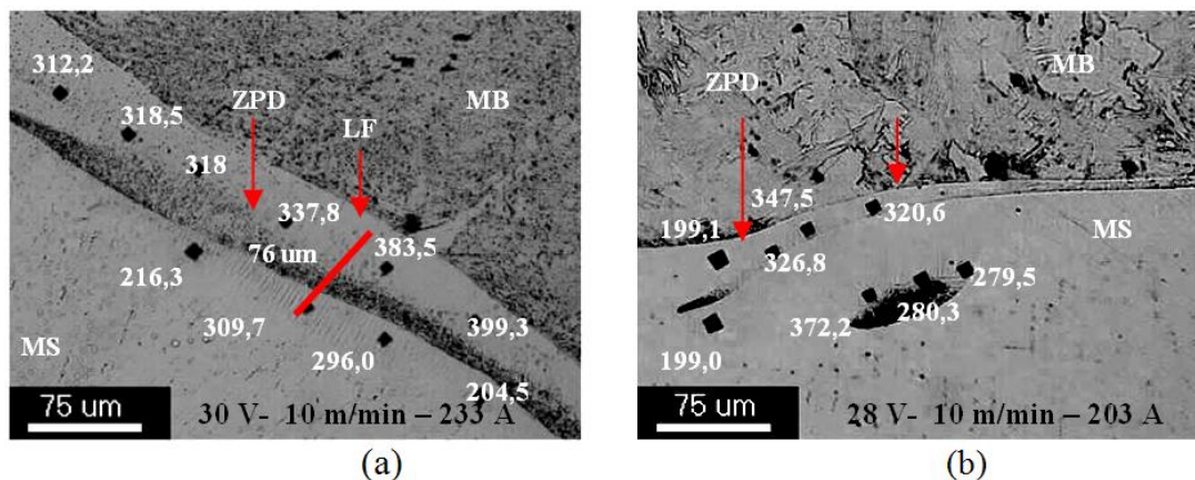
Figura 41. Interface da linha de fusão de soldas dissimilares depositadas em diferentes condições de tensão, velocidade de alimentação e pré-aquecimento T_o = 523 \text{ K} ( 250 \text{ }^{\circ}\text{C} ) para (a) H = 8,39 \text{ kJ/cm} , (b) H = 6,82 \text{ kJ/cm} .
