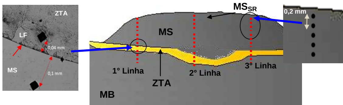
Figura 16. Desenho esquemático para o ensaio de microdureza na seção transversal.
