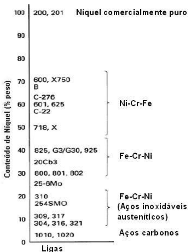
Figura 1. Agrupamento de ligas base-níquel em função do conteúdo de Ni. O conteúdo de Cr varia de 18 a 20%.
