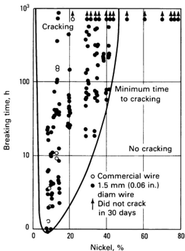
Figura 6. Efeito da adição de níquel em um aço com 17 a 24% de cromo na resistência a fissuração por corrosão sob tensão em solução de 42% de cloreto de magnésio.
