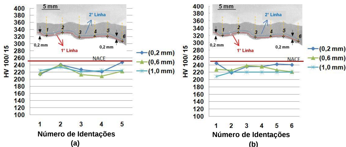
Figura 44: Perfil de microdureza próximo a superfície do revestimento com tensão de 22 V, velocidade de alimentação de 5 m/mim. (a) com pré-aquecimento 423 K (150 °C) e (b) sem pré-aquecimento.
