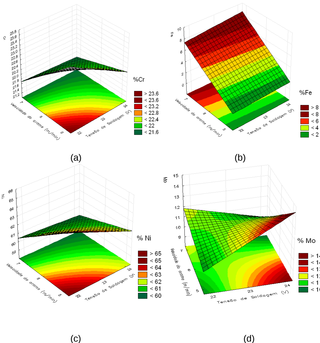
Figura 72 - Superfícies de resposta da tensão de soldagem vs. velocidade de alimentação do arame nas amostras soldadas sem pré-aquecimento. Tendo como respostas os teores de: (a) Cr (b) Fe (c) Ni (d) Mo.
