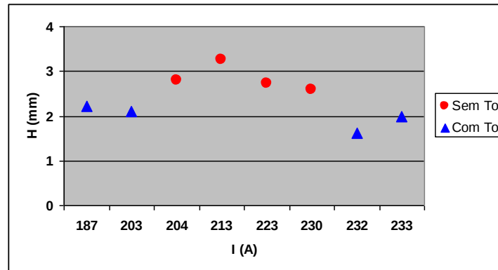
Figura 32. Relação entre a altura do cordão de solda (H), corrente de soldagem (I) e temperatura de pré-aquecimento.
