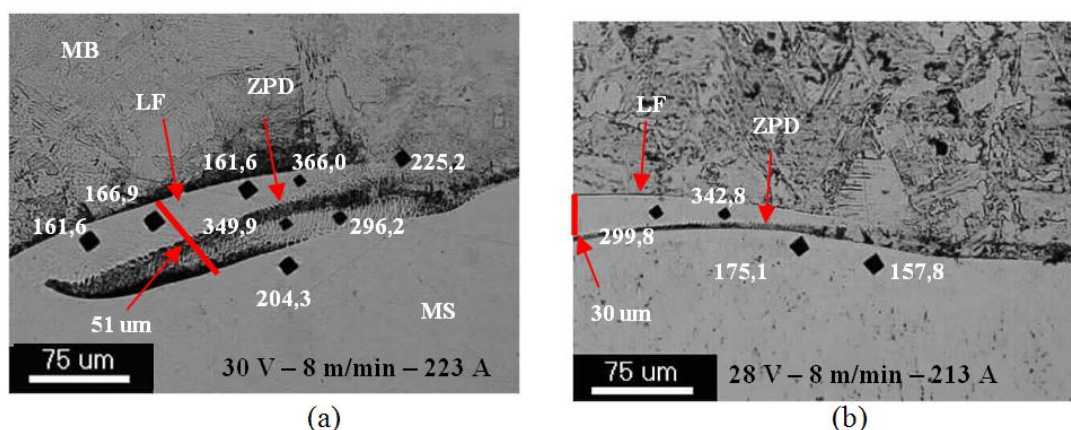
Figura 40. Interface da linha de fusão de soldas dissimilares depositadas em diferentes condições de tensão e velocidade de alimentação e sem pré-aquecimento para (a) H = 10,70 \text{ kJ/cm} e (b) H = 9,54 \text{ kJ/cm} .
