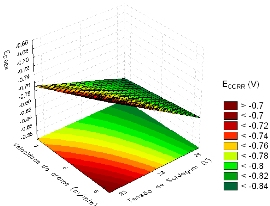
Figura 66: Superfície de resposta da tensão de soldagem vs. velocidade de alimentação do arame tendo como resposta o potencial de corrosão.
