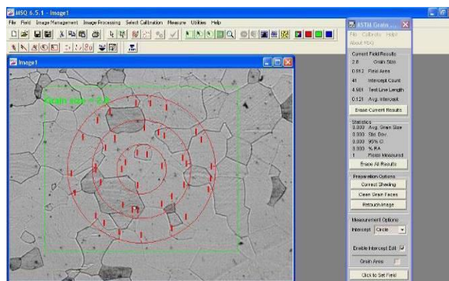
Figura 13. Analisador de imagem MSQ TM Express.
