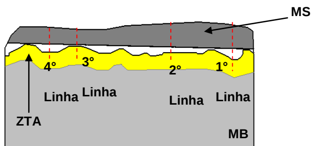
Figura 17. Desenho esquemático para o ensaio de microdureza na seção longitudinal.
