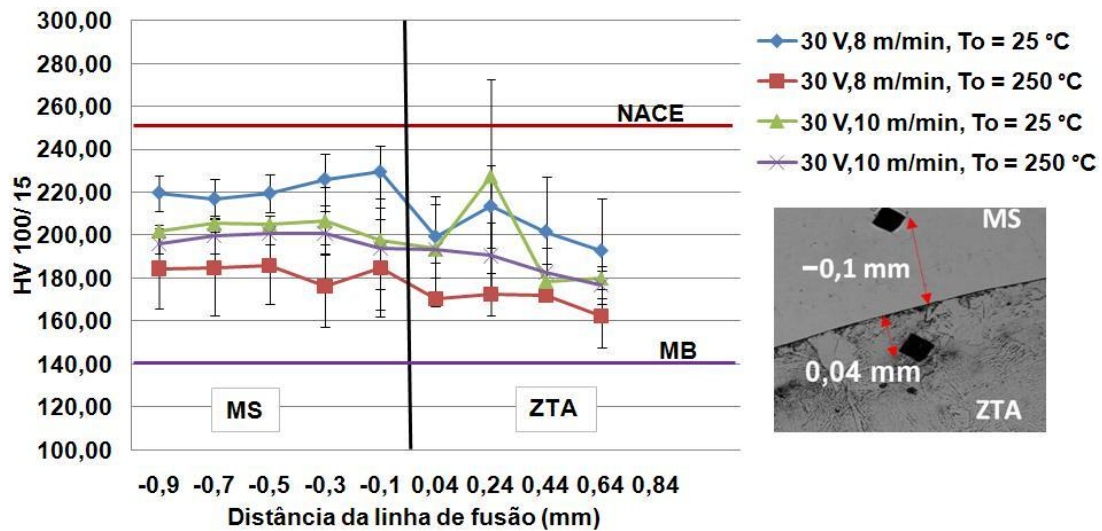
Figura 37. Perfil de microdureza ao longo do MS e ZTA para uma tensão de 30 V na seção longitudinal.
