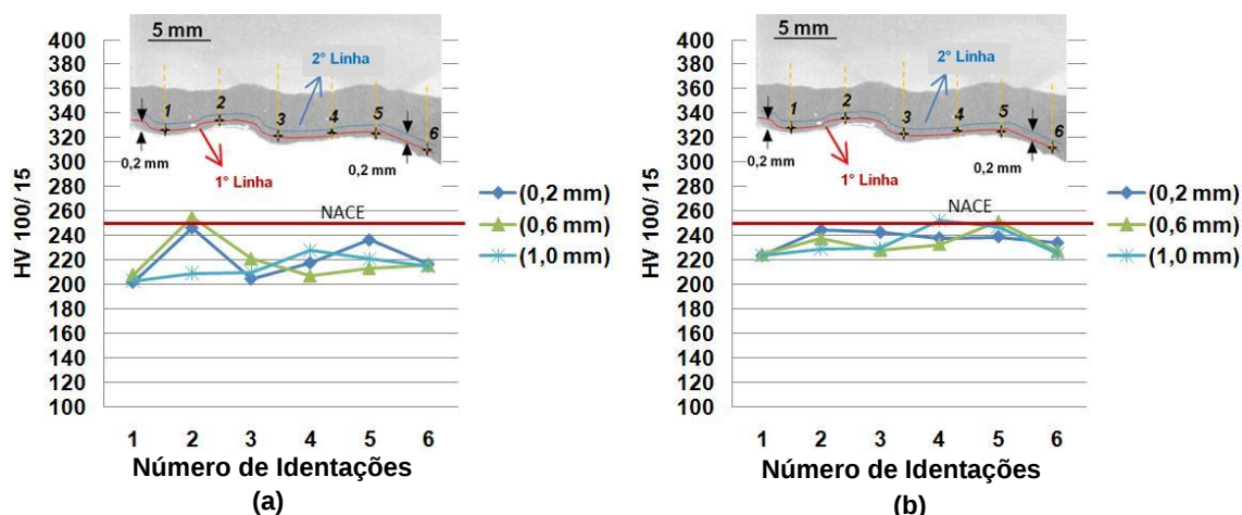
Figura 59: Perfil de microdureza próximo a superfície do revestimento com tensão de 22 V, velocidade de alimentação de 7 m/mim. (a) sem pré-aquecimento e (b) com pré-aquecimento 423 K (150 °C).
