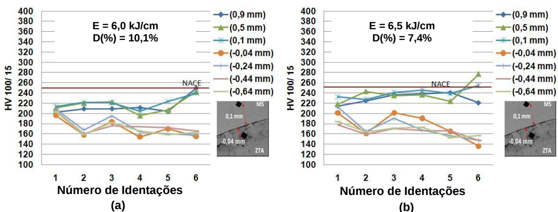
Figura 60: Perfil de microdureza ao longo do revestimento próximo a linha de fusão (interface) com tensão de 22 V, velocidade de alimentação de 7 m/mim. (a) Sem pré-aquecimento e (b) Com pré-aquecimento 423 K (150 °C).
