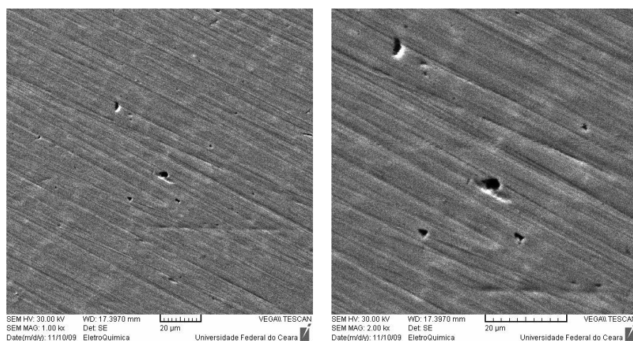
Figura 75 – Superfície de análise da amostra 22-7-S
