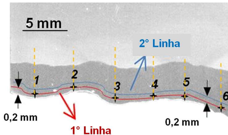
Figura 19. Ilustração das linhas de microdureza no revestimento.
