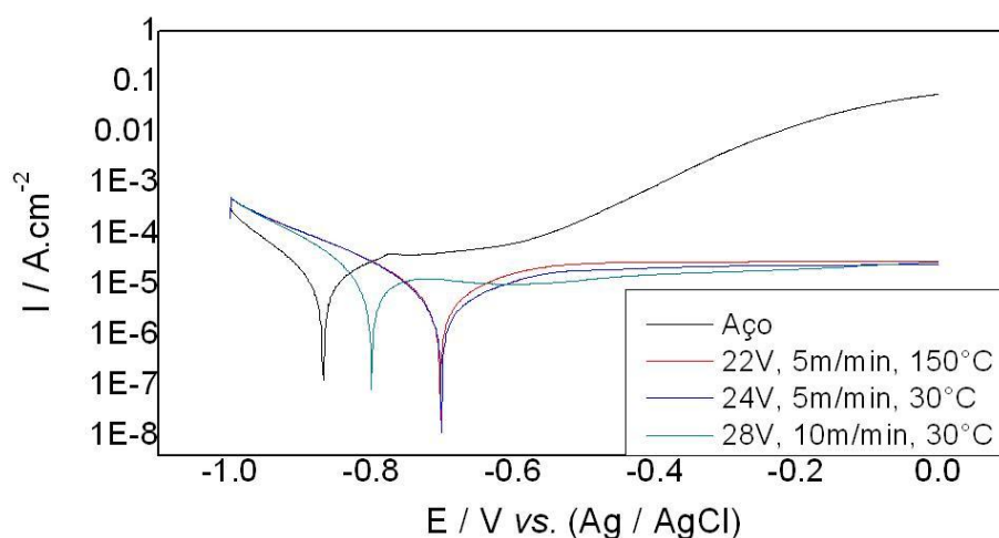
Figura 82: Curva de polarização relacionadas aos revestimos otimizados obtidos sem e com pré-aquecimento de 423 K (150 °C), comparados com o substrato de aço API 5L Gr.B.
