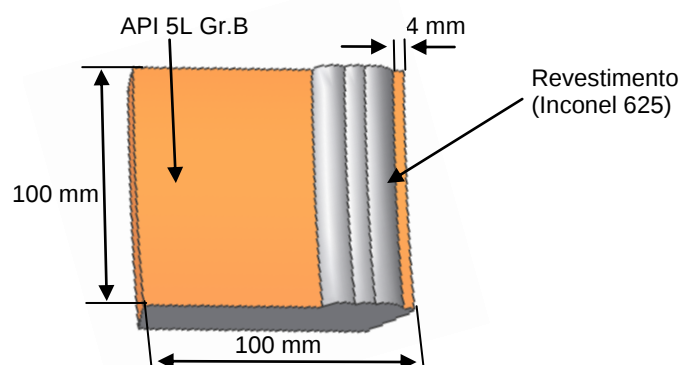
Figura 11. Corpo de prova revestido com liga Ni (Inconel 625)
