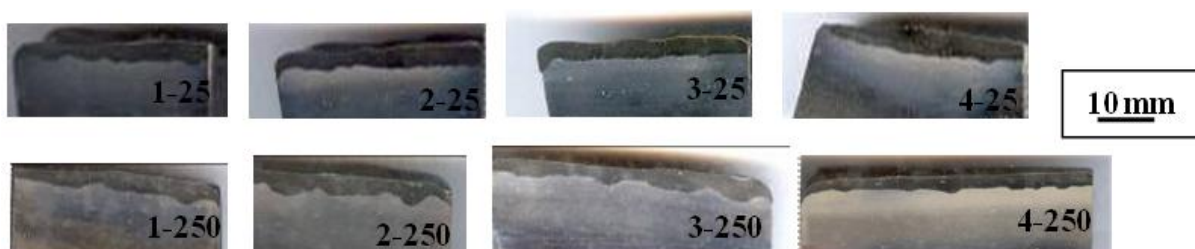
Figura 30. Macrografias longitudinal das soldas depositadas em um único passe.
