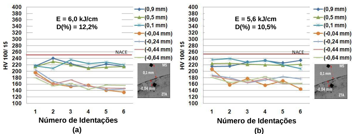
Figura 54: Perfil de microdureza ao longo do revestimento próximo a linha de fusão (interface) com pré-aquecimento 423 K (150 °C). (a) condição 24 V, 5 m/mim. (b) condição 22 V, 5 m/min.
