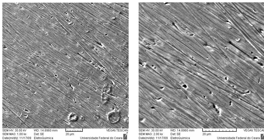
Figura 76 – Superfície de análise da amostra 24-7-S
