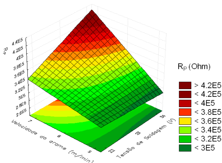
Figura 67: Superfície de resposta da tensão de soldagem vs. velocidade de alimentação do arame tendo como resposta a resistência de polarização.
