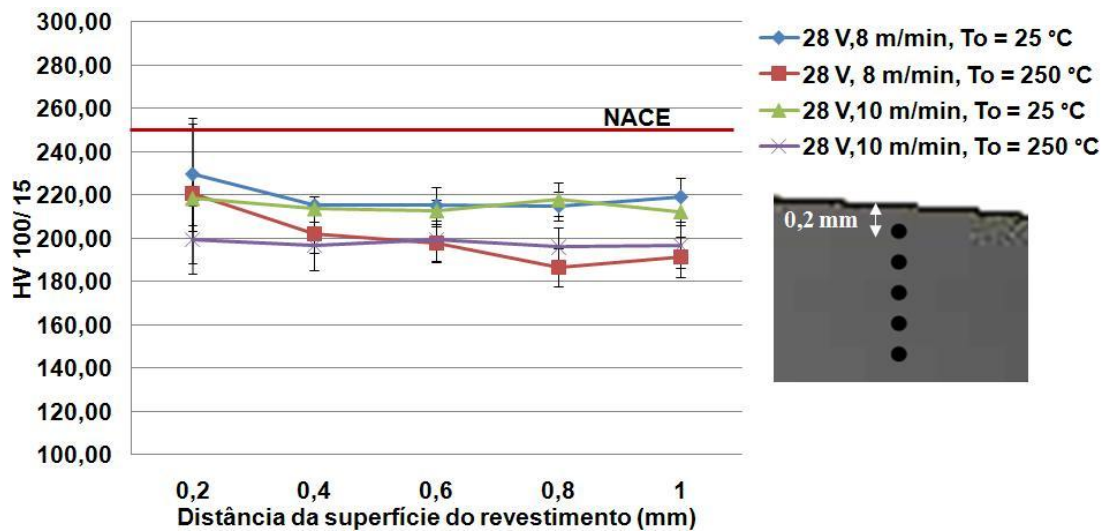
Figura 36. Perfil de microdureza próximo a superfície do revestimento soldado com tensão de 28 V na seção longitudinal.
