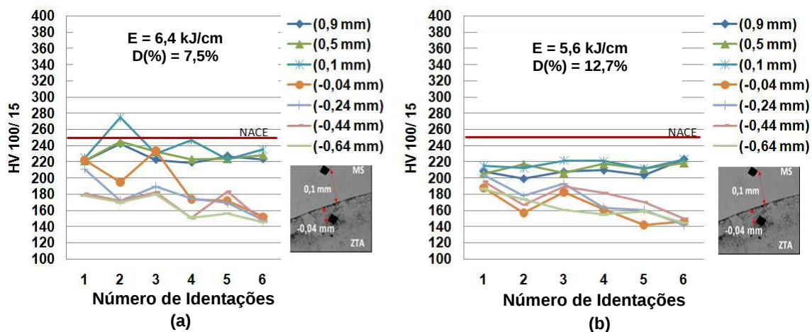
Figura 50: Perfil de microdureza ao longo do revestimento próximo a linha de fusão (interface) com tensão de 22 V, velocidade de alimentação de 7 m/min. (a) Sem pré-aquecimento e (b) Com pré-aquecimento 423 K (150 °C).
