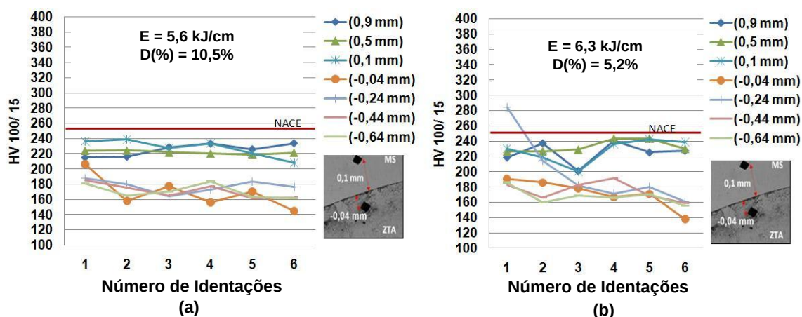
Figura 45: Perfil de microdureza ao longo do revestimento próximo a linha de fusão (interface) com tensão de 22 V, velocidade de alimentação de 5 m/mim. (a) com pré-aquecimento 423 K (150 °C) e (b) sem pré-aquecimento.
