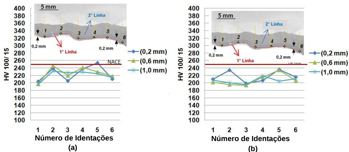
Figura 49: Perfil de microdureza próximo a superfície do revestimento com tensão de 22 V, velocidade de alimentação de 7 m/min. (a) sem pré-aquecimento e (b) com pré-aquecimento 423 K (150 °C).
