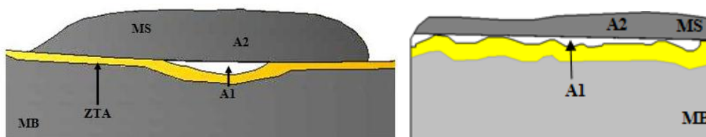
Figura 18. Áreas para o cálculo da diluição.
