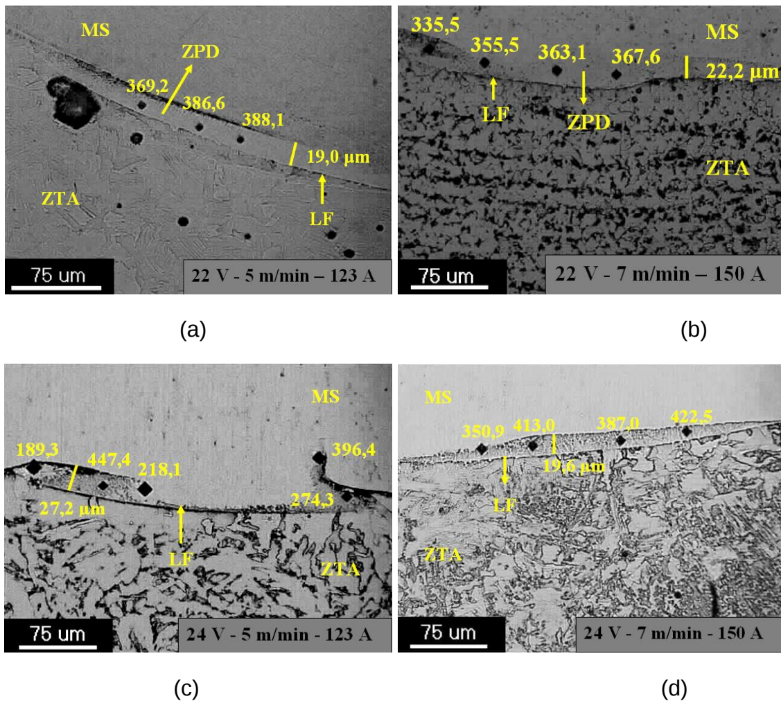
Figura 64. Interface da linha de fusão de soldas dissimilares depositadas em diferentes condições de tensão, velocidade de alimentação e pré-aquecimento T_o = 150\text{ }^{\circ}\text{C} para (a) H = 5,59\text{ kJ/cm} , (b) H = 5,56\text{ kJ/cm} , (c) 6,09\text{ kJ/cm} e (d) 5,97\text{ kJ/cm}
