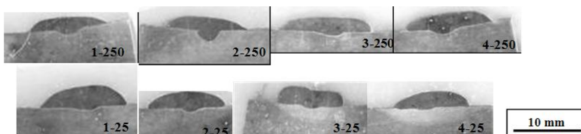
Figura 29. Macrografias transversal das soldas depositadas em um único passe.
