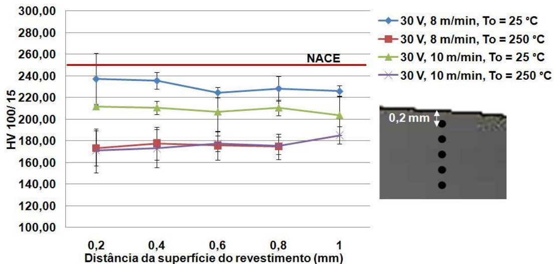
Figura 39. Perfil de microdureza próximo a superfície do revestimento soldado com tensão de 30 V na seção longitudinal.
