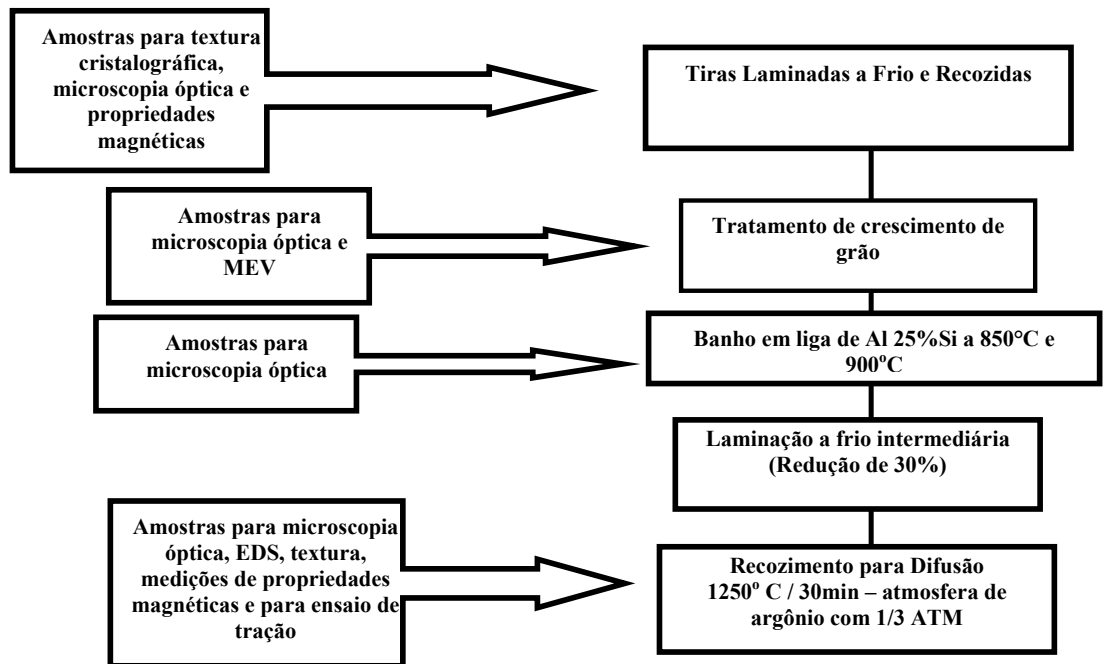
FIG. 3.16 Amostras retiradas de cada processo termomecânico
