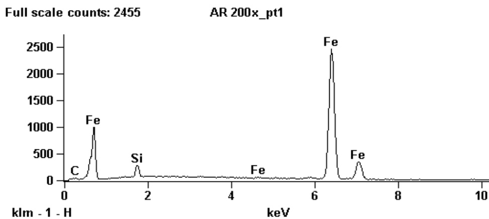
FIG. 4.65 Espectro de EDS da amostra AR como recebida
