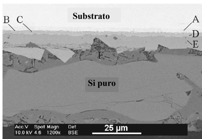
FIG. 2.18 Camadas depositadas após imersão por 20s (ROS-YÁÑEZ et al., 2004a)
