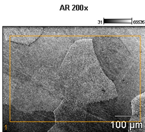
FIG. 4.64 Micrografia através do MEV da amostra AR indicando os pontos de análise de EDS
