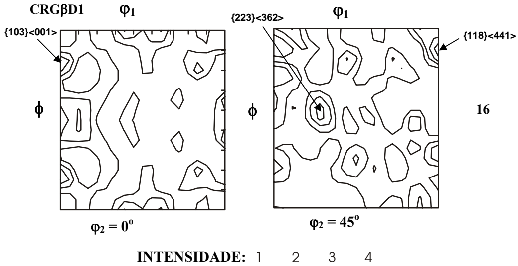
FIG. 4.57 FDOC da amostra CRG \beta D1, seções \phi_2 = 0^\circ e \phi_2 = 45^\circ , notação de Bunge
