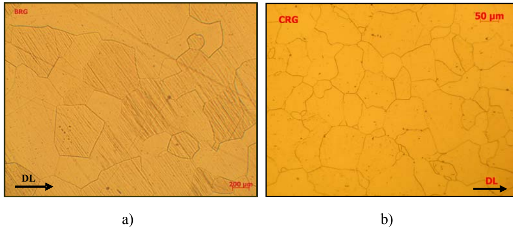
FIG. 4.13 Fotomicrografias microestruturais das amostras com tratamento de crescimento de grão: a) aço elétrico com 3,02%Si e espessura de 0,5 mm; b) aço elétrico com 0,8%Si e espessura de 0,6 mm
