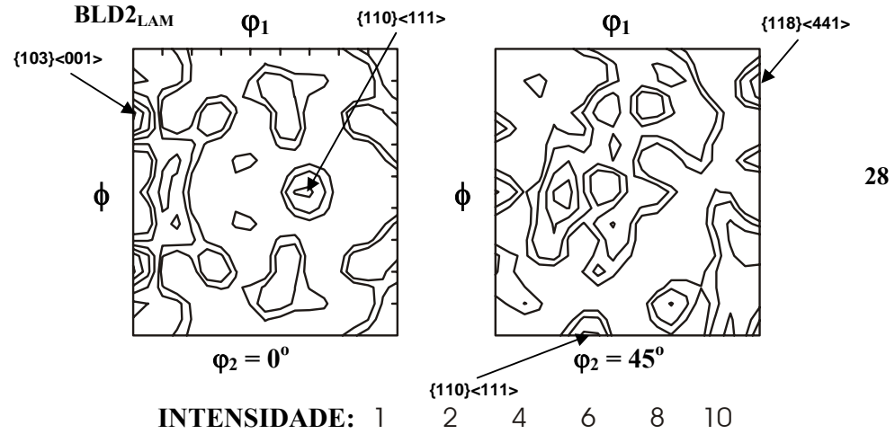
FIG. 4.51 FDOC da amostra BLD2 Lam , seções \phi_2 = 0^\circ e \phi_2 = 45^\circ , notação de Bunge
