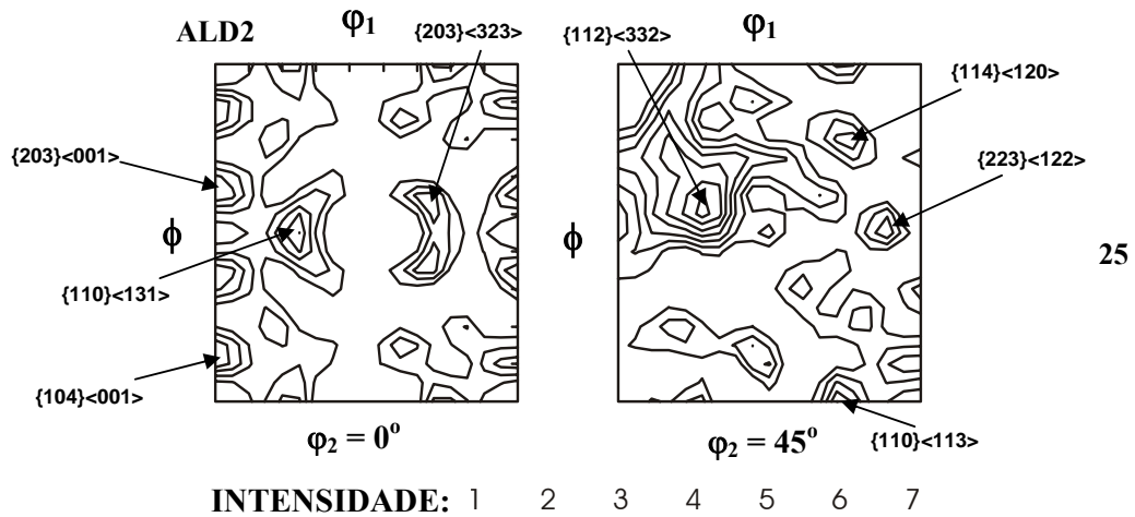
FIG. 4.42 FDOC da amostra ALD2, seções \phi_2 = 0^\circ e \phi_2 = 45^\circ , notação de Bunge
