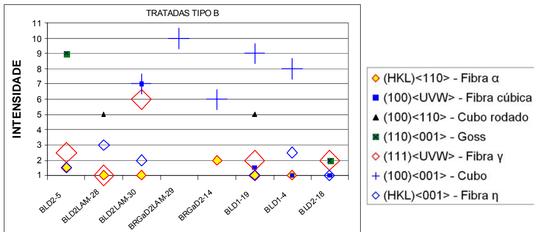
FIG. 4.55 Gráfico relacionando as amostras tratadas do tipo B com as fibras e componentes de textura que mais influenciam nas propriedades magnéticas
