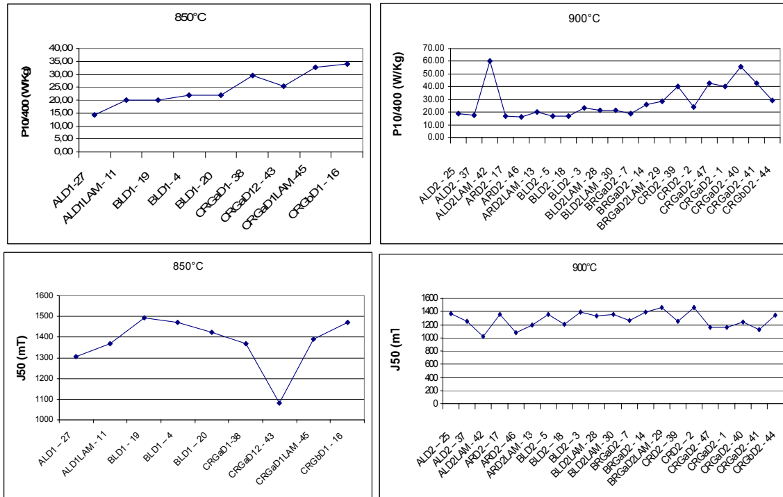
FIG. 5.6 Gráficos relacionando cada amostra com sua respectiva medida de perda e polarização magnética nas temperaturas de imersão a quente de 850°C e 900°C
