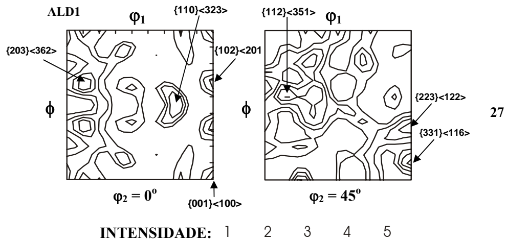
FIG. 4.40 FDOC da amostra ALD1, seções \phi_2 = 0^\circ e \phi_2 = 45^\circ , notação de Bunge
