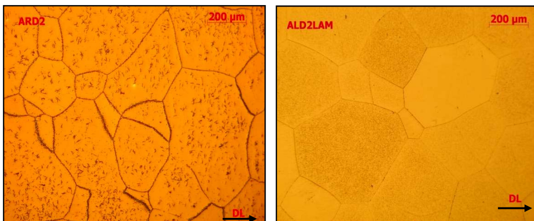
FIG. 4.14 Fotomicrografias microestruturais das amostras com imersão a quente a 900°C seguida de tratamento para difusão: a) aço elétrico do tipo AR sem laminação antes do tratamento para difusão; b) aço elétrico do tipo AL com laminação antes do tratamento de difusão
