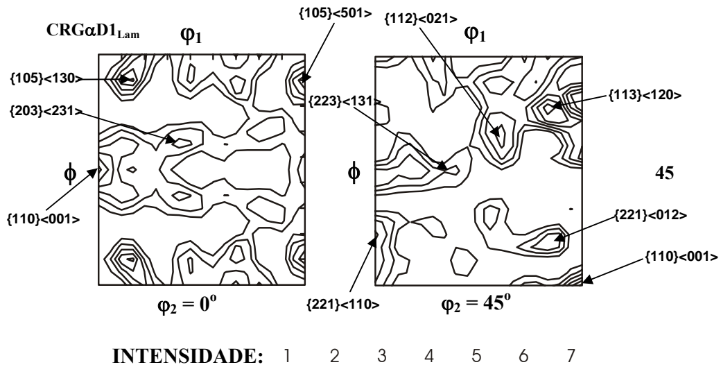
FIG. 4.62 FDOC da amostra CRG \alpha D1 Lam , seções \phi_2 = 0^\circ e \phi_2 = 45^\circ , notação de Bunge
