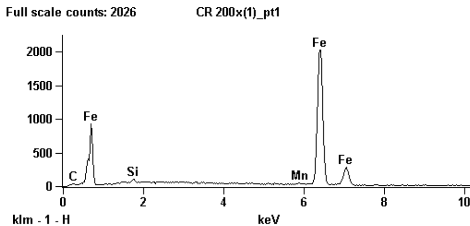
FIG. 4.69 Espectro de EDS da amostra CR como recebida
