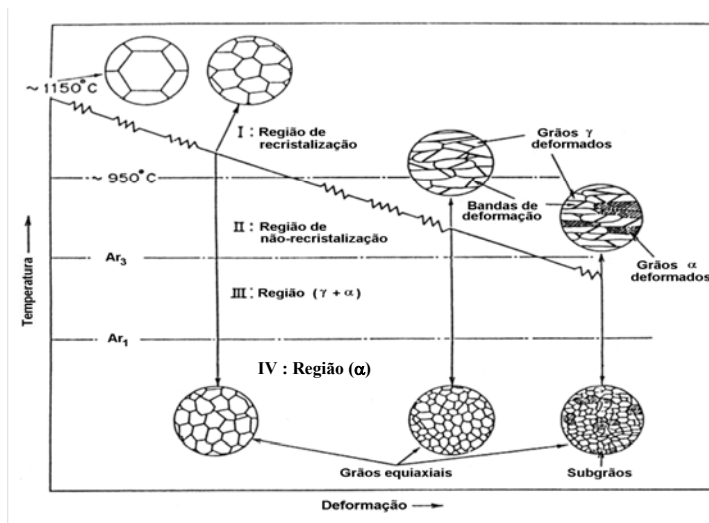
FIG. 2.8 Diagrama esquemático ilustrando os estágios do processo de laminação controlada e as mudanças na microestrutura em cada estágio (RAY e JONAS, 1990)
