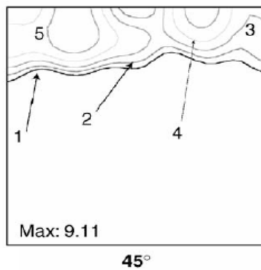
FIG. 2.24 FDOC da camada de Fe_3Si após a imersão a quente em um substrato de FeSi de 3% em peso (HOUBAERT et al., 2006)
