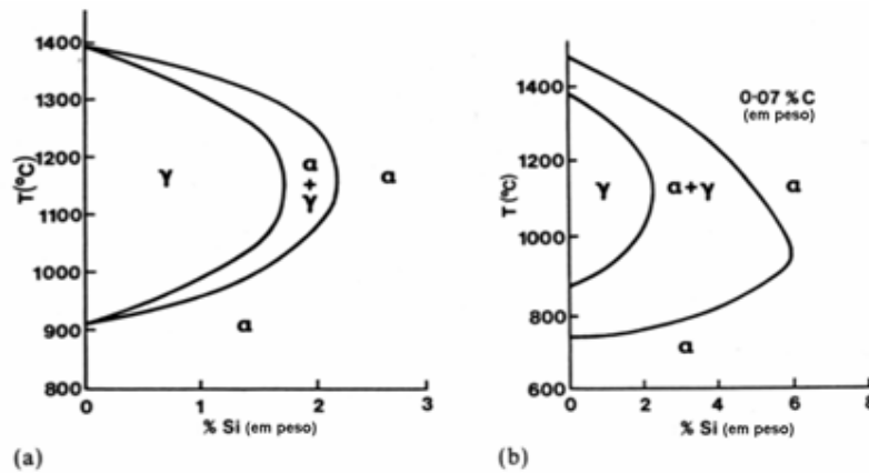
FIG. 2.7 Diagrama Fe-Si, a) Região rica em Fe do diagrama Fe-Si; b) o efeito da adição de 0,07% C nessa região do diagrama (MCCURRIE, 1994)
