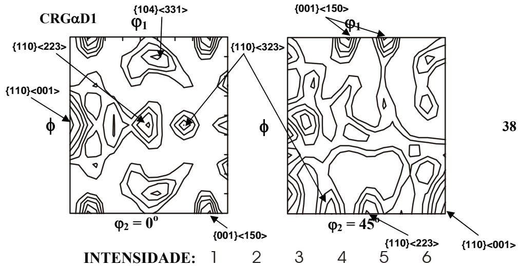
FIG. 4.58 FDOC da amostra CRG \alpha D1, seções \phi_2 = 0^\circ e \phi_2 = 45^\circ , notação de Bunge
