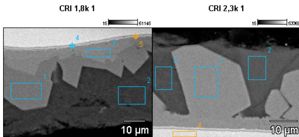
FIG. 4.2 Micrografia através de MEV por imagem de elétrons retroespalhados da amostra CRI com indicação das regiões onde se realizaram os EDS
