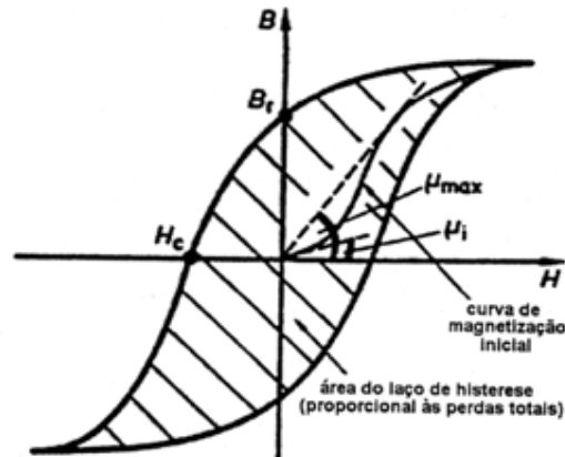
FIG. 2.1 Curva de histerese de um material ferromagnético (BOLL,1992).
