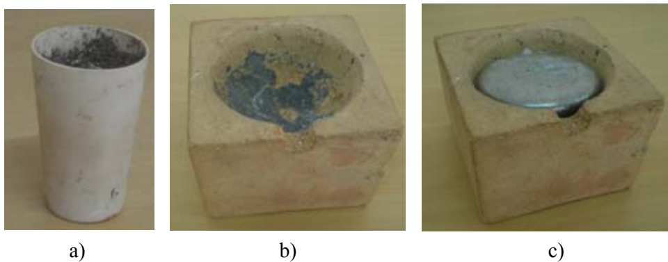
FIG. 3.11 a) cadinho de alumina; b) cadinho robusto e c) cadinho robusto com a liga solidificada
