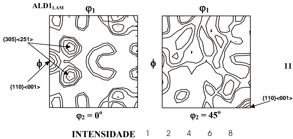
FIG. 4.39 FDOC da amostra ALD1 Lam , seções \phi_2 = 0^\circ e \phi_2 = 45^\circ , notação de Bunge
