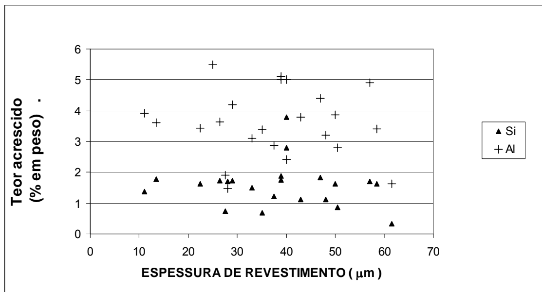
FIG. 5.2 Gráfico relacionando o teor de Al e Si acrescido em porcentagem em peso com a espessura de revestimento
