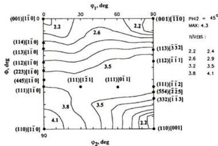
FIG. 2.14 Mapa do coeficiente M de Taylor, calculado seguindo o modelo "full-constraint". Seção \phi_2=45^\circ . Notação de Bunge (RAY ET AL., 1994)
