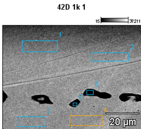
FIG. 4.24 Imagem de elétrons retroespalhados dos poro indicando as regiões de EDS
