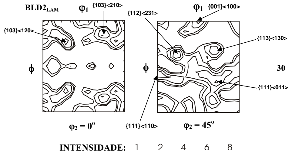
FIG. 4.52 FDOC da amostra BLD2 LAM , seções \phi_2 = 0^\circ e \phi_2 = 45^\circ , notação de Bunge
