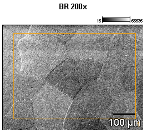
FIG. 4.66 Micrografia através do MEV da amostra BR indicando os pontos de análise de EDS
