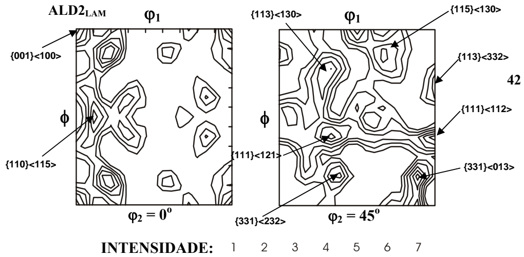
FIG. 4.43 FDOC da amostra ALD2 Lam , seções \phi_2 = 0^\circ e \phi_2 = 45^\circ , notação de Bunge
