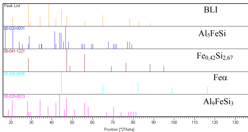
FIG. 4.8 Difratoograma padrão e da amostra BLI
