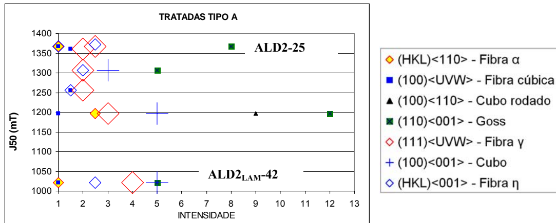
FIG. 5.18 Gráfico relacionando as induções de saturação magnética J_{50} com as fibras e componentes de textura que mais influenciam nas propriedades magnéticas (amostras do tipo A)
