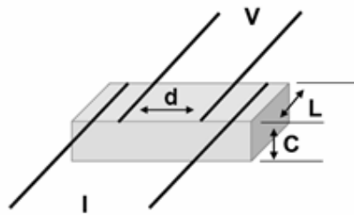
FIG. 3.27 Configuração convencional dos contatos para o cálculo da resistividade em uma amostra polidral. I e V representam os fios de corrente e voltagem respectivamente
