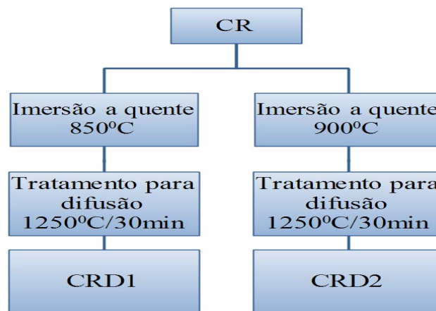
FIG. 3.5 Fluxograma dos tratamentos termomecânicos realizados a partir da amostra CR como recebida sem o tratamento de aperfeiçoamento de textura
