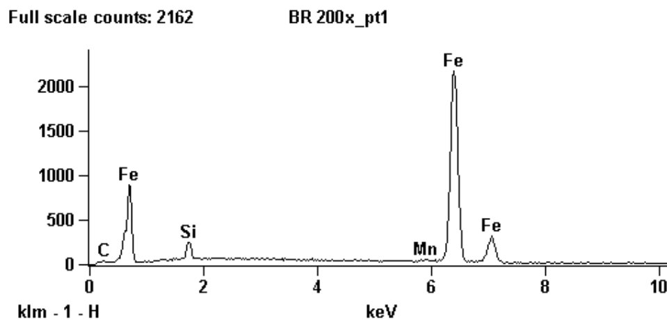
FIG. 4.67 Espectro de EDS da amostra BR como recebida
