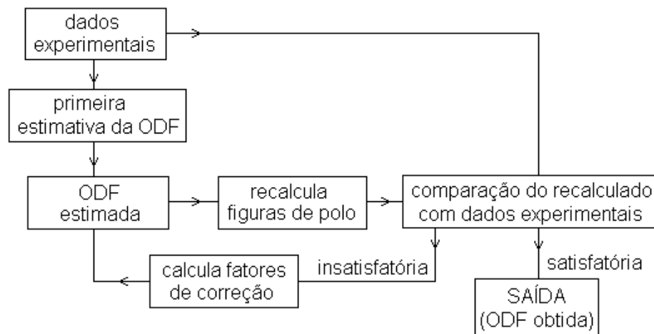
FIG. 3.22 Algoritmo do método WIMV (baseado em KALLEND, 1998)
