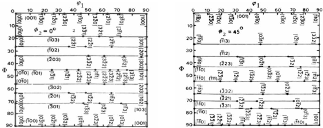
FIG. 2.33 Ábacos de \varphi_2 = 0^\circ e \varphi_2 = 45^\circ para interpretar as FDOCs em termos de ângulos de Euler e índices (hkl)[uvw]
