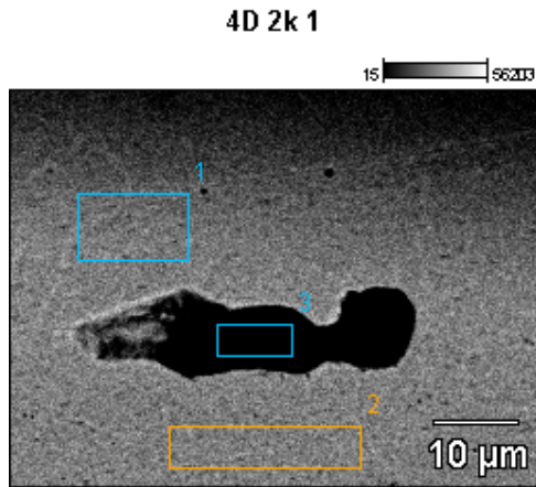
FIG. 4.23 Imagem de elétrons retroespalhados do poro indicando as regiões de EDS
