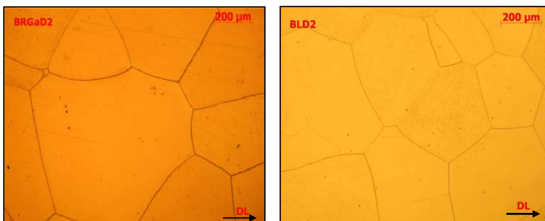
FIG. 4.15 Fotomicrografias microestruturais das amostras com imersão a quente a 900°C com tratamento para difusão: a) aço elétrico do tipo BR com tratamento de crescimento de grão antes da imersão a quente; b) aço elétrico do tipo BL
