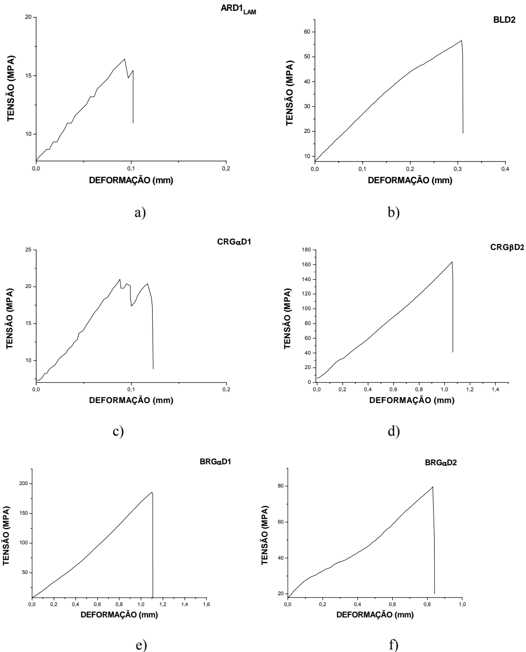
FIG. 4.74 Curva de tensão-deformação de engenharia das amostras com recozimento de difusão: a) ARD1 LAM , b) BLD2, c) CRG \alpha D1, d) CRG \beta D2, e) BRG \alpha D1 e f) BRG \alpha D2
