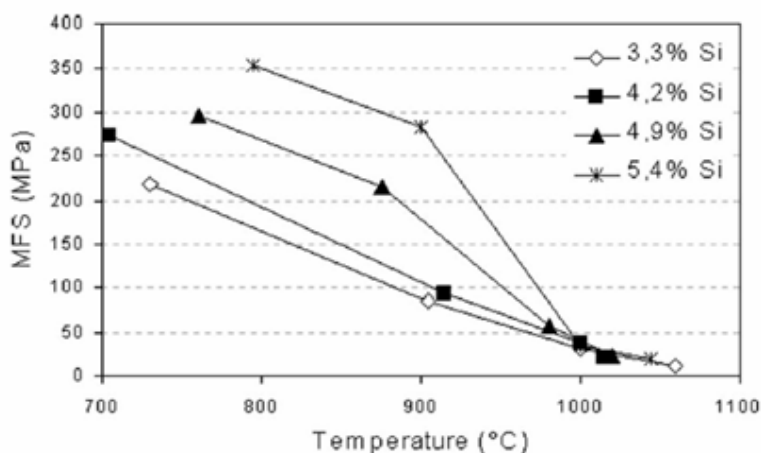
FIG. 2.15 Evolução da tensão de fluxo médio com temperatura durante laminação a quente em quatro passes ( 80, 80, 40 e 35% de redução por passe), todas as amostras reaquecidas em 1150°C (ROS-YÁÑEZ et al., 2004a)
