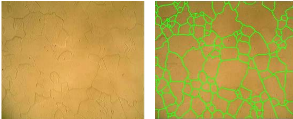
FIG. 4.9 Exemplo de determinação dos contornos de grão pelo programa AxioVision
