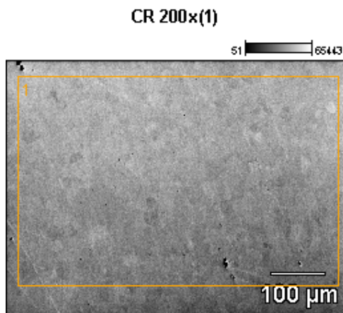
FIG. 4.68 Micrografia através do MEV da amostra CR indicando os pontos de análise de EDS
