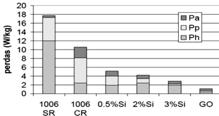
FIG. 2.4 Perdas totais e suas componentes histerética (Ph), parasita (Pp) e anômala (Pa) em seis diferentes aços elétricos utilizados no Brasil (LANDGRAF, 2002)
