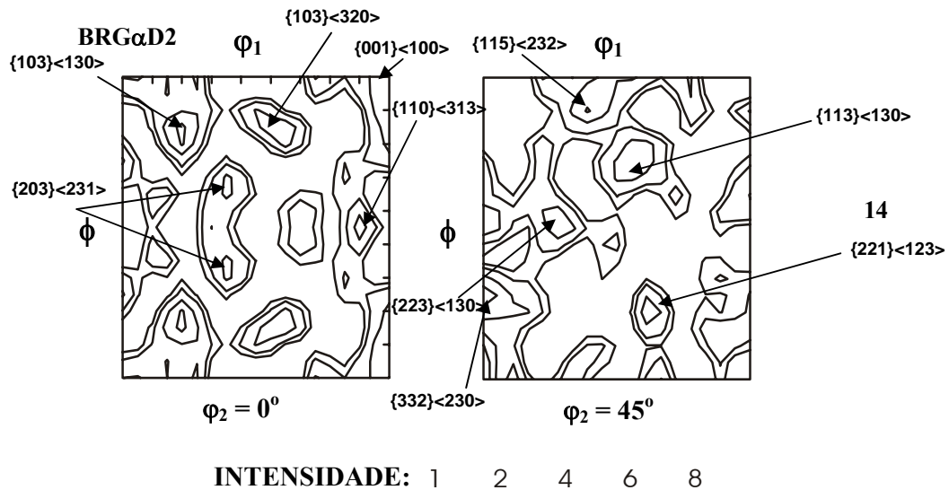
FIG. 4.54 FDOC da amostra BRGαD2, seções \phi_2 = 0^\circ e \phi_2 = 45^\circ , notação de Bunge
