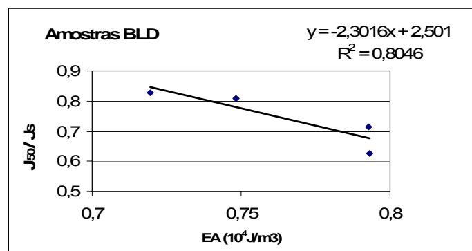
FIG. 5.23 J_{50}/J_S versus E_a das amostras tratadas do tipo BLD
