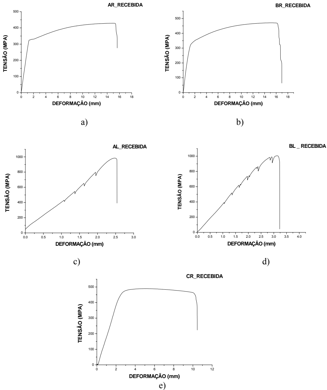
FIG. 4.73 Curvas de tensão-deformação de engenharia das amostras como recebida: a) amostra AR, b) amostra BR, c) amostra AL, d) amostra BL e e) amostra CR
