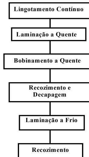
FIG. 2.6 Processo convencional de fabricação dos aços elétricos
