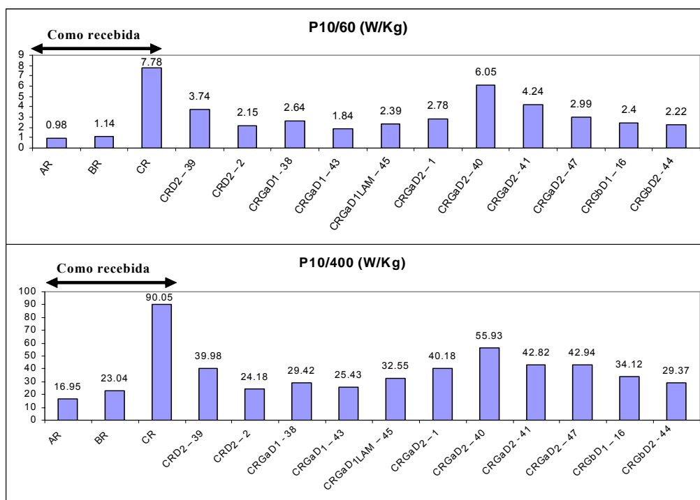
FIG. 5.11 Perdas Magnéticas ( P_{10/60} e P_{10/400} ) das amostras como recebidas e das tratadas da Brasmetal
