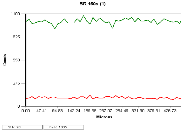
FIG. 4.71 Perfil de concentração ao longo da espessura da amostra como recebida AR
