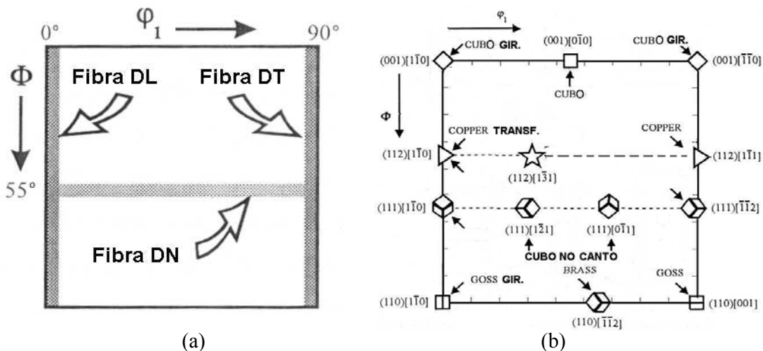
FIG. 2.34 (a) Seção de \varphi_2 = 45^\circ com as fibras clássicas do sistema cúbico; (b) Seção de \varphi_2 = 45^\circ mostrando os nomes de orientações clássicas do sistema cúbico
