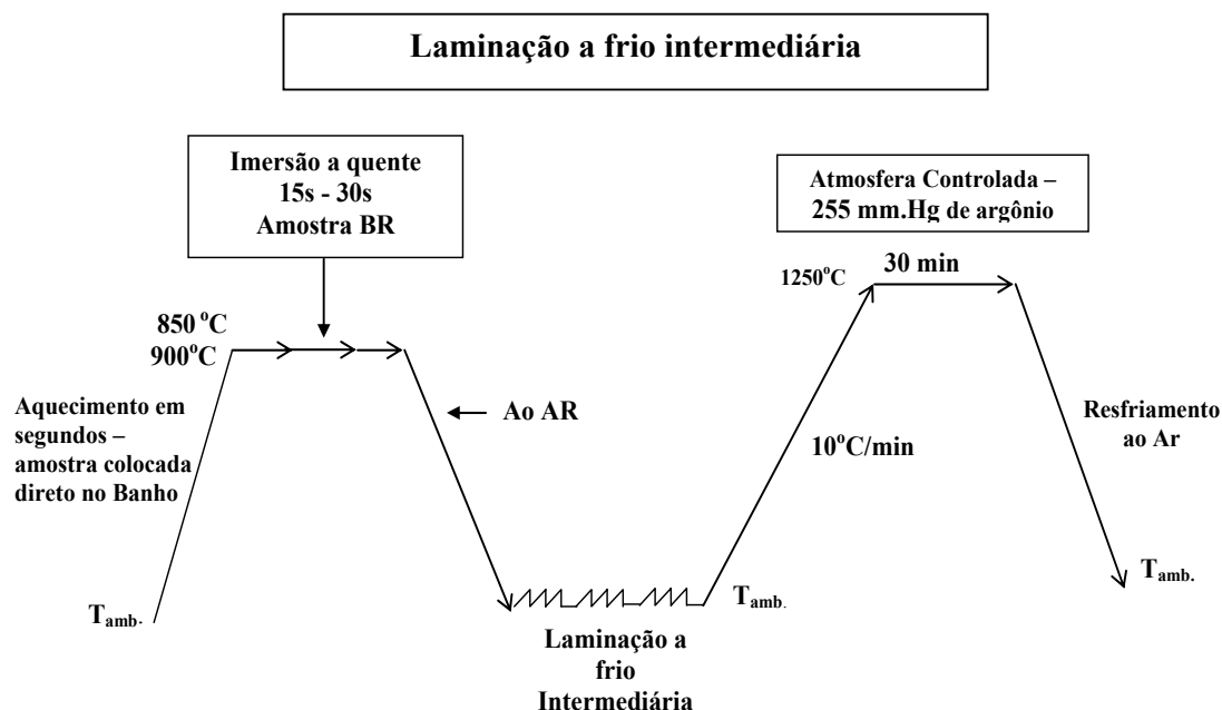
FIG. 3.12 Fluxograma da Imersão a quente e recozimento de difusão com laminação intermediária
