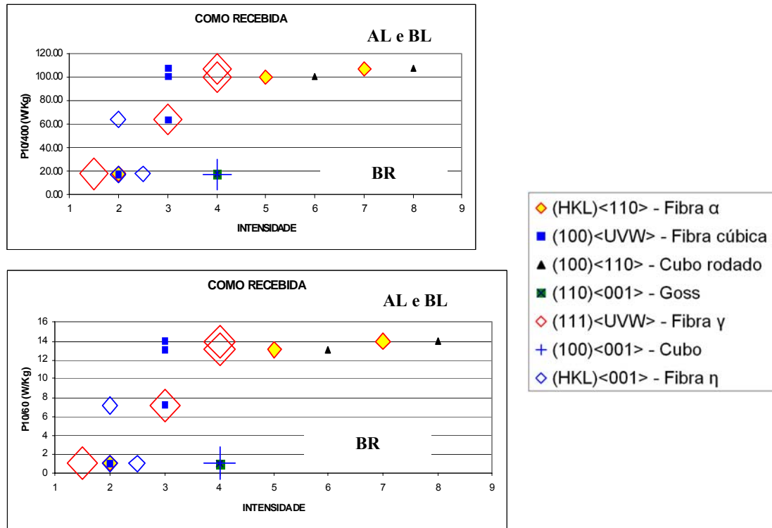
FIG. 5.13 Gráfico relacionando as perdas magnéticas com as fibras e componentes de textura que mais influenciam nas propriedades magnéticas (amostras como recebida)
