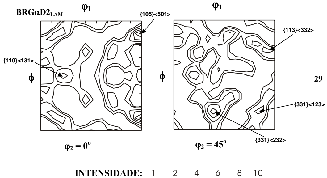
FIG. 4.53 FDOC da amostra BRG \alpha D2 LAM , seções \phi_2 = 0^\circ e \phi_2 = 45^\circ , notação de Bunge
