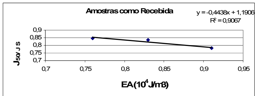
FIG. 5.21 J_{50}/J_S versus E_a das amostras como recebida
