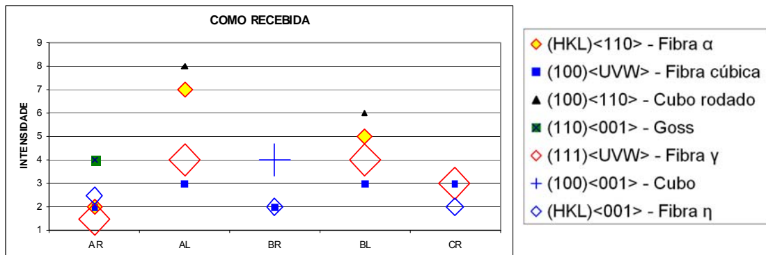
FIG. 4.38 Gráfico relacionando as amostras como recebida com as fibras e componentes de textura que mais influenciam as propriedades magnéticas
