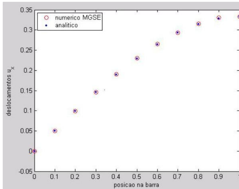
Figura 26: Comparativo entre a solução analítica e a numérica do MGSE para força f^B(x) proporcional à posição.
