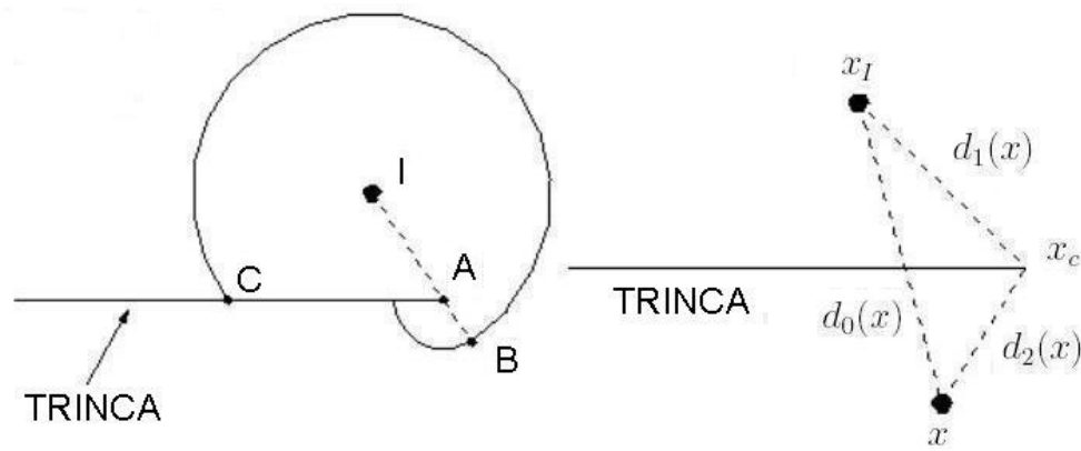
Figura 22: Representação do domínio de influência do nó segundo o critério de difração.
