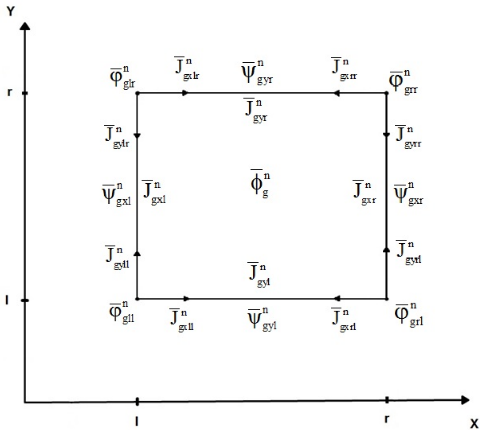
Figura 3.2 - Dados para o cálculo dos coeficientes c_{ij,g}^n .
