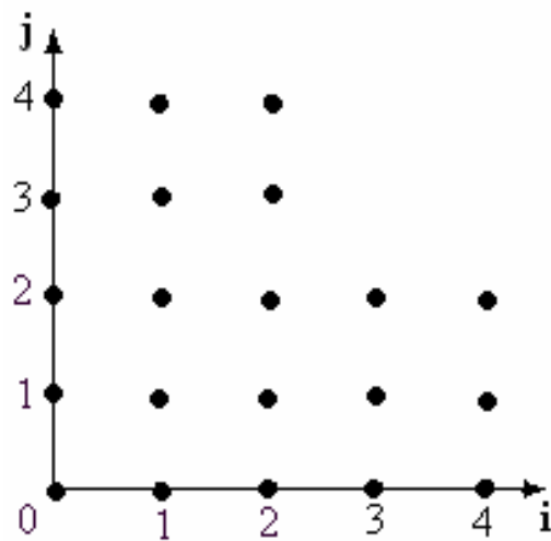
Figura 3.1 - Os coeficientes c_{ij,g}^n \neq 0 usados neste método.
