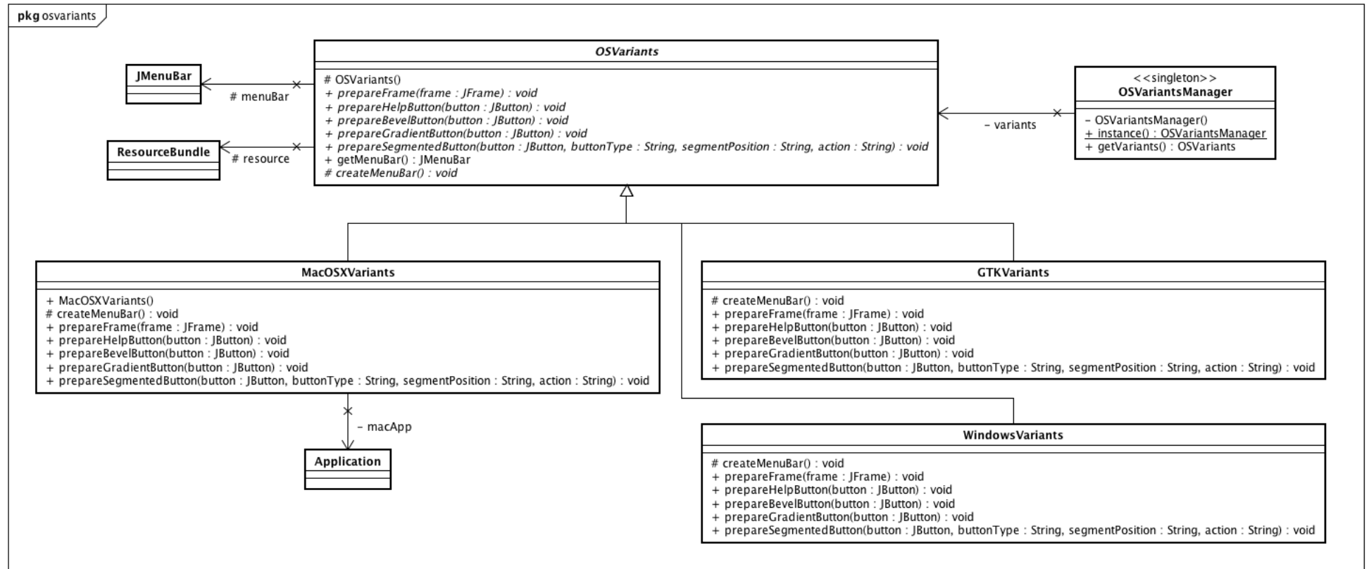
Figura 5.10: Classes responsáveis pela integração com o sistema operacional.
