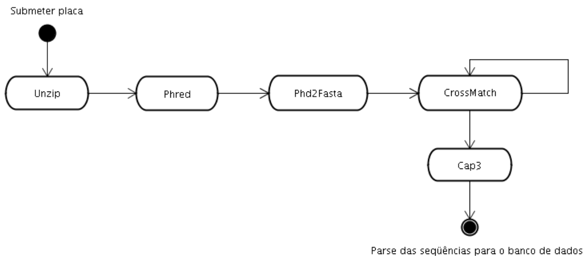
Figura 2.11: Exemplo de seqüência de programas executados na fase de submissão.
