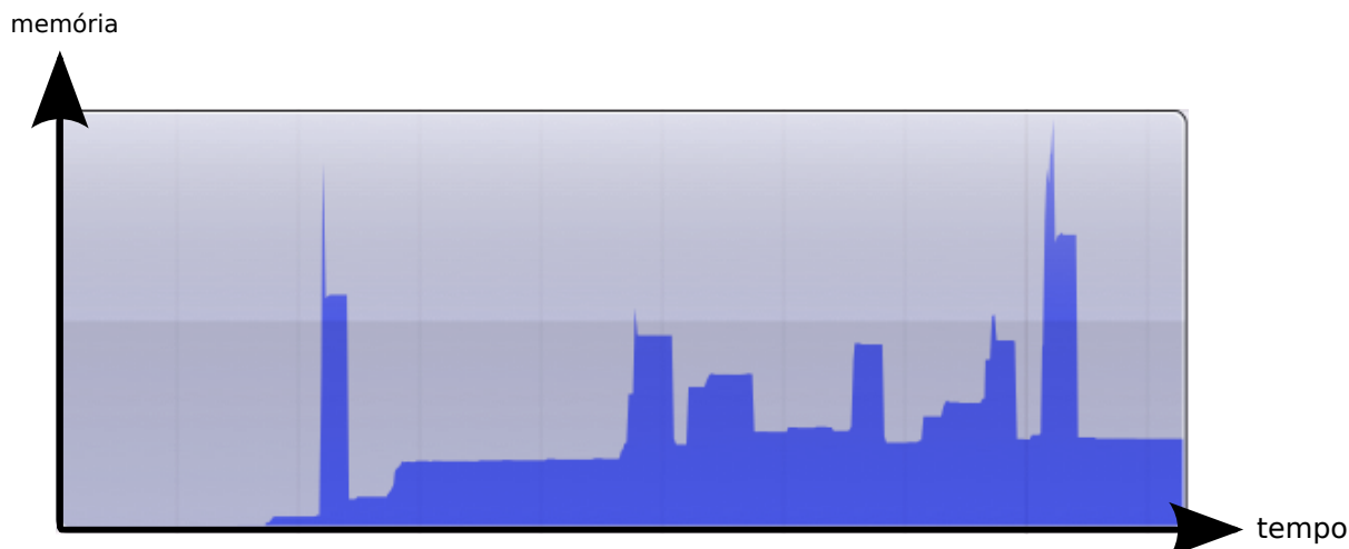
Figura 6.5: Consumo de memória do Syntainia ao longo do tempo. O tempo inicia após a abertura da aplicação. Em seguida é feita a geração de um novo gráfico, comparando dois genomas. O tempo se encerra com a exibição do gráfico. No eixo vertical, o consumo de memória varia de 0 a 14 MB.
