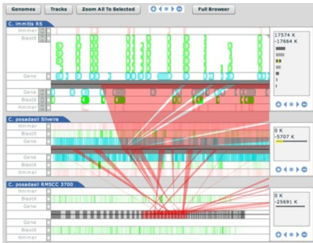
Figura 3.15: Módulo de visualização Stack Map do MEDEA, mostrando a comparação entre três genomas.
