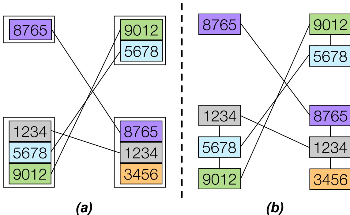
Figura 5.5: Visualização de genes no Syntainia como um grafo. Em (a) é apresentado um exemplo da visualização dos genes pelo Syntainia. Em (b) a visualização é extrapolada para evidenciar as relações entre os genes como um grafo. É importante destacar que ao tentar reduzir o cruzamento de arestas, não é possível fazer um novo arranjo entre os vértices do grupo 1234–5678–9012, por exemplo, uma vez que a ordem dos genes em questão precisa ser preservada. O que pode ser feito é movimentar o grupo 9012–5678 para baixo do grupo 8765–1234–3456 no genoma à direita.
