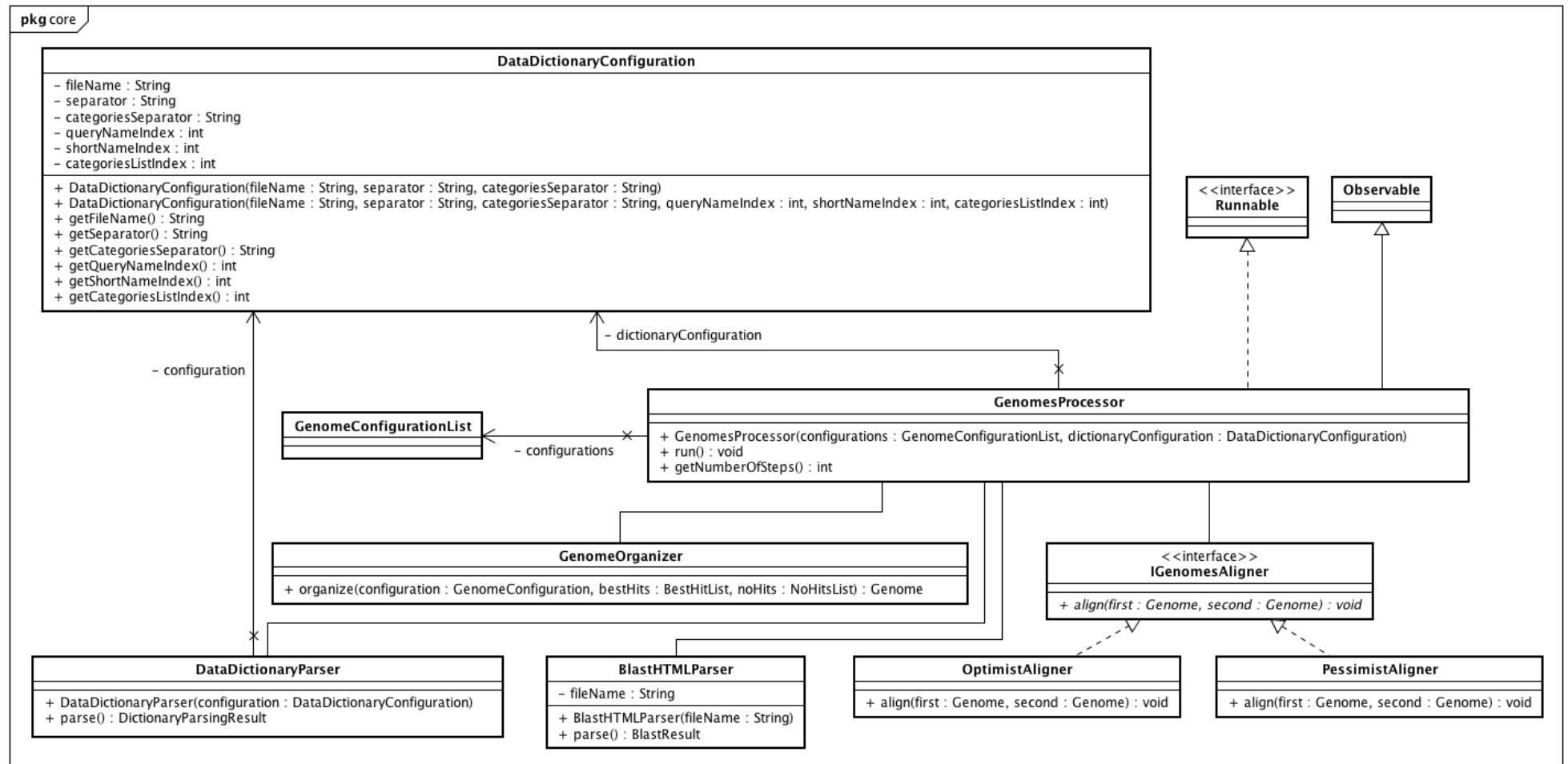
Figura 5.8: Classes do núcleo do Syntainia, responsáveis pela organização das estruturas de dados para geração do gráfico.
