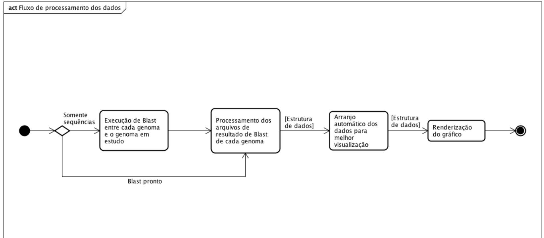
Figura 5.7: Fluxo de processamento dos dados no Syntainia.
