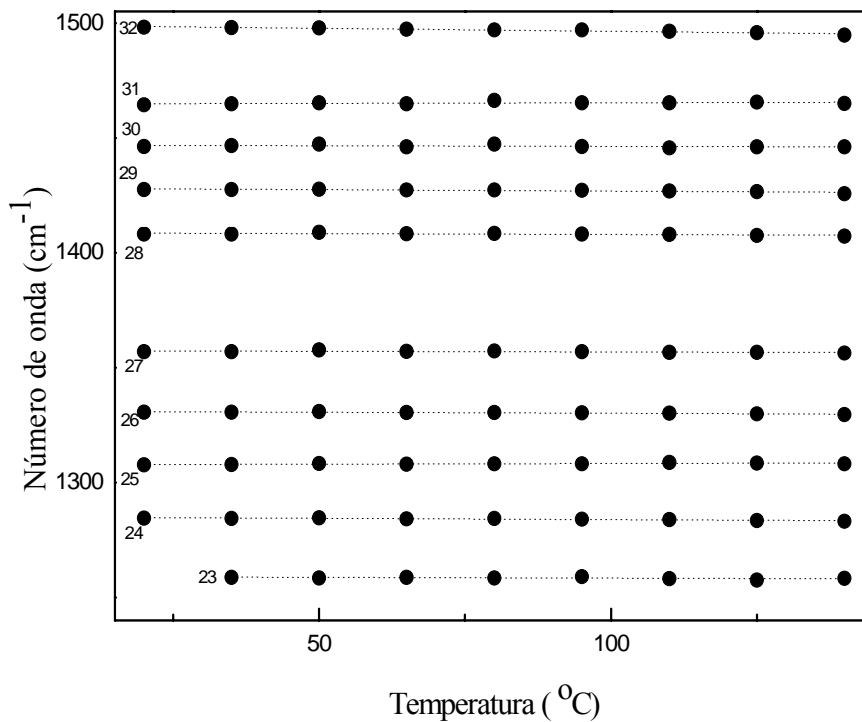
Figura 5.9a Gráfico do número de onda versus temperatura na região espectral entre 1200\text{ cm}^{-1} e 1500\text{ cm}^{-1} .
