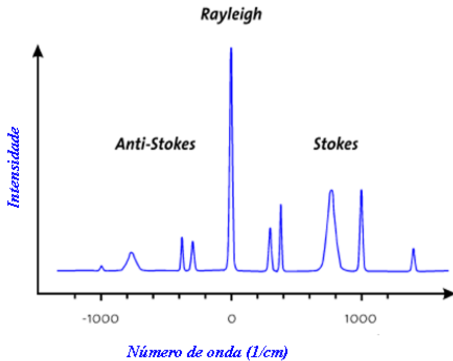
Figura 1.5 Ilustração de espectro Raman típico. As diferenças de intensidade entre as linhas anti-Stokes, Rayleigh e Stokes são expostas.
