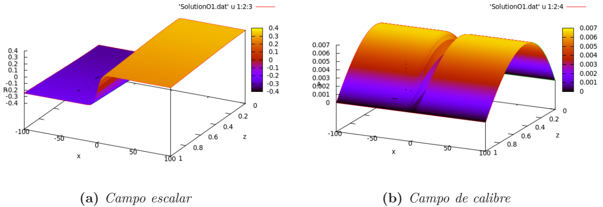
Figura 4.1: Solução para os campos na teoria \mathcal{O}_1
