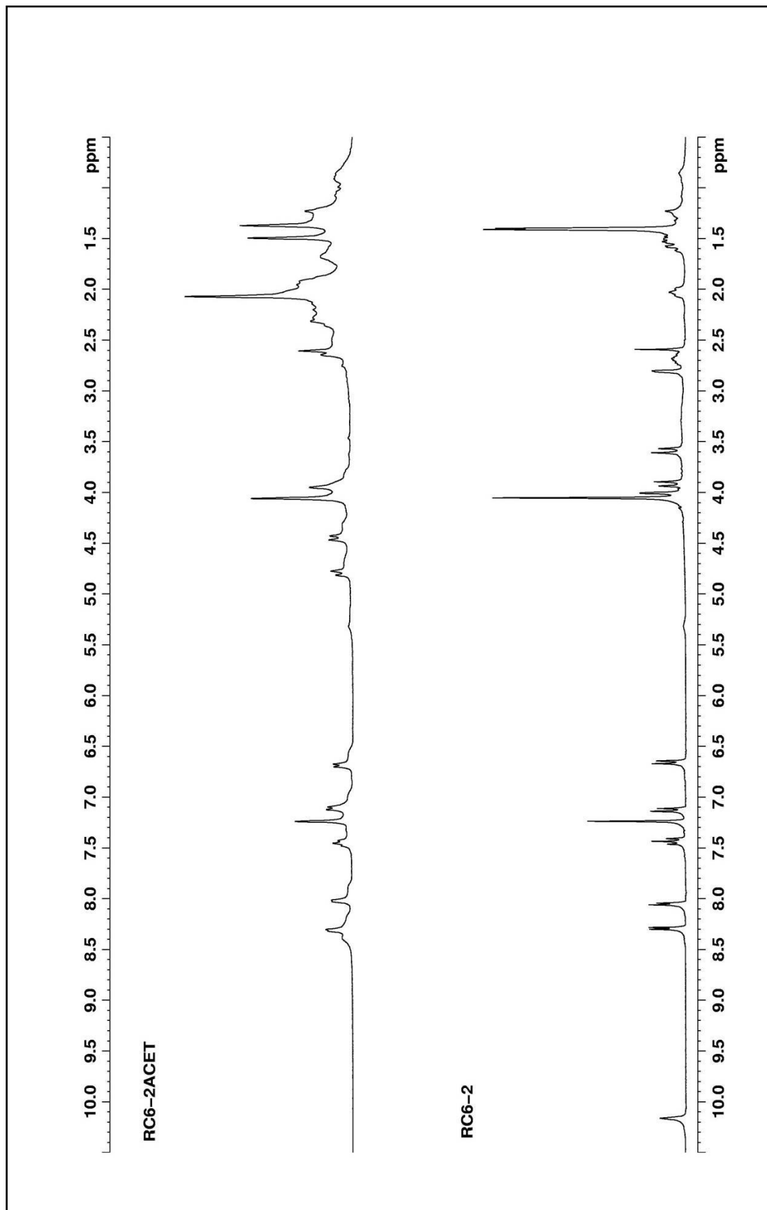
Figura 21 - Espectros de RMN ^1\text{H} da Substância 1 e da Substância 1 acetilada ( \text{CDCl}_3 , 300 MHz).
