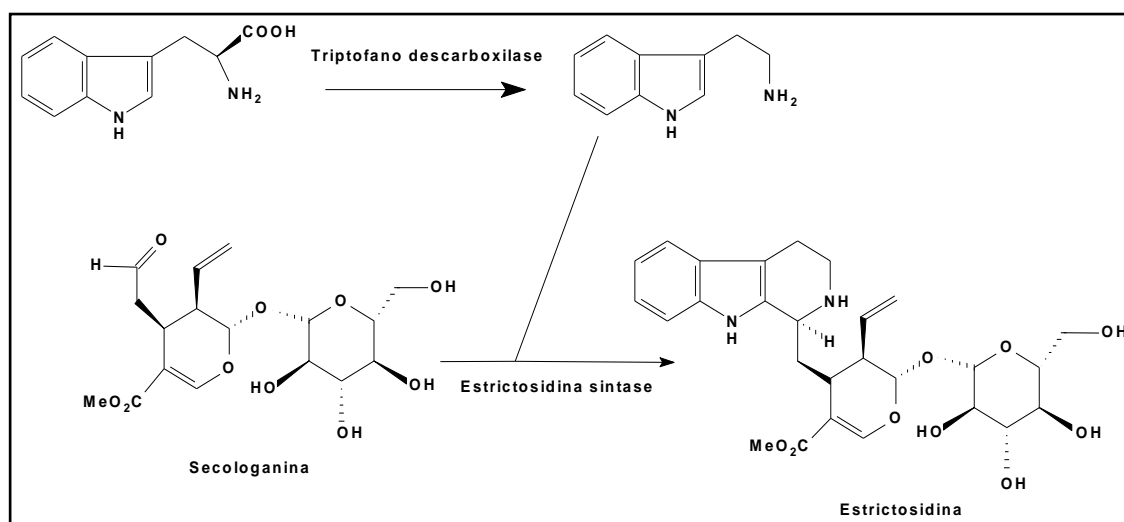
Figura 29 - Primeiras etapas na biossíntese dos alcalóides indol-monoterpênicos.
