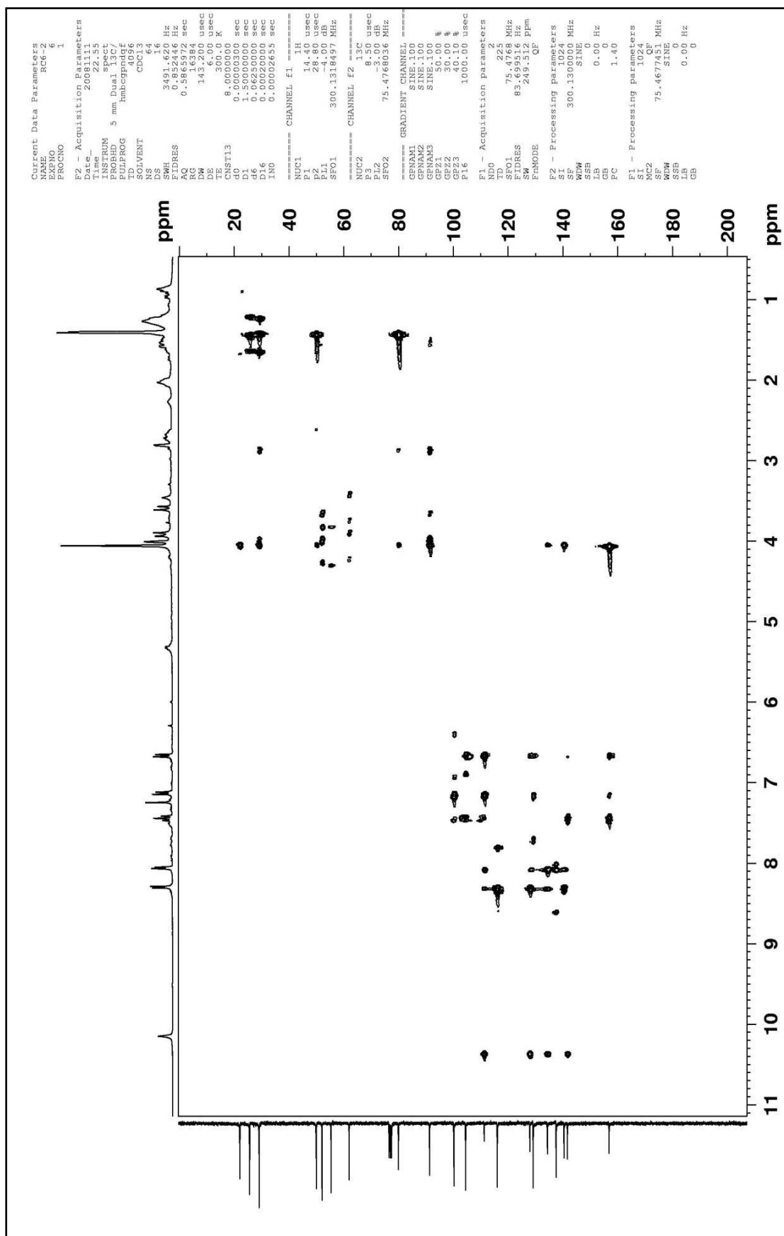
Figura 18 - Espectro de RMN HMBC da Substância 1 (CDCl3, 300/75 MHz).
