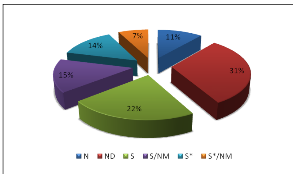
Figura 2 – Micromoléculas anticâncer descobertas no período de 01/1981 – 06/2006, segundo a origem (N = 81). Adaptado de: Newman e Cragg (2007).
