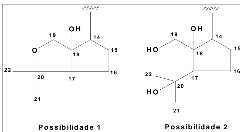
Figura 20 – Propostas de estruturas para a porção não aromática da Substância 1.
