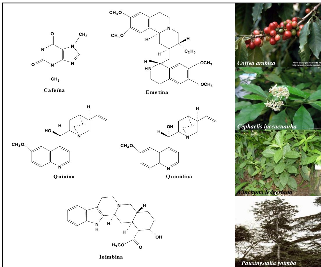
Figura 5 – Exemplares de rubiáceas e alguns de seus metabólitos secundários de importância econômica.
