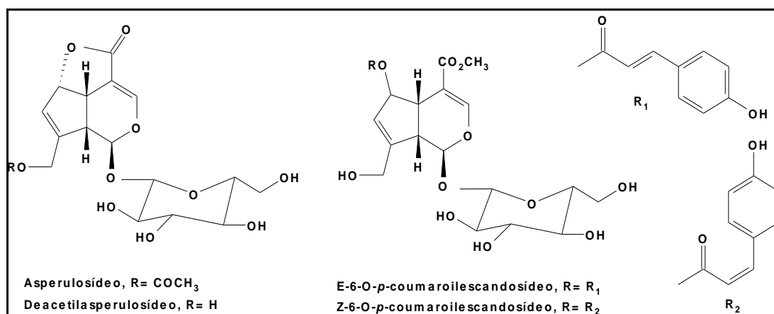
Figura 7 – Estruturas moleculares dos componentes químicos isolados de G. brasiliensis .
