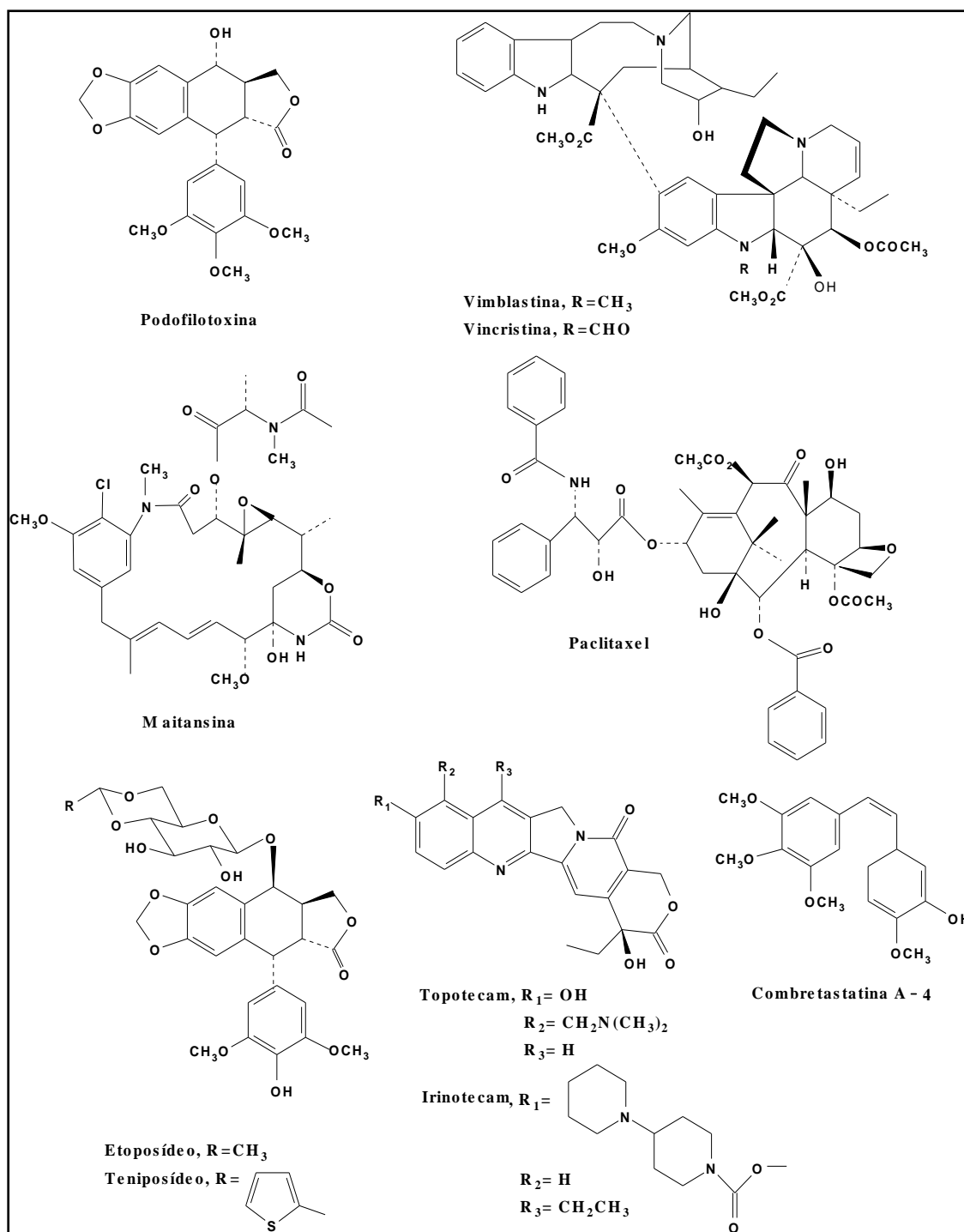
Figura 1– Estruturas químicas de alguns compostos anticâncer originados ou derivados de plantas.
