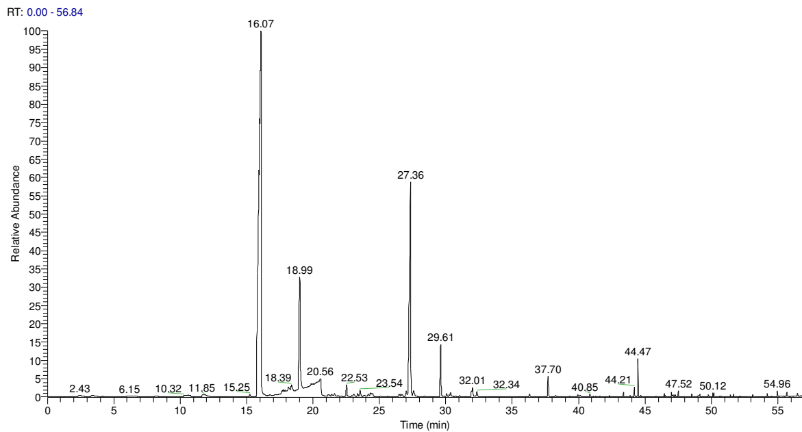
Figura A.18 – Perfil cromatográfico dos compostos voláteis do headspace do genótipo Tanasio.
