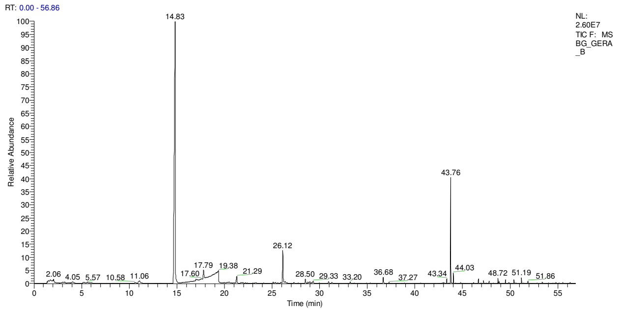
Figura A.10 – Perfil cromatográfico dos compostos voláteis do headspace do genótipo Gera.
