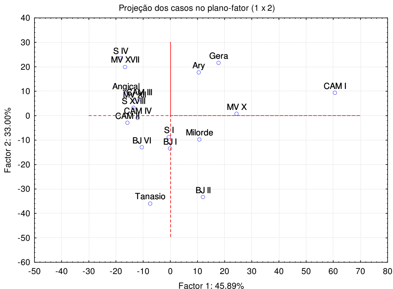
Figura 14 – Gráfico de dispersão de escores para o primeiro e segundo componentes principais, em relação às médias das intensidades relativas dos genótipos de pequizeiro.
