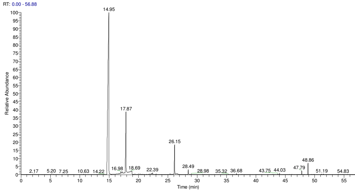
Figura A.9 – Cromatograma dos compostos voláteis do headspace do genótipo CAM IV.
