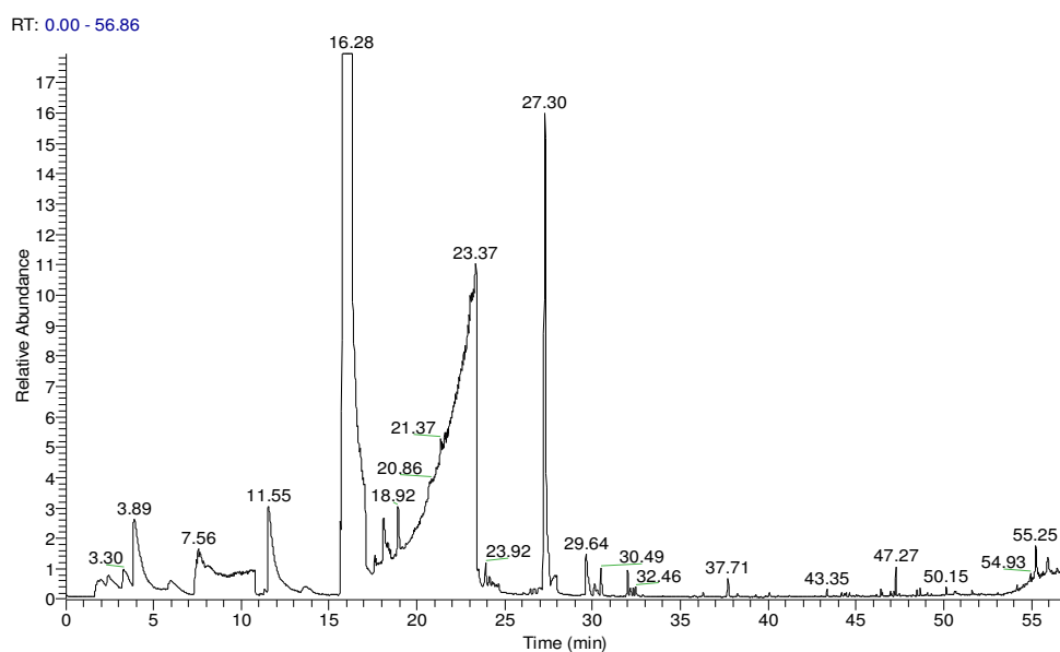
Figura 12 – Cromatogramas do perfil de compostos voláteis extraídos pela fibra de CAR-PDMS: (a) Cromatograma total; (b) Cromatograma ampliado.
