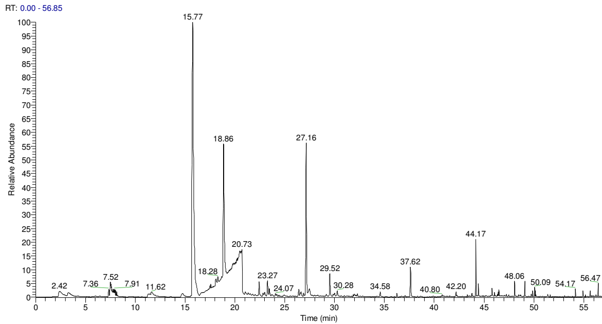
Figura A.4 – Perfil cromatográfico dos compostos voláteis do headspace do genótipo BJ II.
