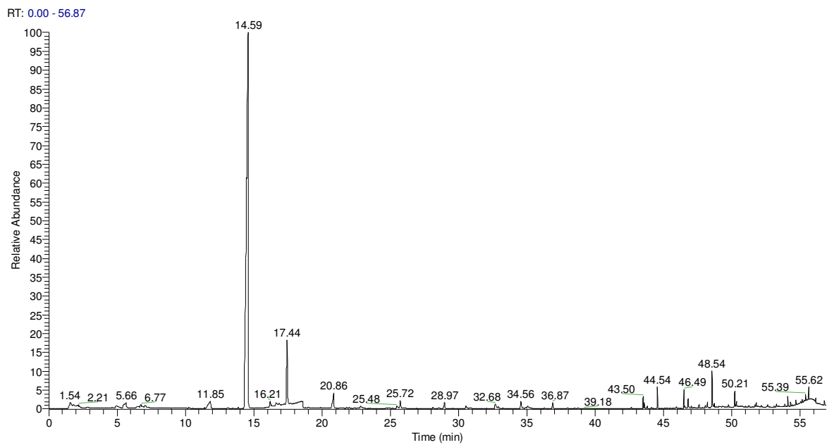
Figura A.14 – Perfil cromatográfico dos compostos voláteis do headspace do genótipo MV XVII.
