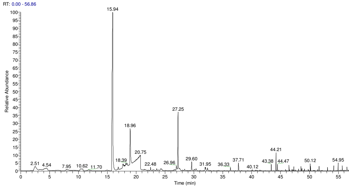
Figura A.3 – Perfil cromatográfico dos compostos voláteis do headspace do genótipo BJ I.
