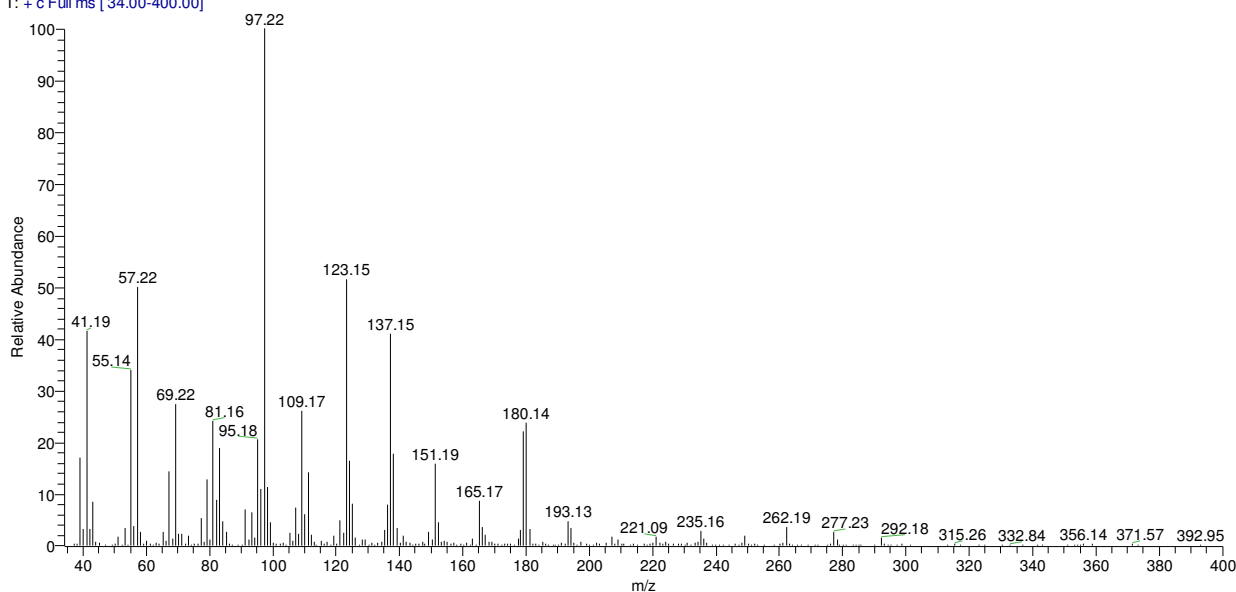
Figura 10 – Espectro de massas do composto desconhecido.
