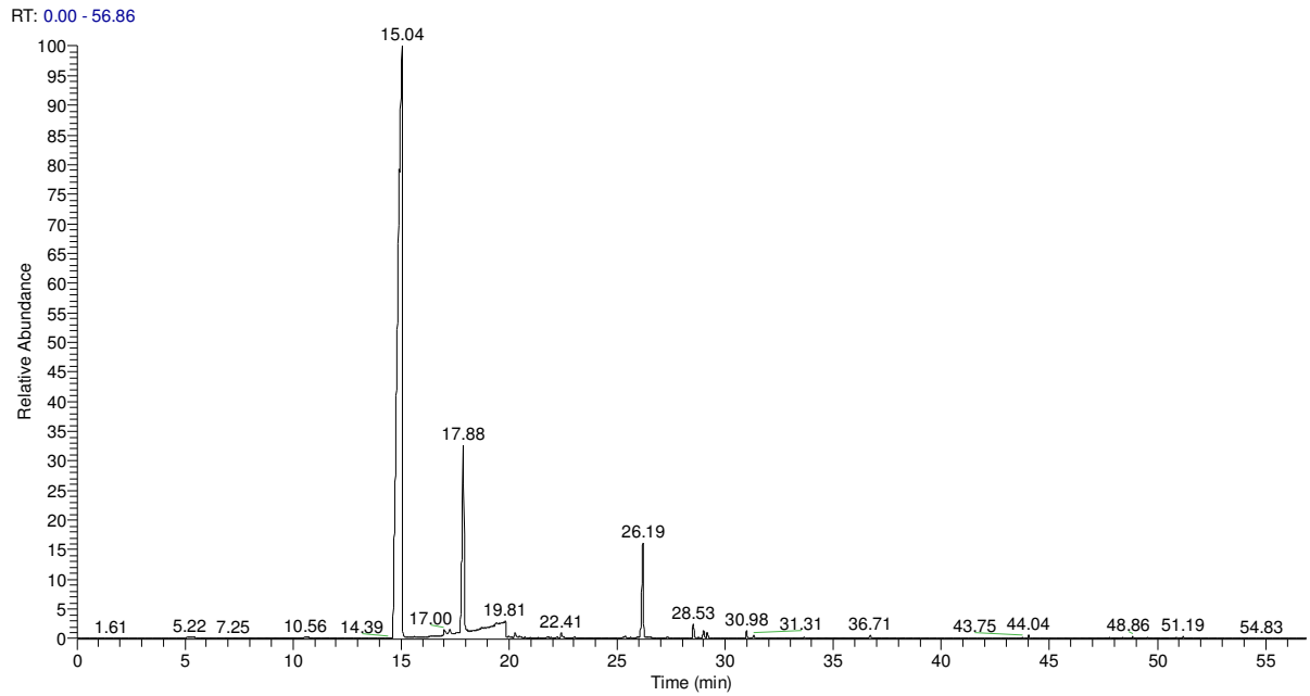
Figura A.17 – Perfil cromatográfico dos compostos voláteis do headspace do genótipo S XVIII.
