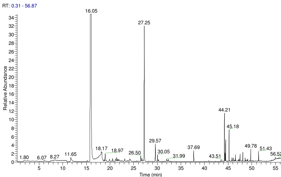
Figura 9 – Cromatogramas do perfil de compostos voláteis extraídos pela fibra de PDMS: (a) Cromatograma total; (b) Cromatograma ampliado.
