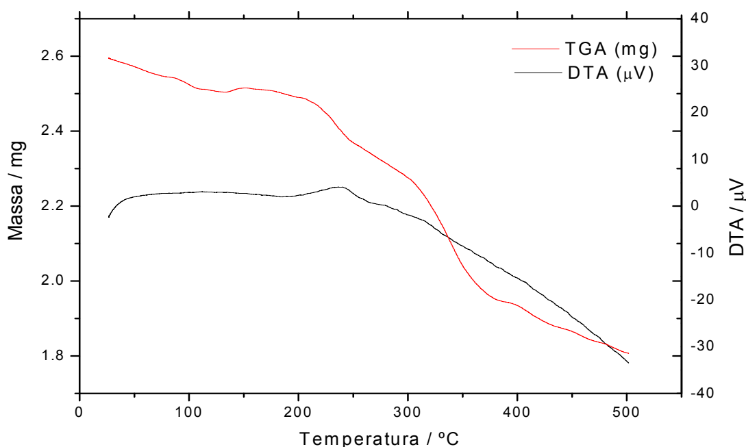
Figura 43 - Curvas TG e DTA para o precursor K_2[Pd\{Pd(opba)\}(OH)_2].H_2O .
