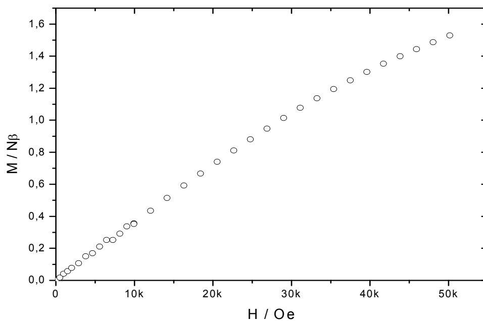
Figura A.2 - Curva de primeira magnetização para o composto heterometálico [\text{Pd}_2(\text{ppba})_2\{\text{Cu}_2(\text{bpca})_2\}].5\text{DMSO}.5\text{H}_2\text{O} .
