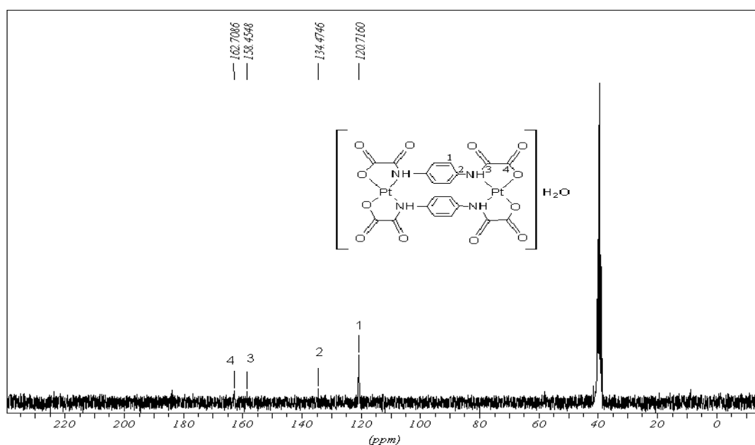
Figura 81 - Espectro de ressonância magnética de carbono para [\text{Pt}_2(\text{ppba})_2]\cdot\text{H}_2\text{O} .
