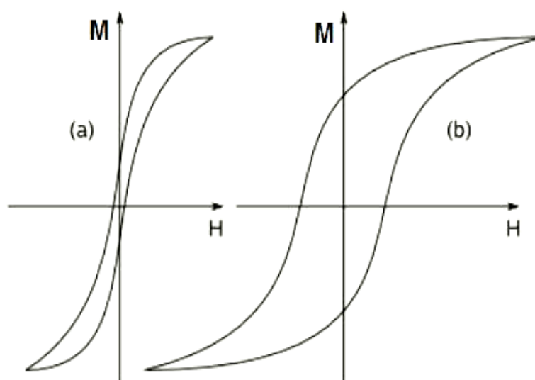
Figura 14 - Comparação entre materiais magnéticos macios (a) e duros (b).
