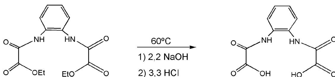
Figura 18 - Esquema de obtenção do ligante ácido H 4 opba.
