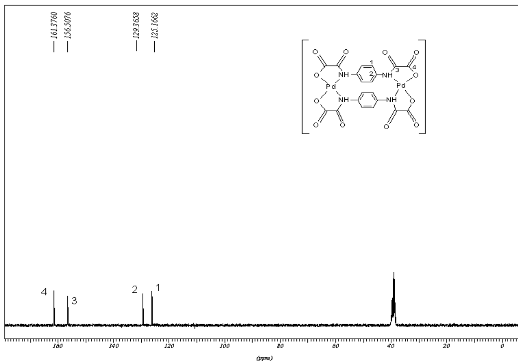
Figura 54 - Espectro de ressonância magnética de carbono para [\text{Pd}_2(\text{ppba})_2]\cdot 4\text{H}_2\text{O} .
