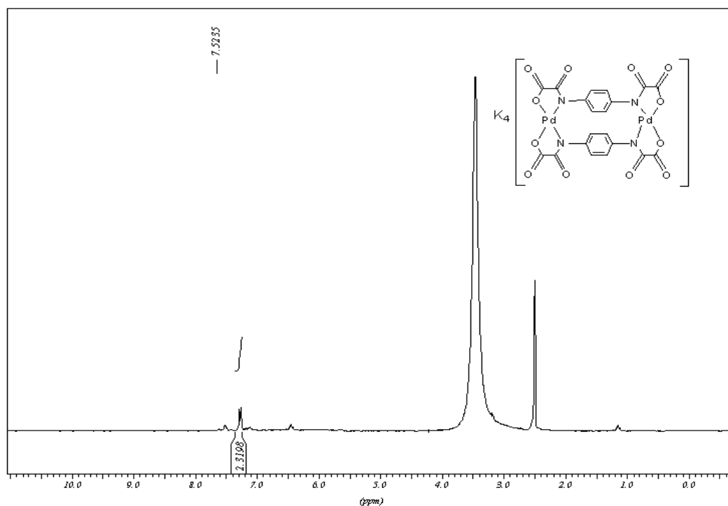
Figura 57 - Espectro de ressonância magnética de próton para K_4[Pd_2(ppba)_2] \cdot 4H_2O
