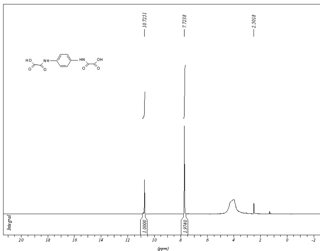
Figura 26 - Espectro de ressonância magnética de próton para o ligante H 4 ppba.
