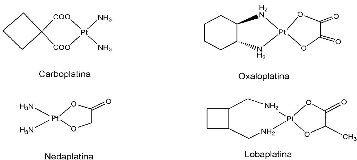
Figura 4 - Medicamentos comercializados contendo platina(II).
