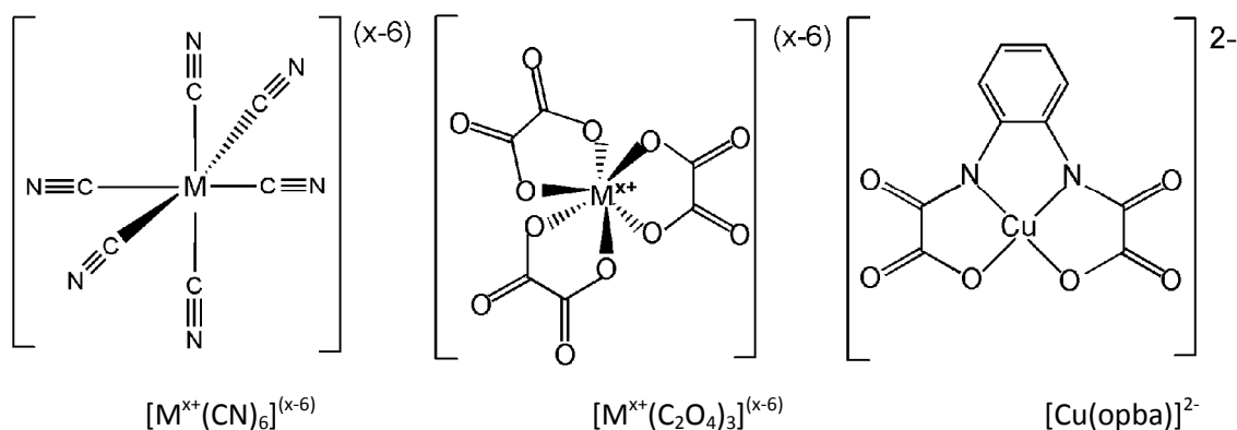
Figura 6 - Exemplos de unidades constituintes utilizadas na obtenção de magnetos moleculares.
