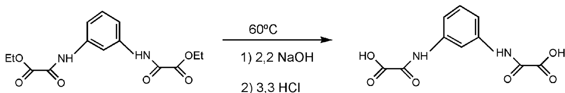
Figura 19 - Esquema de obtenção do ligante ácido H 4 mpba.
