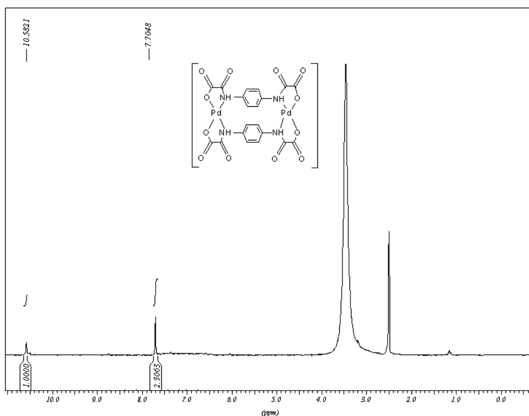
Figura 53 - Espectro de ressonância magnética de próton para [\text{Pd}_2(\text{ppba})_2] \cdot 4\text{H}_2\text{O} .
