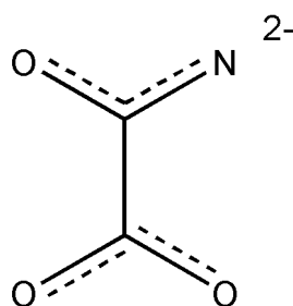
Figura 15 - Esquema de uma ponte oxamato. As linhas pontilhadas representam a deslocalização da nuvem eletrônica \pi .
