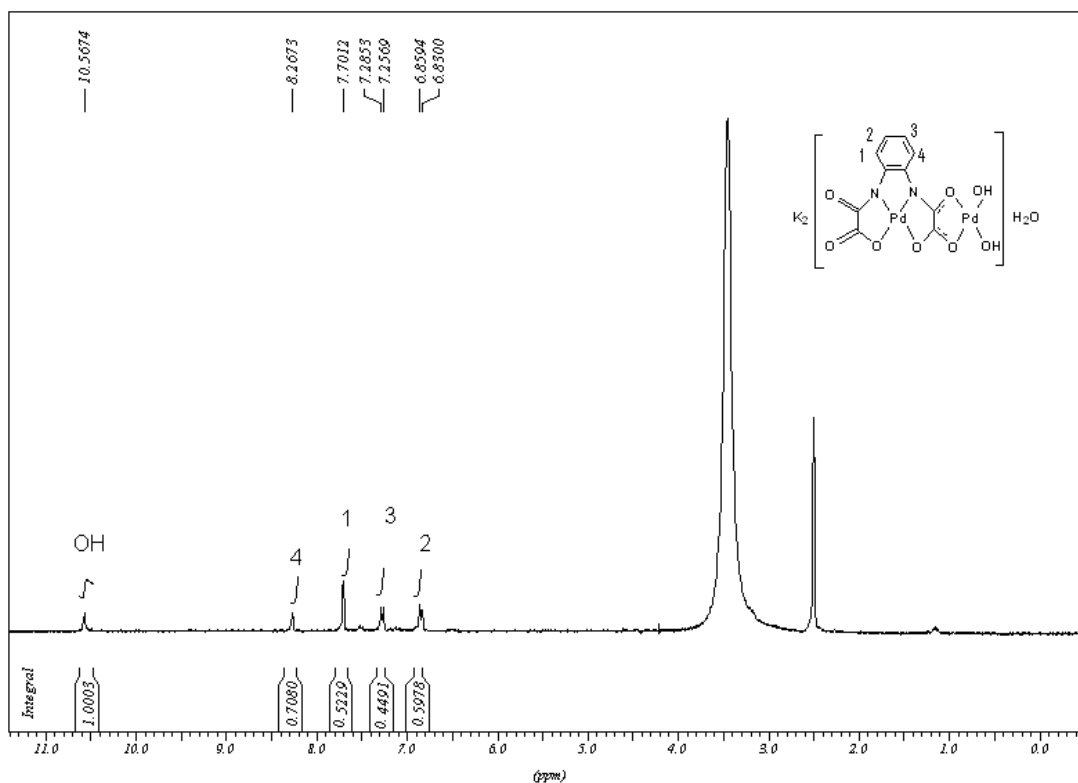
Figura 41 - Espectro de ressonância magnética de próton para \text{K}_2[\text{Pd}\{\text{Pd}(\text{opba})\}(\text{OH})_2]\cdot\text{H}_2\text{O} .
