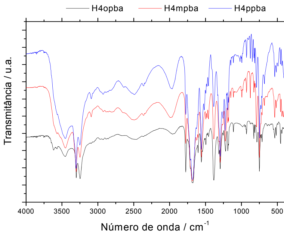
Figura 21 - Espectro qualitativo de absorção na região do IV para os ligantes H 4 opba, H 4 mpba e H 4 ppba.
