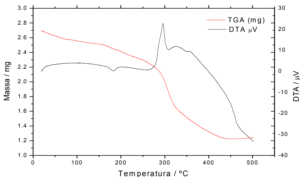
Figura 59 - Curvas TG e DTA para o precursor K 4 [Pd 2 (ppba) 2 ].4H 2 O.
