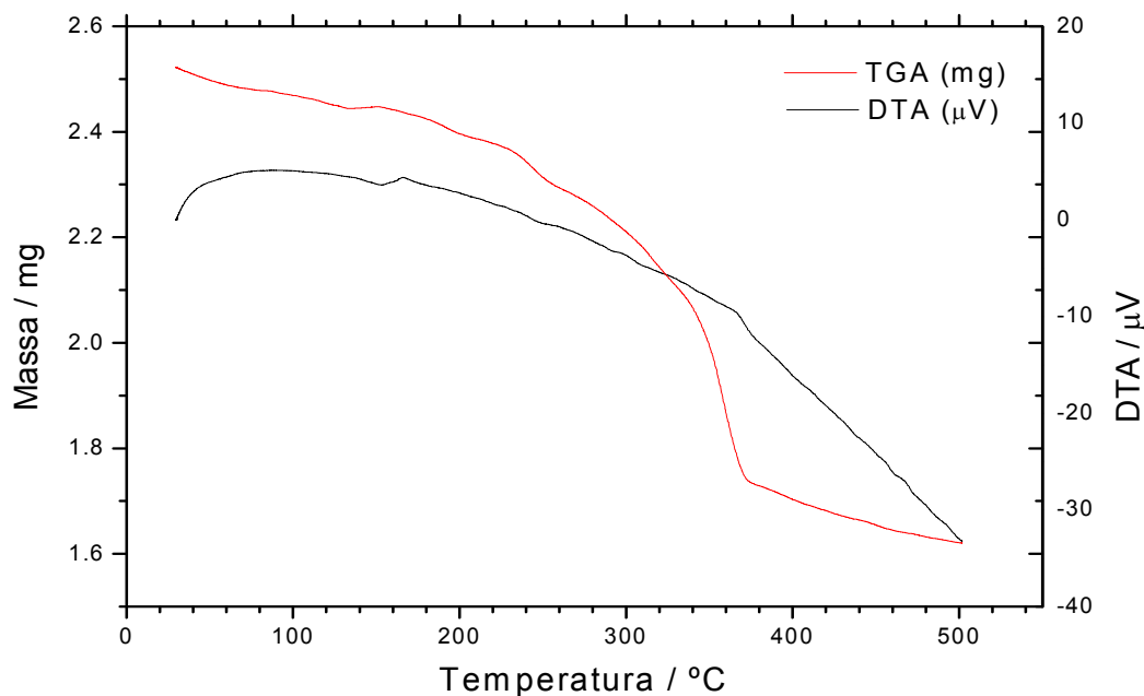
Figura 39 – Curvas TG e DTA para o precursor K 2 [Pd(opba)].H 2 O.
