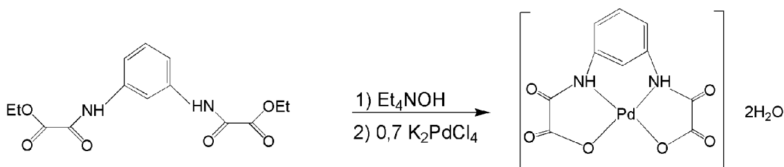
Figura 31 - Esquema de obtenção do precursor [Pd(mpba)].2H 2 O.
