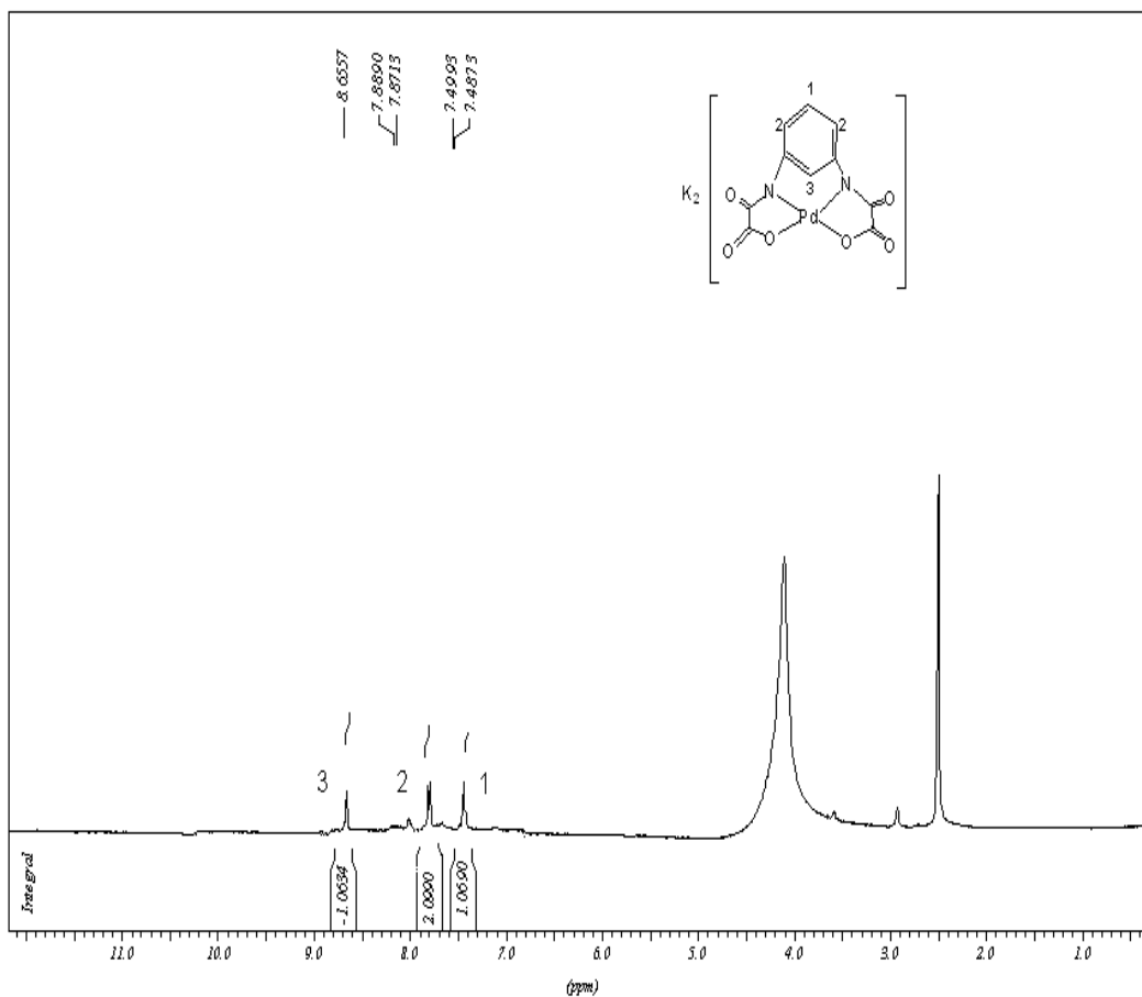
Figura 49 - Espectro de ressonância magnética de próton para K_2[Pd(mpba)].2H_2O .
