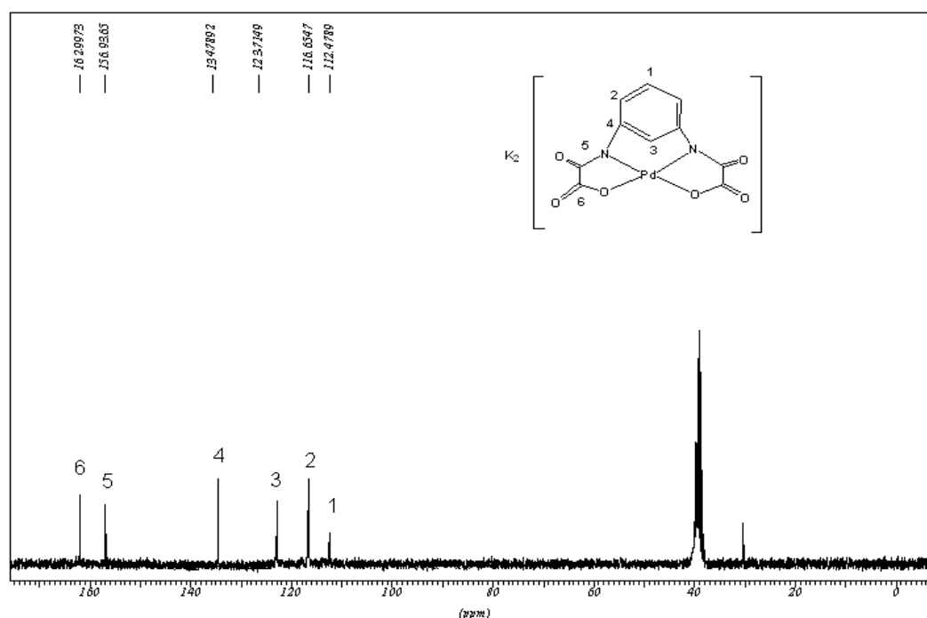
Figura 50 - Espectro de ressonância magnética de carbono para K 2 [Pd(mpba)].2H 2 O.
