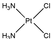
Figura 3 - Representação da estrutura da Cisplatina.
