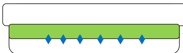
Figura 8 - Placa de Petri utilizada em um experimento de evaporação lenta.
