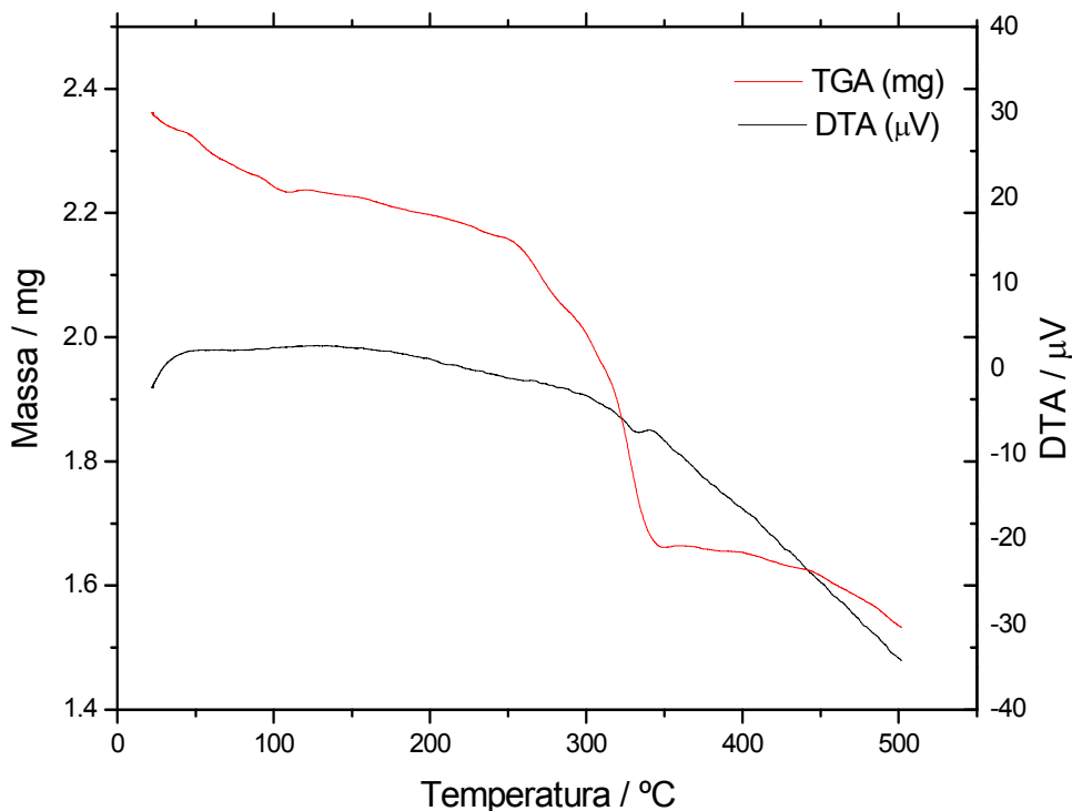
Figura 51 – Curvas TG e DTA para o precursor K_2[Pd(mpba)].2H_2O .
