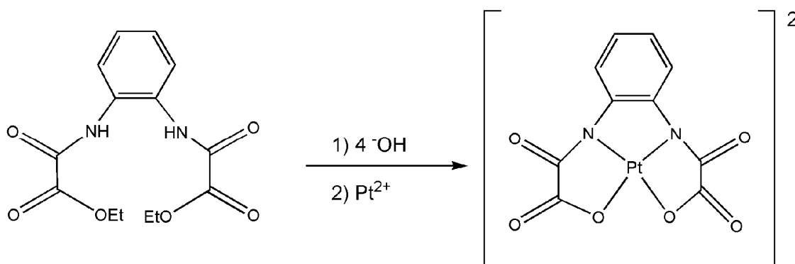
Figura 72 - Esquema geral para a síntese da unidade construtora [Pt(opba)]^{2-} .
