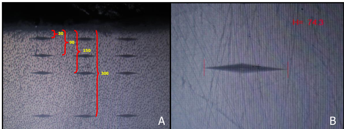
Figura 11: A- Marcações realizadas no espécime em triplicata nas quatro profundidades (30 \mu\text{m} , 90 \mu\text{m} , 150 \mu\text{m} , 300 \mu\text{m} ) (aumento 100x); B- Determinação das extremidades do losângulo para determinação da medida de microdureza Knoop (aumento de 400x).
