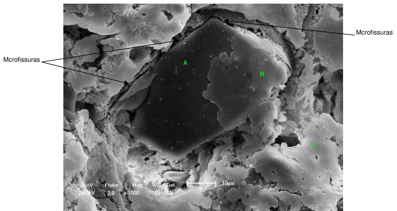
Figura 4.32 – Detalhe de uma partícula de quartzo “imersa” em fase vítrea no corpo de prova da formulação DN15, com aumento de 1000x.
