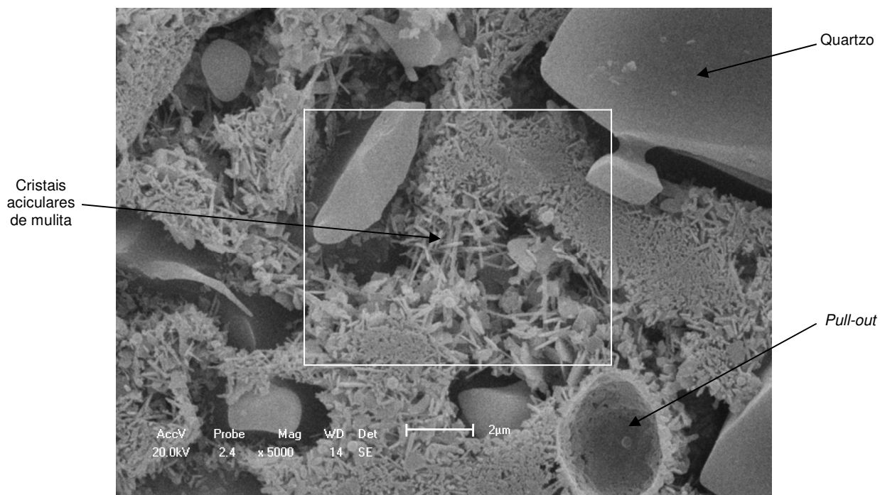
Figura 4.37 – Detalhe das partículas de quartzo e cristais aciculares do corpo de prova da formulação DN10, com aumento de 5000x.
