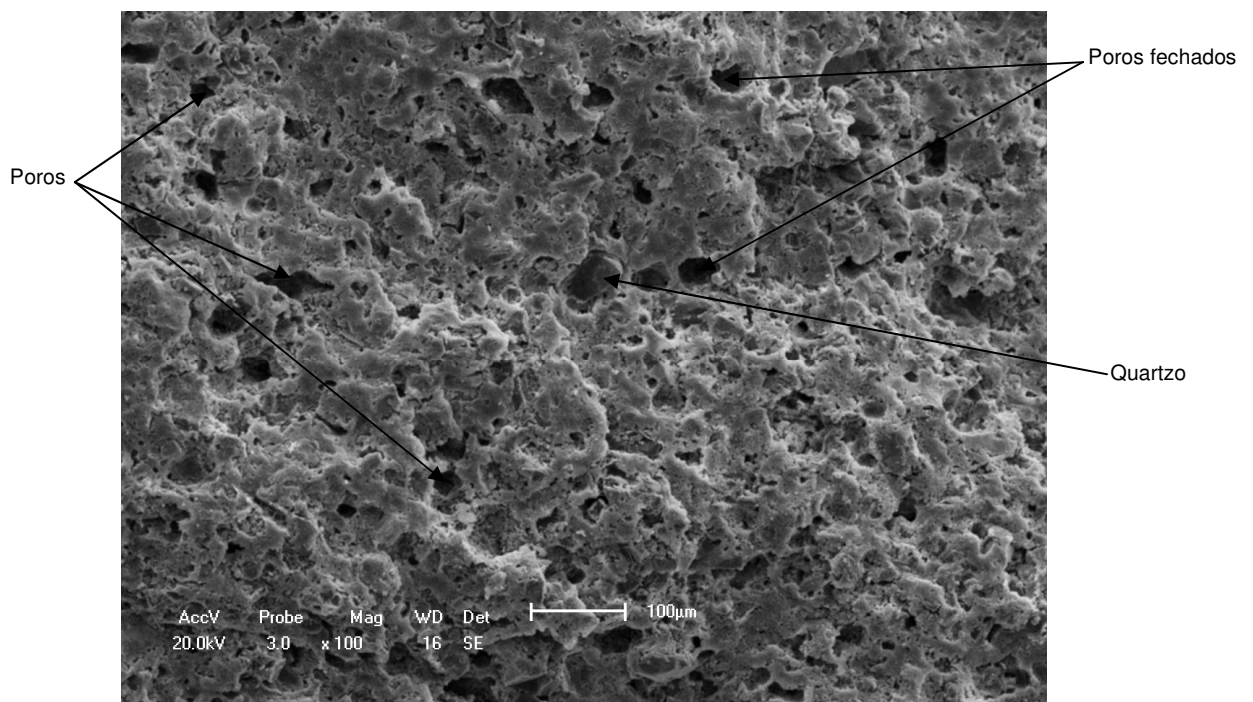
Figura 4.29 – Superfície de fratura de um corpo de prova da formulação DN15, com aumento de 100x.
