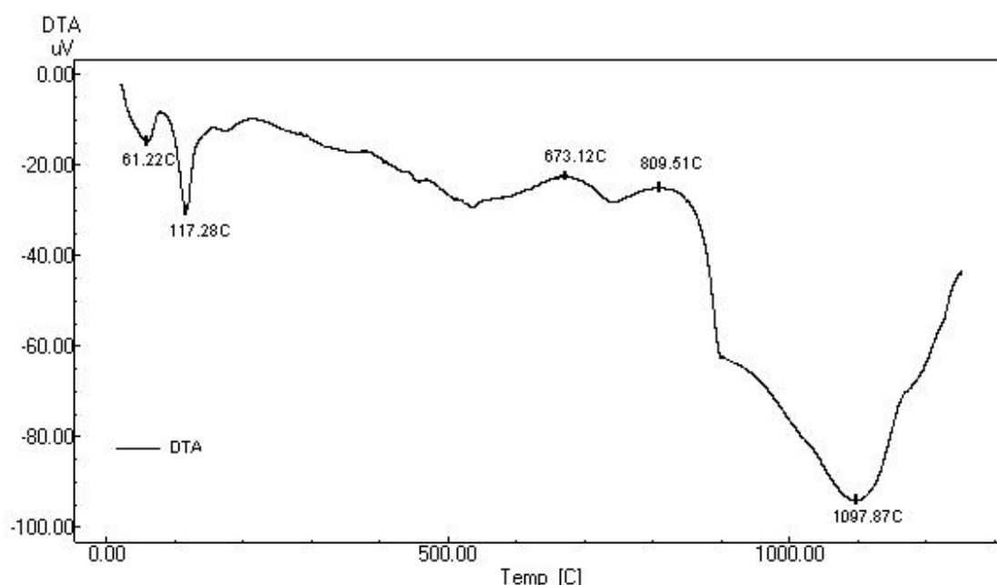
Figura 4.8 – Análise térmica diferencial da cinza.
