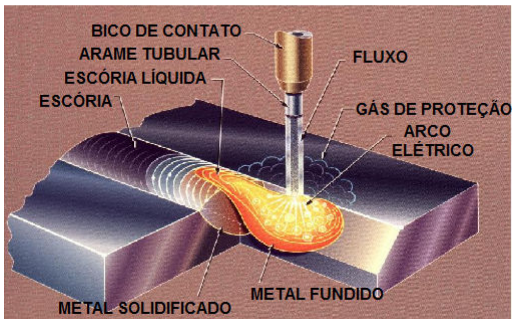
Figura 3.13 - Esquema de soldagem com arame tubular pelo processo FCAW-S adaptado de Welding Handbook (1991).
