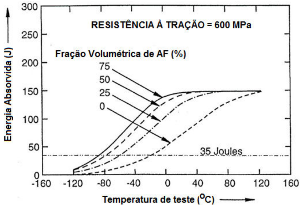
Figura 3.21 - Influência do teor de AF na energia absorvida por impacto CHARPY. (GRONG, 1994).
