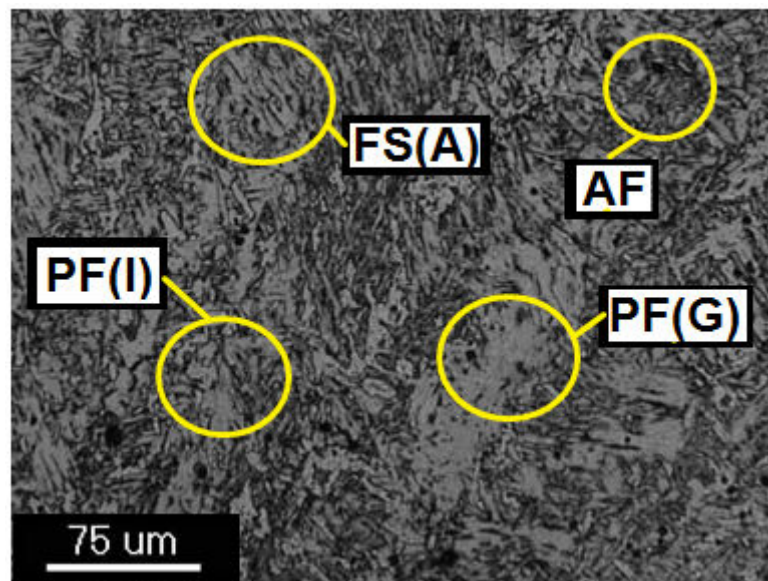
Figura 5.25 - Microestrutura no metal de solda do processo M2, MO. 200X, Nital 1%.
