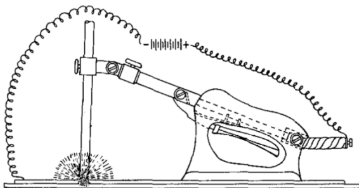
Figura 3.15 – Ilustração da primeira patente de processo de soldagem. (The Lincoln Electric Company, 1973)
