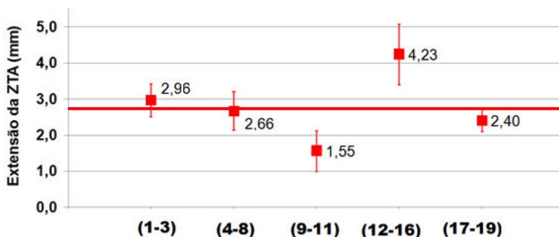
Figura 5.4 - Valores médios em cada grupo de medidas na ZTA para processo M2.
