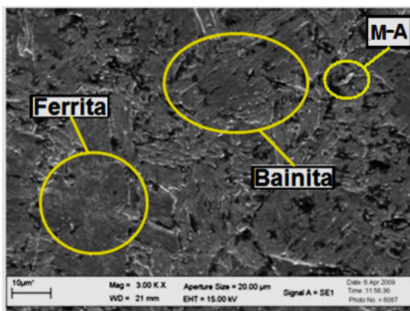
Figura 5.8 - Microestrutura na região da ZTA GG, processo M1, MEV. 3000X, Nital 3%.
