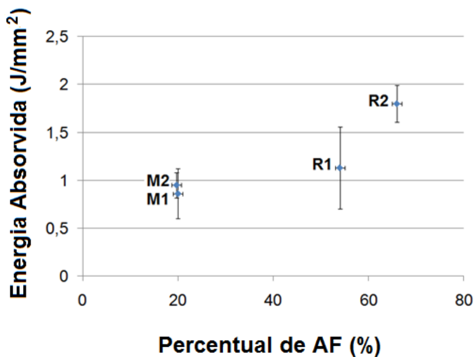
Figura 5.61 – Relação entre o percentual de AF e a energia absorvida em ensaio charpy, entalhe no passe de raiz.
