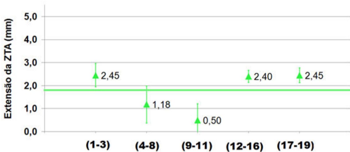
Figura 5.5 - Valores médios em cada grupo de medidas na ZTA para processo R1. Média=1,796
