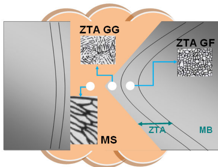
Figura 4.8 - Representação das regiões da junta soldada.
