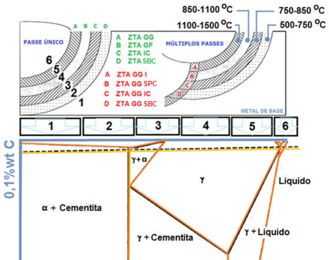
Figura 3.18 - Principais regiões da junta soldada, adaptado de (DAVIS & KING, 1994; BHADESHIA & HONEYCOMBE, 2006).
