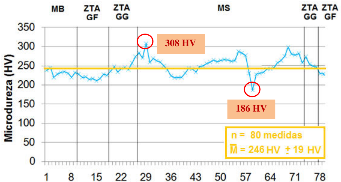
Figura 5.43 - Medidas de microdureza na linha intermediária da junta soldada. Processo R2.
