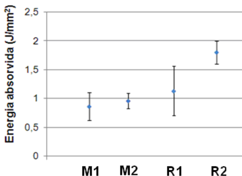
Figura 5.45 - Energia absorvida no ensaio de impacto Chapy. Corpos de prova com entalhe posicionado no passe de raiz.
