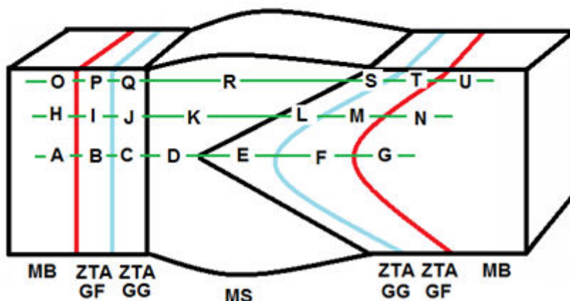
Figura 5.44 - Representação geral das médias de microdureza em todas as regiões da junta soldada, processo R2.
