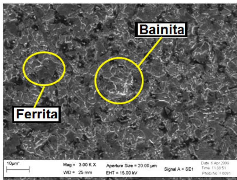
Figura 5.23 - Microestrutura na região da ZTA GF, processo R2, MEV. 3000X, Nital 3%.
