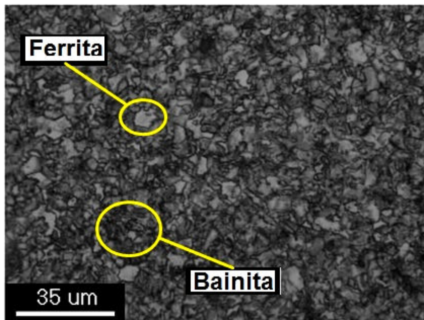
Figura 5.18 - Microestrutura na região da ZTA GF, processo M2, MO. 500X, Nital 1%.
