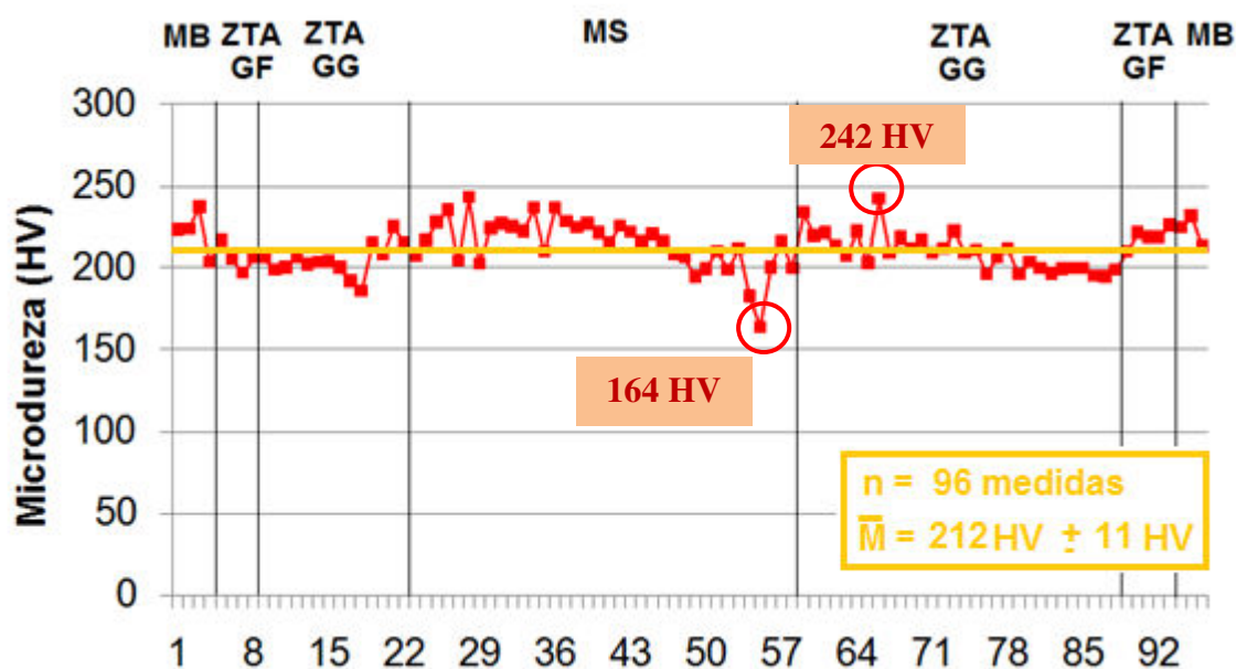
Figura 5.34 - Medidas de microdureza na linha intermediária da junta soldada, processo M2.
