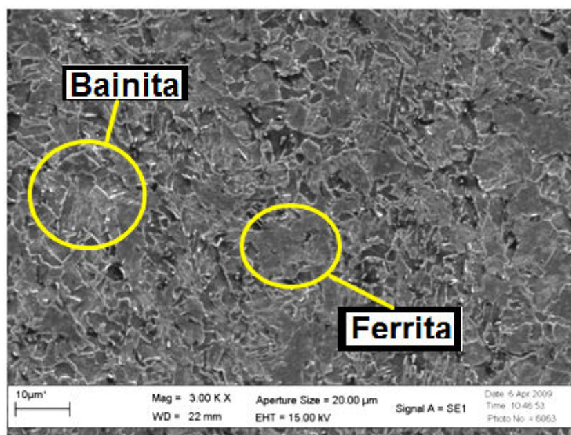
Figura 5.21 - Microestrutura na região da ZTA GF, processo R1, MEV. 3000X, Nital 3%.
