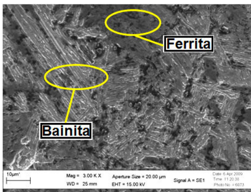
Figura 5.15 - Microestrutura na região da ZTA GG, processo R2, MEV. 3000X, Nital 3%.
