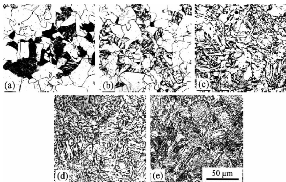
Figura 3.8 - Microestruturas de um aço API 5L X80 com diversas taxas de resfriamento. a) Taxa de resfriamento de 0,1^{\circ}\text{C/s} : microestrutura de PF + B; b) Taxa de resfriamento de 0,3^{\circ}\text{C/s} : microestrutura de PF + B; c) Taxa de resfriamento de 1^{\circ}\text{C/s} : microestrutura de QF + GF; d) Taxa de resfriamento de 18^{\circ}\text{C/s} : microestrutura de GF; e) Taxa de resfriamento de 95^{\circ}\text{C/s} : microestrutura de BF + M (CIZEK et al., 2005).
