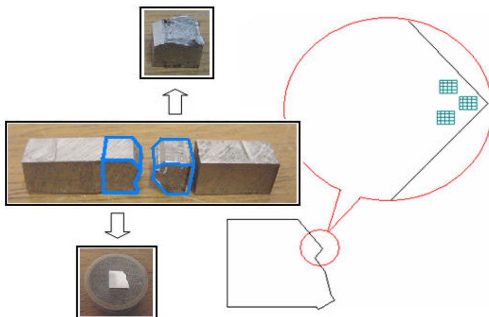
Figura 4.16 –Procedimento de análise da fratura por MO (com embutimento) e MEV (sem embutimento).
