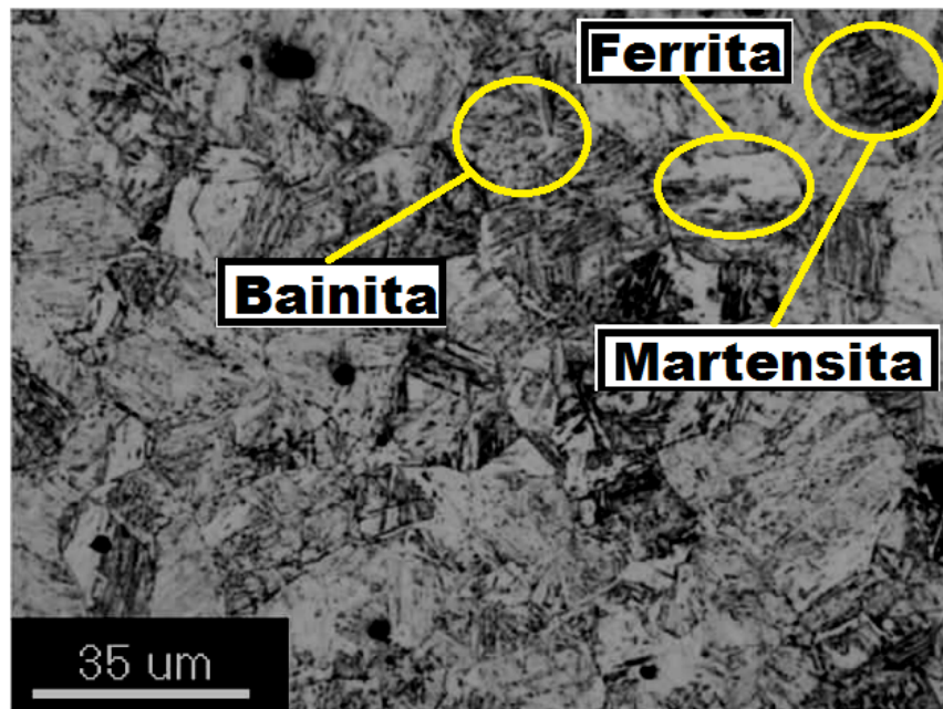
Figura 5.11 - Microestrutura na região da ZTA GG, processo R1, MO. 500X, Nital 1%.
