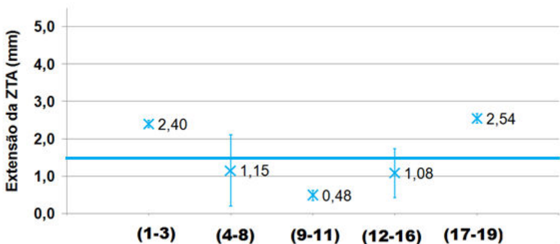
Figura 5.6 - Valores médios em cada grupo de medidas na ZTA para processo R2. Média=1,53
