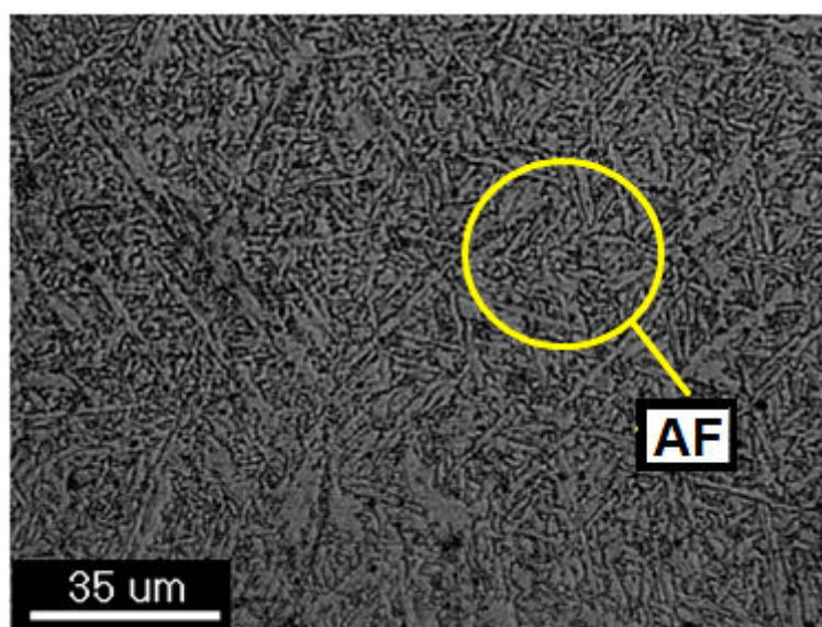
Figura 5.28 - Microestrutura no metal de solda do processo R2, MO. 500X, Nital 1%.
