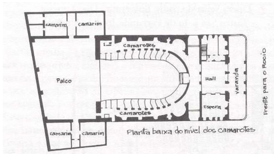
Fig. 2 Planta baixa do Teatro São João de Fernando José de Almeida.
