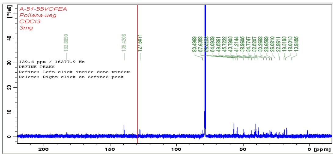
Figura 29: Espectro de RMN 13 C (125 MHz, CDCl 3 ) do 51-55 VCFEA.
