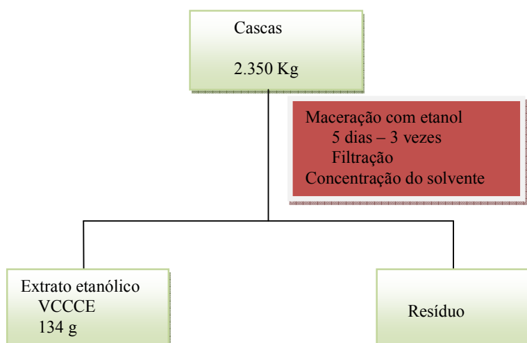
Figura 11: Fluxograma de obtenção do extrato bruto das cascas de V. cinnamomea .
