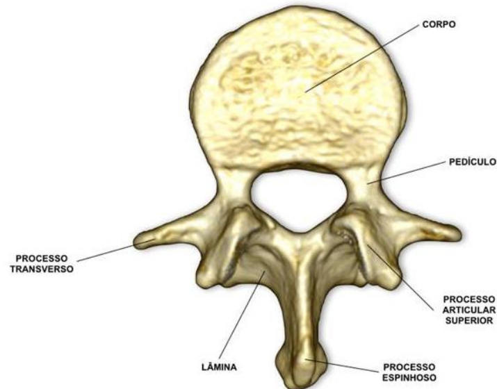
Figura 4 – Vértebra lombar em vista superior mostrando os principais elementos anatômicos que a compõe. (Reconstrução tridimensional a partir de imagens de Tomografia Computadorizada).
