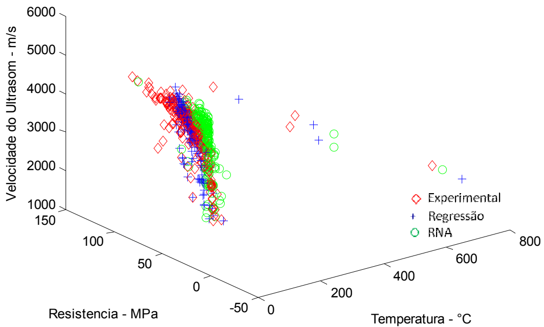
Figura 7.28: Relação VPU x f_c – rede 7x2x20x4x1 – Dados de Teste
