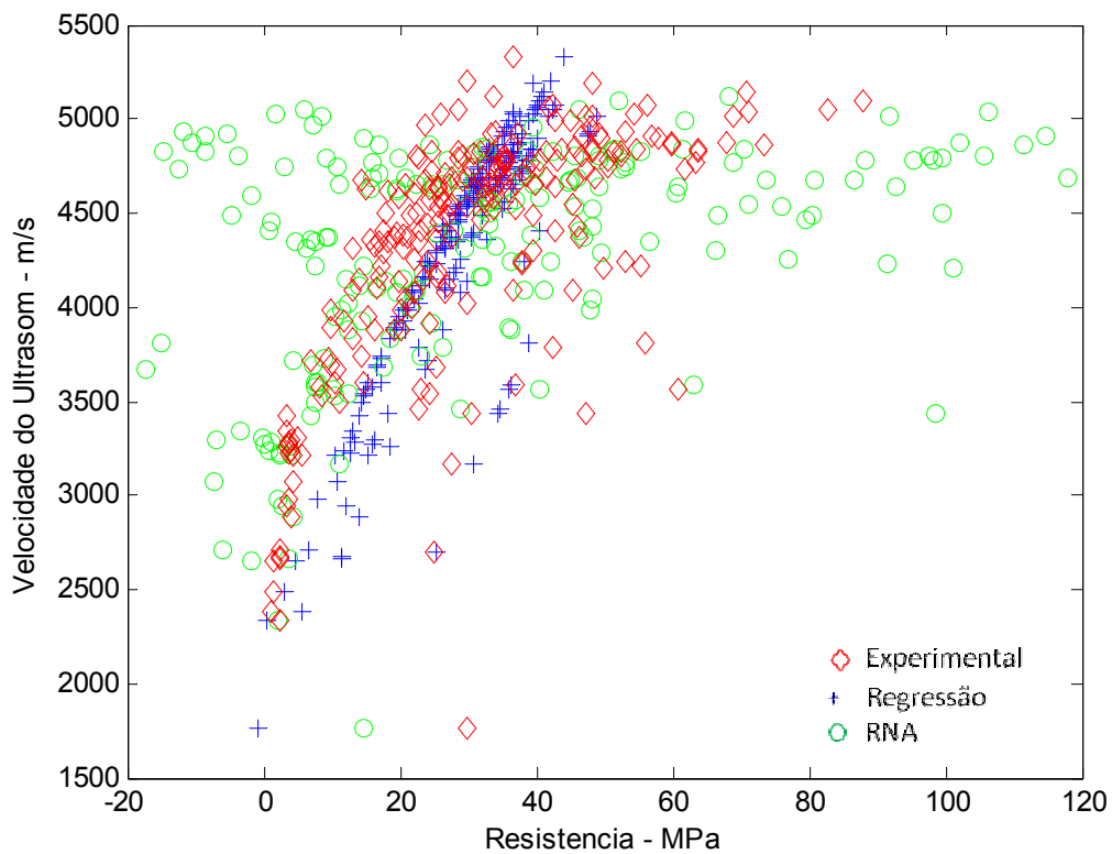
Figura 7.54: Relação VPU x f_c – rede 7x6x20x20x1 – Dados de Teste
