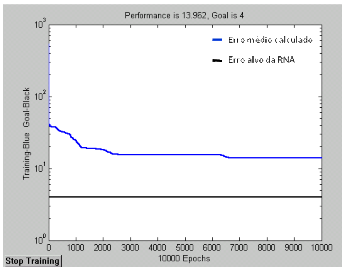
Figura 6.4: treinamento da RNA para 10000 épocas – 2x4x16x1
