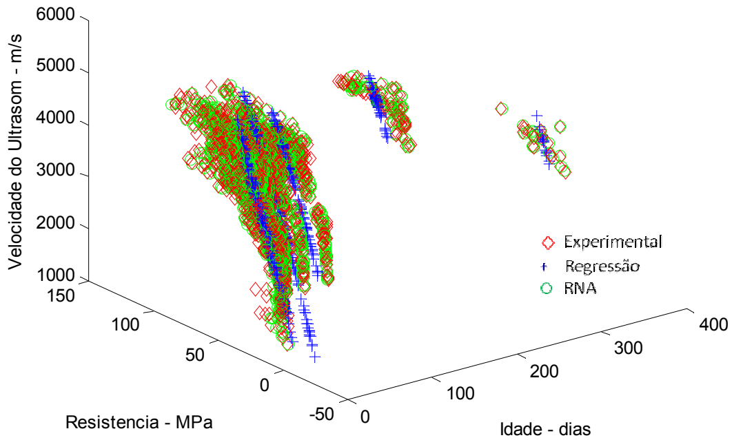
Figura 7.39: Relação VPU x f_c x Idade – rede 7x6x20x12x1 – Dados de Treinamento
