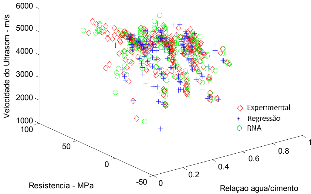
Figura 7.66: Relação VPU x F_c x Relação a/c – rede 7x8x20x20x1 – Dados de Teste
