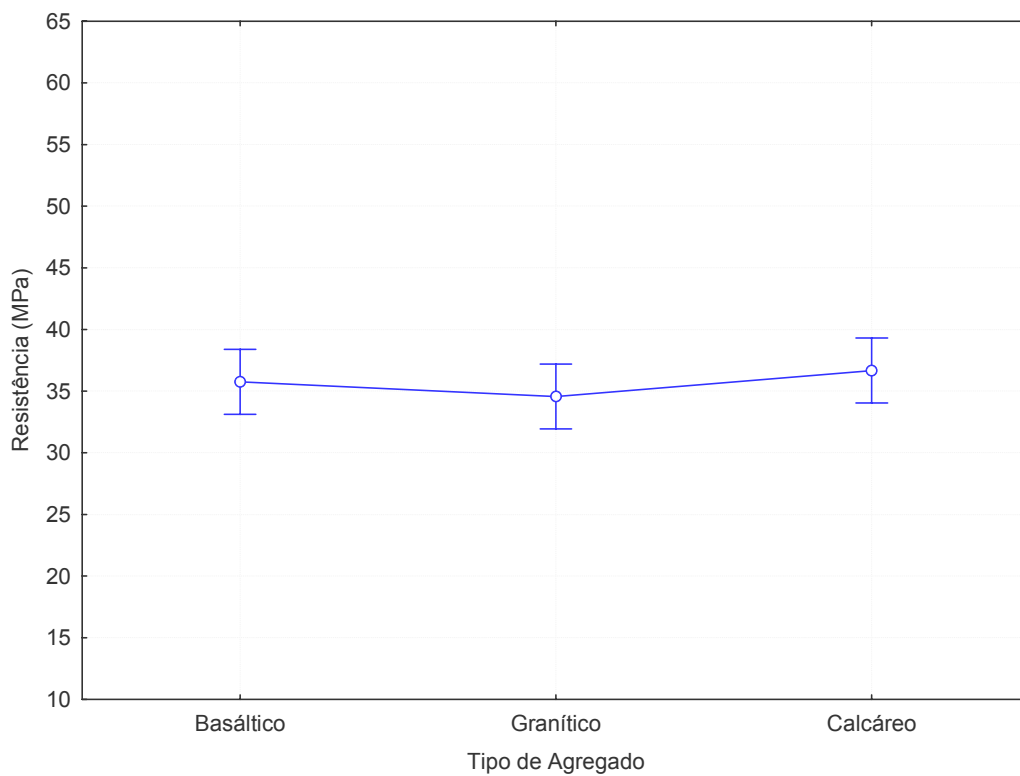
Figura 5.6: influência do tipo de agregado no Ensaio de Resistência Mecânica à Compressão
