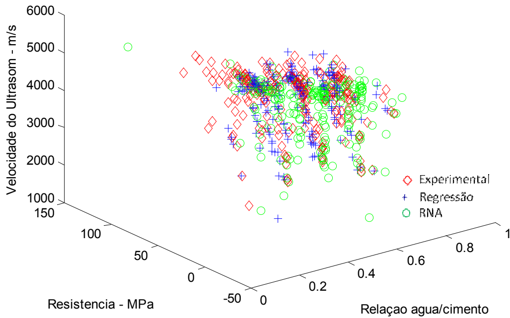
Figura 7.50: Relação VPU x f_c x Relação a/c – rede 7x2x20x20x1 – Dados de Teste
