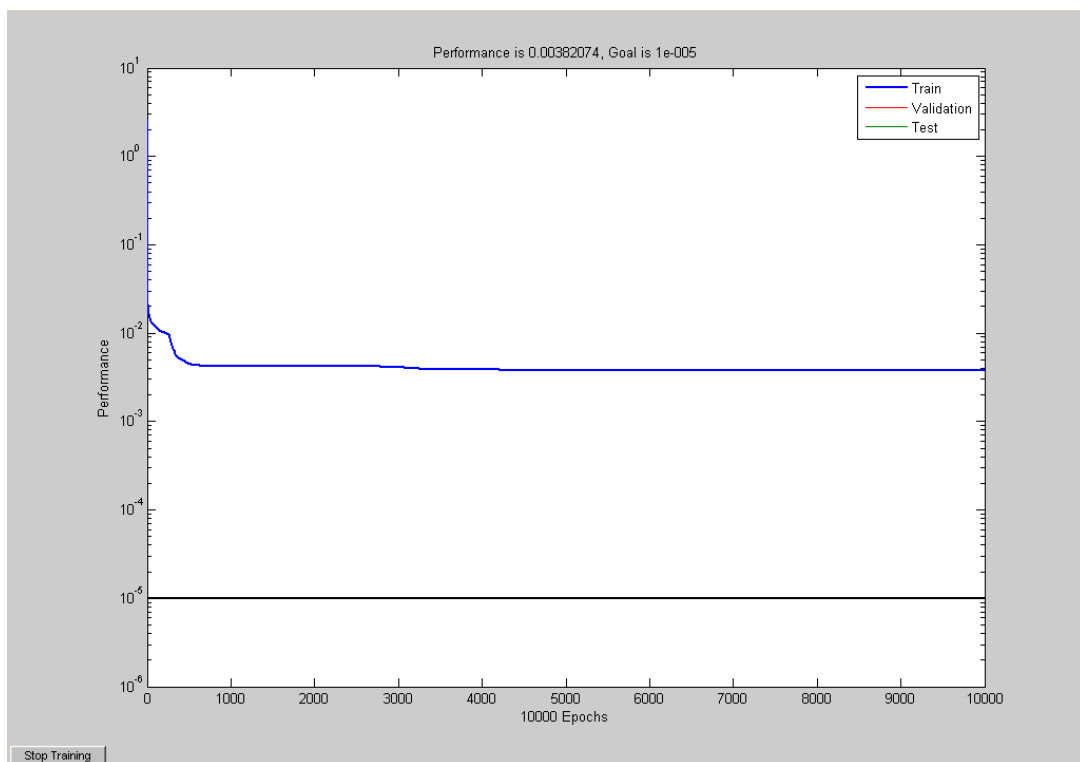
Figura 7.7: evolução do treinamento da RNA para 10000 épocas – Rede 7x8x20x20x1
