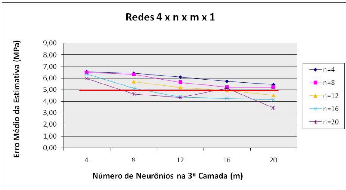
Figura 7.9: Erro médio da estimativa – Redes com 4 neurônios na 1ª camada oculta.
