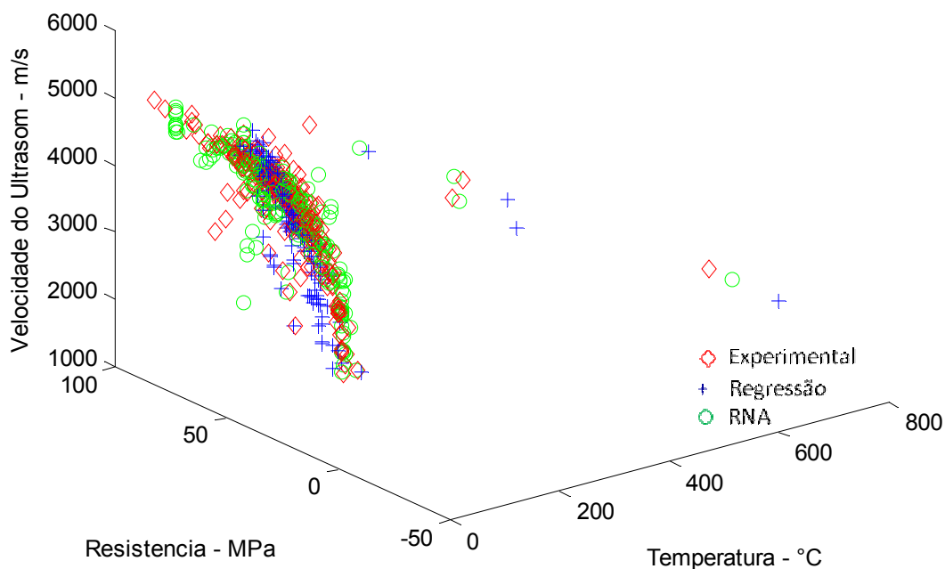
Figura 7.36: Relação VPU x f_c x Temperatura – rede 7x4x20x4x1 – Dados de Teste
