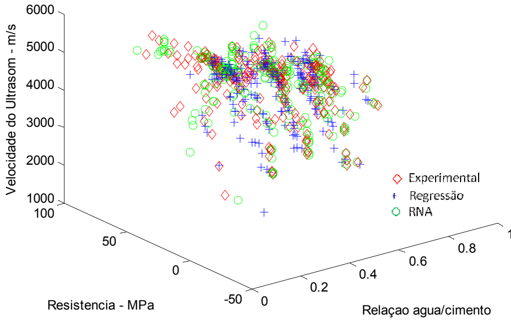
Figura 7.34: Relação VPU x f_c x Relação a/c – rede 7x4x20x4x1 – Dados de Teste
