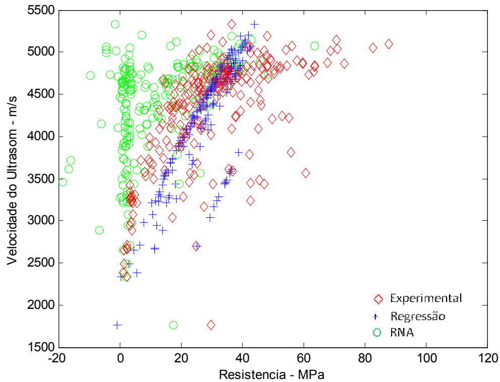
Figura 7.46: Relação VPU x f_c – rede 7x2x20x20x1 – Dados de Teste
