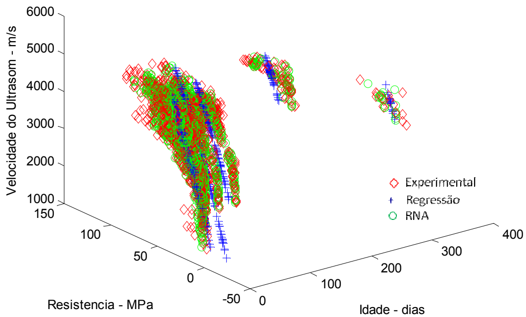
Figura 7.63: Relação VPU x f_c x Idade – rede 7x8x20x20x1 – Dados de Treinamento
