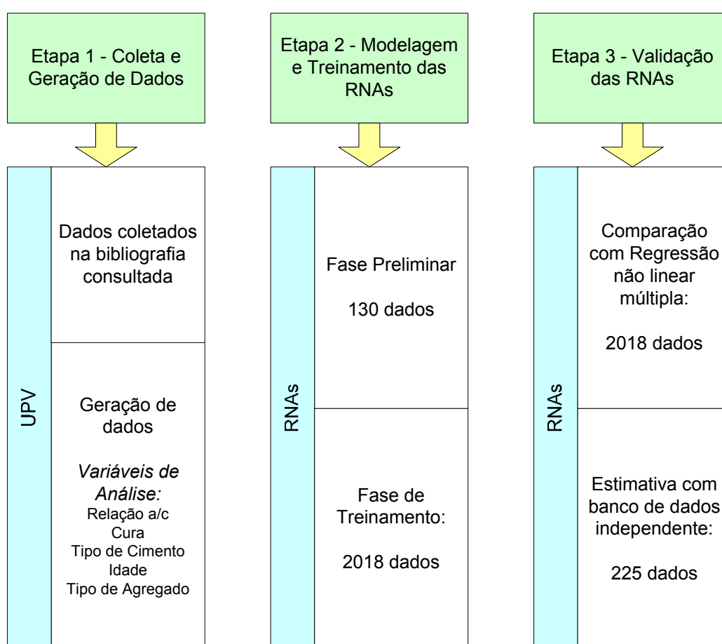
Figura 4.1: fluxograma do programa experimental
