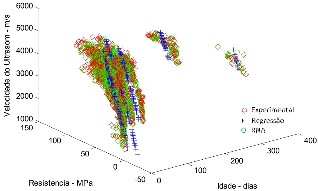
Figura 7.23: Relação VPU x f_c x Idade – rede 7x2x20x4x1 – Dados de Treinamento.
