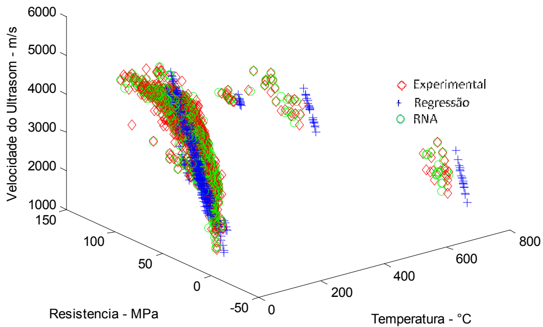
Figura 7.51: Relação VPU x f_c x Temperatura – rede 7x2x20x20x1 – Dados de Treinamento
