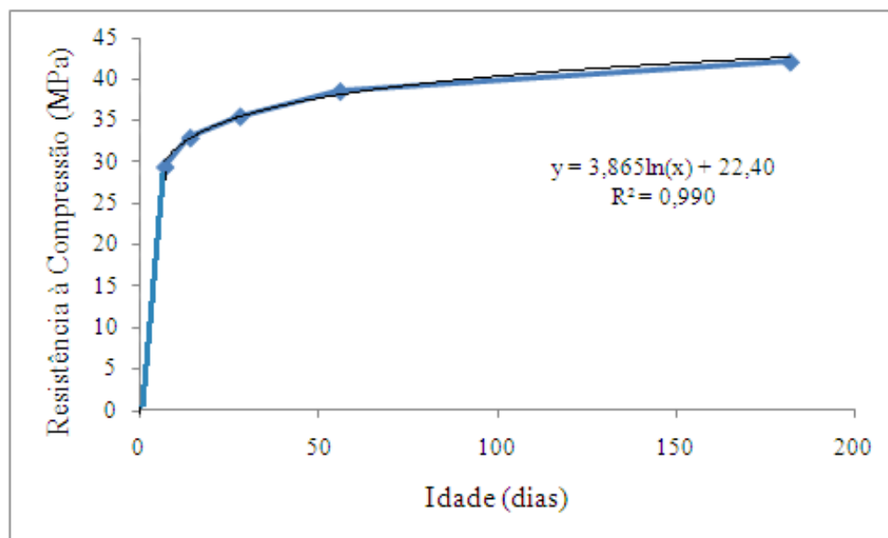
Figura 5.12: influência da idade no Ensaio de Resistência Mecânica à Compressão
