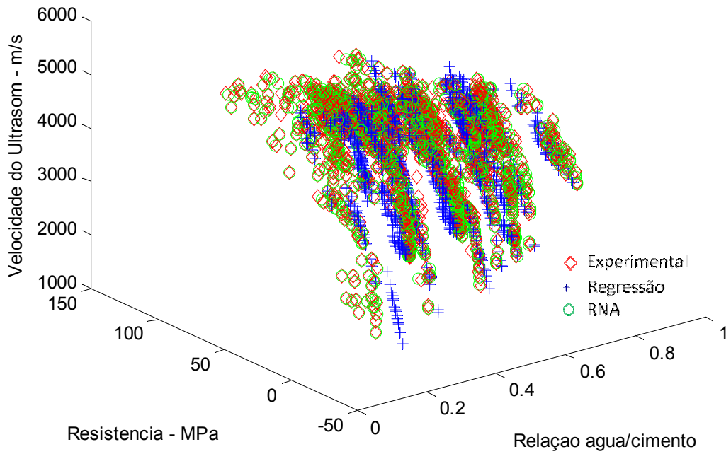
Figura 7.57: Relação VPU x f_c x Relação a/c – rede 7x6x20x20x1 – Dados de Treinamento
