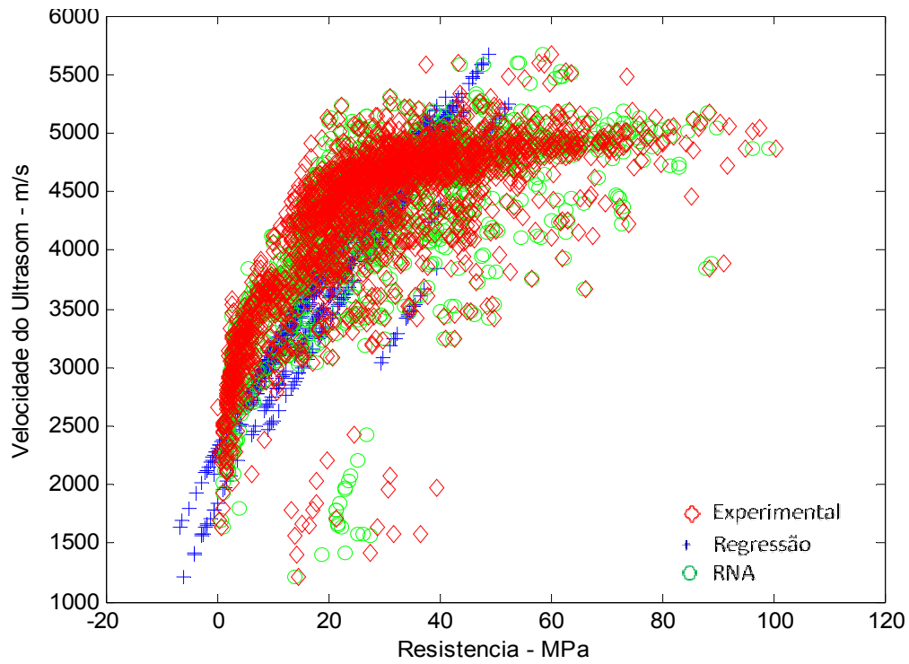
Figura 7.37: Relação VPU x f_c – rede 7x6x20x12x1 – Dados de Treinamento
