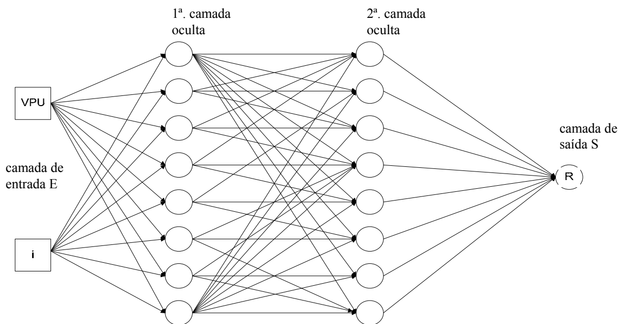
Figura 6.1: Rede neural utilizada na fase preliminar.
