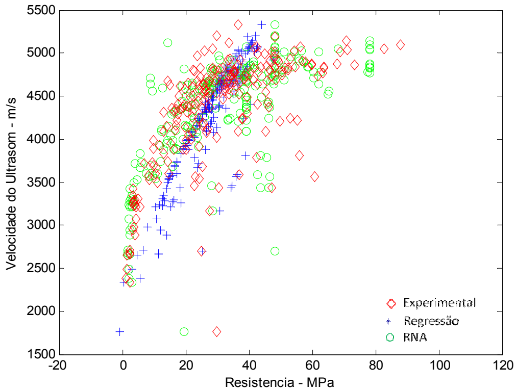
Figura 7.62: Relação VPU x f_c – rede 7x8x20x20x1 – Dados de Teste
