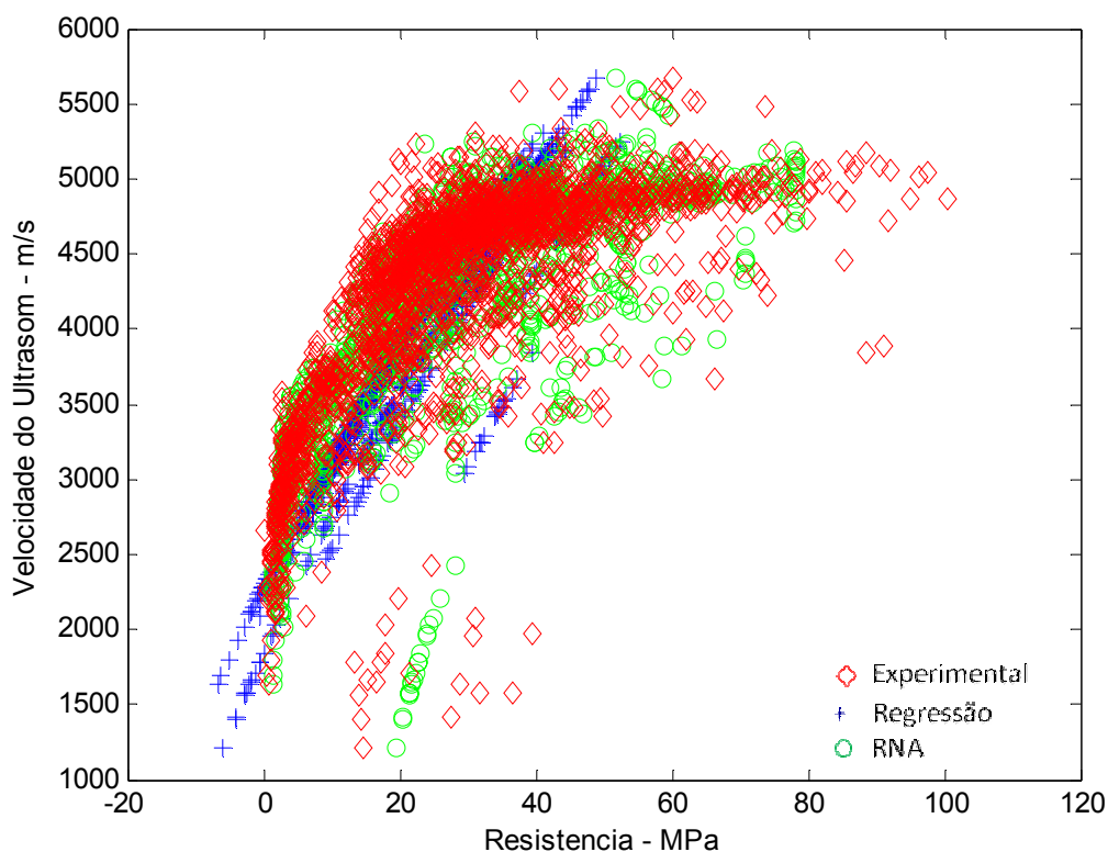
Figura 7.61: Relação VPU x f_c – rede 7x8x20x20x1 – Dados de Treinamento
