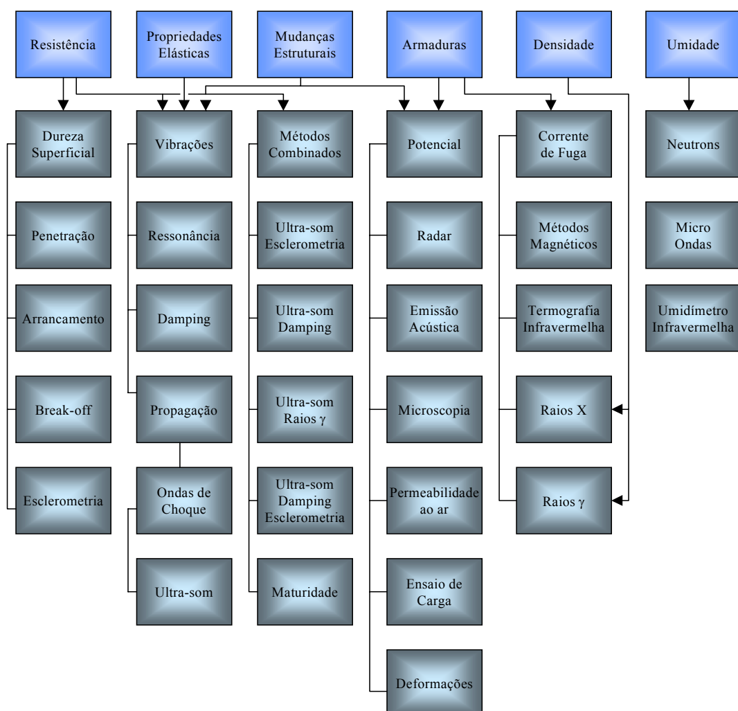
Figura 2.1: ensaios não destrutivos utilizados no concreto (Teodoru e Mommens apud HAMASSAKI, 1993).
