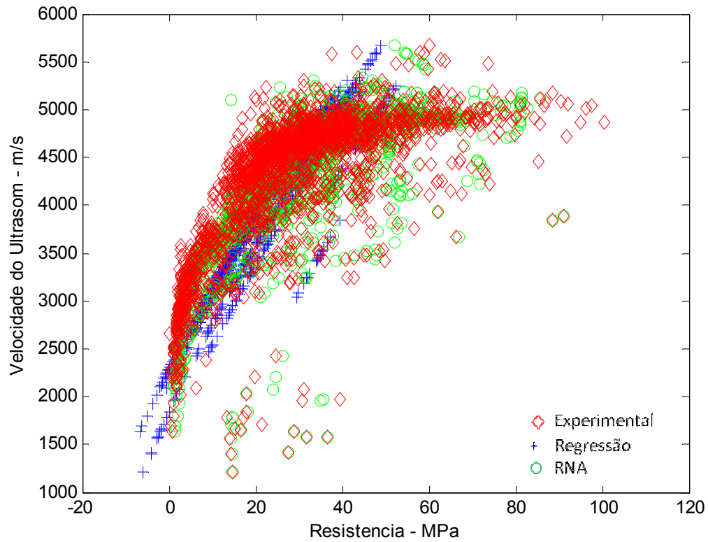
Figura 7.21: Relação VPU x f_c – rede 7x2x20x4x1 – Dados de Treinamento
