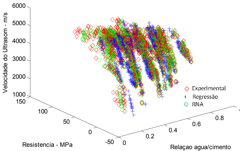
Figura 7.33: Relação VPU x f_c x Relação a/c – rede 7x4x20x4x1 – Dados de Treinamento
