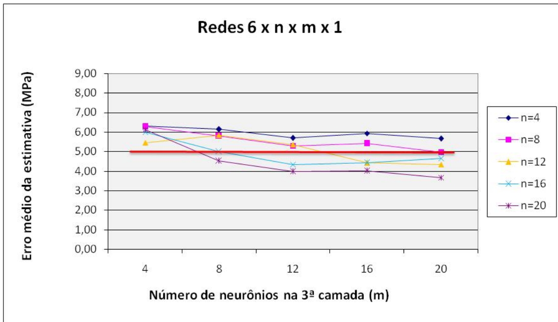
Figura 7.10: Erro médio da estimativa – Redes com 6 neurônios na 1ª camada oculta
