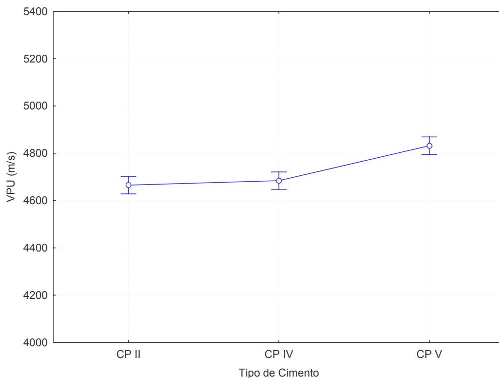
Figura 5.15: influência do tipo de cimento no Ensaio de VPU
