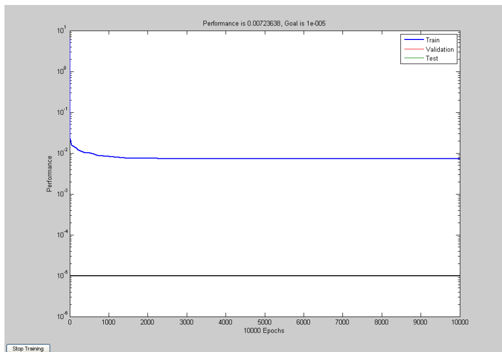
Figura 7.6: evolução do treinamento da RNA para 10000 épocas – Rede 7x8x16x20x1
