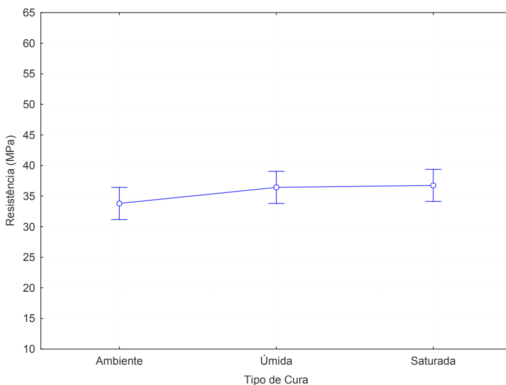
Figura 5.8: influência do tipo de cura no Ensaio de Resistência Mecânica à Compressão
