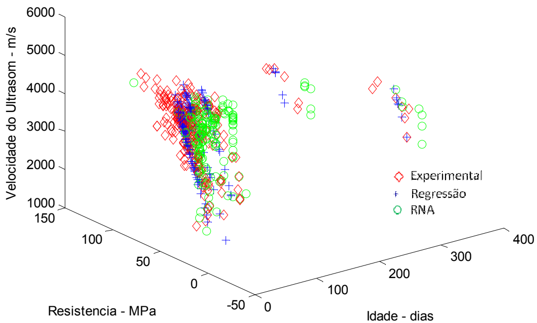
Figura 7.24: Relação VPU x f_c x Idade – rede 7x2x20x4x1 – Dados de Teste
