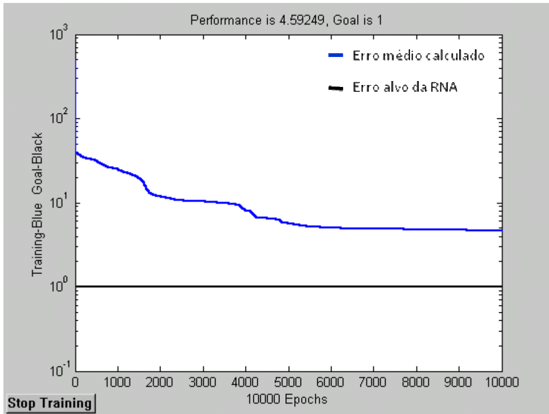
Figura 6.6: treinamento da RNA para 6986 épocas – 2x8x48x1
