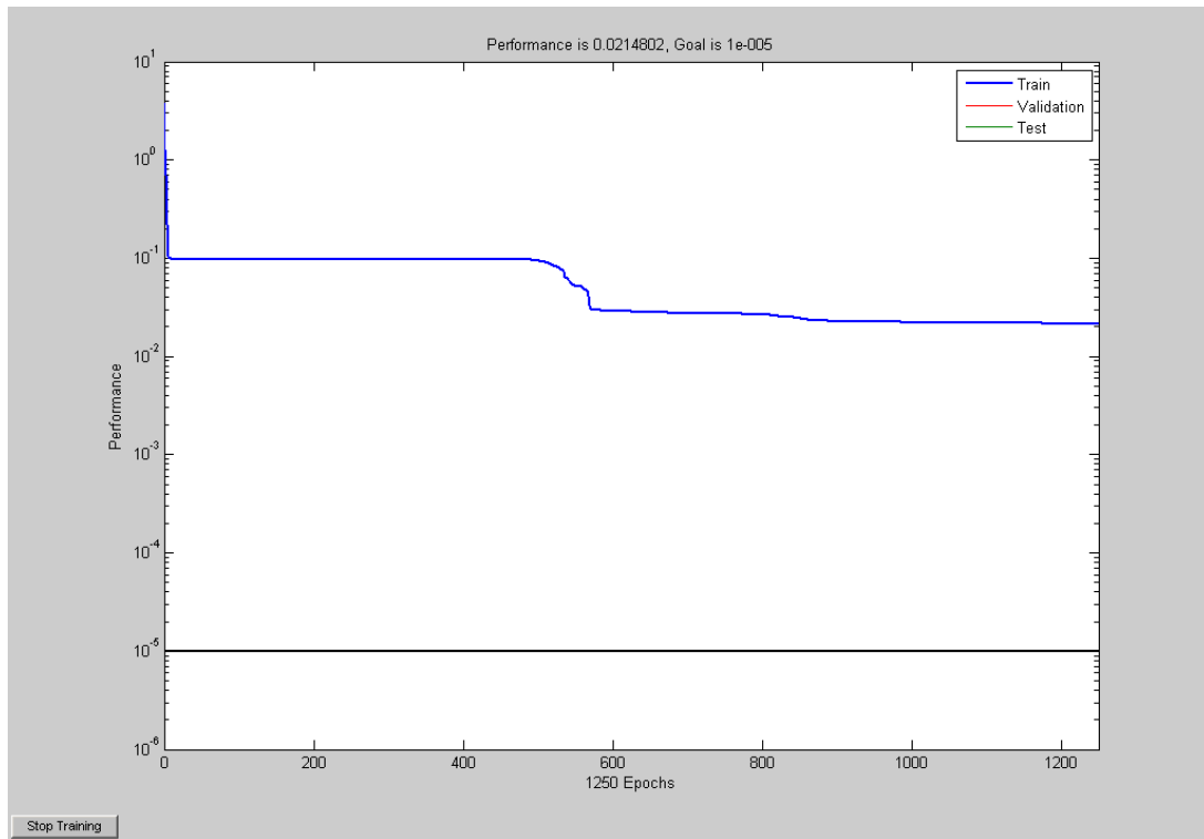
Figura 7.2: evolução do treinamento da RNA para 1250 épocas – Rede 7x2x8x16x1
