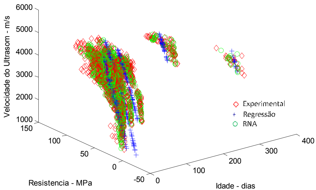
Figura 7.31: Relação VPU x f_c x Idade – rede 7x4x20x4x1 – Dados de Treinamento
