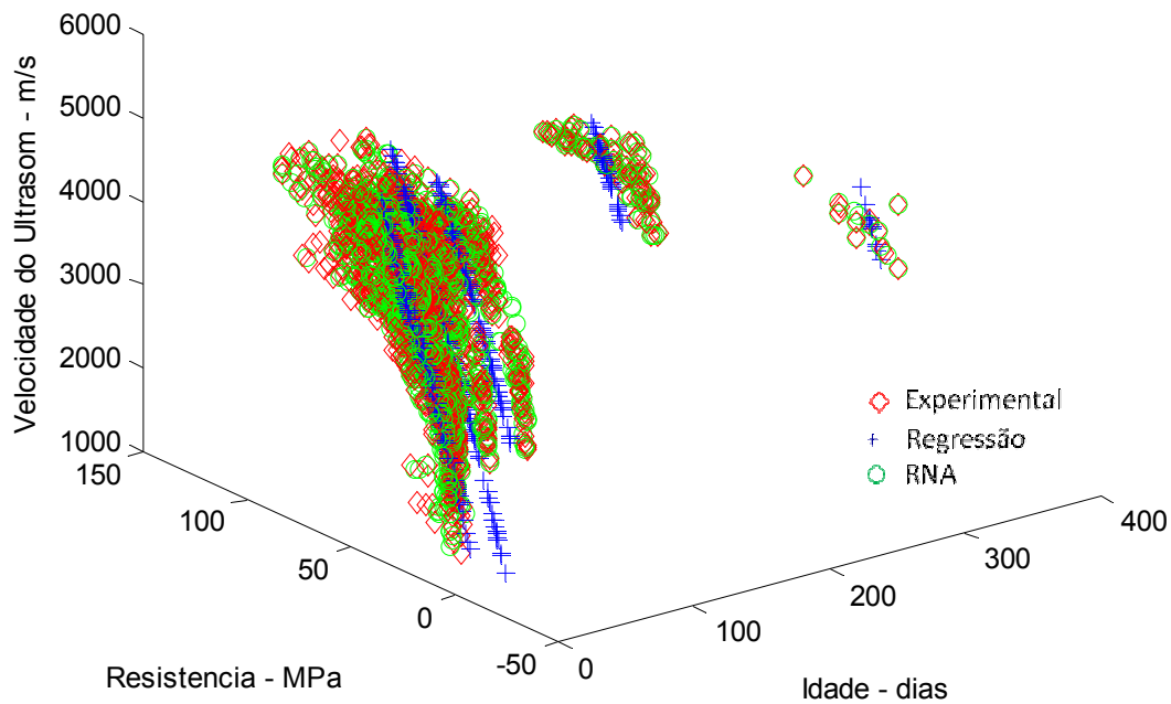
Figura 7.47: Relação VPU x f_c x Idade – rede 7x2x20x20x1 – Dados de Treinamento.
