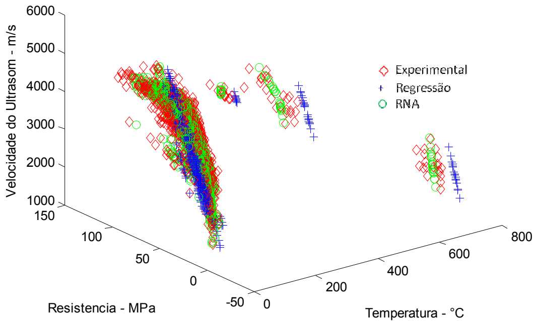
Figura 7.19: Relação VPU x f_c x Temperatura – rede 7x2x4x4x1 – Dados de Treinamento.
