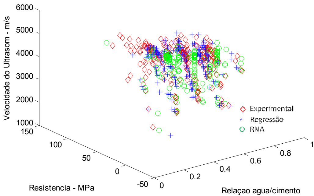
Figura 7.26: Relação VPU x f_c x Relação a/c – rede 7x2x20x4x1 – Dados de Teste
