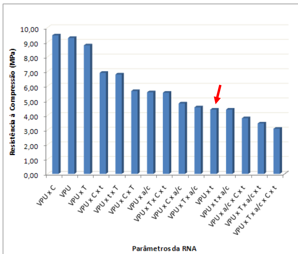
Figura 7.69: Erros médios obtidos considerando diferentes parâmetros de entrada.
