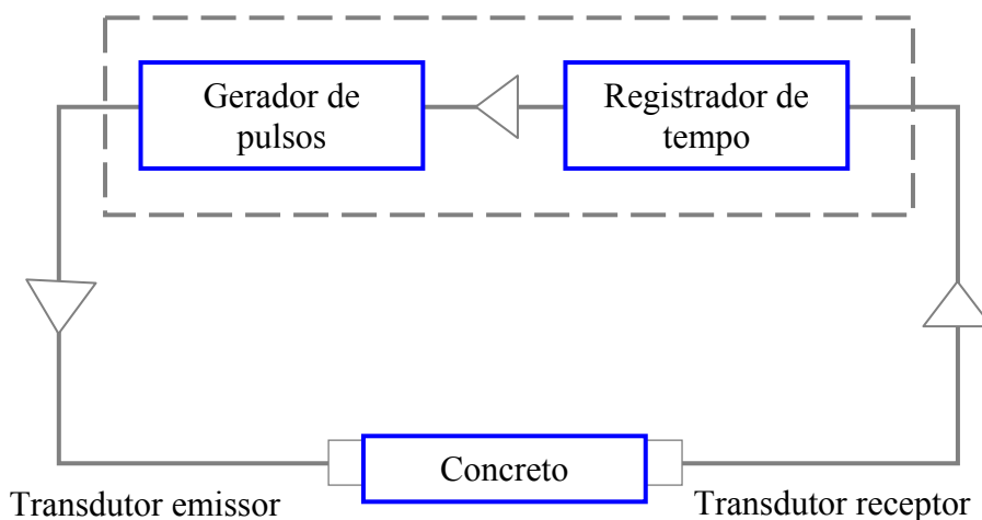
Figura 2.2: princípio de Funcionamento de Ensaio de VPU.
