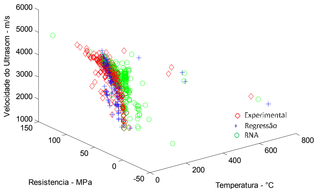
Figura 7.52: Relação VPU x f_c x Temperatura – rede 7x2x20x20x1 – Dados de Teste
