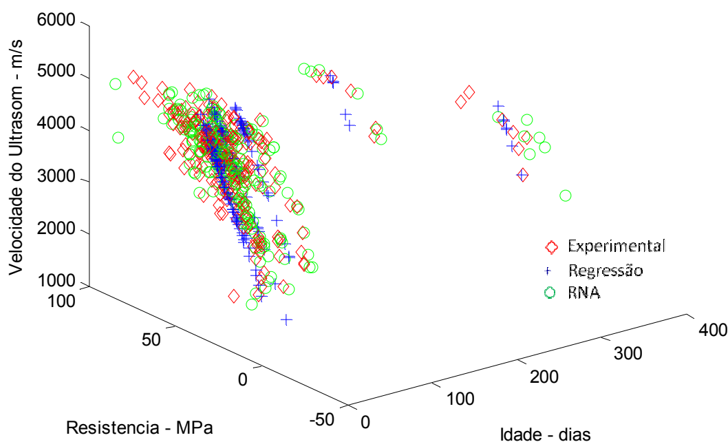
Figura 7.16: Relação VPU x f_c x Idade – rede 7x2x4x4x1 – Dados de Teste
