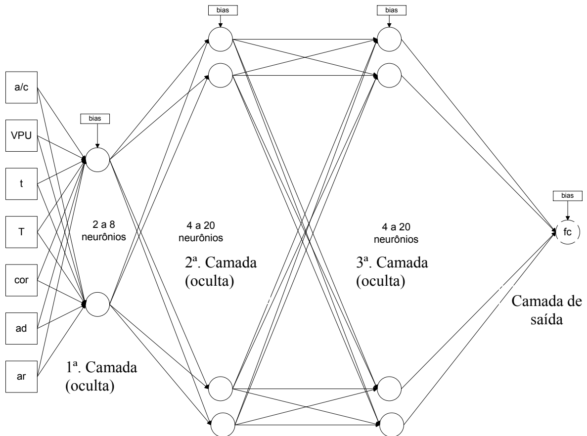
Figura 7.1: Morfologia básica das RNAs testadas.
