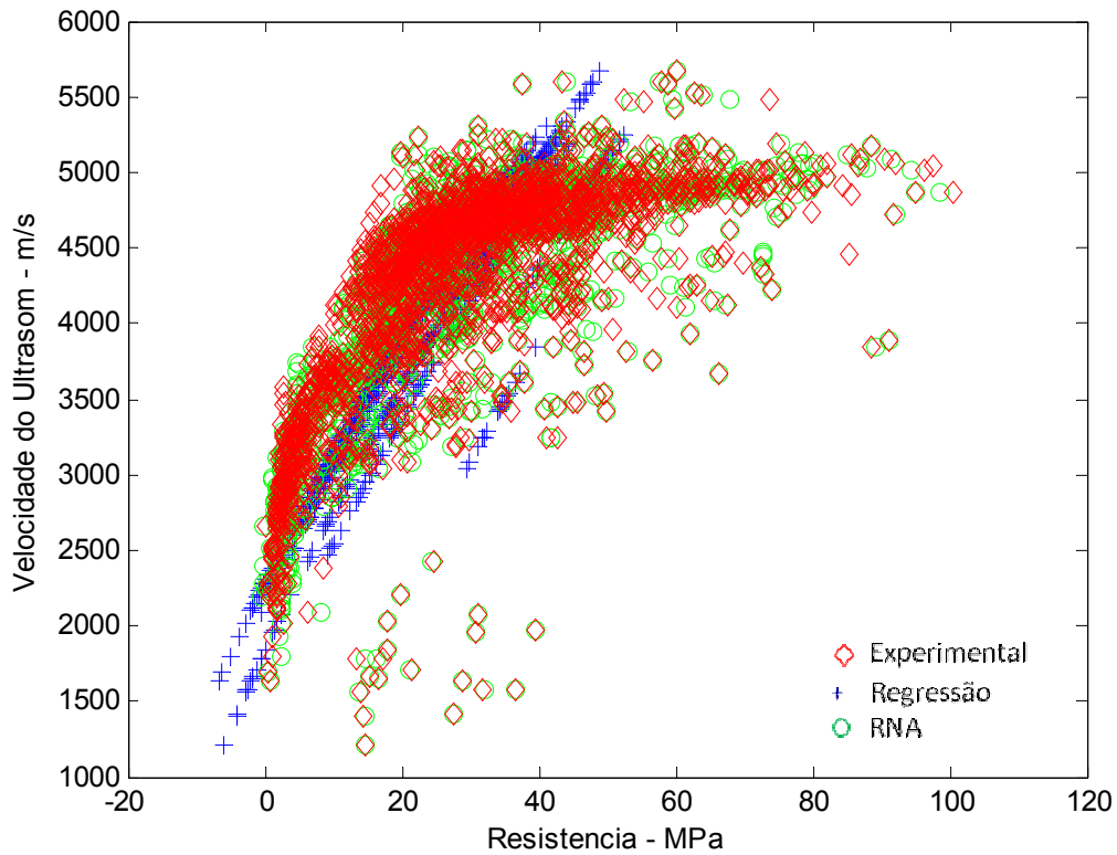
Figura 7.53: Relação VPU x f_c – rede 7x6x20x20x1 – Dados de Treinamento.
