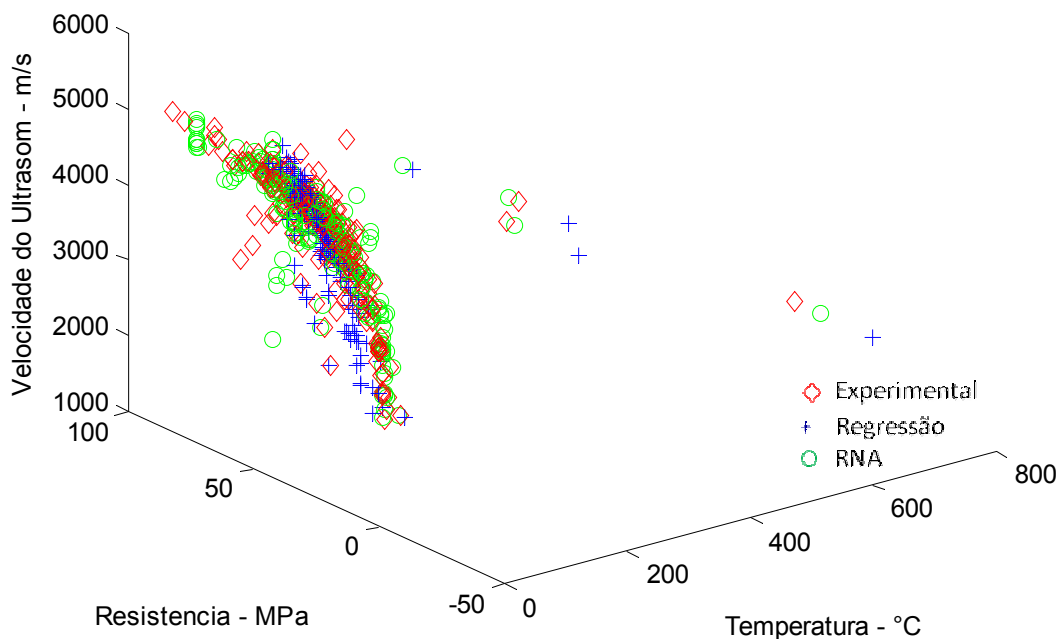
Figura 7.68: Relação VPU x f_c x Temperatura – rede 7x8x20x20x1 – Dados de Teste
