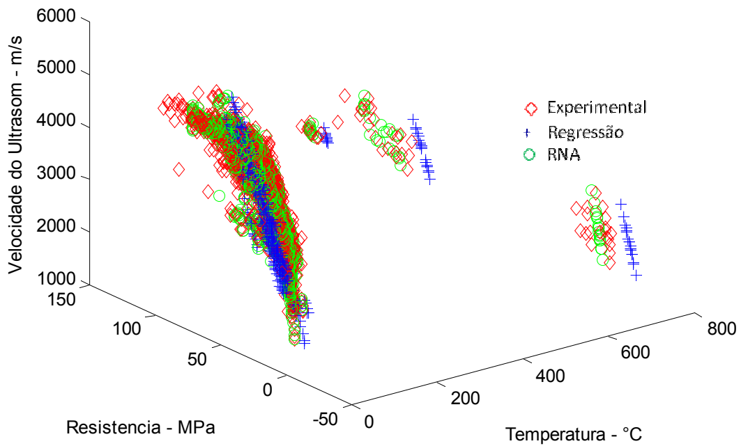
Figura 7.35: Relação VPU x f_c x Temperatura – rede 7x4x20x4x1 – Dados de Treinamento
