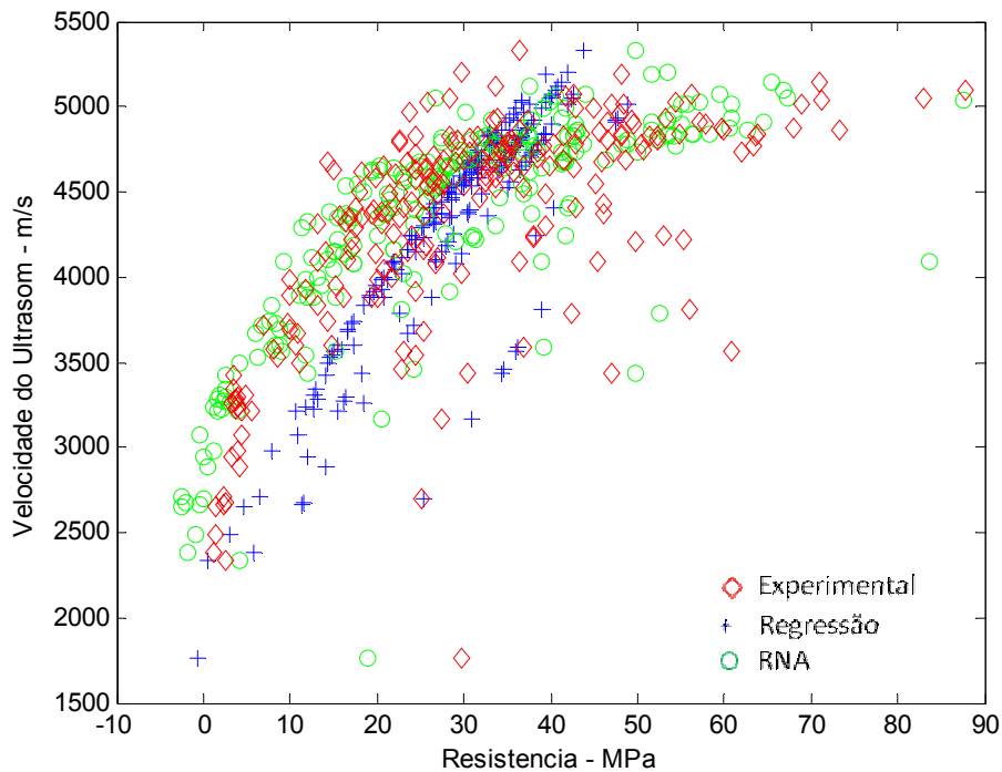
Figura 7.14: Relação VPU x f_c – rede 7x2x4x4x1 – Dados de Teste.
