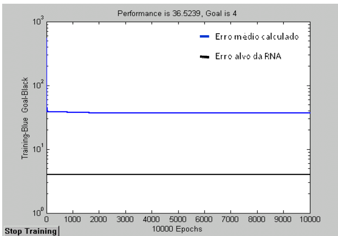
Figura 6.3: treinamento da RNA para 10000 épocas – 2x2x10x1
