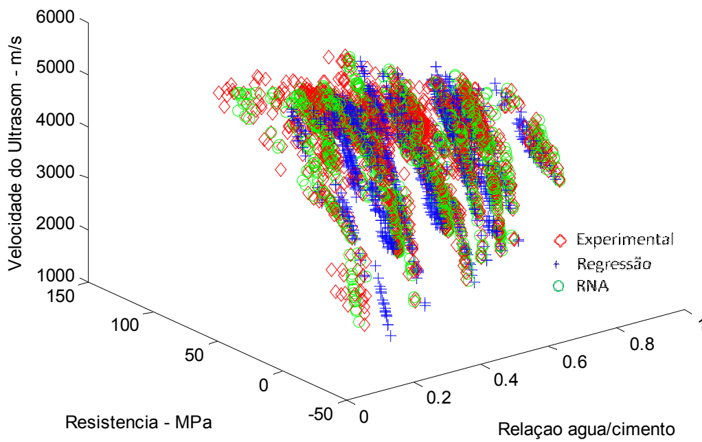
Figura 7.17: Relação VPU x f_c x Idade x relação a/c – rede 7x2x4x4x1 – Dados de Treinamento.
