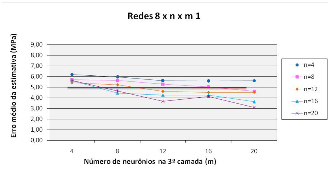
Figura 7.11: Erro médio da estimativa – Redes com 8 neurônios na 1ª camada oculta
