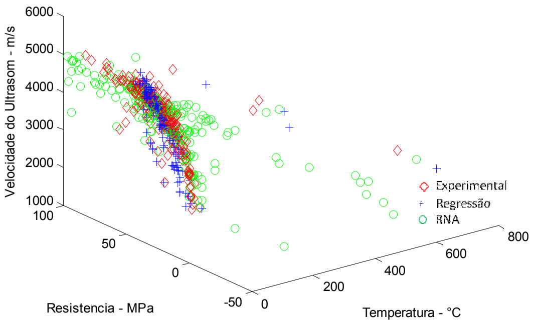
Figura 7.60: Relação VPU x f_c x Temperatura – rede 7x6x20x20x1 – Dados de Teste
