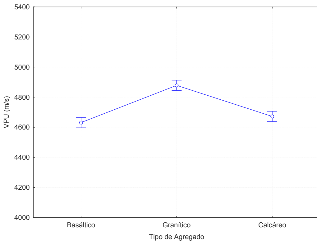
Figura 5.7: influência do tipo de agregado no Ensaio de VPU
