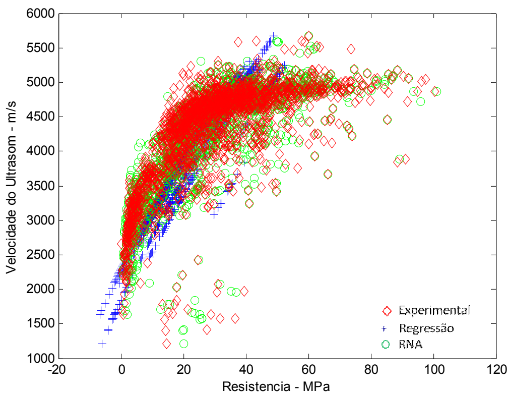
Figura 7.45: Relação VPU x f_c – rede 7x2x20x20x1 – Dados de Treinamento.
