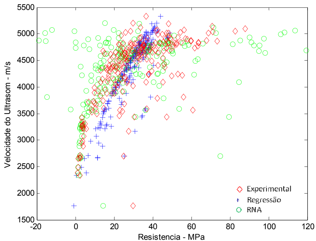
Figura 7.38: Relação VPU x f_c – rede 7x6x20x12x1 – Dados de Teste
