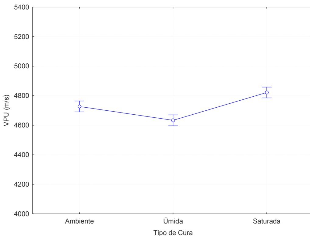
Figura 5.9: influência do tipo de cura no Ensaio de VPU.
