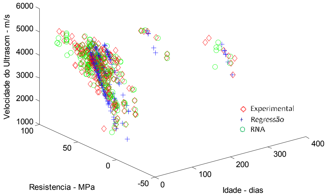
Figura 7.32: Relação VPU x f_c x Idade – rede 7x4x20x4x1 – Dados de Treinamento
