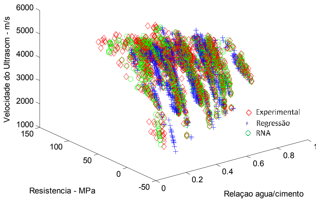
Figura 7.65: Relação VPU x f_c x Relação a/c – rede 7x8x20x20x1 – Dados de Treinamento
