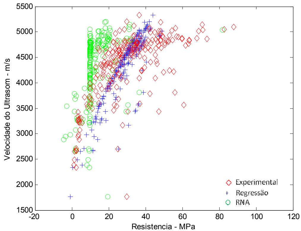
Figura 7.22: Relação VPU x f_c – rede 7x2x20x4x1 – Dados de Teste
