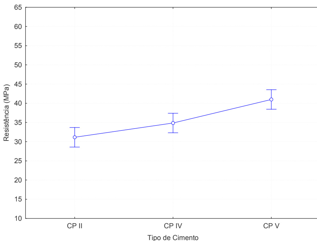
Figura 5.14: influência do tipo de cimento no Ensaio de Resistência Mecânica à Compressão
