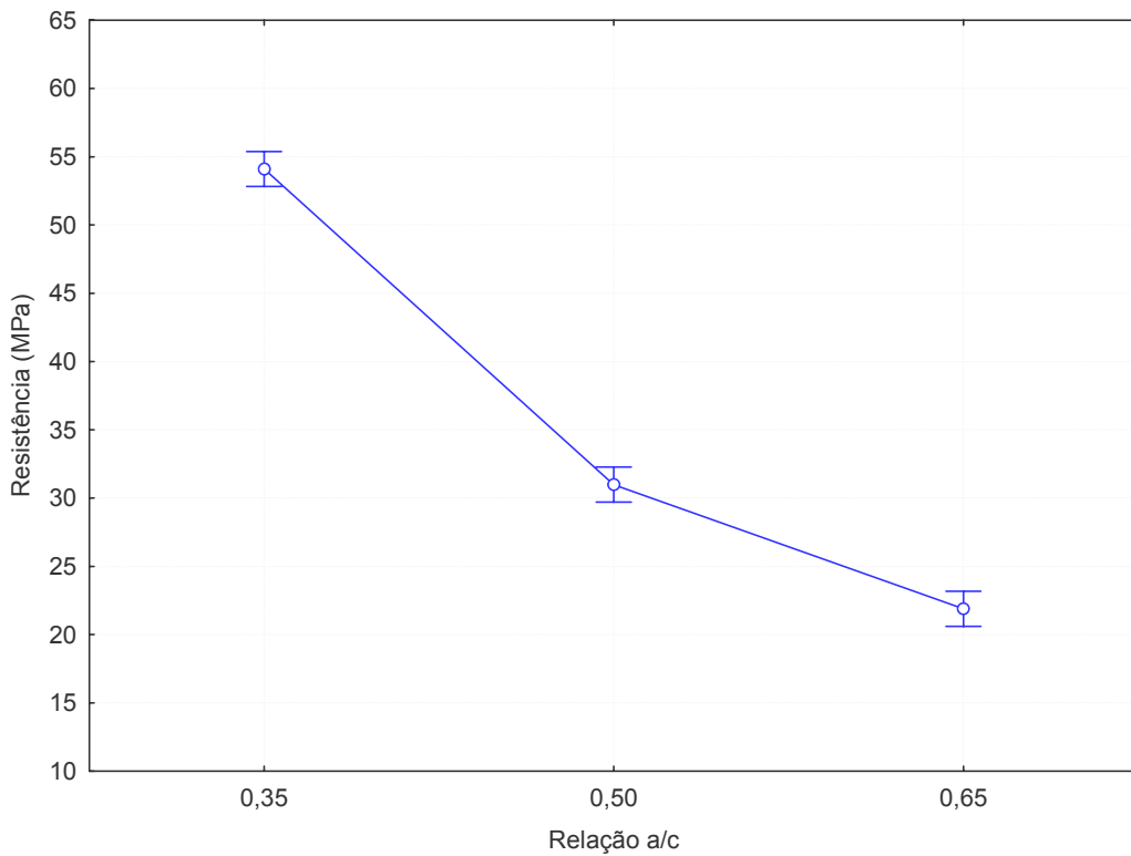
Figura 5.10: influência da relação a/c no Ensaio de Resistência Mecânica à Compressão
