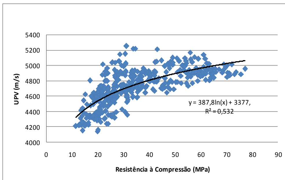
Figura 5.16: relação entre a Resistência Mecânica à Compressão do Concreto e a VPU para os concretos ensaiados
