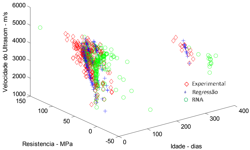
Figura 7.48: Relação VPU x f_c x Idade – rede 7x2x20x20x1 – Dados de Teste
