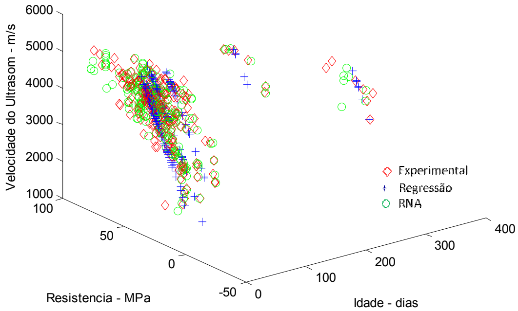
Figura 7.64: Relação VPU x f_c x Idade – rede 7x8x20x20x1 – Dados de Teste
