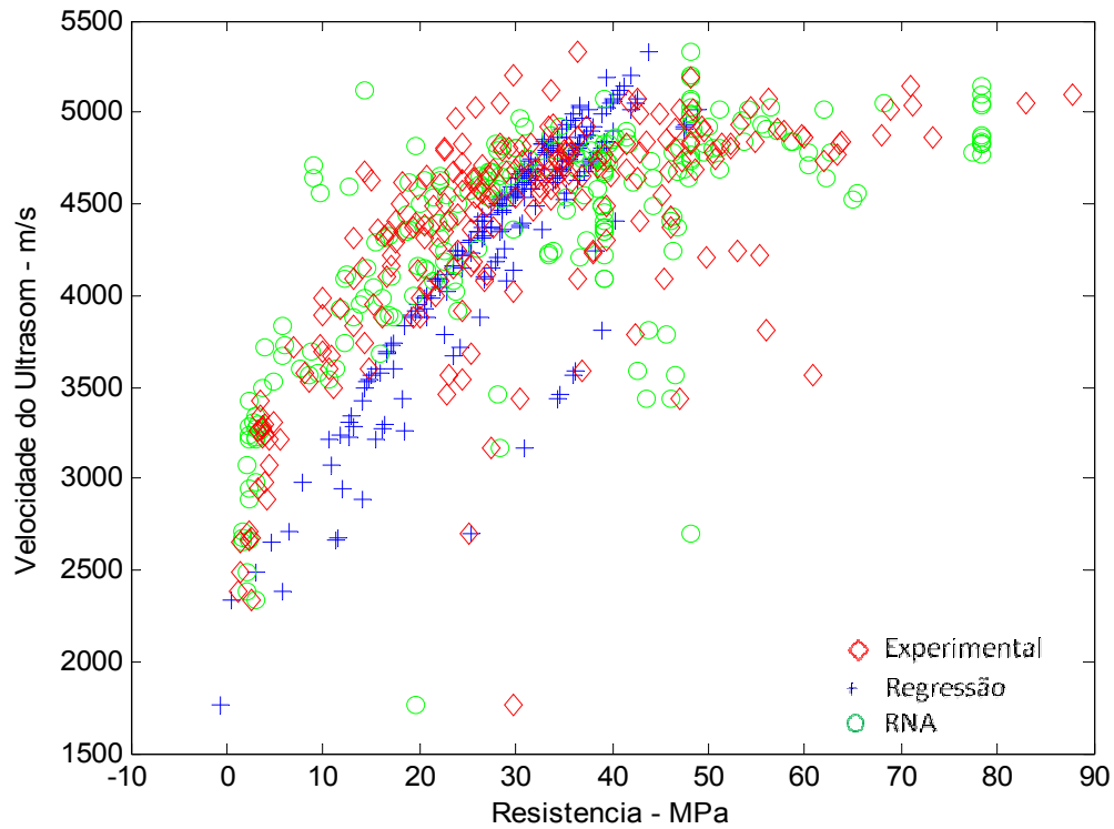
Figura 7.30: Relação VPU x f_c – rede 7x4x20x4x1 – Dados de Teste
