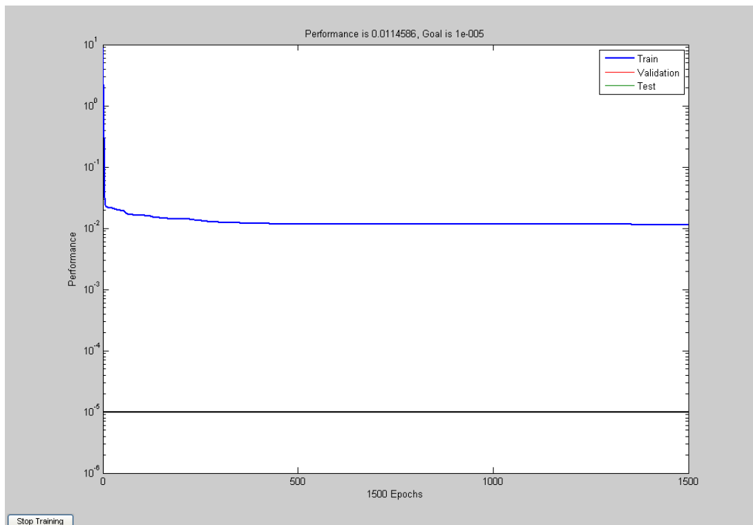
Figura 7.4: evolução do treinamento da RNA para 1500 épocas – Rede 7x4x8x16x1
