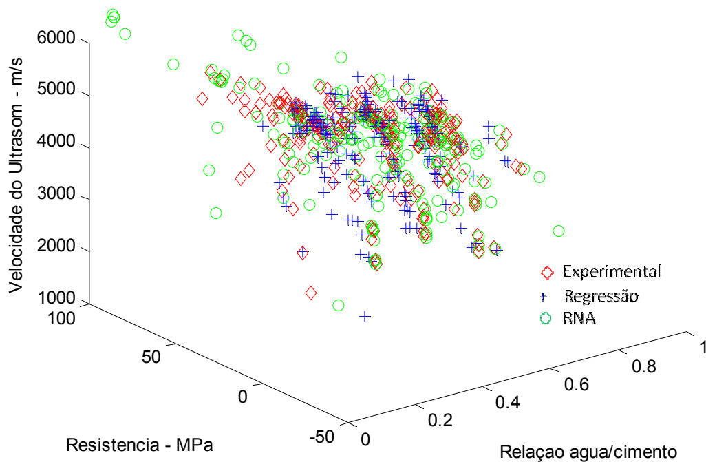
Figura 7.42: Relação VPU x f_c x Relação a/c – rede 7x6x20x12x1 – Dados de Teste
