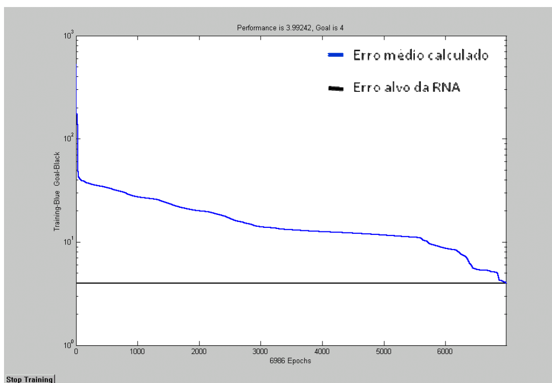
Figura 6.5: treinamento da RNA para 10000 épocas – 2x8x48x1
