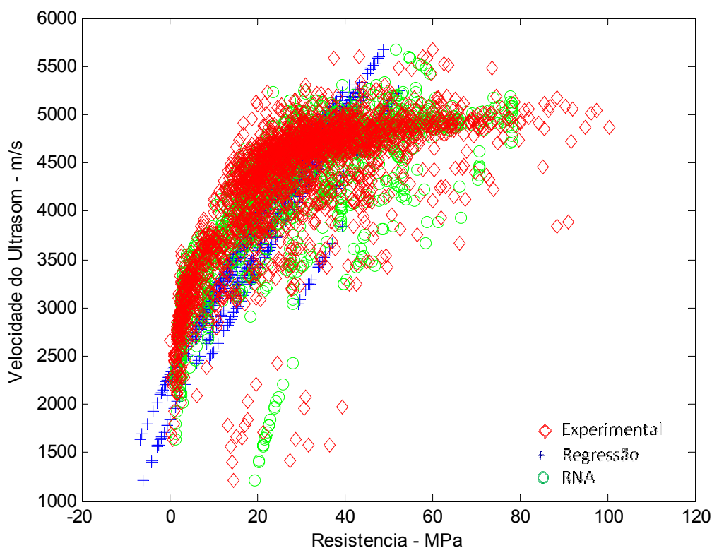
Figura 7.29: Relação VPU x f_c – rede 7x4x20x4x1 – Dados de Treinamento
