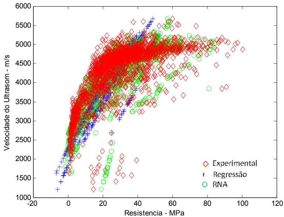
Figura 7.13: Relação VPU x f_c – rede 7x2x4x4x1 – Dados de Treinamento.
