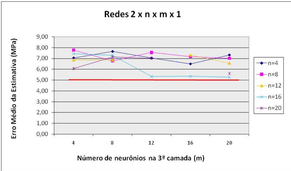
Figura 7.8: Erro médio da estimativa – Redes com 2 neurônios na 1ª camada oculta.
