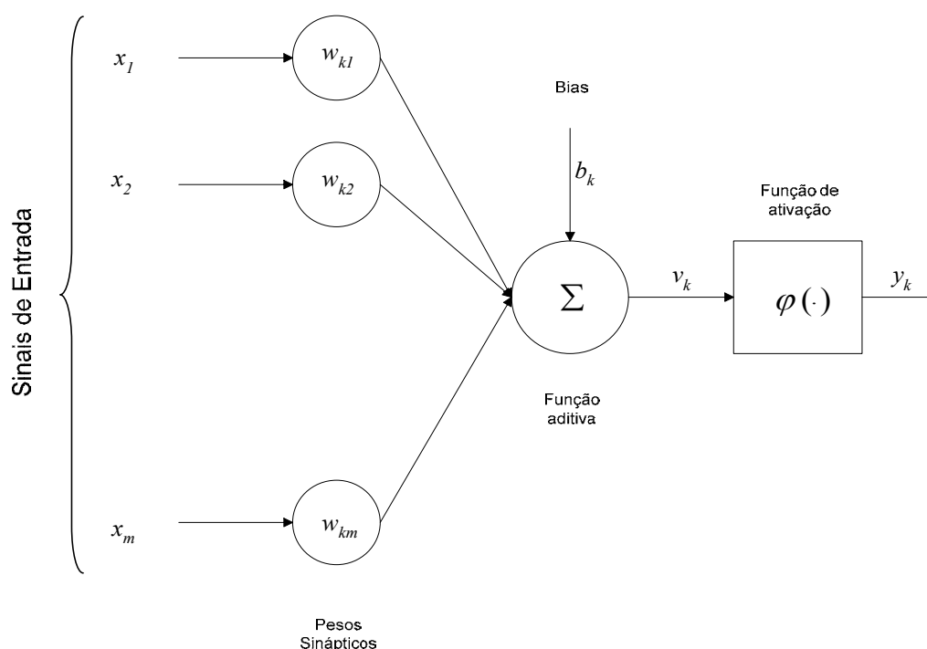
Figura 3.2: modelo não-linear de um neurônio (HAYKIN, 2001).
