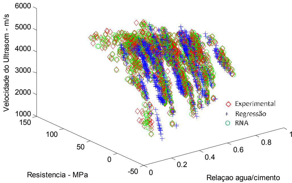
Figura 7.41: Relação VPU x f_c x Relação a/c – rede 7x6x20x12x1 – Dados de Treinamento
