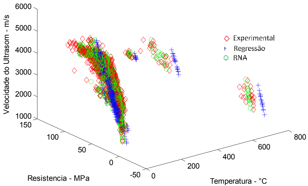
Figura 7.67: Relação VPU x f_c x Temperatura – rede 7x8x20x20x1 – Dados de Treinamento
