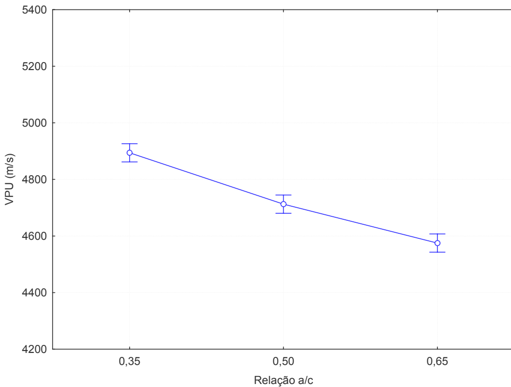
Figura 5.11: influência da relação a/c no Ensaio de VPU.
