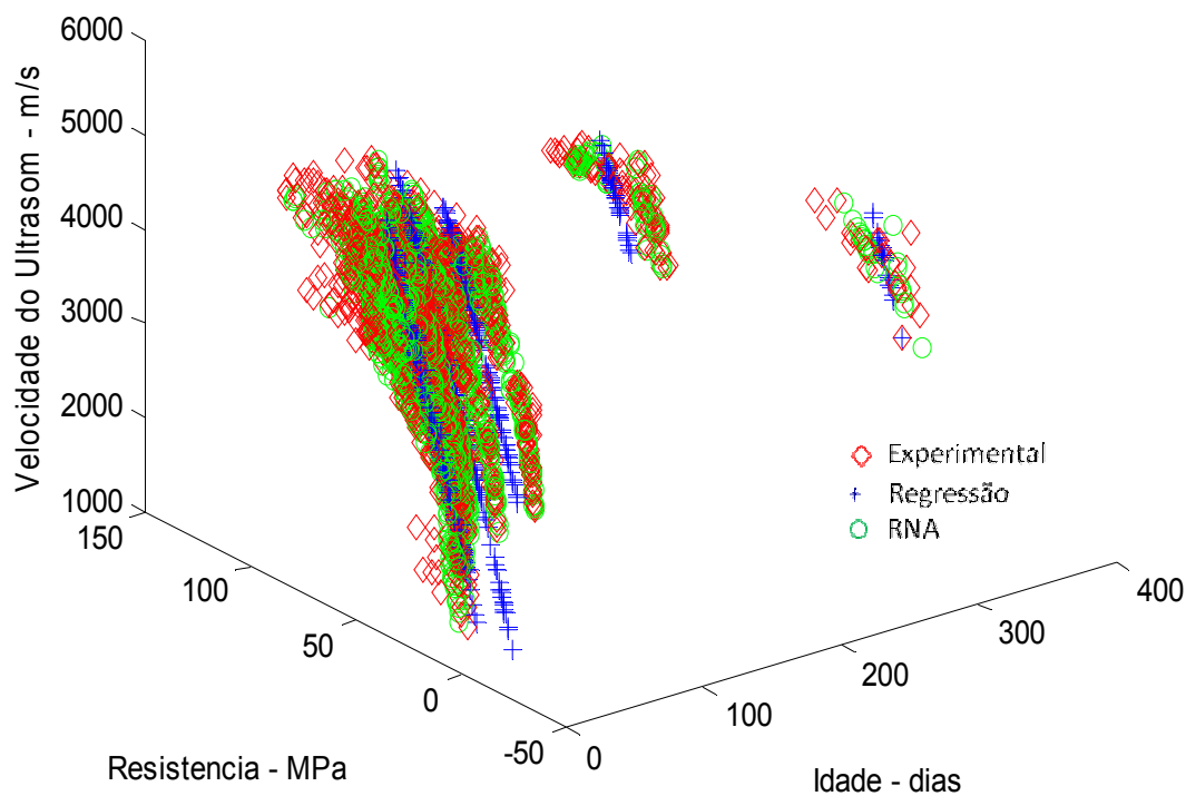
Figura 7.15: Relação VPU x f_c x Idade – rede 7x2x4x4x1 – Dados de Treinamento.
