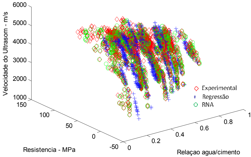
Figura 7.25: Relação VPU x f_c x Relação a/c – rede 7x2x20x4x1 – Dados de Treinamento
