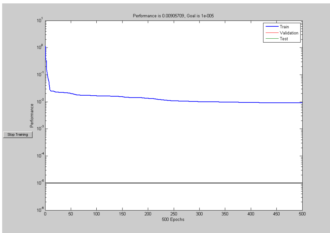
Figura 7.5: evolução do treinamento da RNA para 500 épocas – Rede 7x6x12x20x1
