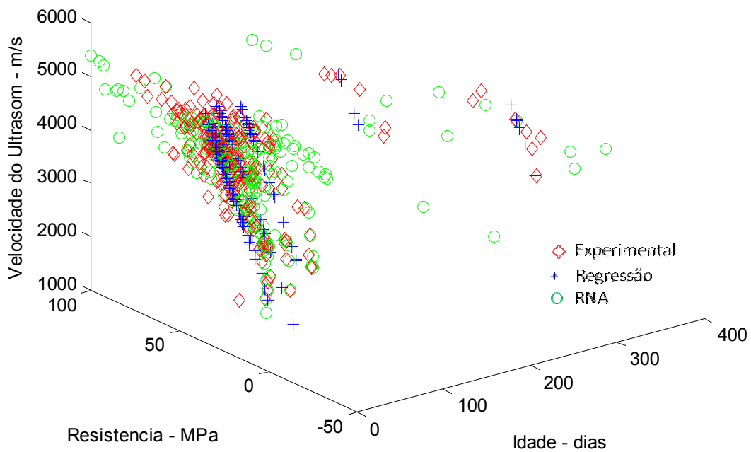
Figura 7.40: Relação VPU x f_c x Idade – rede 7x6x20x12x1 – Dados de Teste
