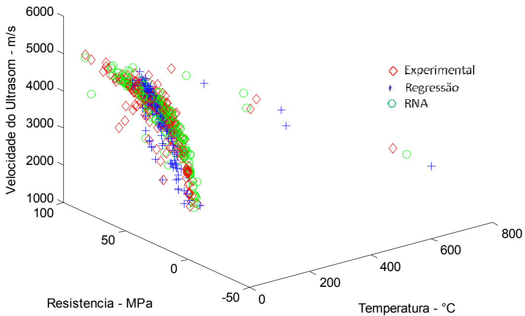
Figura 7.20: Relação VPU x f_c x Temperatura – rede 7x2x4x4x1 – Dados de Teste.
