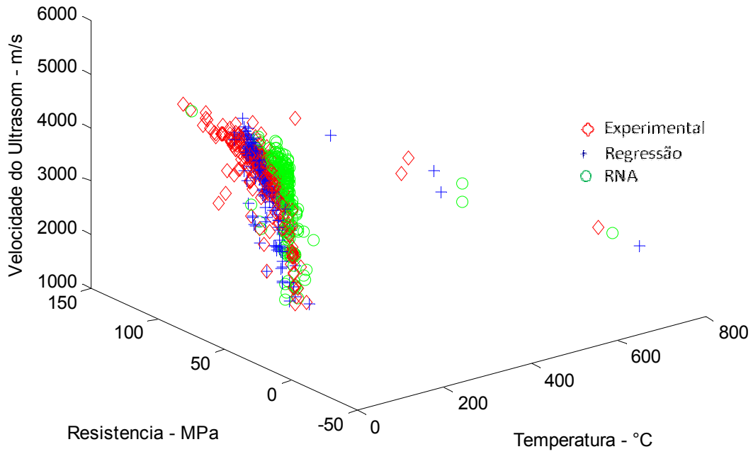
Figura 7.27: Relação VPU x f_c x Temperatura – rede 7x2x20x4x1 – Dados de Treinamento
