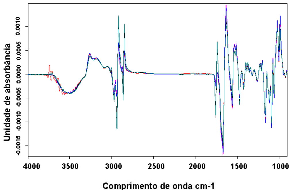
Figura 11 – Médias espectrais sobrepostas em primeira derivada de amostras em triplicata das cepas Candida albicans 22 e Candida glabrata 107. Intervalo de 900-4000 \text{cm}^{-1} .
