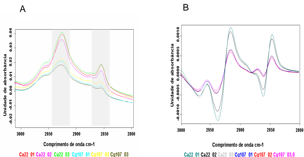
Figura 08 – (A) Espectros sem derivada (B) Espectros em primeira derivada. Espectros representando os picos das médias espectrais FT-IR das cepas C. albicans 22 (Ca 22) e C. glabrata 107 (Cg 107) em triplicata. Cada média espectral correspondente a cepa analisada foi destacada por uma cor. Janela espectral de 2800-3000 \text{cm}^{-1} (intervalo espectral que representa ligações moleculares de lipídios). É possível observar pelas áreas destacadas em cinza as diferenças de intensidade das bandas espectrais.
