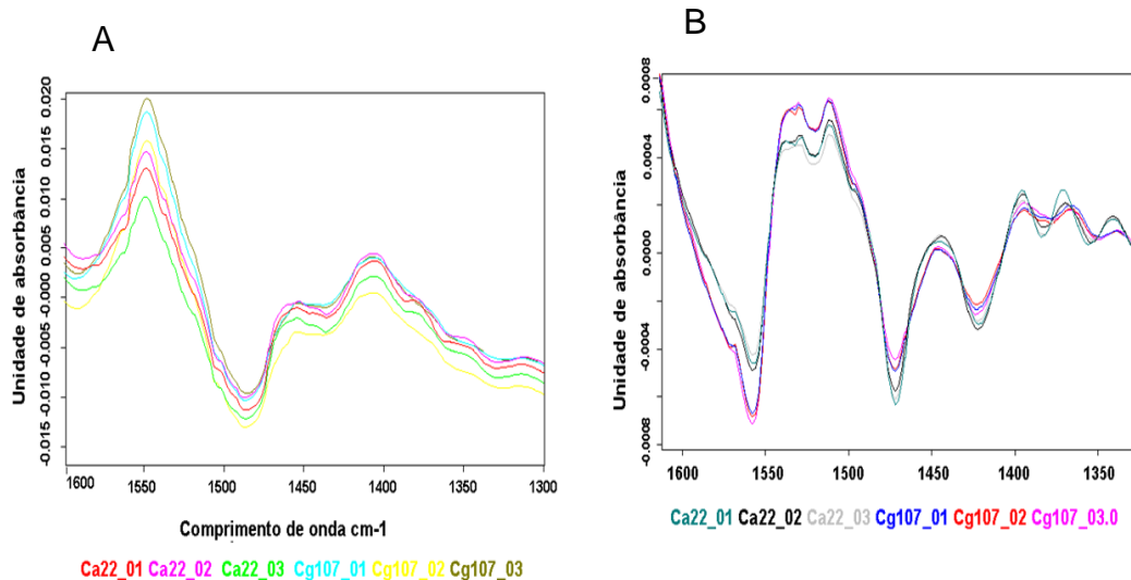
Figura 09 – (A) Espectros sem derivada (B) Espectros em primeira derivada. Espectros representando os picos das médias espectrais FT-IR das cepas C. albicans 22 (Ca 22) e C. glabrata 107 (Cg 107) em triplicata. Cada média correspondente a cepa analisada foi destacada por uma cor. Janela espectral de 1300-1600 \text{cm}^{-1} (intervalo espectral que representa ligações moleculares de proteínas).
