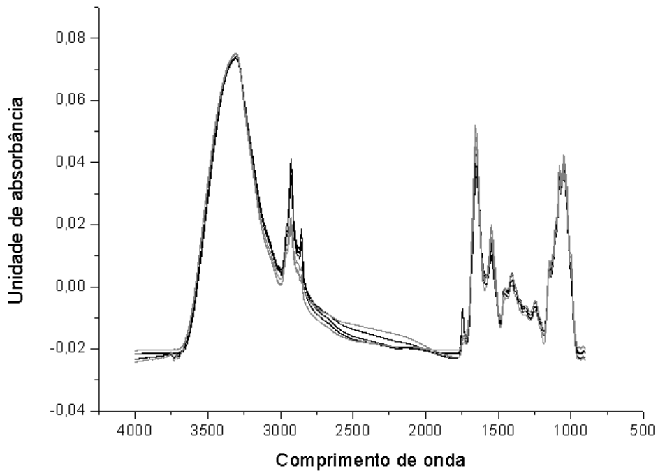
Figura 07 – Médias espectrais FT-IR sobrepostas, das cepas C. albicans 22 e C. glabrata 107 em triplicata submetidas a correção de linha de base e normalização vetorial.
