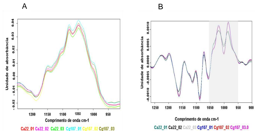
Figura 10 – (A) Espectros sem derivada (B) Espectros em primeira derivada. Médias espectrais FT-IR das cepas C. albicans 22 (Ca 22) e C. glabrata 107 (Cg 107) em triplicata. Cada média espectral correspondente a cepa analisada foi destacada por uma cor. Janela espectral de 900-1250 \text{cm}^{-1} (intervalo espectral que representa ligações moleculares de polissacarídeos).
