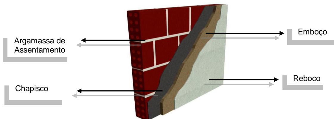
Figura 2.7. Argamassas utilizadas em alvenaria. Fonte Azeredo 1987.
