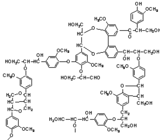
Figura 4 – Estrutura química da lignina Adaptado de LIGNIN INSTITUTE (2001)
