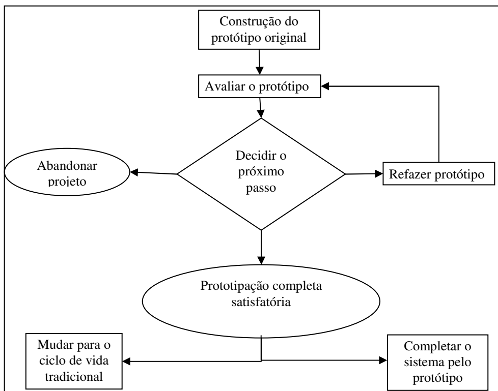
Figura 3 - Construção de protótipos Fonte: adaptado de Alter (2002, p. 438).
