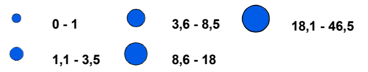
Figura 29 - Mapa de Zonas de Captura e Concentração de Águas Subterrâneas
