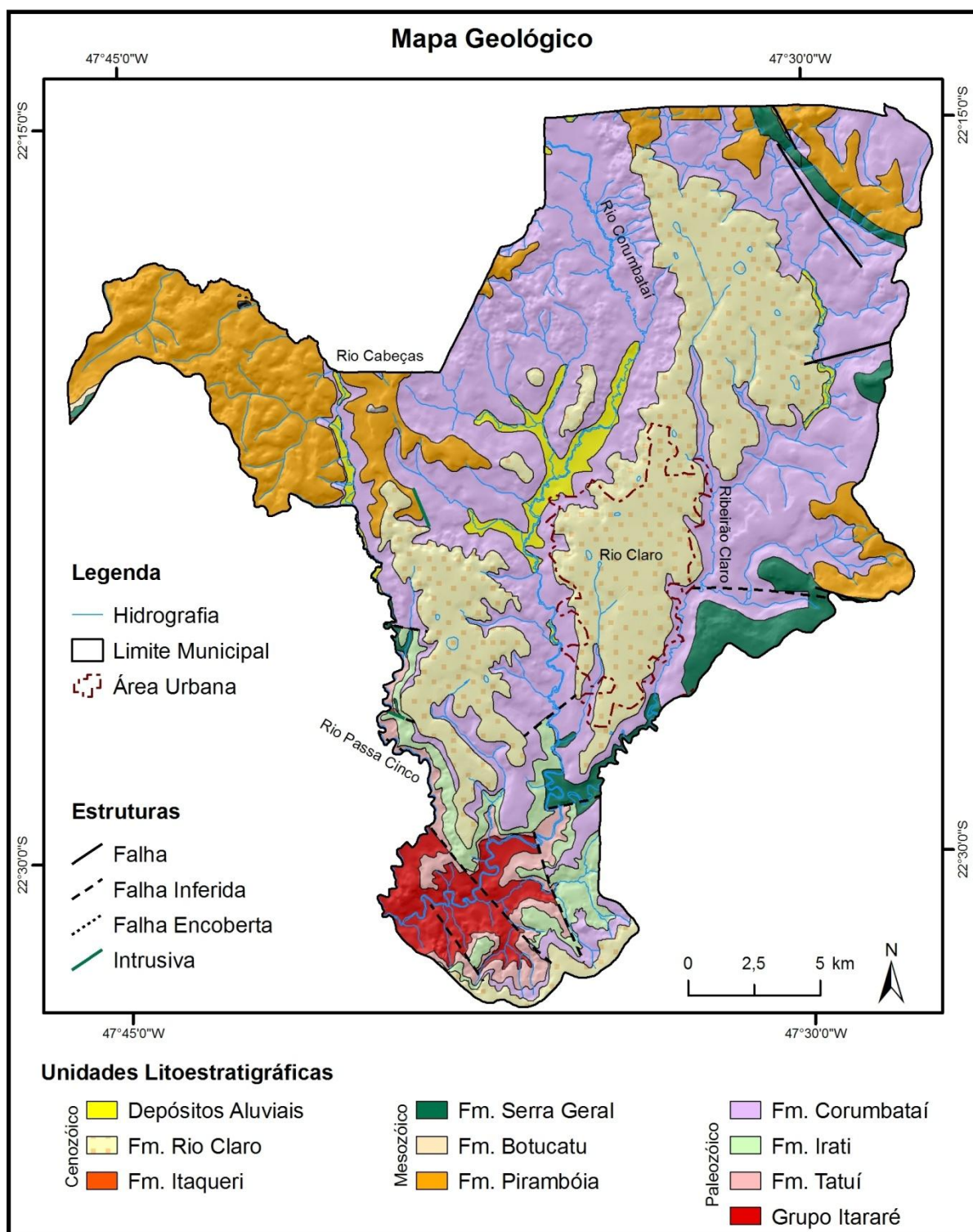
Figura 6: Mapa Geológico do município de Rio Claro (SP) (SOUSA, 2002).
