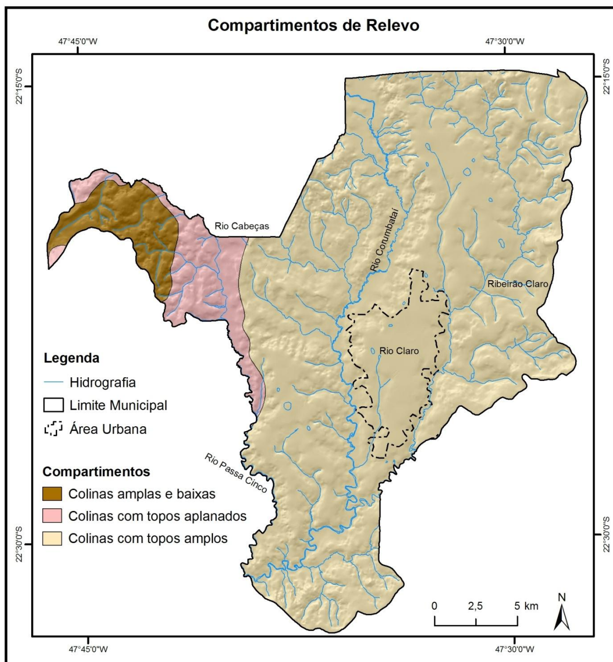
Figura 4: Mapa com os principais tipos de modelados presentes no município de Rio Claro (SP) (ROSS & MOROZ, 1997).
