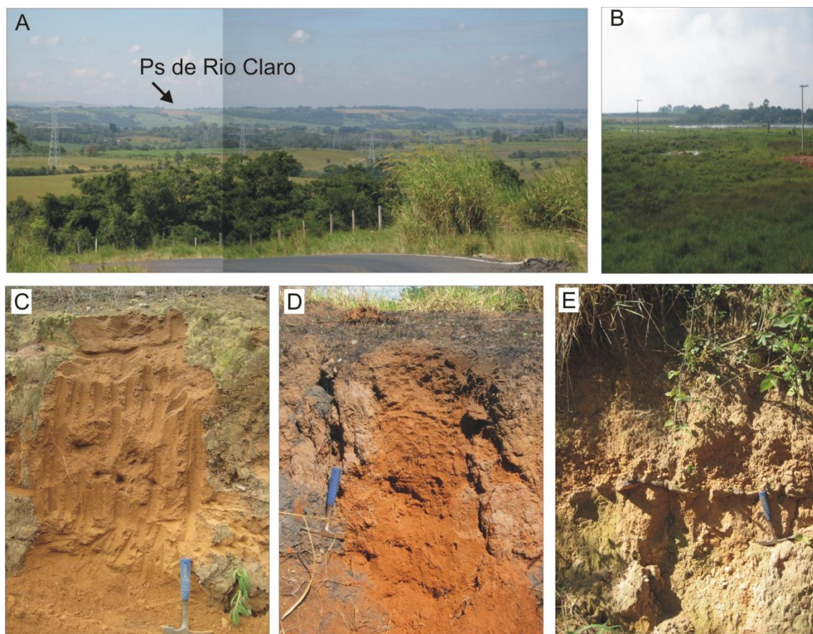
Figura 27: Paisagens representativas da unidade do Planalto Sedimentar. A) topo do Ps de Rio Claro suavemente inclinado no sentido N/S (Ponto 169) ; B) lagoa abandonada típica dos planaltos sedimentares (Ponto 146); C) Cambissolo típico dos topos (Ponto 58); D) Argissolo presentes nas encostas (Ponto 138); E) depósito colúvio-aluvial de encosta (Ponto 17).
