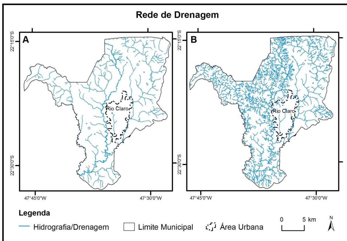
Figura 12: Rede de drenagem da área. A) folhas topográficas 1:50.000 e B) fotografias aéreas 1:25.000.
