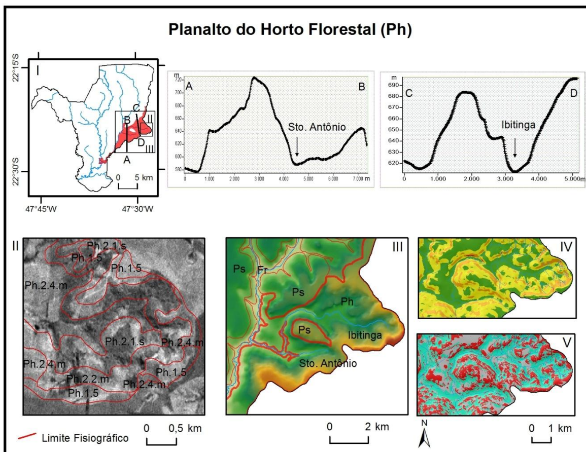
Figura 35: Representação esquemática da unidade do Planalto do Horto Floresta. I) localização e distribuição da unidade; II) relevo típico da unidade Ph e subpaisagens; III) níveis altimétricos da unidade Ph; IV) declividade; V) curvatura terreno; A-B e C-D) perfis transversais representativos da paisagem.
