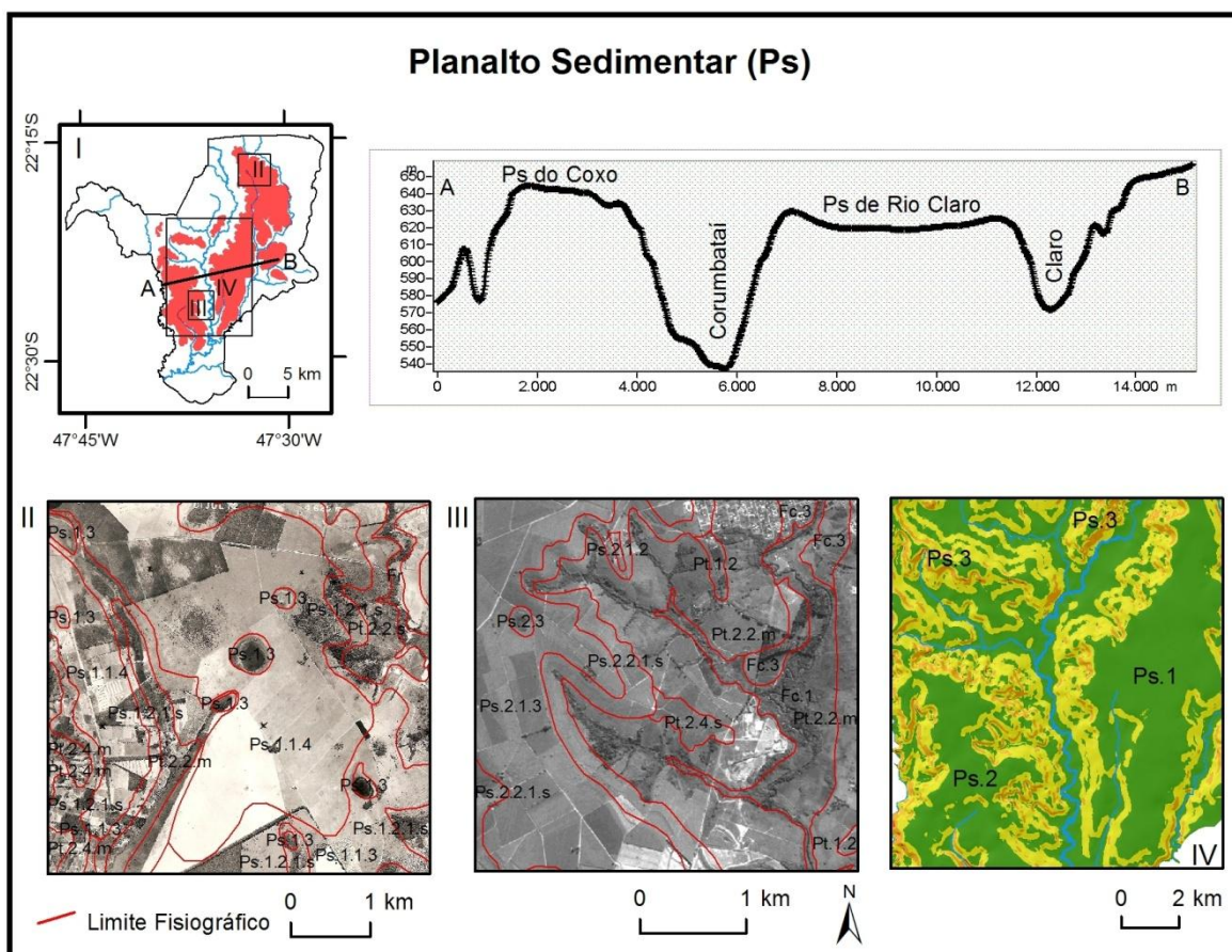
Figura 26: Representação esquemática da unidade dos Planaltos Sedimentares. I) localização e distribuição da unidade; II) trecho do Ps de Rio Claro que representa as subpaisagens de topo, lagoa abandonada e encosta; III) trecho do Ps do Campo do Coxo representando a relação de contato entre o Planalto Sedimentar e os Planaltos/Terraços Dissecados; IV) representação do relevo plano que predomina nos topos e relevo suave ondulado das encostas; A-B) perfil transversal representativo da paisagem.
