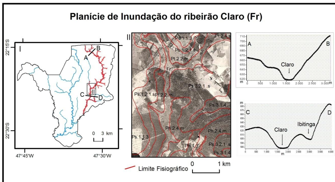
Figura 24: Representação esquemática da unidade Planície de Inundação do ribeirão Claro. I) localização e distribuição da unidade; II) trecho da planície do ribeirão Claro próxima ao horto florestal; A-B, C-D) perfis transversais representativos da paisagem.
