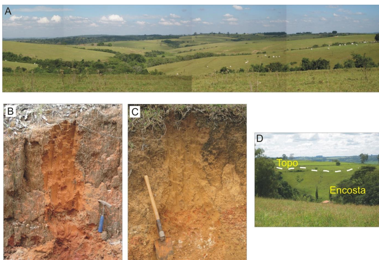
Figura 31: Paisagens representativas da unidade do Planalto de Itapé. A) vista geral da unidade Pi (Ponto 178); B) depósito colúvio-aluvial de topo, com cascalheira basal (Ponto 123); C) depósito colúvio-aluvial em discordância com plintito da Fm. Pirambóia (Ponto 116); D) exemplo de ruptura de relevo negativa entre topo com depósito colúvio-aluvial e encosta sobre Plintossolo da Fm. Pirambóia (Ponto 142).
