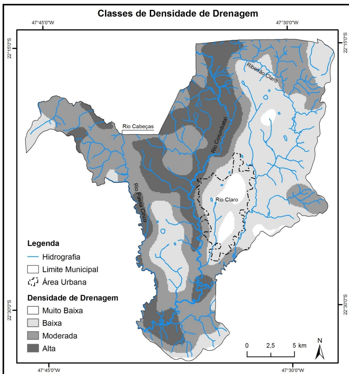
Figura 13: Mapa de densidade de drenagem do município de Rio Claro – SP.
