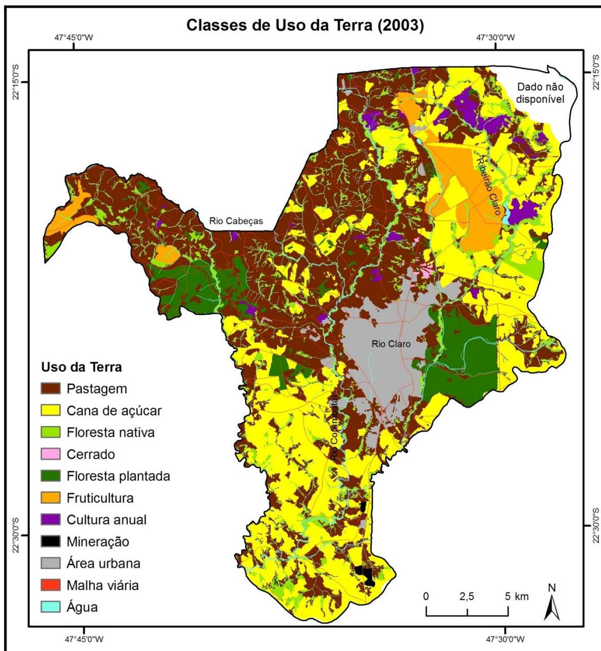
Figura 84: Classes de uso da terra do município de Rio Claro-SP, ano de 2003 (CEAPLA, 2010).
