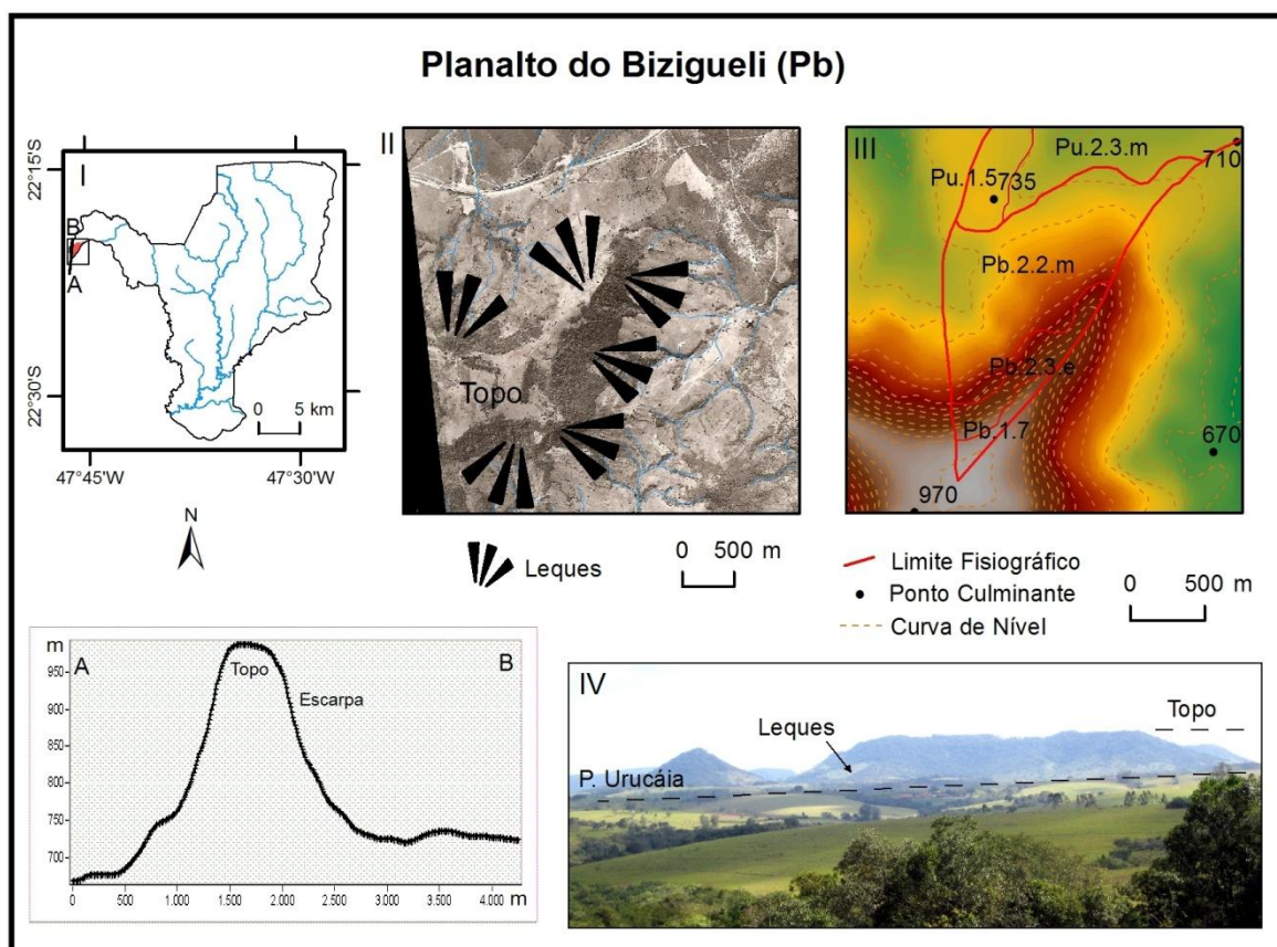
Figura 34: Representação esquemática da unidade do Planalto do Bizigueli. I) localização e distribuição da unidade; II) visualização das subpaisagens em fotografias aéreas; III) níveis altimétricos da unidade Pb; IV) elementos que compõem a paisagem do Pb e sua relação com o Pu (Ponto 175, rumo 230°); A-B) perfil transversal representativo da paisagem.
