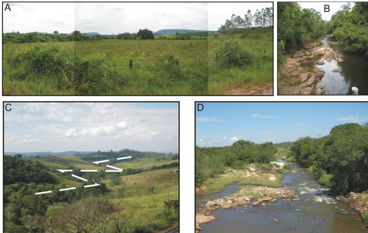
Figura 23: Paisagens representativas da unidade da Planície de Inundação dos rios Passa Cinco/Cabeças. A) planície de inundação do rio Cabeças (Ponto 135); B) leito rochoso (Diabásio) do rio Passa Cinco (Ponto 195); C) controle estrutural no rio Cabeças (Ponto 182); D) leito rochoso (Fm. Pirambóia) e estreita planície de inundação do rio Cabeças (Ponto 173).
