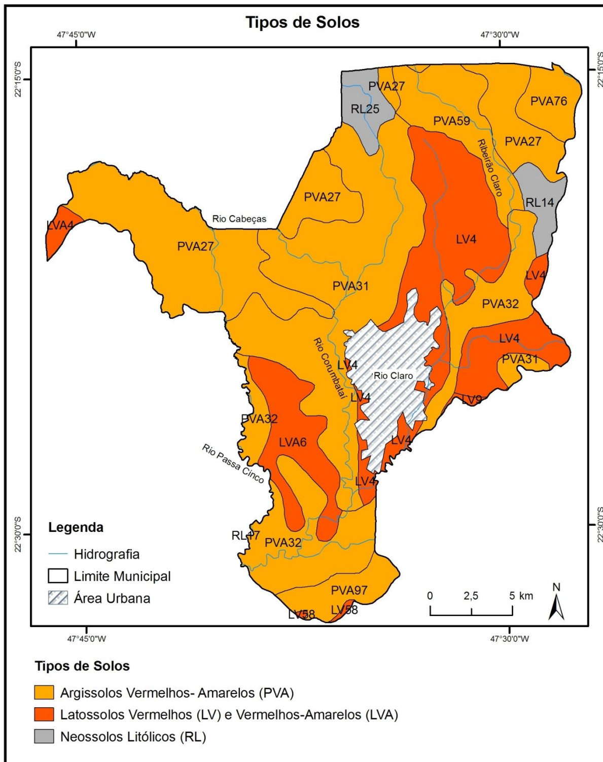
Figura 5: Tipos de solos do município de Rio Claro-SP (OLIVEIRA, 1999).
