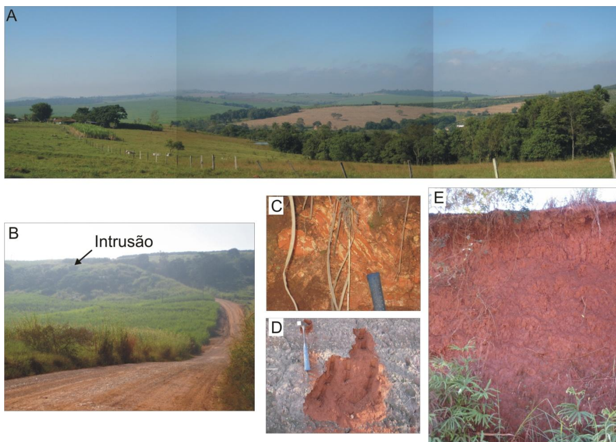
Figura 38: Paisagens representativas da unidade do Planalto da Mata Negra. A) vista geral da unidade Pm (Ponto 150); B) controle estrutural por intrusão de Diabásio (Ponto 148); C) Fm. Corumbataí com pequenas dobras e alterada (Ponto 22); D) material de topo, concrecionário e muito friável (Ponto 23); E) Argissolo com substrato da Fm. Corumbataí (Ponto 22).
