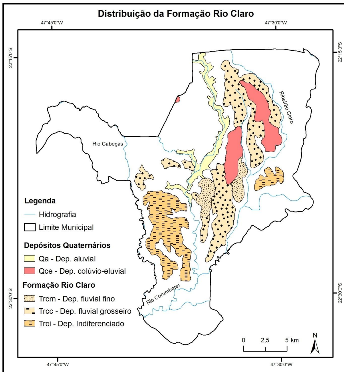
Figura 8: Distribuição dos depósitos da Fm. Rio Claro e depósitos quaternários no município de Rio Claro-SP (MELO, 1995).
