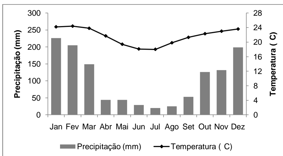
Figura 6: Climograma do município de Rio Claro-SP com a distribuição das chuvas e temperaturas médias. Fonte DAEE-ESALQ, período de 1941 a 1977 ( http://ce.esalq.usp.br/bhbrasil/Saopaulo/ ).
