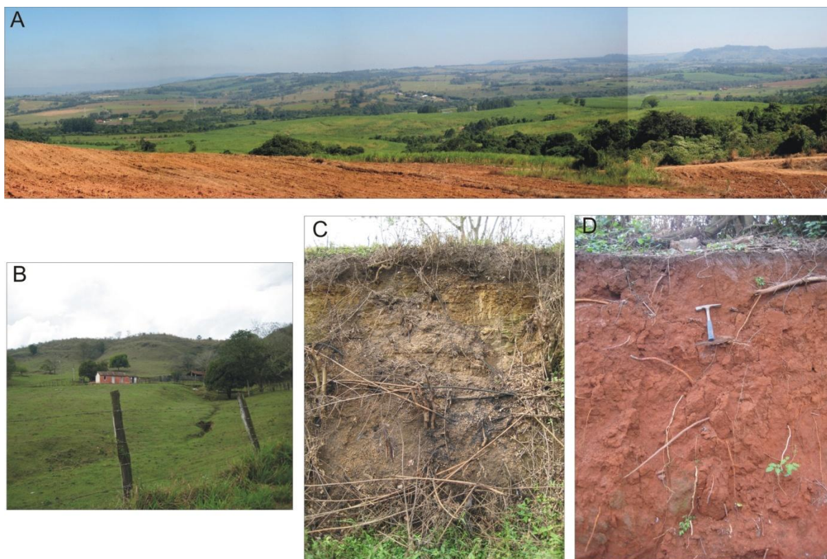
Figura 29: Paisagens representativas da unidade do Planaltos/Terraços dissecados. A) vista geral da unidade Pt (Ponto 162) ; B) processos erosivos sobre depósitos de encosta (Ponto 63); C) Neossolo Litólico da Fm. Corumbataí (Ponto 61); D) Argissolo próximo ao distrito de Ferraz (Ponto 72).
