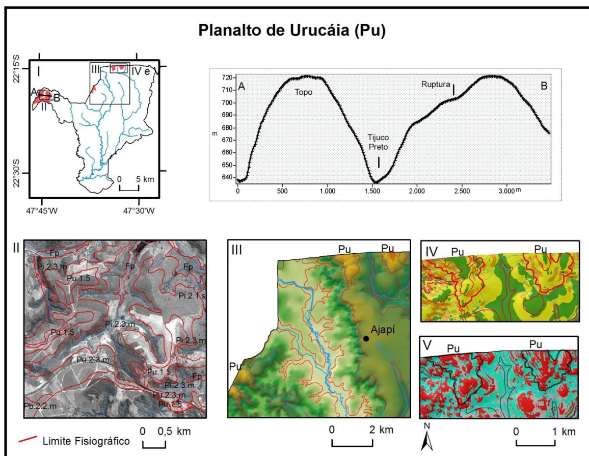
Figura 3932: Representação esquemática da unidade do Planalto de Urucáia. I) localização e distribuição da unidade; II) relevo típico da unidade Pu e subpaisagens; III) níveis altimétricos da unidade Pu na porção nordeste da área ; IV) declividade; V) curvatura terreno; A-B) perfil transversal representativo da paisagem.
