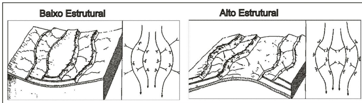
Figura 3: Modelo de altos e baixos estruturais, modificado de Soares et al. (1981).
