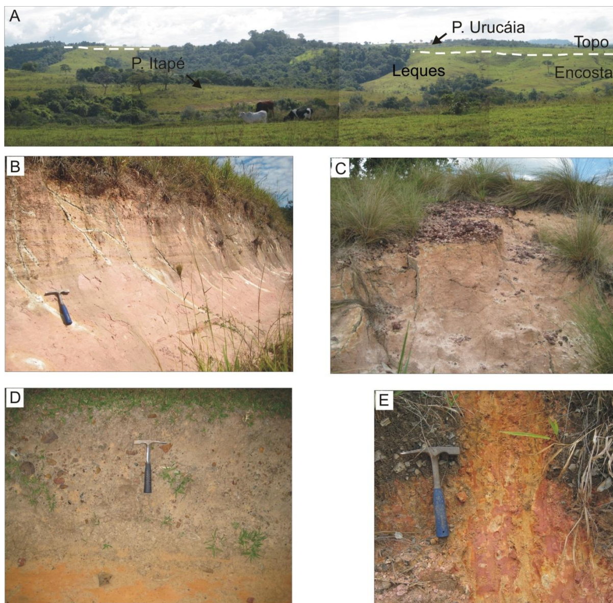
Figura 33: Paisagens representativas da unidade do Planalto de Urucáia. A) vista geral da unidade Pu em contato com a unidade Pi (Ponto 179); B) Plintossolo da Fm. Pirambóia (Ponto 181); C) lateritas espessas sobre Plintossolo da Fm. Pirambóia (Ponto 143) ; D) depósito colúvio-aluvial grosseiro (Ponto 117); E) Fm. Pirambóia fortemente alterada (Plintossolo) (Ponto115).
