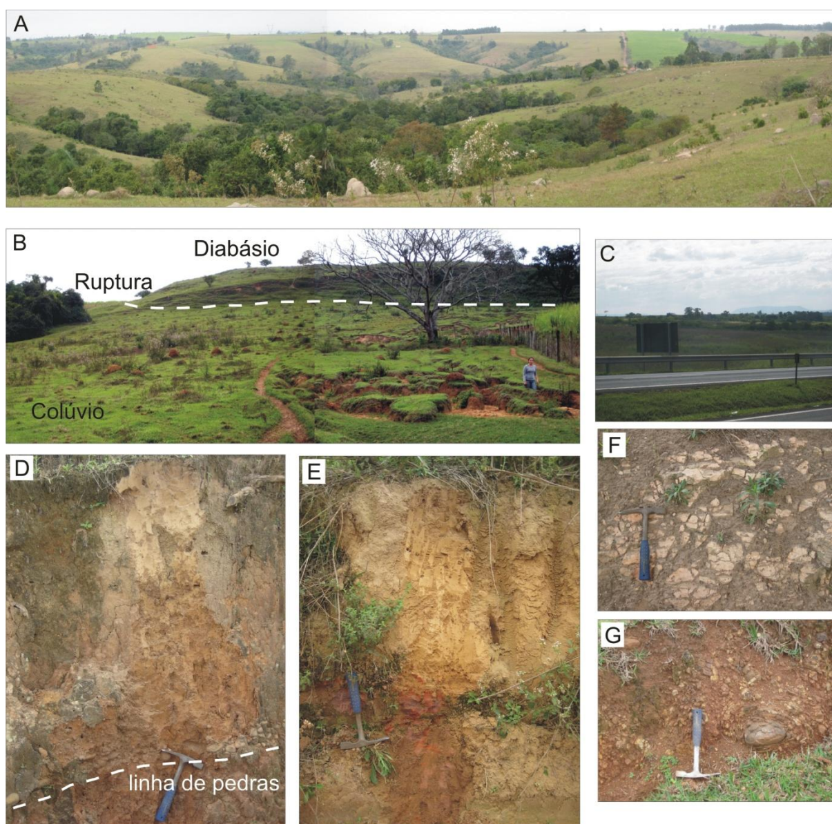
Figura 40: Paisagens representativas da unidade do Domo de Pitanga. A) vista geral da unidade do Domo de Pitanga (Ponto 48); B) controle estrutural evidente por intrusões de Diabásio e rupturas de relevo abruptas (Ponto 37); C) planície de inundação situada na meia encosta, evidência de soerguimento (Ponto 187); D) depósito colúvio-aluvial com base cascalhenta (Ponto 36); E) depósito colúvio-aluvial sobre Plintossolo do grupo Itararé (Ponto 46); F). siltito do grupo Itararé (Ponto 34); G) alteração esferoidal de Diabásio (Ponto 41).
