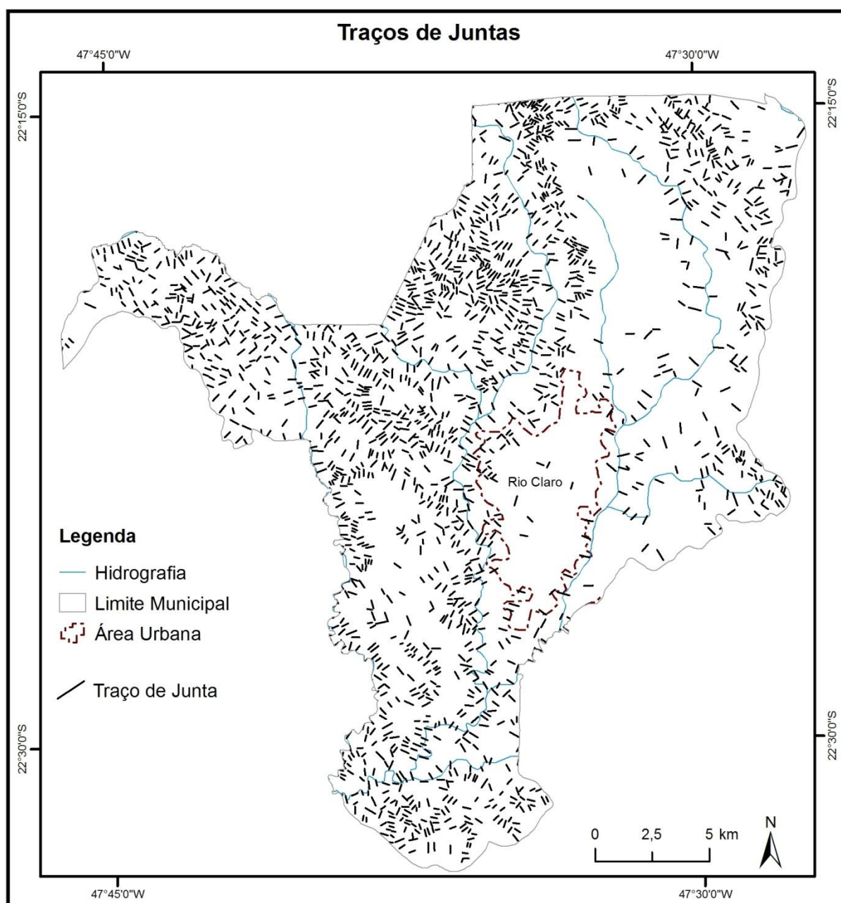
Figura 16: Mapa de traços de juntas do município de Rio Claro - SP.
