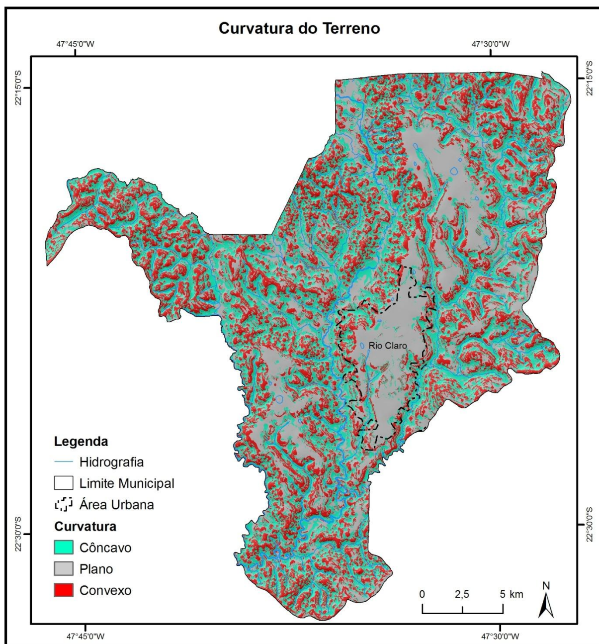
Figura 11: Classes de curvatura do terreno do município de Rio Claro - SP.
