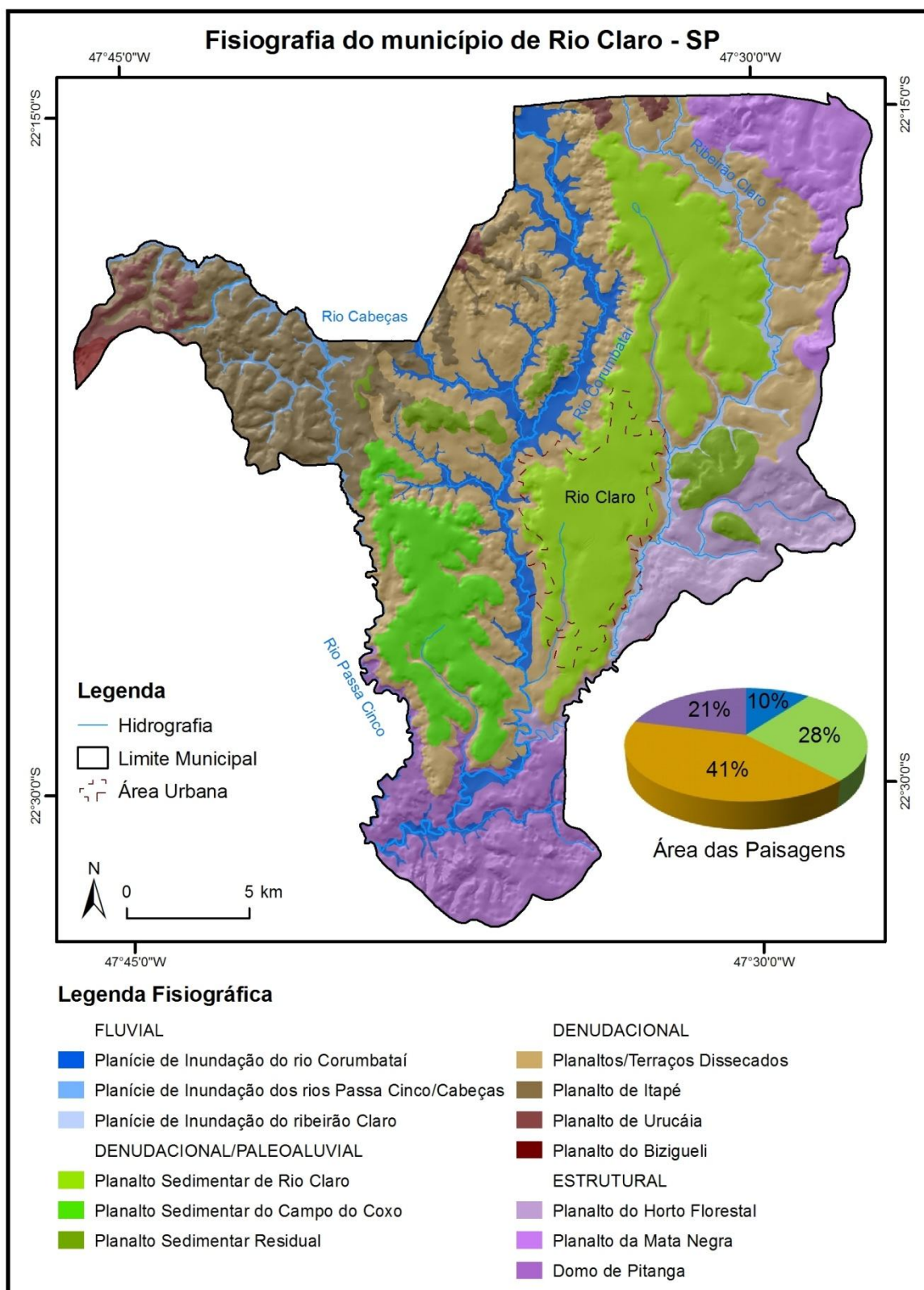
Figura 20: Representação das Paisagens Fisiográficas do município de Rio Claro-SP.
