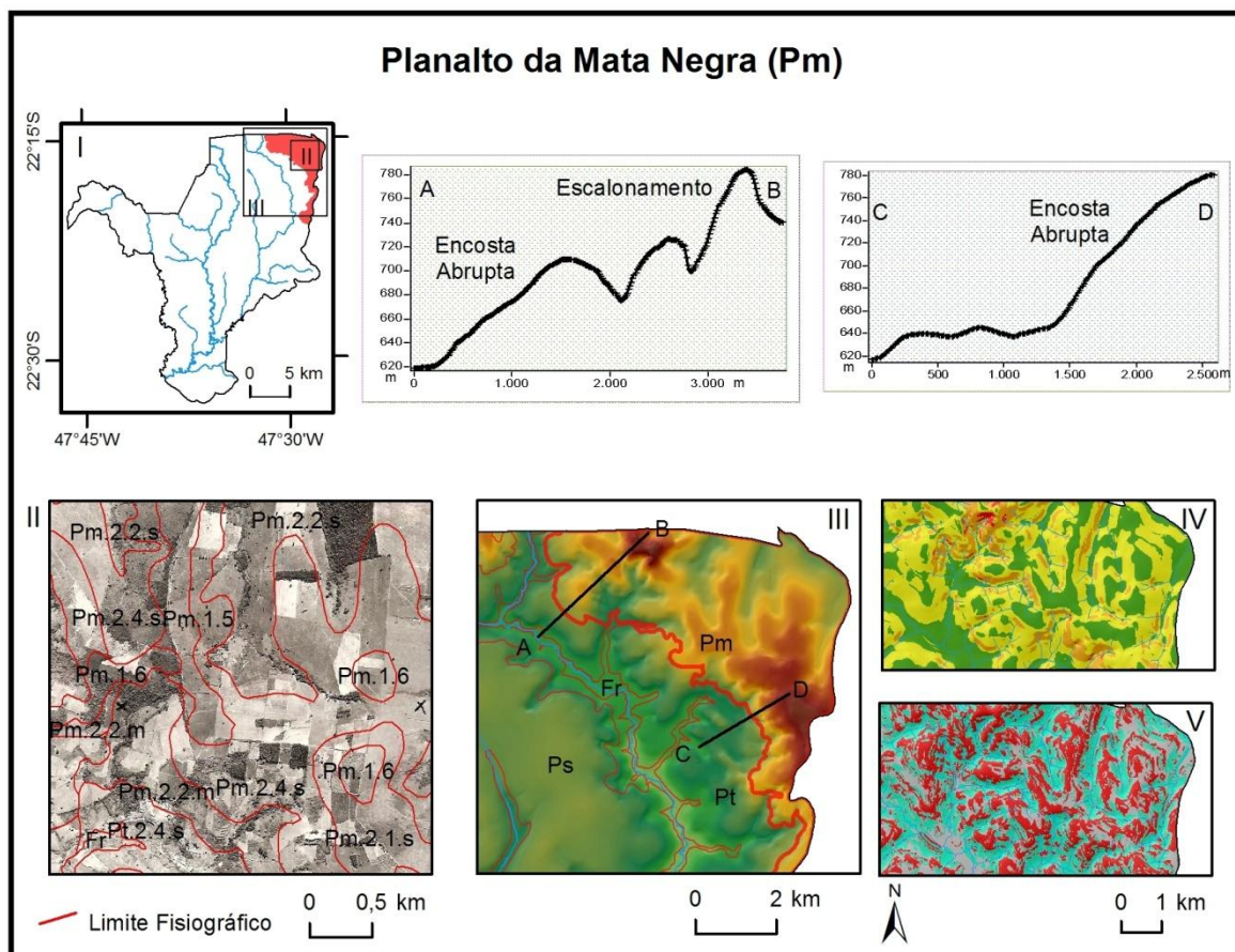
Figura 37: Representação esquemática da unidade do Planalto da Mata Negra. I) localização e distribuição da unidade; II) relevo típico da unidade Pm e subpaisagens; III) níveis altimétricos da unidade Pm na porção nordeste da área; IV) declividade; V) curvatura terreno; A-B e C-D) perfis transversais representativos da paisagem.
