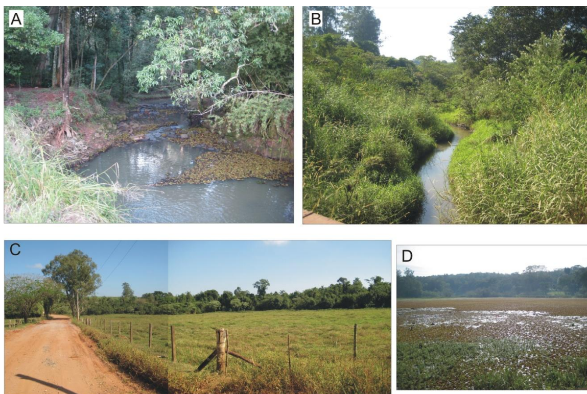
Figura 25: Paisagens representativas da unidade da Planície de Inundação do ribeirão Claro. A) leito do ribeirão Sto. Antônio sobre afloramento de Diabásio (Ponto 83); B) alto curso do ribeirão Claro (Ponto 152); C) planície de inundação no médio curso do ribeirão Claro (Ponto 65) ; D) represa do horto florestal de Rio Claro (Ponto 82).
