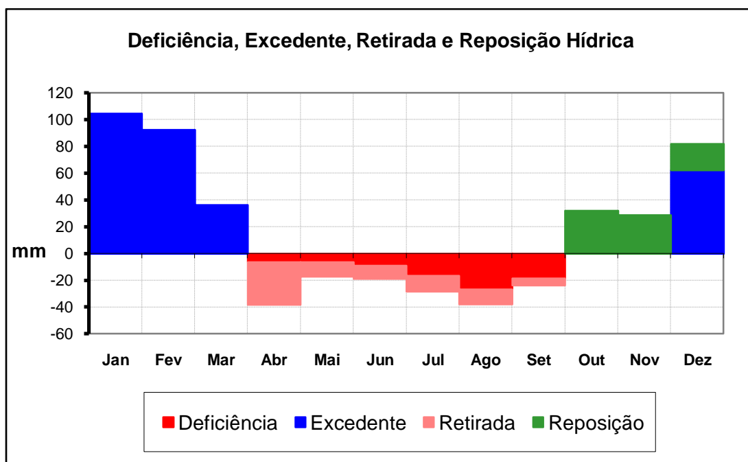
Figura 73: Balanço hídrico e umidade dos solos município de Rio Claro-SP. Fonte DAEE-ESALQ, período de 1941 a 1977 ( http://ce.esalq.usp.br/bhbrasil/Saopaulo/ ).
