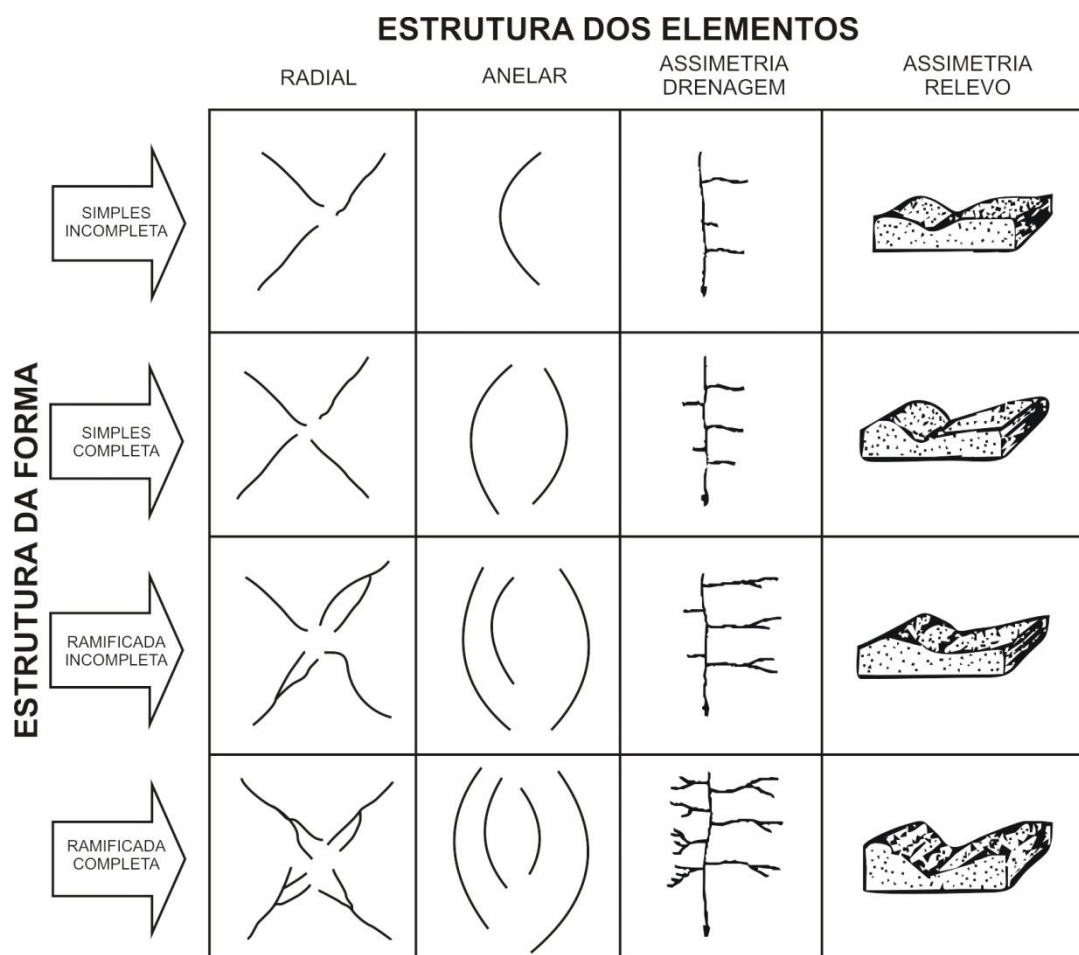
Figura 5: Classificação das formas anômalas, modificado de Soares et al. (1981).
