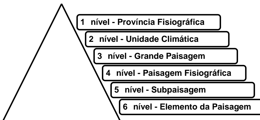
Figura 2: Estrutura piramidal de hierarquização da paisagem, segundo sistema de classificação fisiográfica CIAF – Villota (1992).
