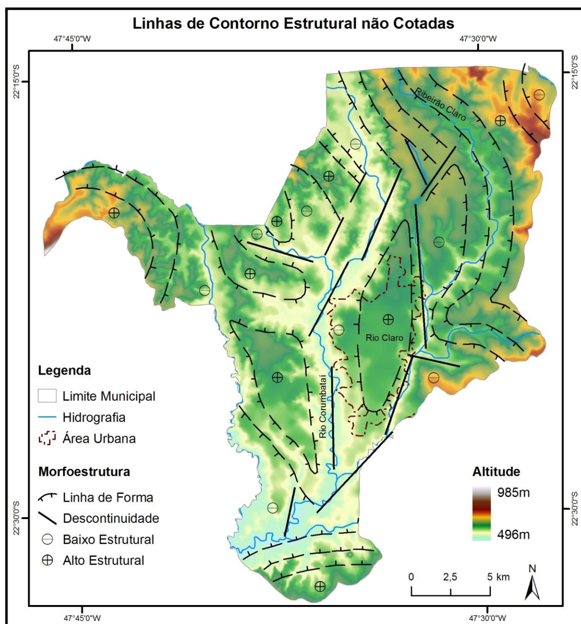
Figura 19: Mapa de linhas de contorno estrutural não cotadas do município de Rio Claro-SP.
