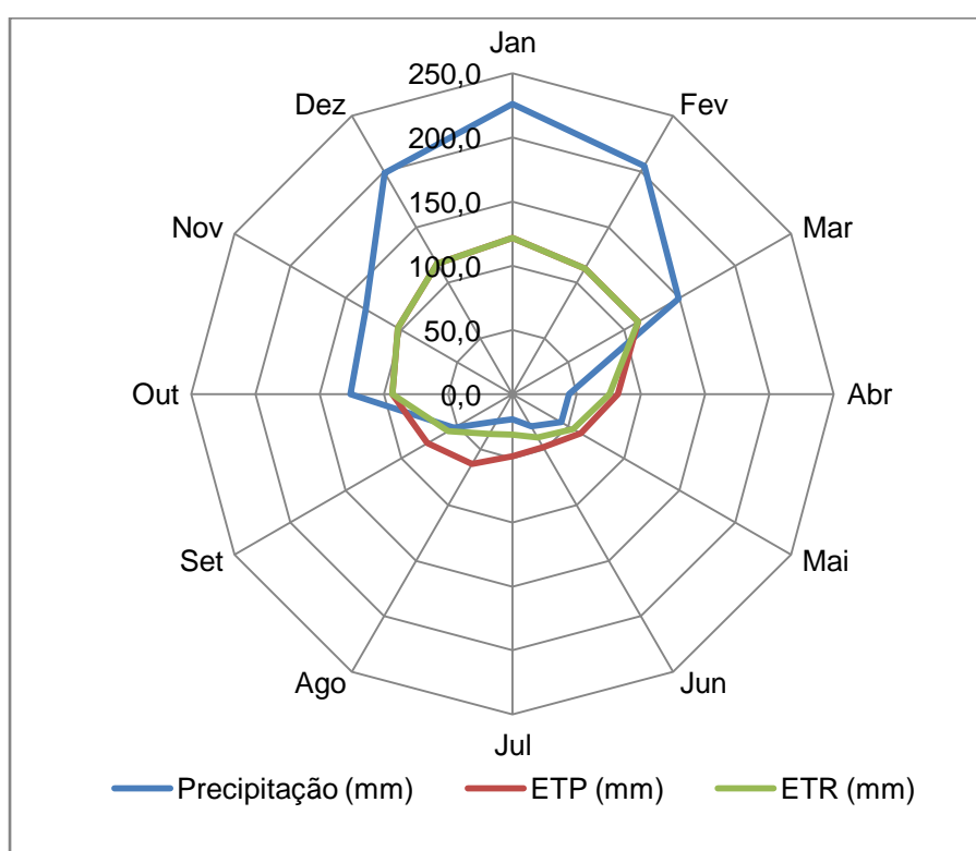
Figura 12: Balanço hídrico do município de Rio Claro-SP. Fonte DAEE-ESALQ, período de 1941 a 1977 ( http://ce.esalq.usp.br/bhbrasil/Saopaulo/ ).
