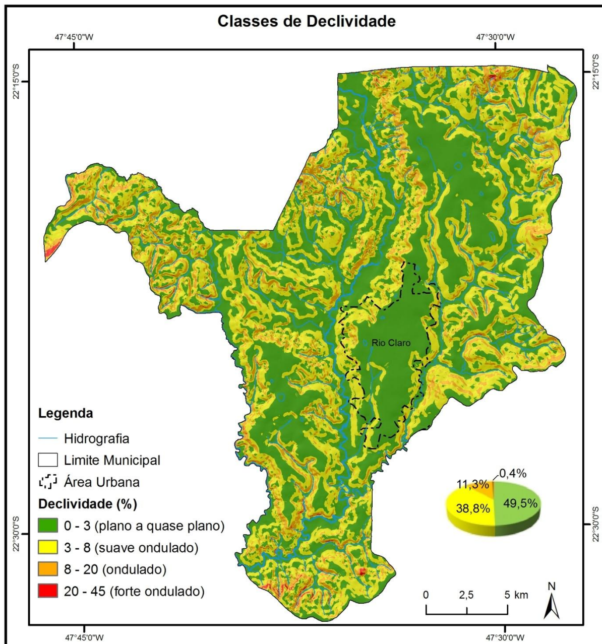
Figura 10: Classes de declividade do município de Rio Claro-SP.
