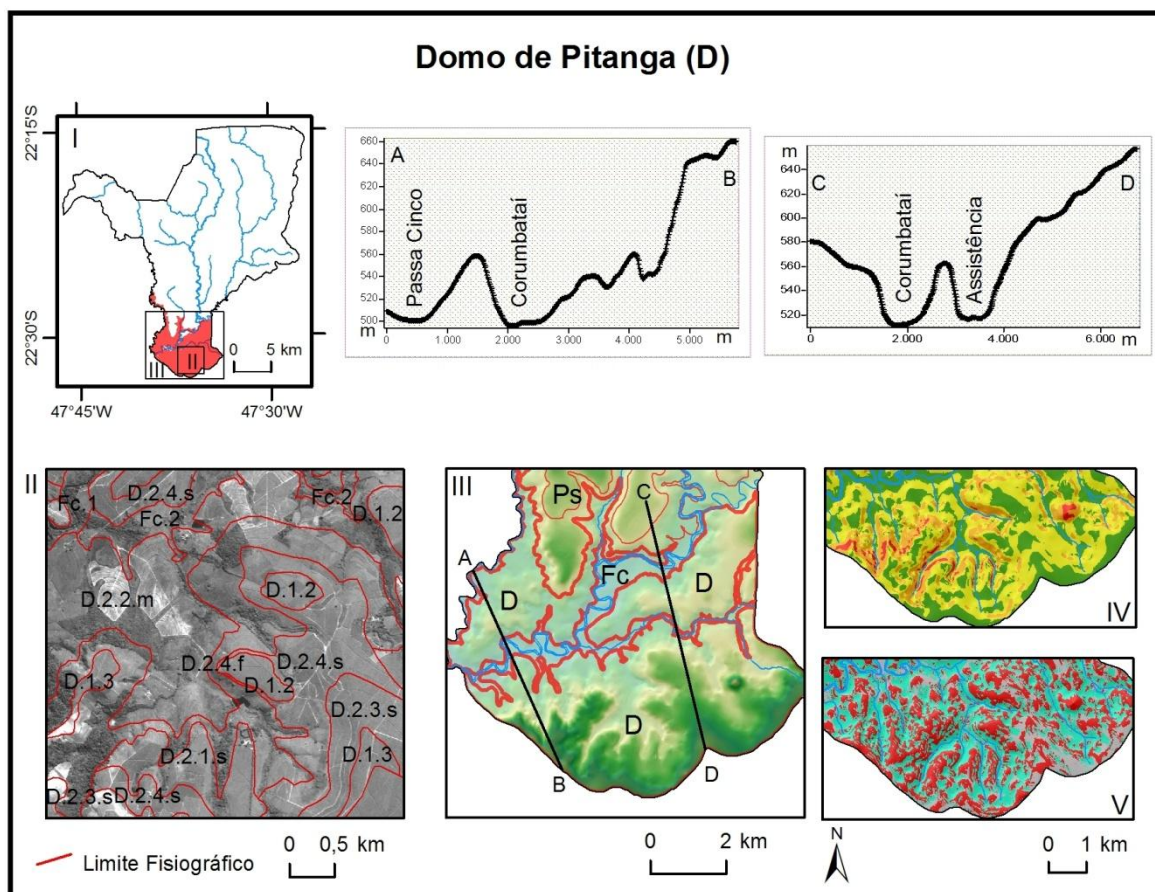
Figura 39: Representação esquemática da unidade do Domo de Pitanga. I) localização e distribuição da unidade; II) relevo típico da unidade D e subpaisagens; III) níveis altimétricos da unidade D na porção sul da área; IV) declividade; V) curvatura terreno; A-B e C-D) perfis transversais representativos da paisagem.
