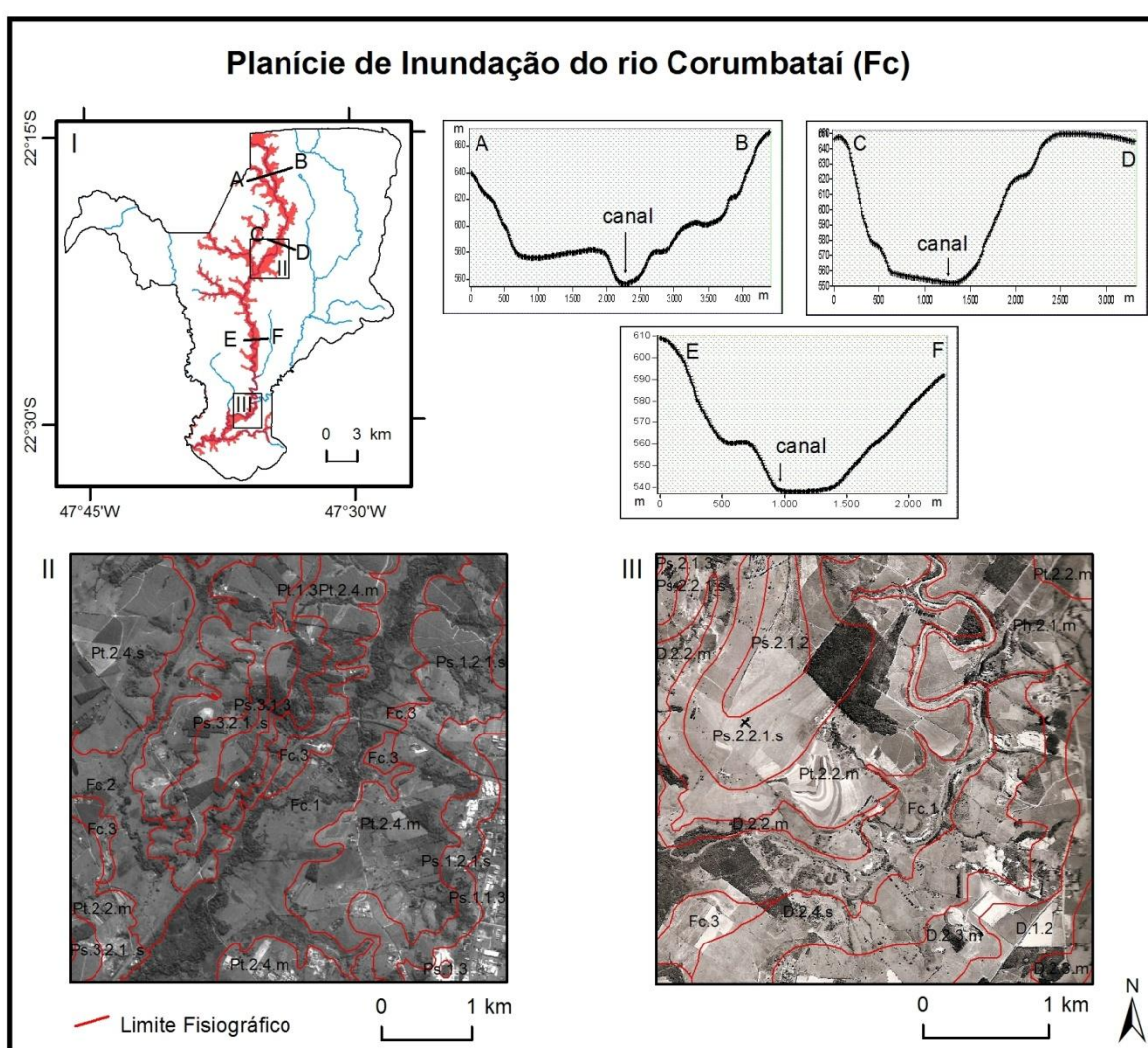
Figura 21: Representação esquemática da unidade Planície de Inundação do rio Corumbataí. I) localização e distribuição da unidade; II) trecho do rio Corumbataí com meandramento e terraços; III) trecho do rio Corumbataí com forte influência estrutural na configuração da planície; A-B, C-D e E-F) perfis transversais representativos da paisagem.
