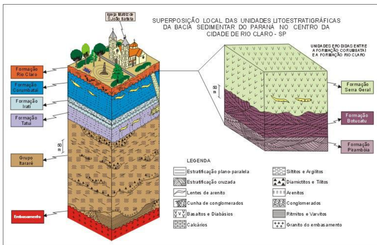
Figura 7: Estratigrafia local da Bacia do Paraná na cidade de Rio Claro - SP, de acordo com Perinotto & Zaine (1996, apud CEAPLA, 2010).
