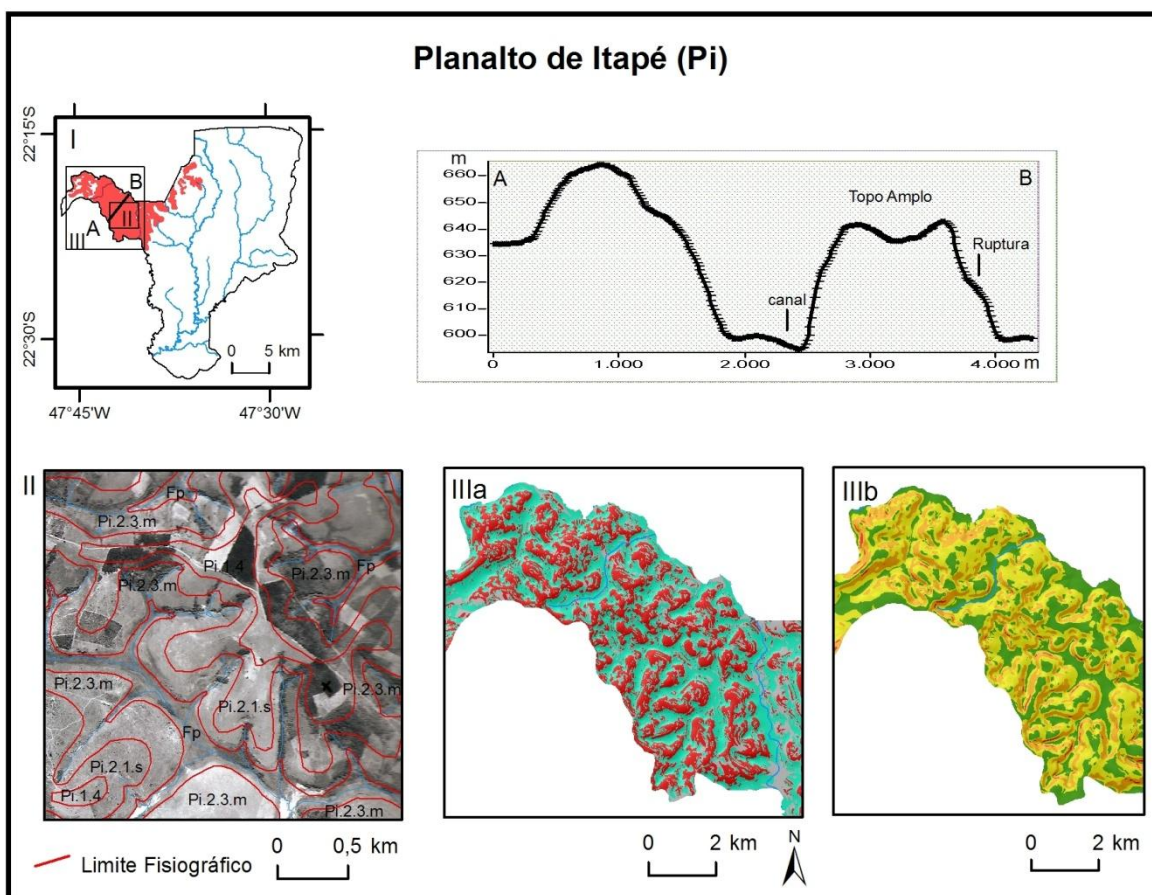
Figura 30: Representação esquemática da unidade do Planalto de Itapé. I) localização e distribuição da unidade; II) relevo típico da unidade Pi e subpaisagens; III) curvatura terreno; IV) declividade; A-B) perfil transversal representativo da paisagem.
