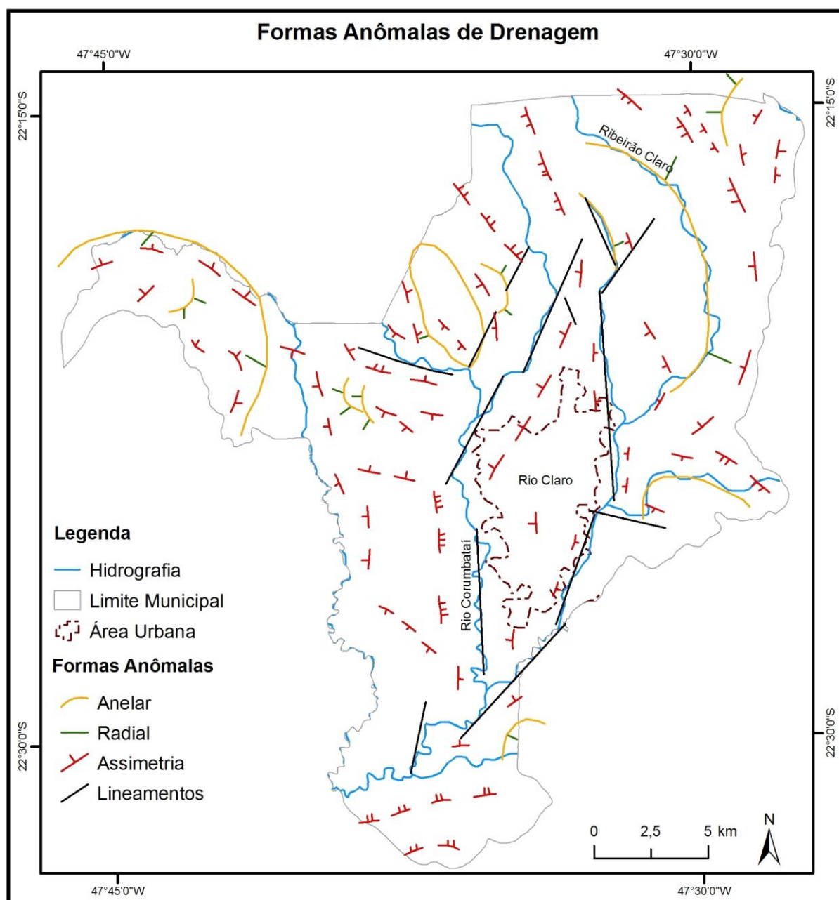
Figura 18: Mapa de formas anômalas de drenagem, a partir de fotografias aéreas 1:25.000.
