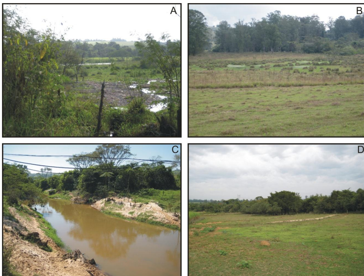
Figura 22: Paisagens representativas da unidade da Planície de Inundação do rio Corumbataí. A) área alagada próxima a cidade de Rio Claro (Ponto 194); B) lagoas marginais (Ponto 153); C) rio Corumbataí e diques marginais (Ponto 165); D) planície do rio Corumbataí na porção sul da área, aproximadamente 4 m acima do nível do rio (Ponto 168).
