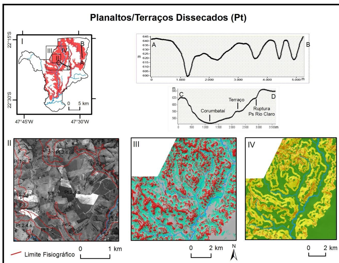
Figura 28: Representação esquemática da unidade dos Planaltos/Terraços dissecados. I) localização e distribuição da unidade; II) relevo típico da unidade Pt e subpaisagens; III) curvatura terreno; IV) declividade; A-B, C-D e E-F) perfis transversais representativos da paisagem.
