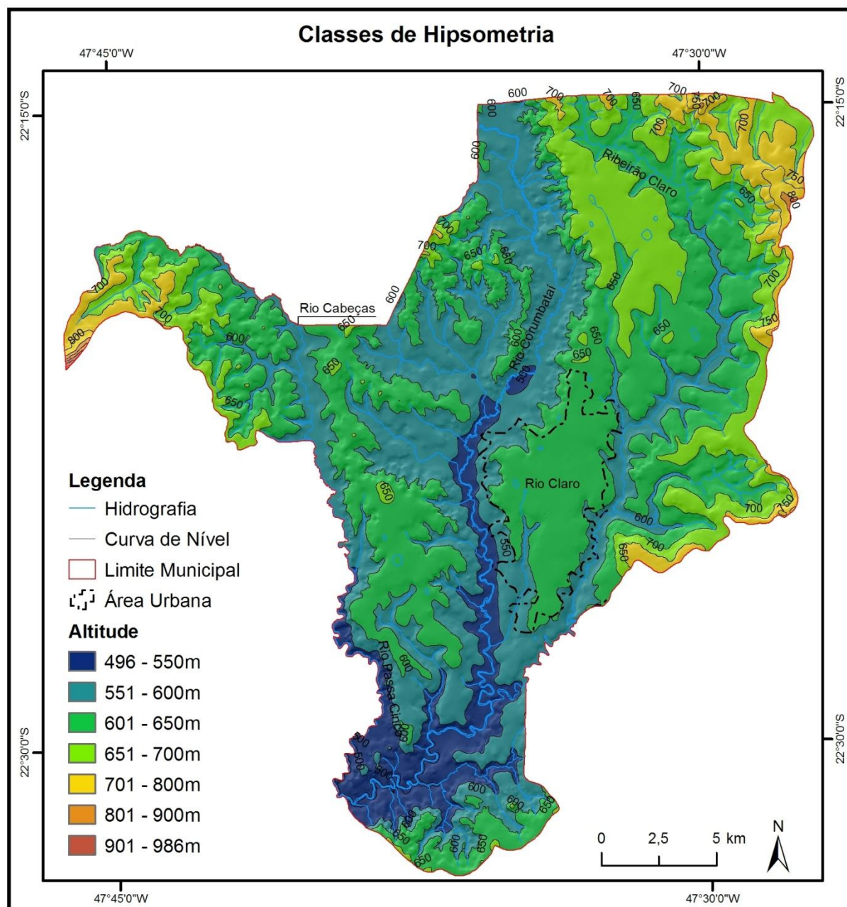
Figura 9: Classes de hipsometria do município de Rio Claro- SP, representando as variações de altitude da área.
