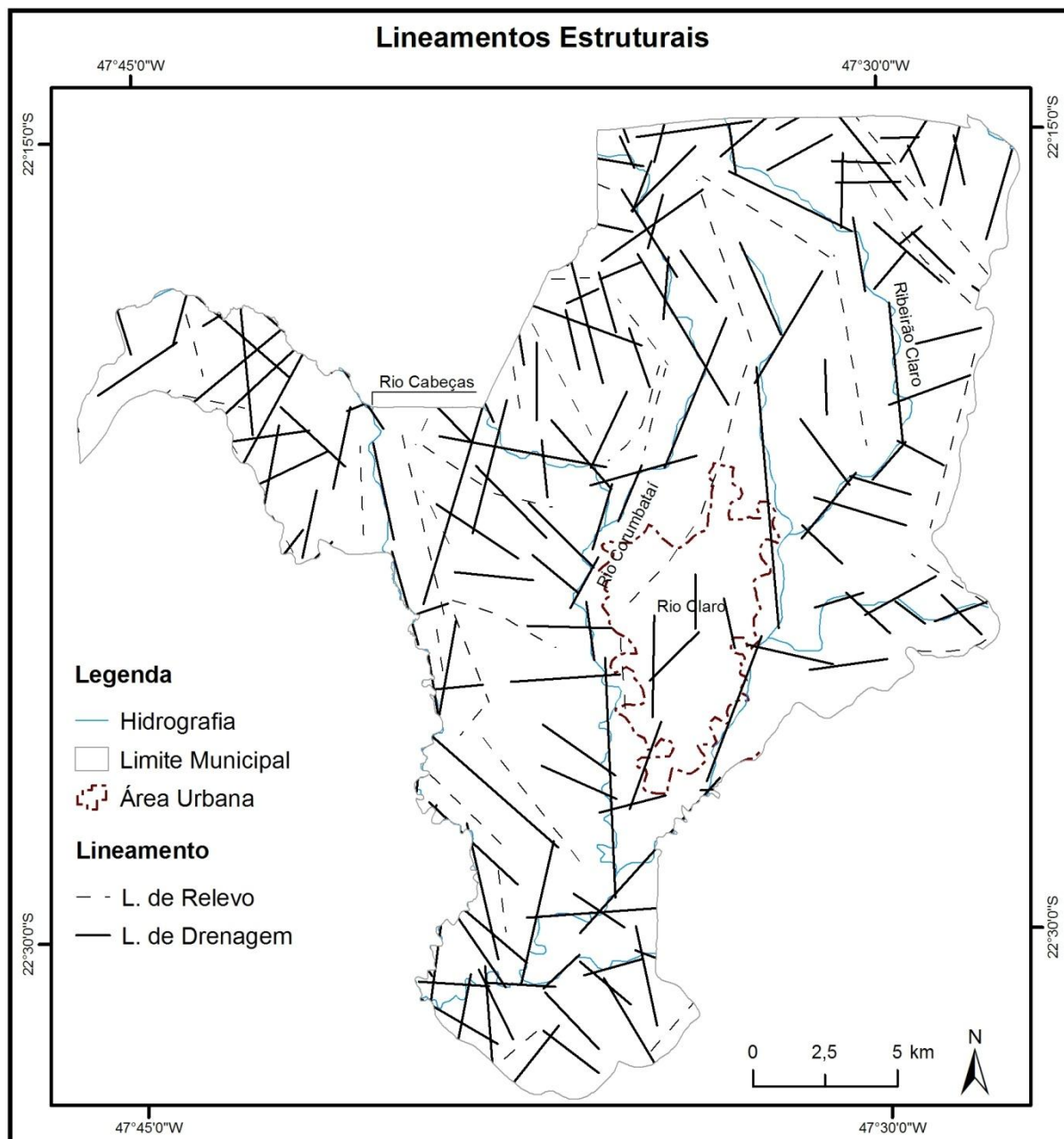
Figura 14: Mapa de lineamentos estruturais do município de Rio Claro - SP.
