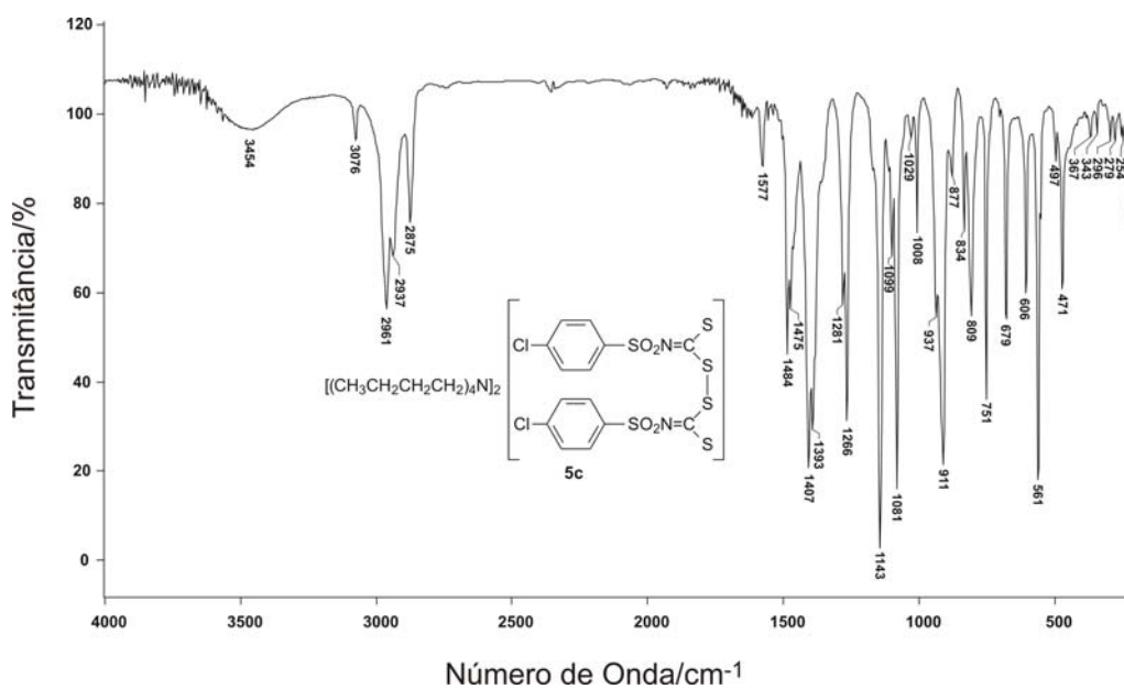
Espectro no infravermelho do bis(4-clorofenilsulfonilthiocarbimoyl)disulfeto de tetrabutilamônio 5c (pastilha de CsI)
