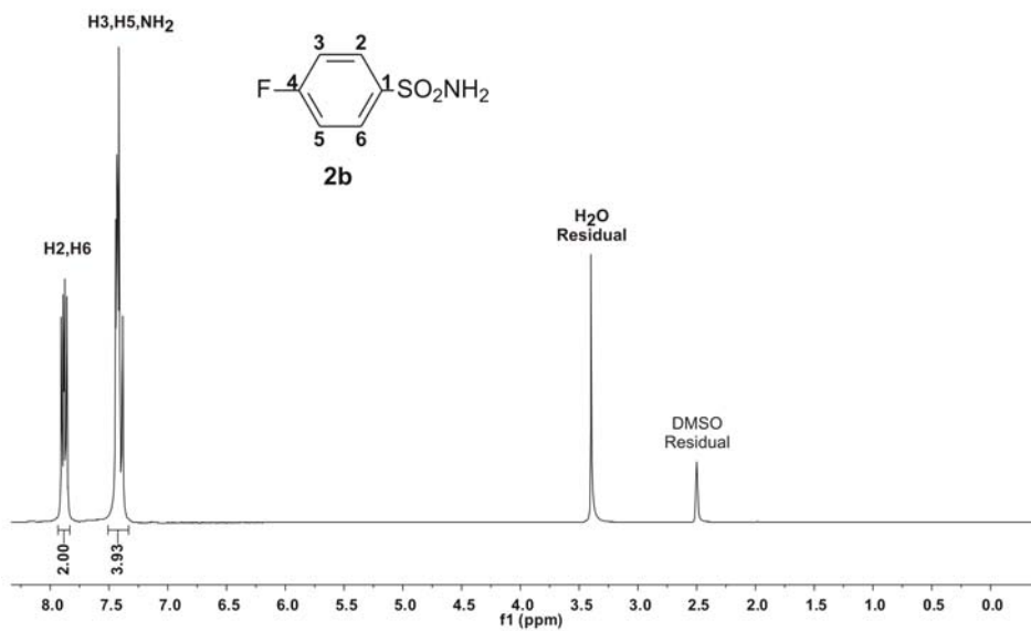
Figura 1.42: Espectro de RMN de 1 H da 4-fluorobenzenossulfonamida 2b em DMSO-D 6 (300 MHz)
