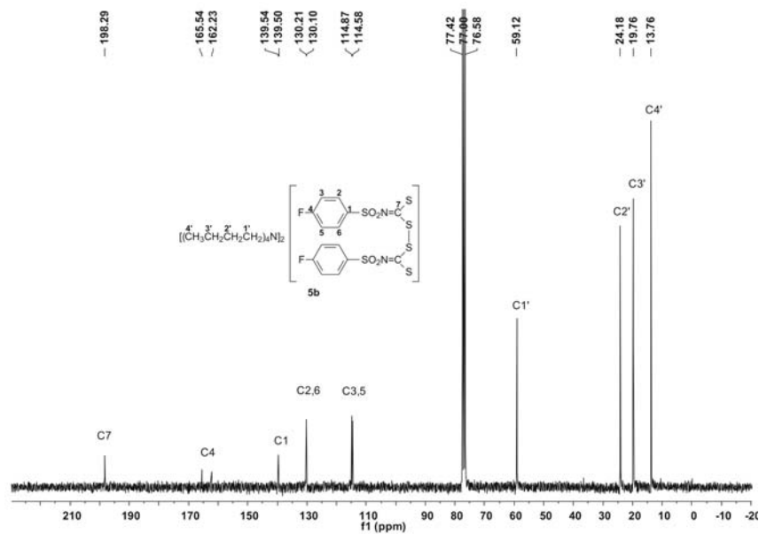
Espectro de RMN de ^{13}\text{C} do bis(4-fluorofenilsulfoniltiocarbimoyl)dissulfeto de tetrabutilamônio 5b ( \text{CDCl}_3 , 75 MHz)
