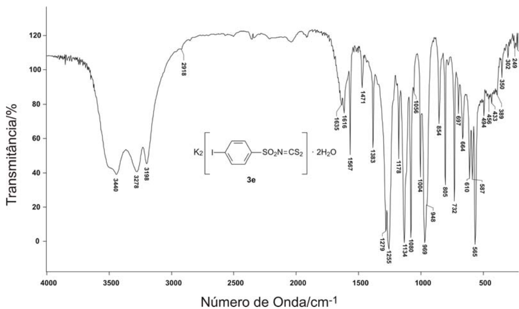
Espectro no infravermelho do 4-iodofenilsulfonilditiocarbimato de potássio diidratado 3e (pastilha de CsI)
