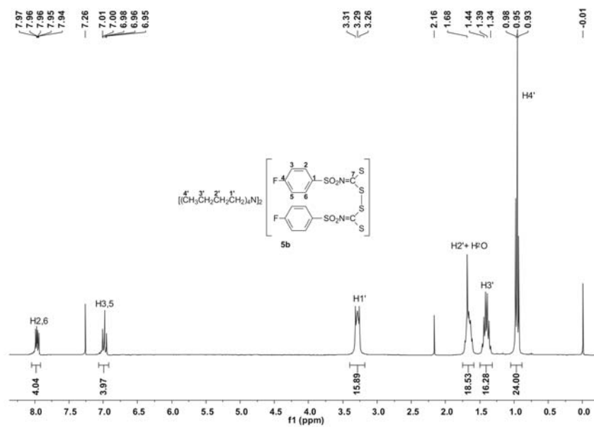
Espectro de RMN de ^1\text{H} do bis(4-fluorofenilsulfoniltiocarbimoyl)dissulfeto de tetrabutilamônio 5b ( \text{CDCl}_3 , 300 MHz)
