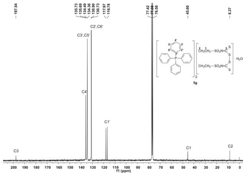
Espectro de RMN de ^{13}\text{C} do bis(etilsulfonilthiocarbimoi)dissulfeto de tetrafenilfosfônio monidratado 5g ( \text{CDCl}_3 , 75 MHz)
