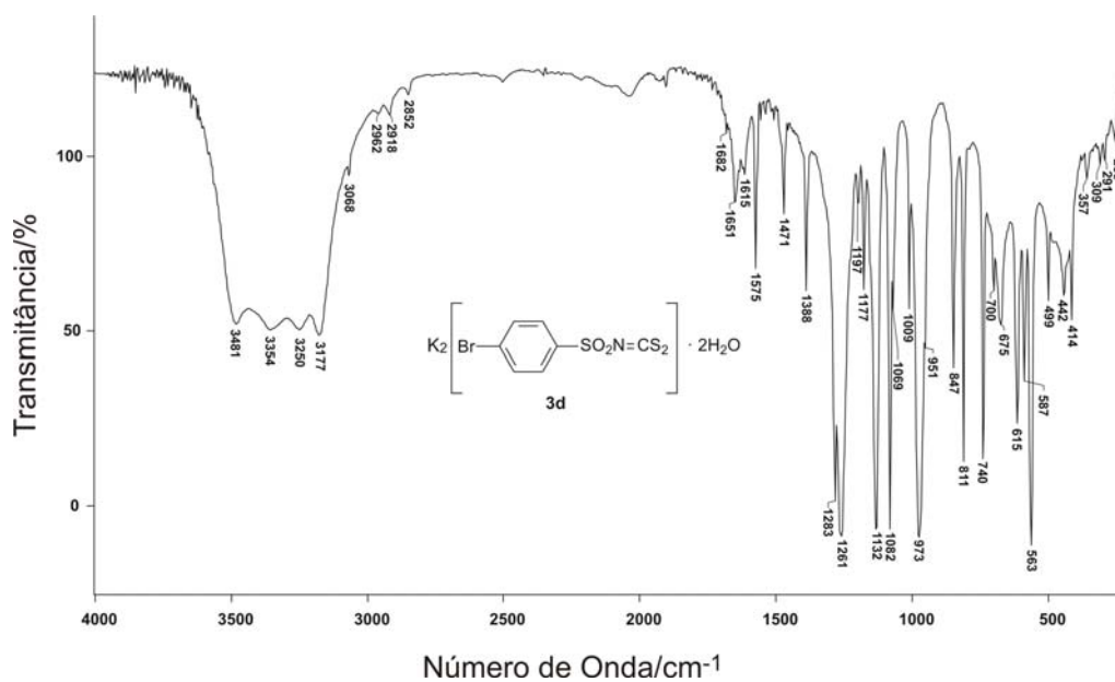
Espectro no infravermelho do 4-bromofenilsulfonilditiocarbimato de potássio diidratado 3d (pastilha de CsI)
