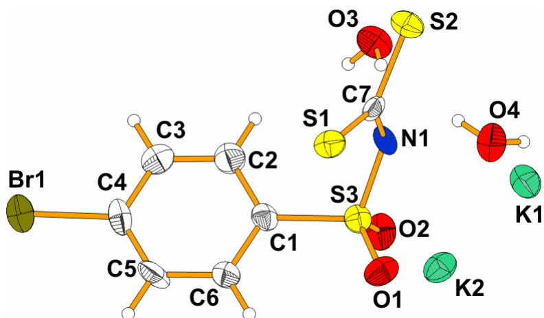
Figura 1.51: Vista molecular obtida por difração de raios-X para o composto 3d
