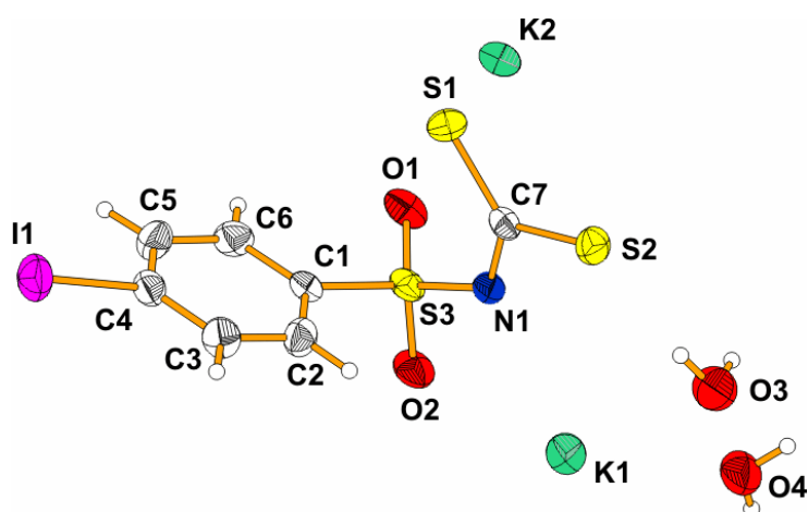
Figura 1.52: Vista molecular obtida por difração de raios-X para o composto 3e
