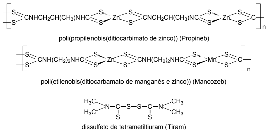
Figura 1.3: Princípios ativos de alguns fungicidas comerciais
