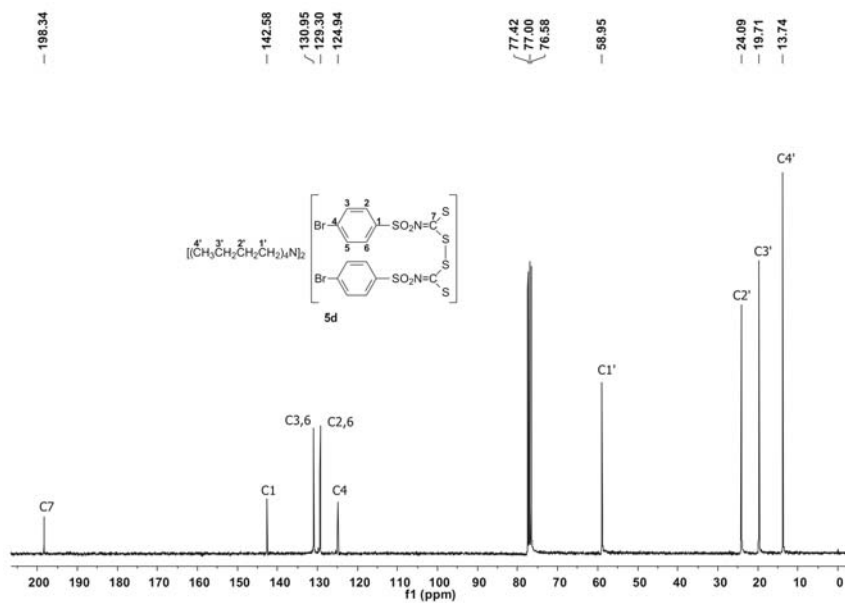
Espectro de RMN de ^{13}\text{C} do bis(4-bromofenilsulfonilcarbimoi) dissulfeto de tetrabutilamônio 5d ( \text{CDCl}_3 , 75 MHz)
