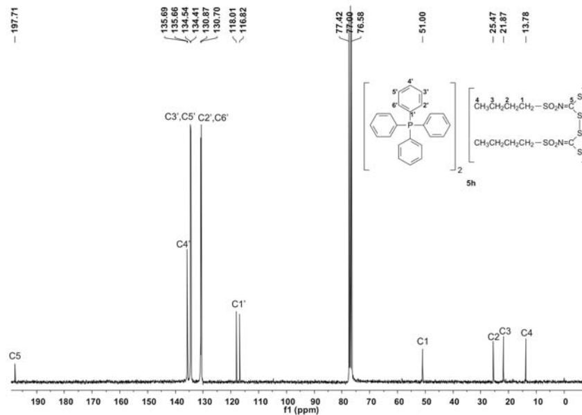
Espectro de RMN de ^{13}\text{C} do bis(butilsulfonilcarbimoi) dissulfeto de tetrafenilfosfônio 5h ( \text{CDCl}_3 , 75 MHz)
