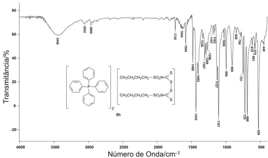
Espectro no infravermelho do bis(butilsulfonilcarbimoi)disulfeto de tetrafenilfosfônio 5h (pastilha de KBr)
