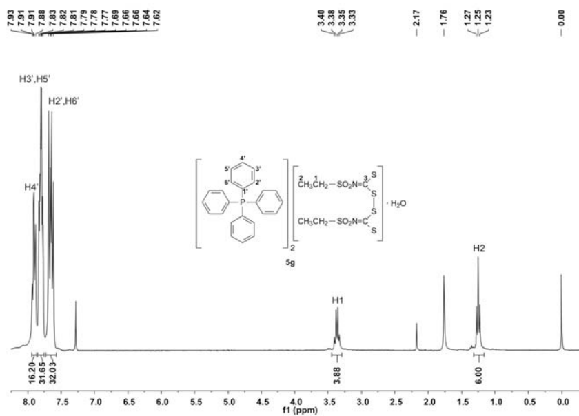
Espectro de RMN de ^1\text{H} do bis(etilsulfonilthiocarbimoi)dissulfeto de tetrafenilfosfônio monidratado 5g ( \text{CDCl}_3 , 300 MHz)
