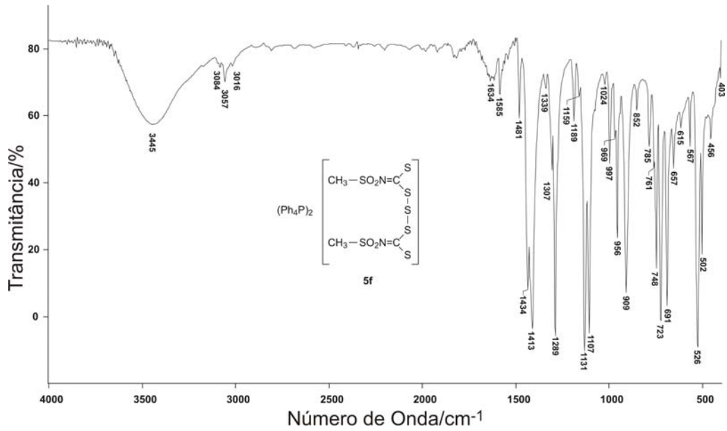
Espectro no infravermelho do bis(metilsulfonilthiocarbimoyl)trissulfeto de tetrafenilfosfônio 5f (pastilha de KBr)
