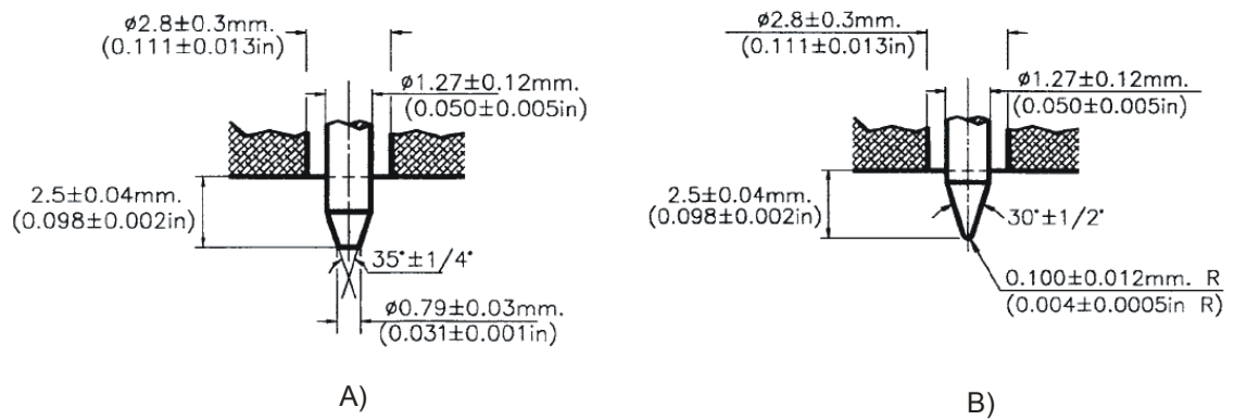
Figura 3.29: Desenhos esquemáticos dos penetradores Shore A (A) e Shore D (B)
