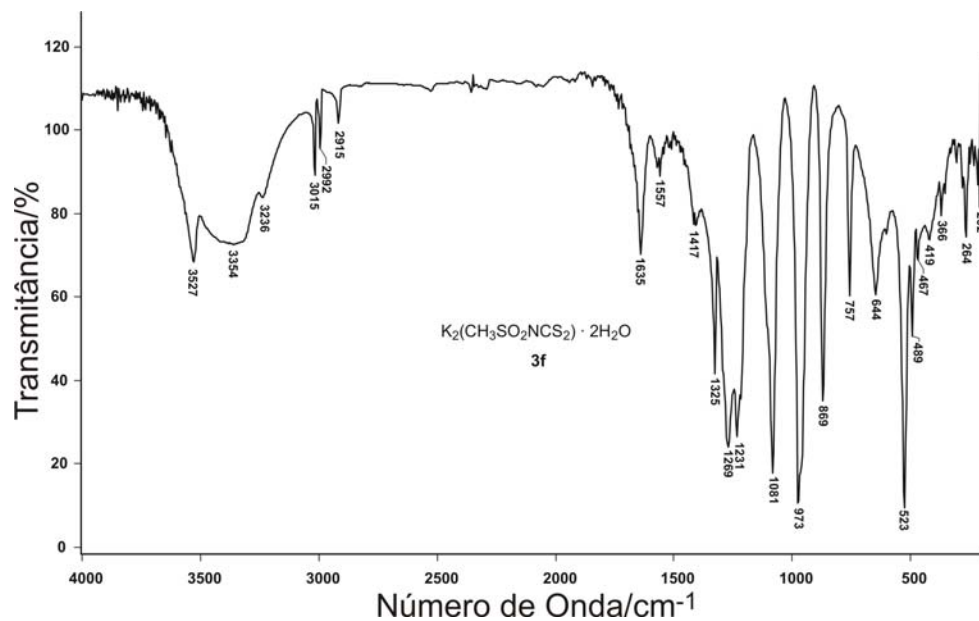
Espectro no infravermelho do metilsulfonilditiocarbimato de potássio diidratado 3f (pastilha de CsI)
