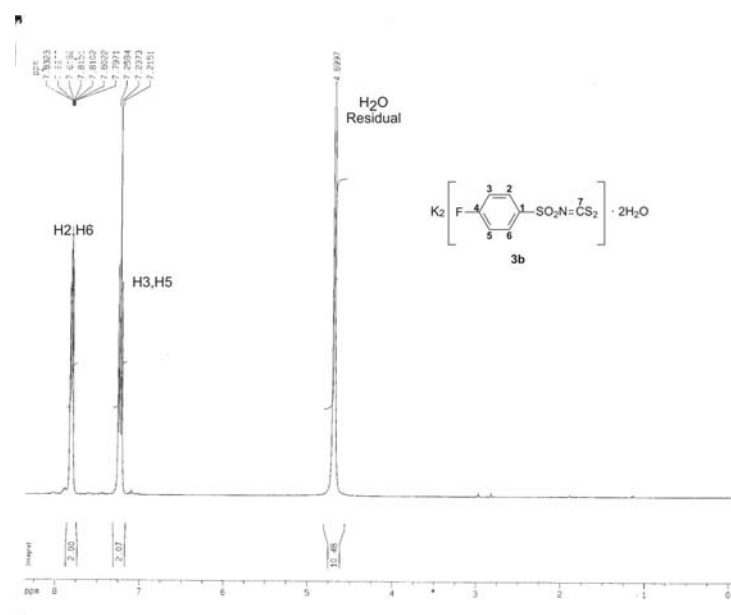
Espectro de RMN de ^1\text{H} do 4-fluorofenilsulfonilditiocarbimato de potássio diidratado 3b ( \text{D}_2\text{O} , 400 MHz)
