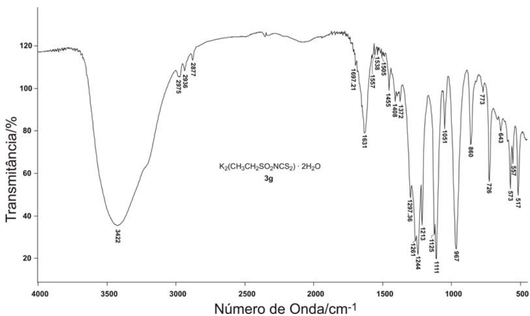
Espectro no infravermelho do etilsulfonilditiocarbimato de potássio diidratado 3g (pastilha de CsI)
