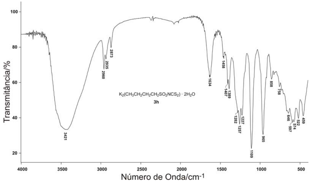
Espectro no infravermelho do butilsulfoniditiocarbimato de potássio diidratado 3h (pastilha de KBr)
