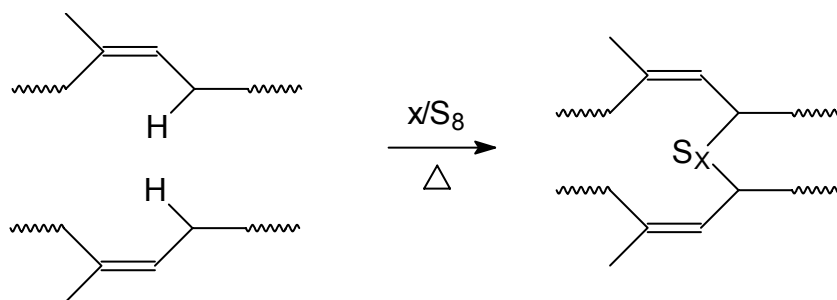
Figura 3.3: Formação de ligações sulfídicas cruzadas
