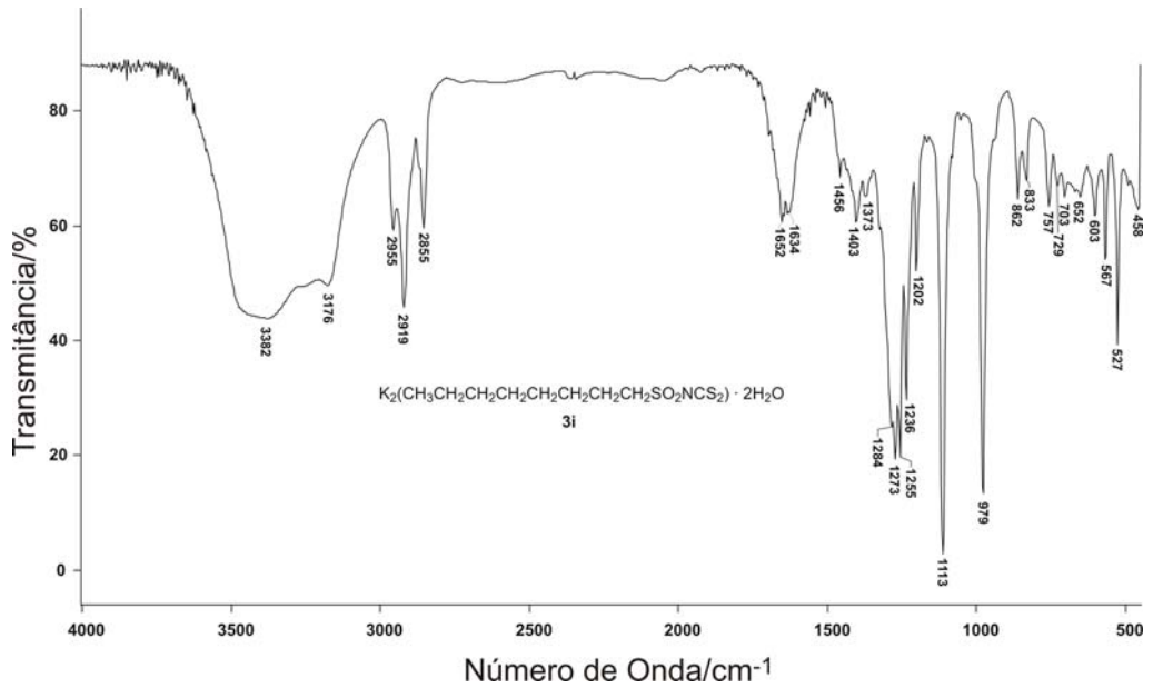
Espectro no infravermelho do octilsulfoniditiocarbimato de potássio diidratado 3i (pastilha de KBr)
