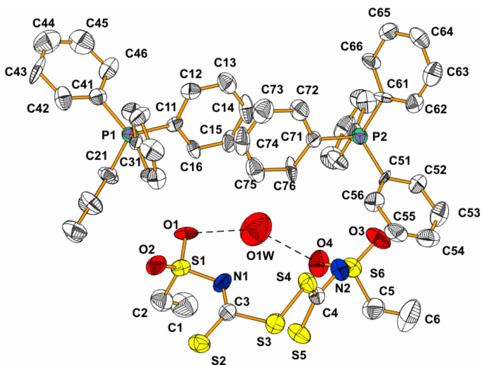
Figura 1.78: Vista molecular da unidade assimétrica do composto 5g
