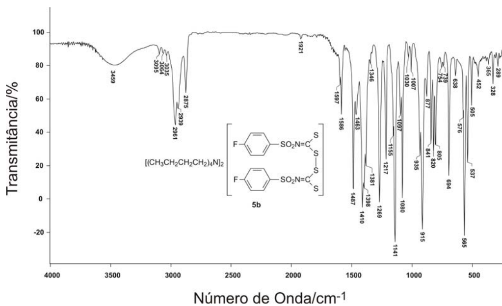
Espectro no infravermelho do bis(4-fluorofenilsulfonilthiocarbimoyl)disulfeto de tetrabutilamônio 5b (pastilha de CsI)
