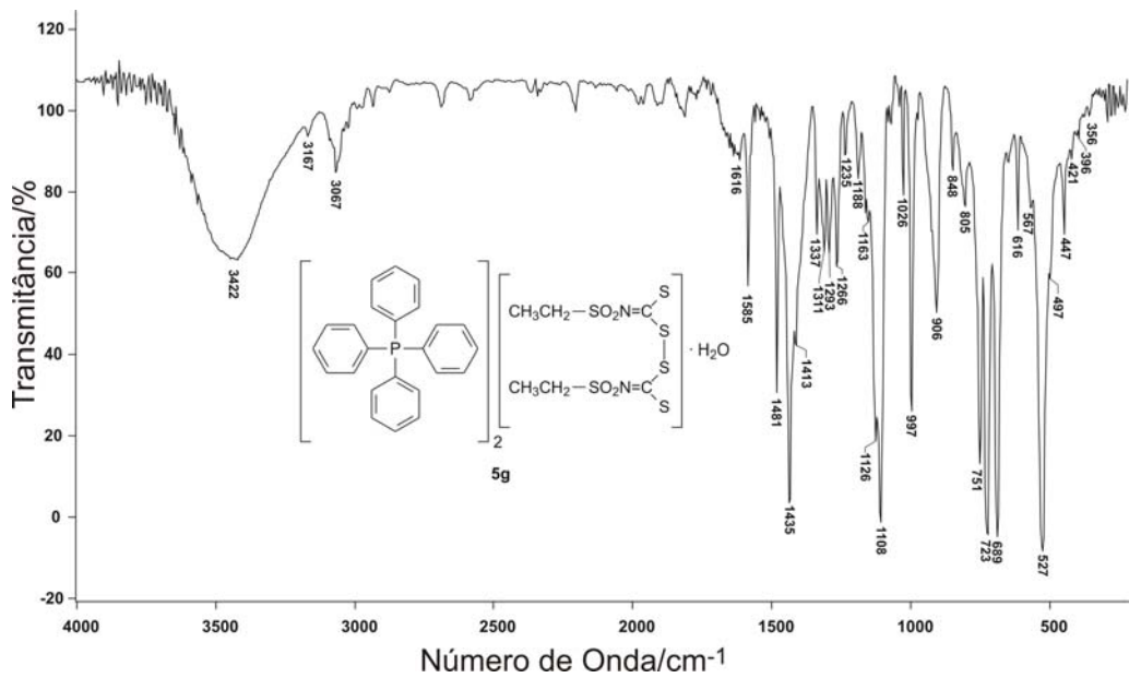
Espectro no infravermelho do bis(etilsulfonilthiocarbimoyl)dissulfeto de tetrafenilfosfônio monidratado 5g (pastilha de CsI)
