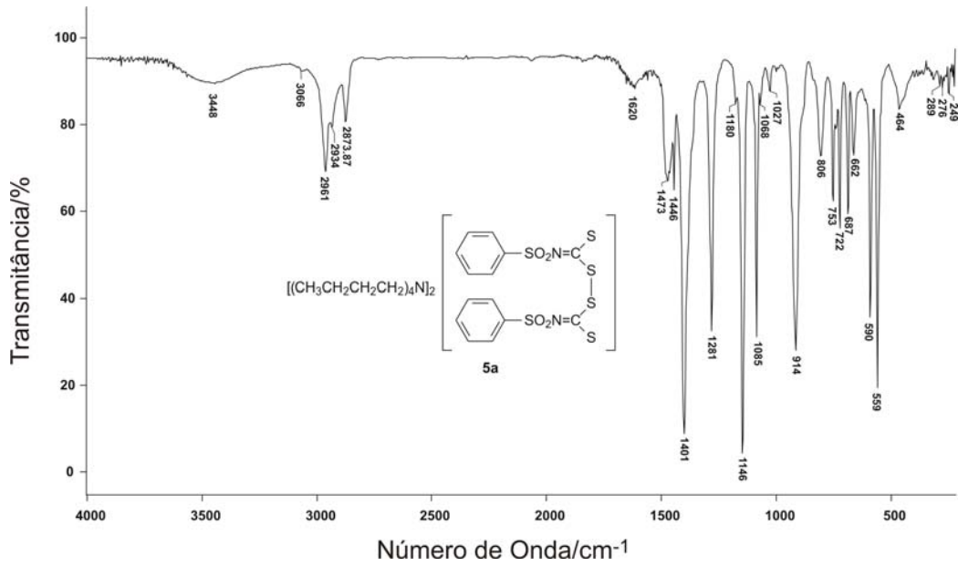
Espectro no infravermelho do bis(fenilsulfoniltiocarbimoi)dissulfeto de tetrabutilamônio 5a (pastilha de CsI)
