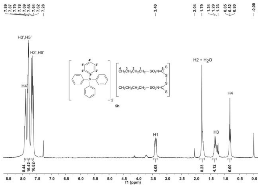
Espectro de RMN de ^1\text{H} do bis(butilsulfonilcarbimoi) dissulfeto de tetrafenilfosfônio 5h ( \text{CDCl}_3 , 300 MHz)
