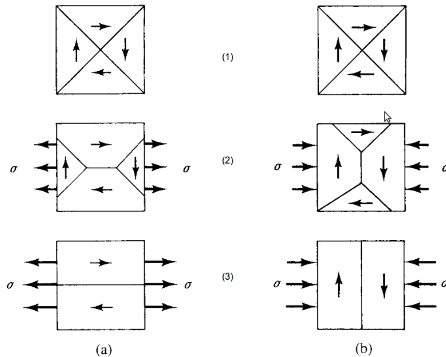
Figura 2.11: Magnetização de um material com magnetostricção positiva. Em (a-1) temos primeiramente o material livre de tensões aplicadas, em (a-2) temos a aplicação de uma tensão que vem a alargar o material na direção horizontal, ou \sigma > 0 , em (a-3) temos como consequência dessa tensão o realinhamento dos momentos magnéticos paralelo a essa, pois \sigma\lambda > 0 . Nas figuras relativas ao conjunto (b) a diferença é o sentido da tensão aplicada sobre o material. Uma compressão resultará em \sigma\lambda < 0 , e assim, o realinhamento é perpendicular à direção da tensão. Extraído de [2].
