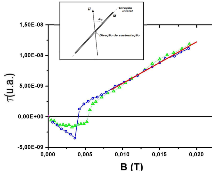
Figura 3.14: Curva \tau vs B para a amostra A4 (500Å sobre vidro), a curva azul é feita para \alpha_c formando 45° com a direção inicial, mostrada no topo da figura, estando o eixo fácil do plano paralelo a essa, e a curva verde é feita da mesma forma, agora, com o eixo de difícil magnetização do plano ao longo da direção inicial. A reta em vermelho é o ajuste linear feito, com a finalidade de determinar a magnetização de saturação, como será discutido em seguida.
