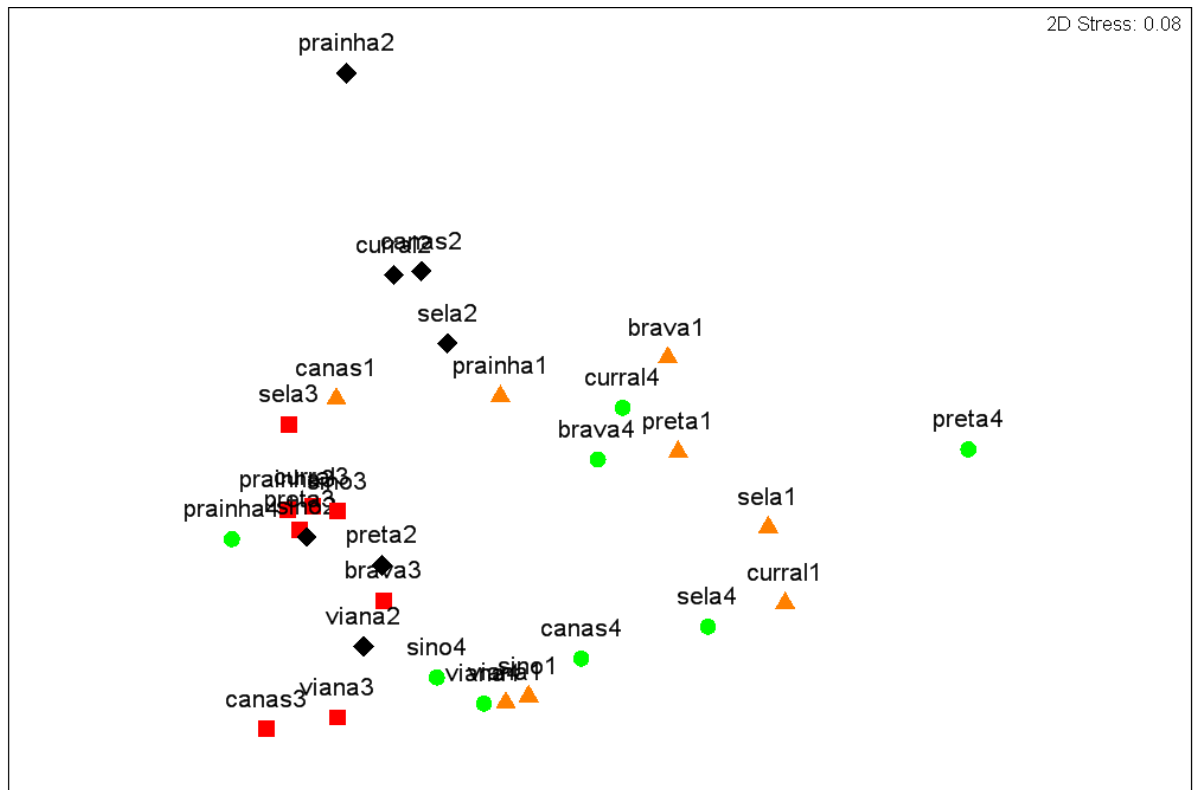
Figura 3. Ordenação do MDS caracterizando o padrão de separação dos períodos amostrais quanto à composição dos grupos tróficos. Onde, \blacktriangle = outono, \blacklozenge = inverno, \blacksquare = primavera e \bullet = verão. Stress = 0.08.
