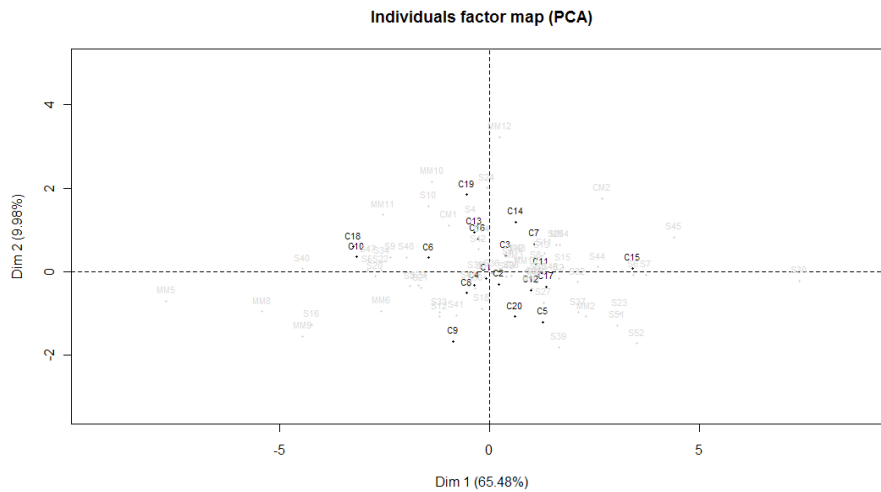
Figura 3 Espaço das amostras, destacando a região do Cerrado mostrada separadamente, para o ano de 2008. Lavras ó MG
