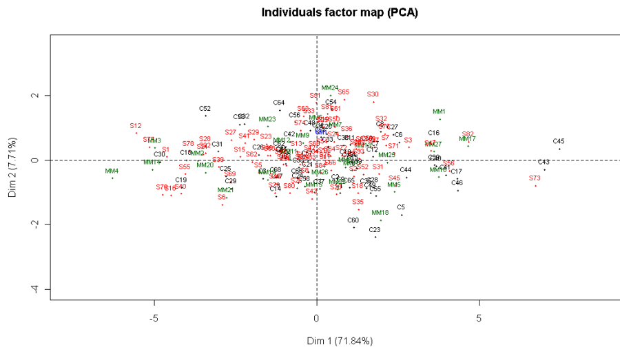
Figura 12 Espaço das amostras, destacando as regiões produtoras (MM: Matas de Minas, CM: Chapadas de Minas, C: Cerrado, S: Sul de Minas), para categoria de Naturais diferenciadas no concurso do ano de 2008. Lavras ó MG
