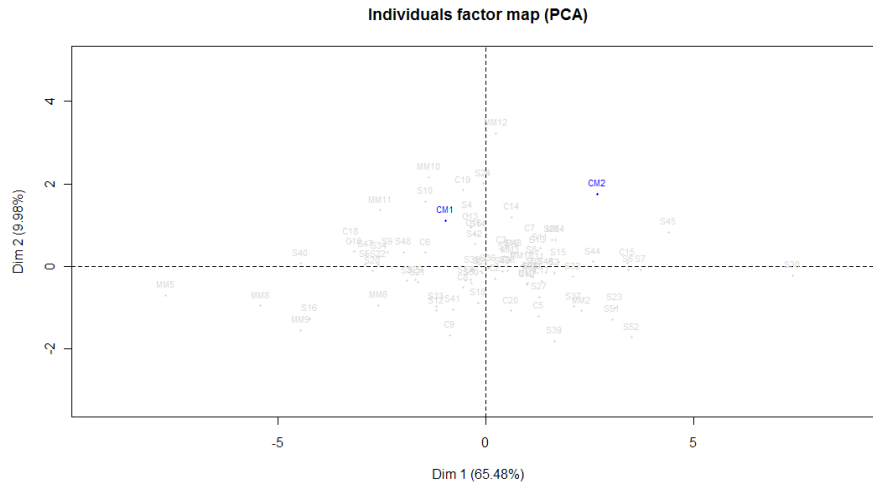
Figura 4 Espaço das amostras, destacando a região das Chapadas de Minas mostrada separadamente, para o ano de 2008. Lavras ó MG
