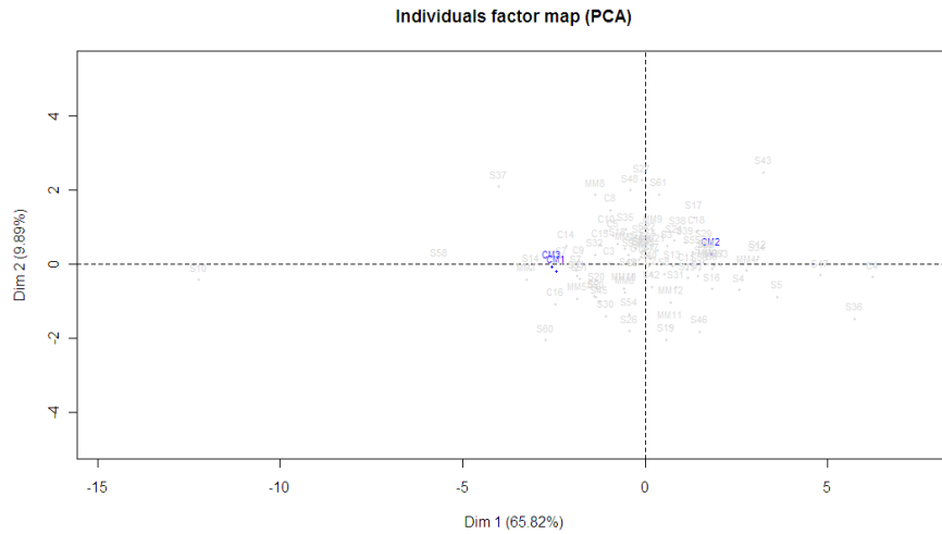
Figura 16 Espaço das amostras, destacando a região das Chapadas de Minas mostrada separadamente, para o ano de 2009. Lavras ó MG
