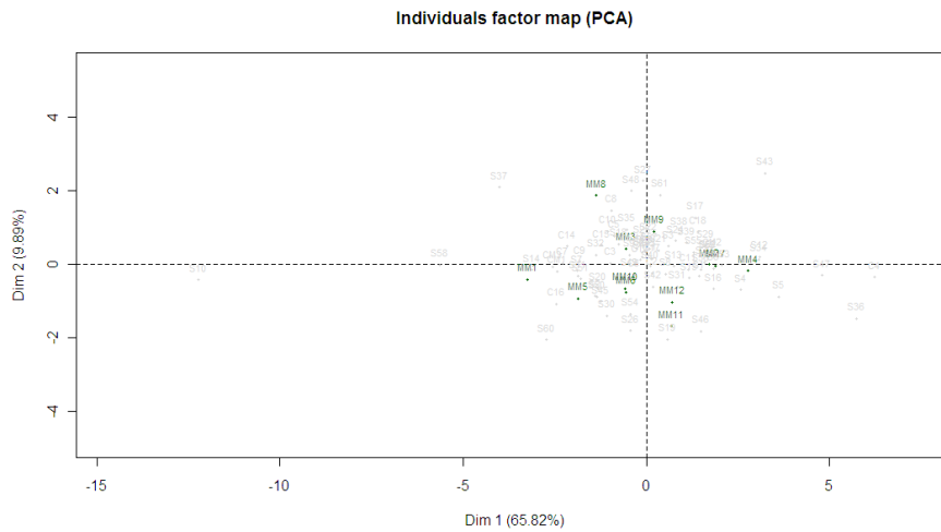
Figura 17 Espaço das amostras, destacando a região das Matas de Minas mostrada separadamente, para o ano de 2009. Lavras ó MG
