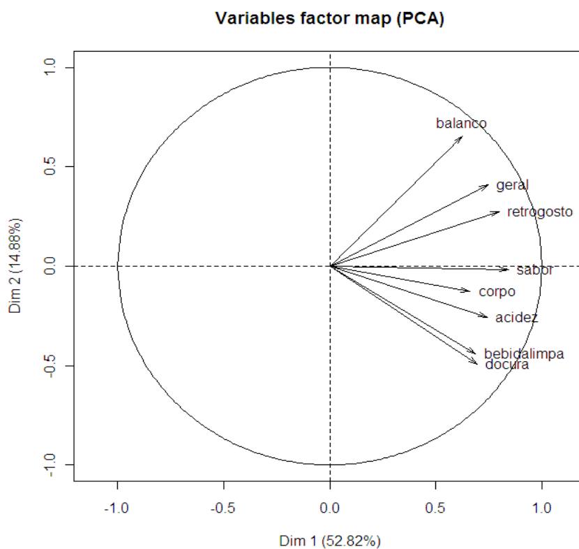
Figura 21 Espaço de variáveis, demonstrando a correlação entre as variáveis sensoriais e os dois primeiros componentes principais dentro do estudo da categoria CD no concurso do ano de 2009. Lavras ó MG
