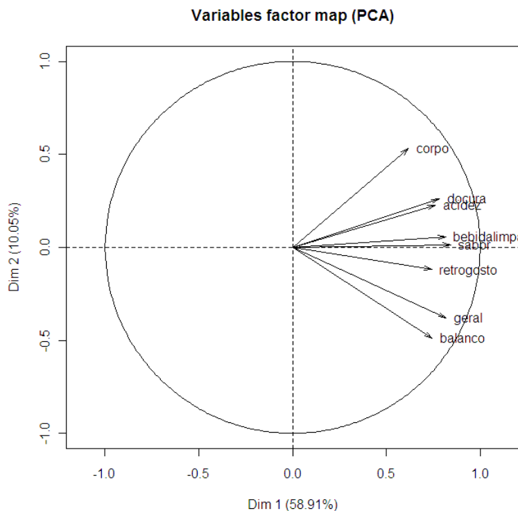
Figura 19 Espaço de variáveis, demonstrando a correlação entre as variáveis sensoriais e os dois primeiros componentes principais dentro do estudo das categorias (Natural e CD) diferenciadas no concurso do ano de 2009. Lavras ó MG
