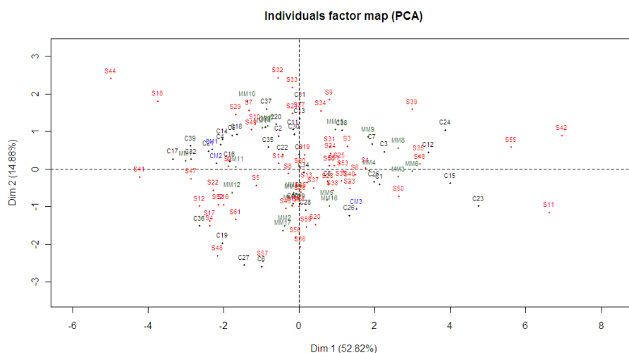
Figura 23 Espaço das amostras, destacando as regiões produtoras (MM: Matas de Minas, CM: Chapadas de Minas, C: Cerrado, S: Sul de Minas), para categoria CD diferenciadas no concurso do ano de 2009. Lavras ó MG
