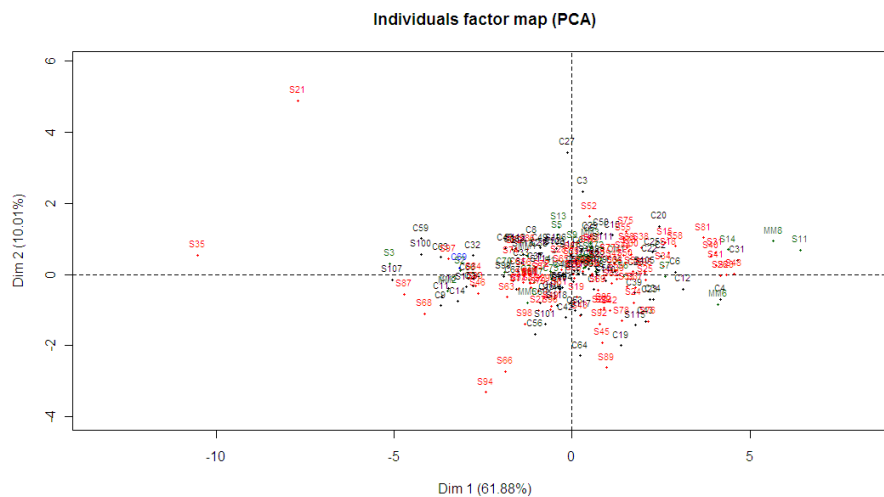
Figura 24 Espaço das amostras, destacando as regiões produtoras (MM: Matas de Minas, CM: Chapadas de Minas, C: Cerrado, S: Sul de Minas), para categoria Natural diferenciadas no concurso do ano de 2009. Lavras ó MG
