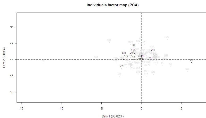
Figura 15 Espaço das amostras, destacando a região do Cerrado mostrada separadamente, para o ano de 2009. Lavras ó MG
