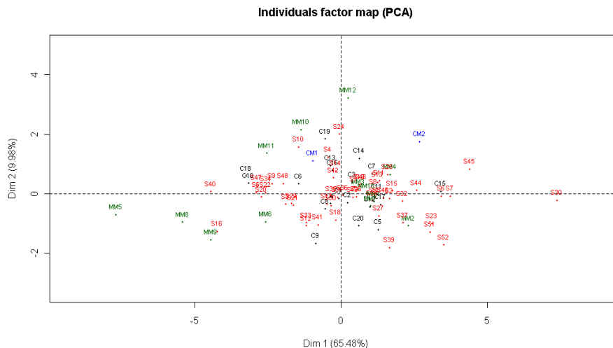
Figura 2 Espaço das amostras, destacando as regiões produtoras (MM: Matas de Minas, CM: Chapadas de Minas, C: Cerrado, S: Sul de Minas), para o ano de 2008. Lavras ó MG
