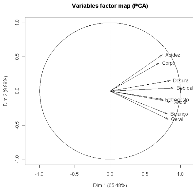
Figura 1 Espaço de variáveis, demonstrando a correlação entre as variáveis sensoriais e os dois primeiros componentes principais dentro das quatro regiões estudadas do ano de 2008. Lavras ó MG
