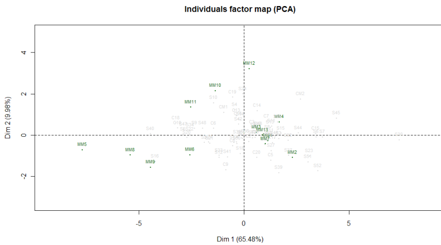
Figura 5 Espaço das amostras, destacando a região das Matas de Minas mostrada separadamente, para o ano de 2008. Lavras ó MG
