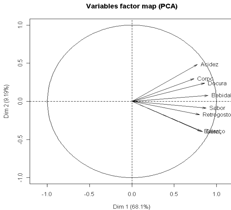
Figura 7 Espaço de variáveis, demonstrando a correlação entre as variáveis sensoriais e os dois primeiros componentes principais dentro do estudo das categorias (Natural e CD) diferenciadas no concurso do ano de 2008. Lavras ó MG
