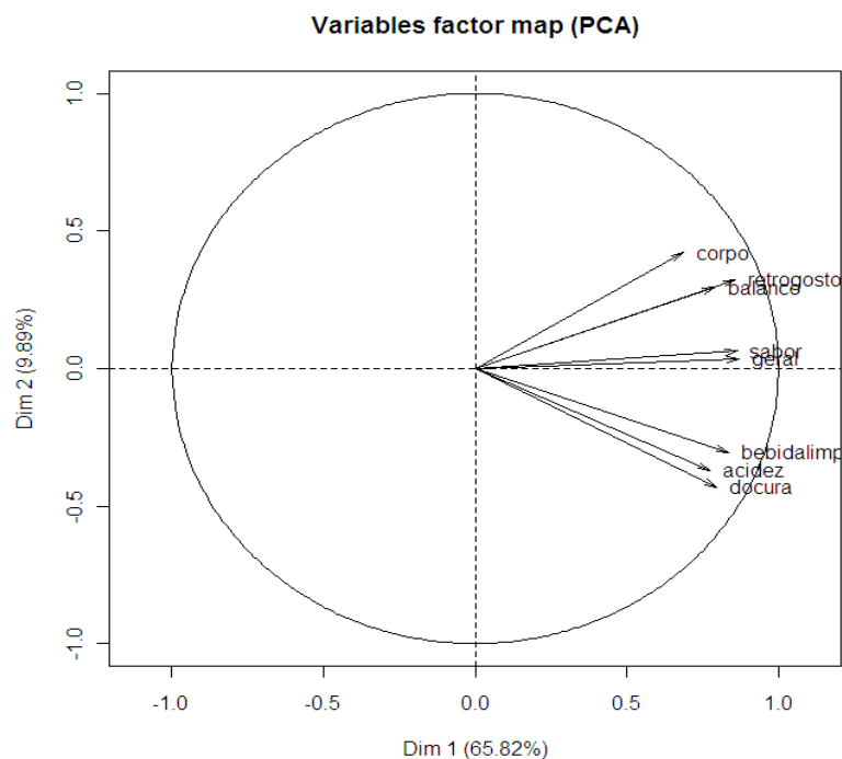
Figura 13 Espaço de variáveis, demonstrando a correlação entre as variáveis sensoriais e os dois primeiros componentes principais dentro das quatro regiões estudadas do ano de 2009. Lavras ó MG
