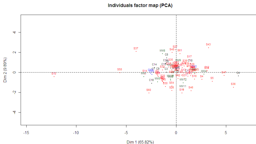
Figura 14 Espaço das amostras, destacando as regiões produtoras (MM: Matas de Minas, CM: Chapadas de Minas, C: Cerrado, S: Sul de Minas), para o ano de 2009. Lavras ó MG
