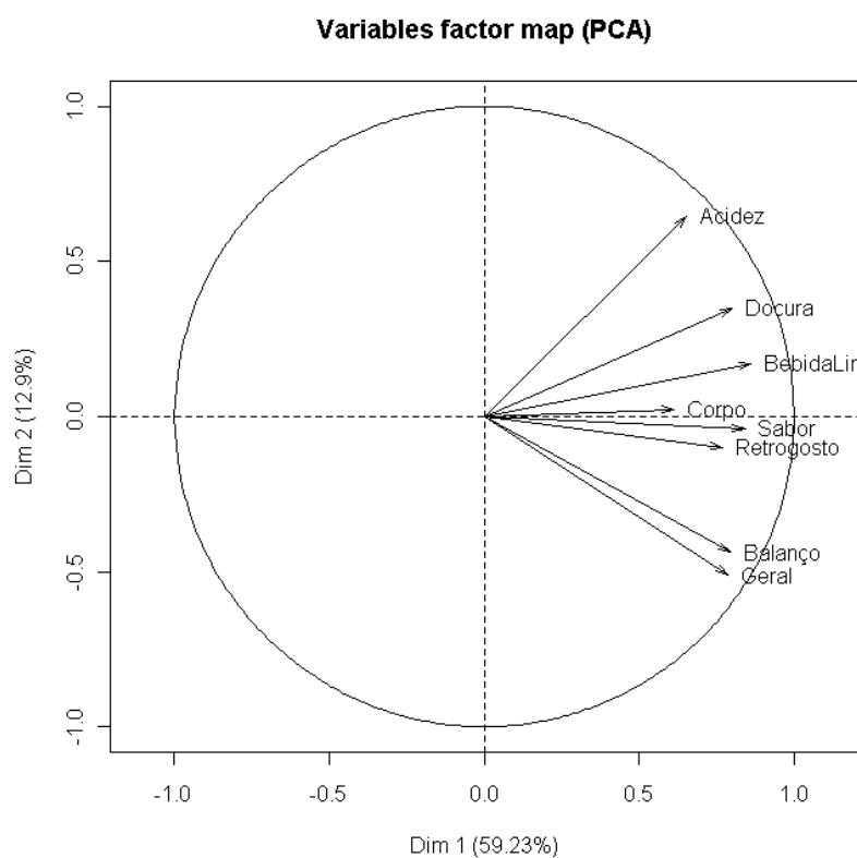
Figura 10 Espaço de variáveis, demonstrando a correlação entre as variáveis sensoriais e os dois primeiros componentes principais dentro do estudo da categoria Natural diferenciadas no concurso do ano de 2008. Lavras ó MG
