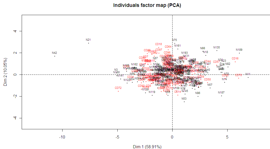
Figura 20 Espaço das amostras, destacando as categorias (Natural e CD) para o ano de 2009. Lavras ó MG
