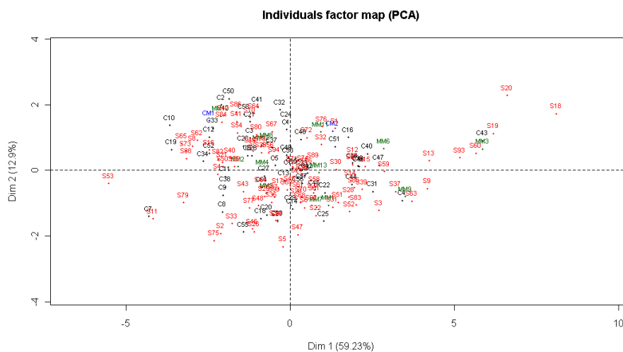
Figura 11 Espaço das amostras, destacando as regiões produtoras (MM: Matas de Minas, CM: Chapadas de Minas, C: Cerrado, S: Sul de Minas), para categoria CD diferenciadas no concurso do ano de 2008. Lavras ó MG
