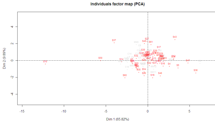
Figura 18 Espaço das amostras, destacando a região Sul de Minas mostrada separadamente, para o ano de 2009. Lavras ó MG
