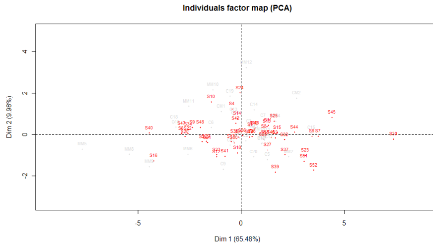
Figura 6 Espaço das amostras, destacando a região do Sul de Minas mostrada separadamente, para o ano de 2008. Lavras ó MG
