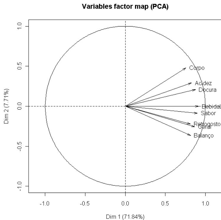
Figura 9 Espaço de variáveis, demonstrando a correlação entre as variáveis sensoriais e os dois primeiros componentes principais dentro do estudo da categoria CD no concurso do ano de 2008. Lavras ó MG
