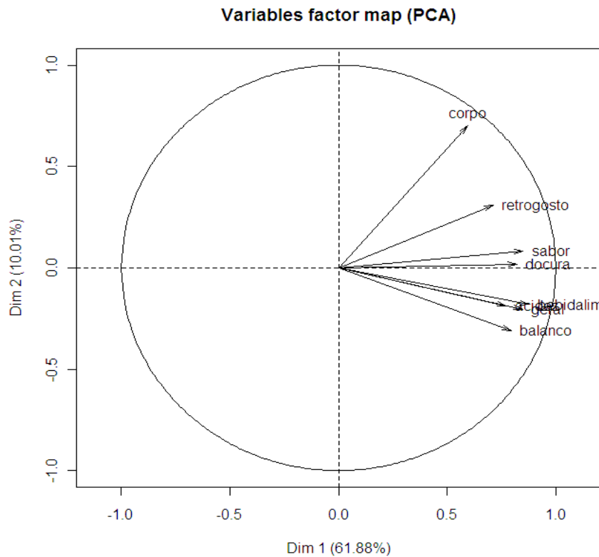
Figura 22 Espaço de variáveis, demonstrando a correlação entre as variáveis sensoriais e os dois primeiros componentes principais dentro do estudo da categoria Natural diferenciadas no concurso do ano de 2009. Lavras ó MG
