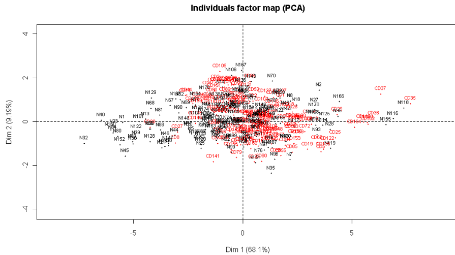
Figura 8 Espaço das amostras, destacando as categorias (Natural e CD) para o ano de 2008. Lavras ó MG
