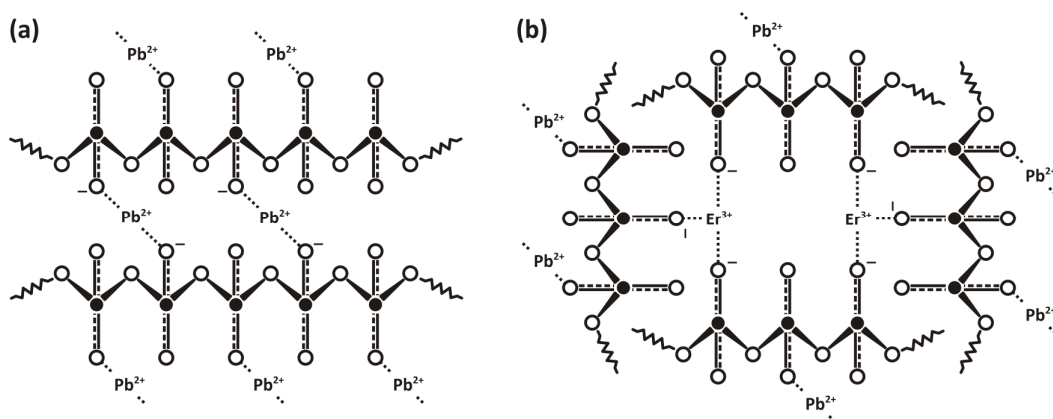
Figura 3.9. Representação esquemática da estrutura dos vidros EDLP evidenciando a ação dos modificadores de rede ( \text{Pb}^{2+} e \text{Er}^{3+} ).
