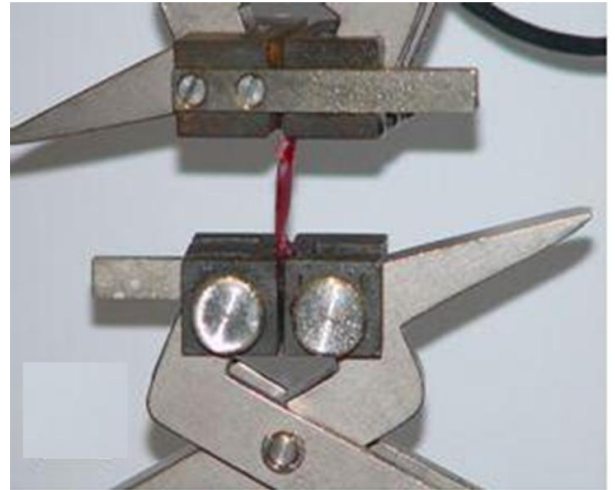
Figura 12 – a) Garra utilizada para fixar o material durante os ensaios de tração; b) músculo sóleo fixado às garras.
