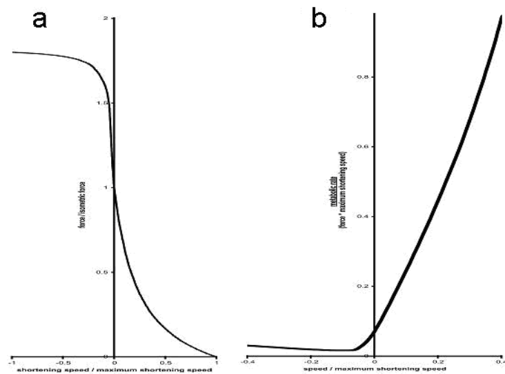
Figura 8 – Propriedades do músculo esquelético de vertebrados a partir de equações empíricas. a) relação força x velocidade de contração do músculo; b) relação do custo metabólico pela velocidade de contração do músculo. Fonte: ALEXANDER, 1997.
