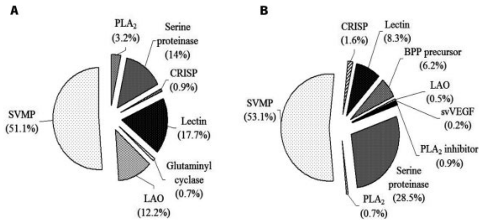
Figura 1.4 – Análise proteômica e transcriptômica de peçonhas de serpente. (A) Composição protéica determinada por proteômica da peçonha de Bothrops jararaca , (B) composição de Bothrops jararaca determinada por transcriptoma. Fonte: Fox et al., 2006.
