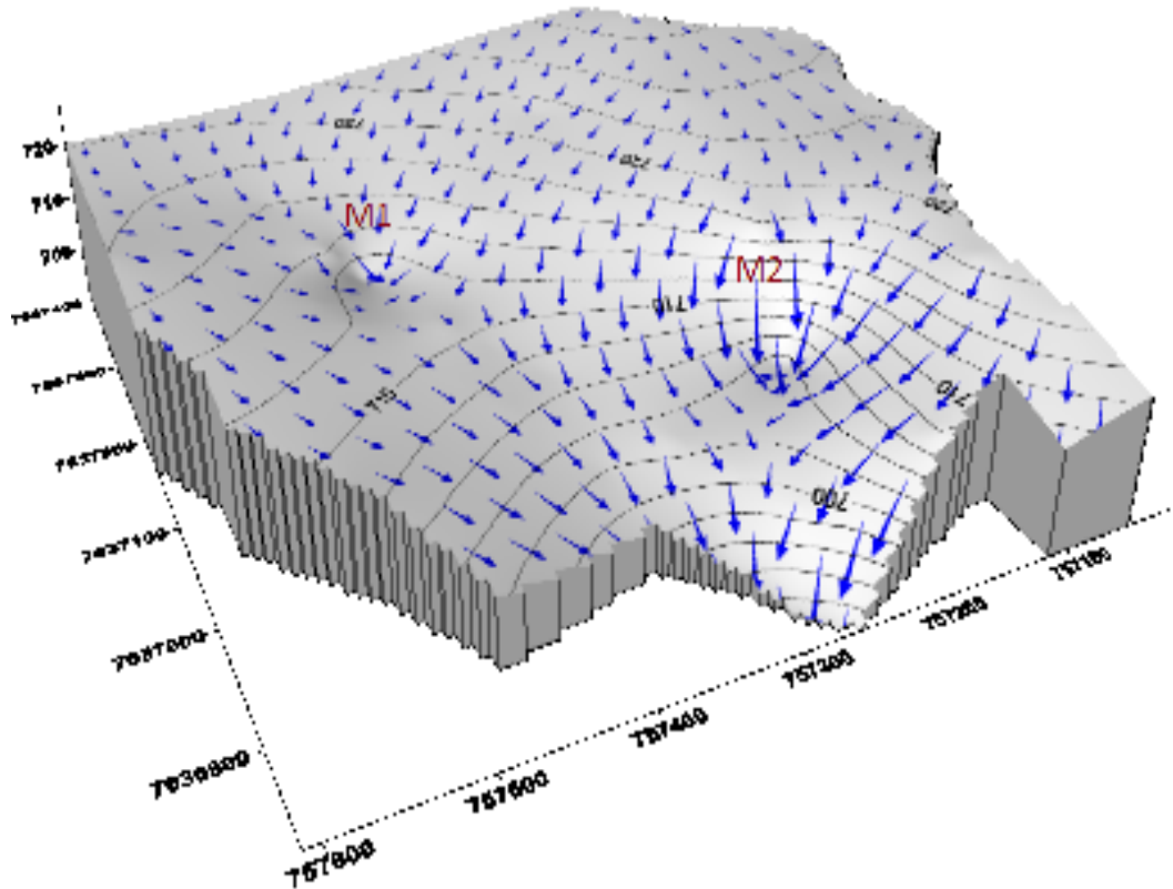
Figura 9. Simulações do fluxo de água e modelo digital de elevação (MDE) das microbacias M1 e M2.
