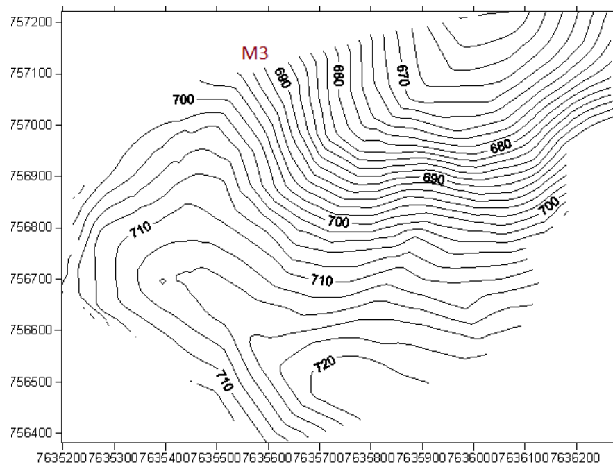
Figura 8. Planialtimetria da microbacia M3.
