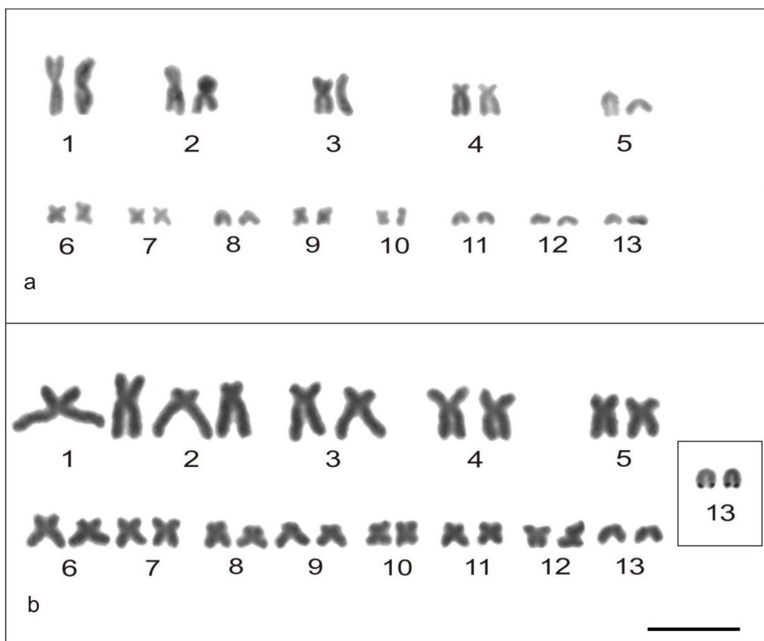
Figura 9. Cariótipos após coloração convencional com 2n=26 de (a) Flectonotus sp. e (b) Gastrotheca microdiscus . Em detalhe é mostrado o par portador da Ag-RON. Barra= 15\mu\text{m}
