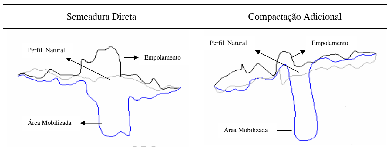
FIGURA 21 – Detalhes da Área Mobilizada, Empolamento e Perfil Natural dos tratamentos estudados.
