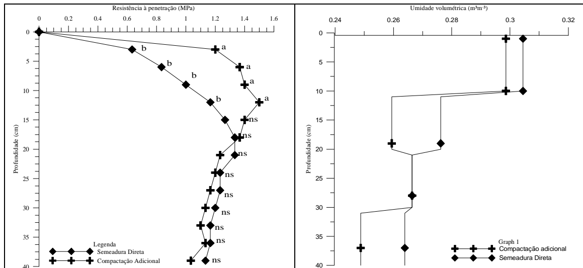
FIGURA 17 – Resistência mecânica à penetração e umidade volumétrica do solo nos diferentes tratamentos. Tratamentos com letras diferentes nas camadas, diferiram estatisticamente pelo teste DMS a 5% de probabilidade de erro. ns. diferença não significativa.
