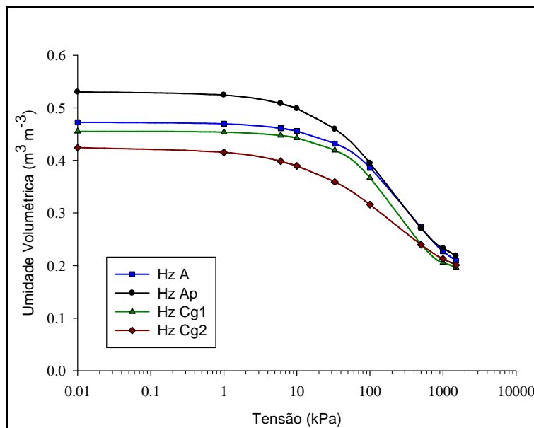
FIGURA 5 – Curva de retenção de água para o Gleissolo Háplico cultivado com arroz irrigado por inundação.
