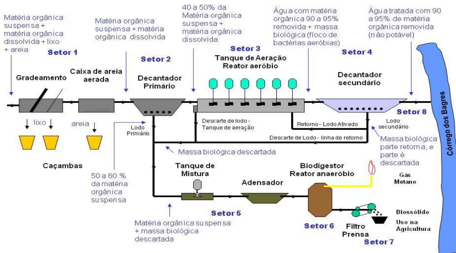
Figura 1. O processo de tratamento de esgotos na ETE de Franca.
