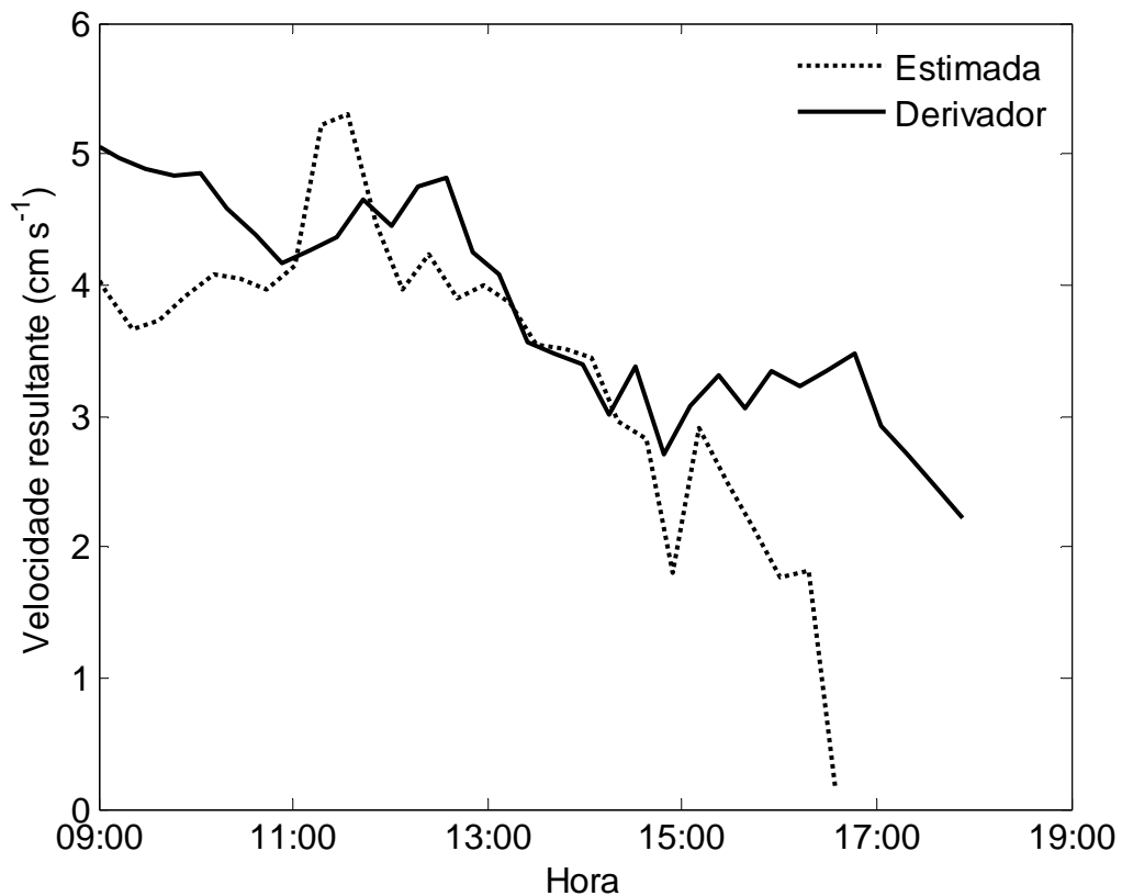
Gráfico 14 – Gráfico da velocidade da corrente a um metro de profundidade. A linha contínua representa os dados observado pelo derivador 1 no dia 13 de janeiro de 2009, e a linha tracejada representa os valores estimados a partir dos dados de vento para o mesmo período de tempo. As séries foram filtradas e foram removidos os sinais com frequência maiores do que \frac{1}{15 \times 60} \text{ s}^{-1} . Os valores estão avançados no tempo por um fator de 2,5 horas.
