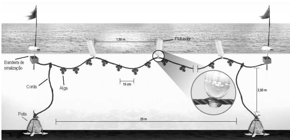
Figura 2. Esquema ilustrativo da implantação da estrutura de cultivo (tipo “long line”) utilizada no cultivo de algas marinhas na praia de Pau Amarelo.
