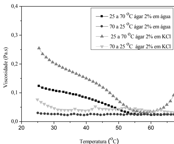
Figura 7. Efeito da temperatura na viscosidade em H 2 O e KCl para uma solução 2% a 1Hz
