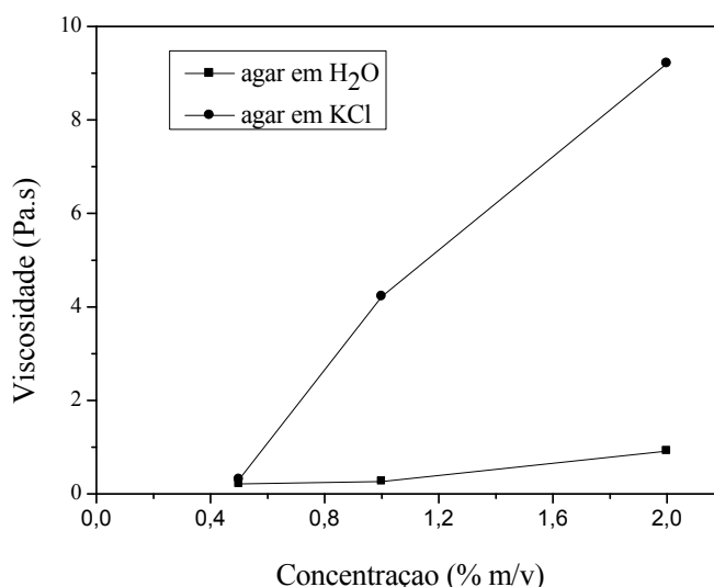
Figura 6. Variação da viscosidade com a concentração de ágar em dois solventes diferentes
