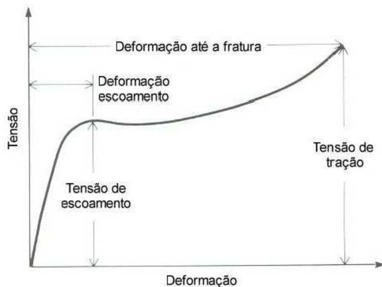
Figura 5: Curva tensão-deformação generalizada para plásticos.
