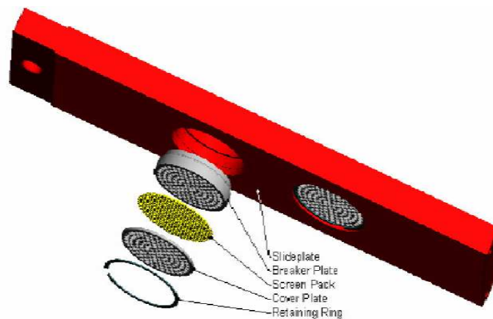
Figura 8: Representação esquemática da posição das telas filtro com anel de vedação, no sistema de filtragem.
