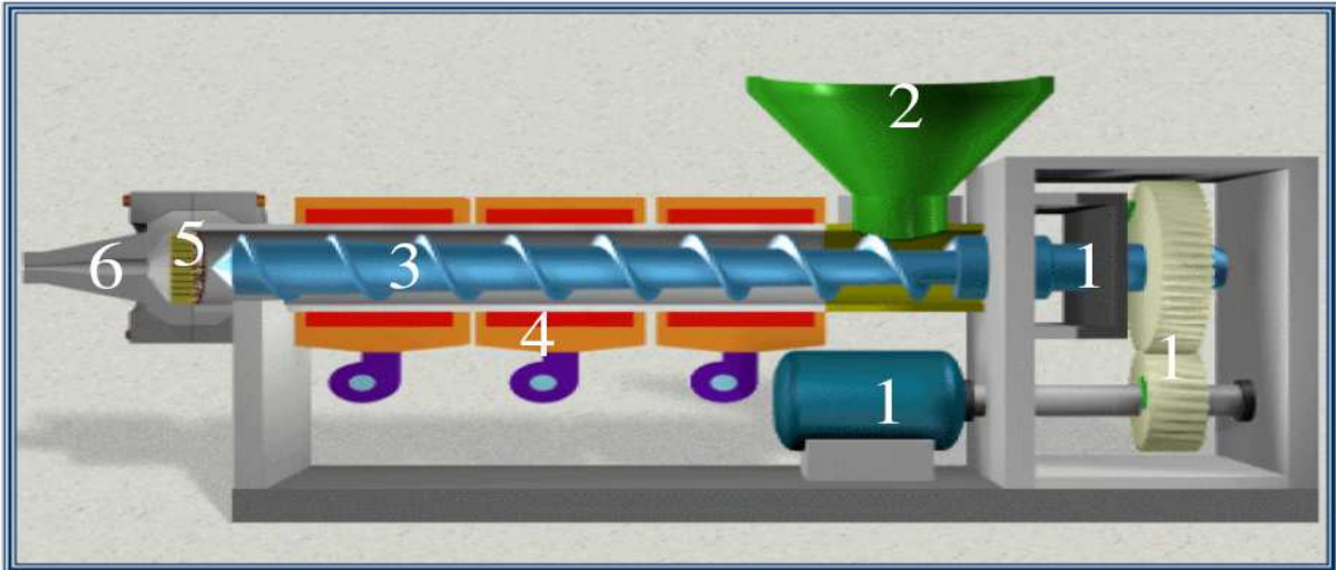
Figura 6. Esquema de uma extrusora monorosca.
