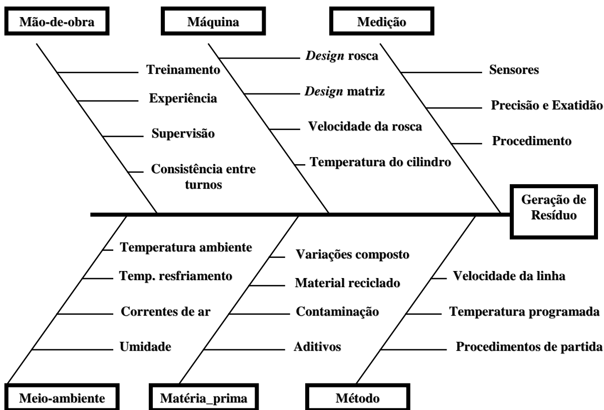
Figura 37: Diagrama de causa e efeito do estudo do processo de extrusão na geração de resíduos.
