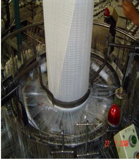
Figura 23: Painel do Tear Fonte: REGISTRO FOTOGRÁFICO DO AUTOR, 2006.
