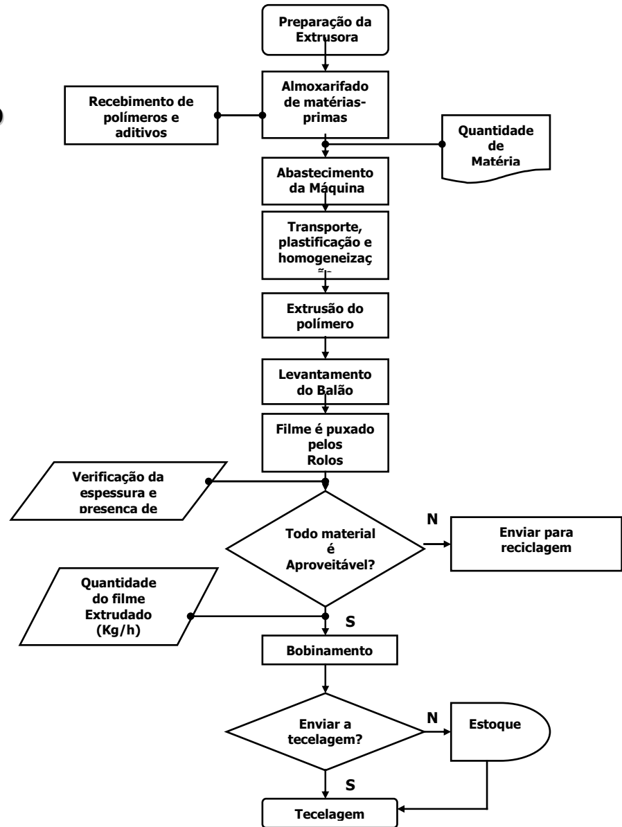
Figura 36: Definição do fluxograma do processo de extrusão
