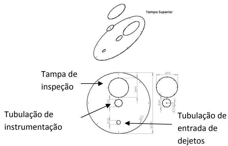
FIGURA 15 - TAMPA DO BIODIGESTOR FONTE: BALMANT (2009)
