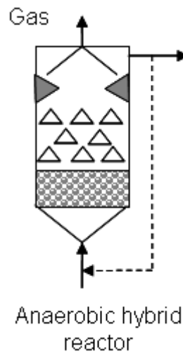
FIGURA 9 - BIODIGESTOR DE LEITO HÍBRIDO
