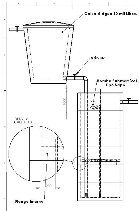
FIGURA 14 - VISÃO LATERAL DO BIODIGESTOR FONTE: BALMANT (2009)
