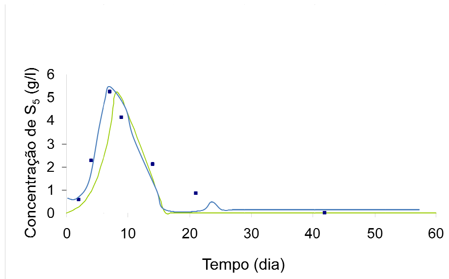
FIGURA 24 - COMPARAÇÃO ENTRE O MODELO E OS RESULTADOS EXPERIMENTAIS (•) PARA A CONCENTRAÇÃO DE S 5
