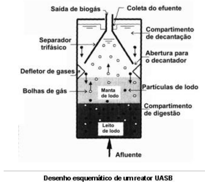
Figura 2 - REATOR UASB TÍPICO FONTE: UASB (2009)
