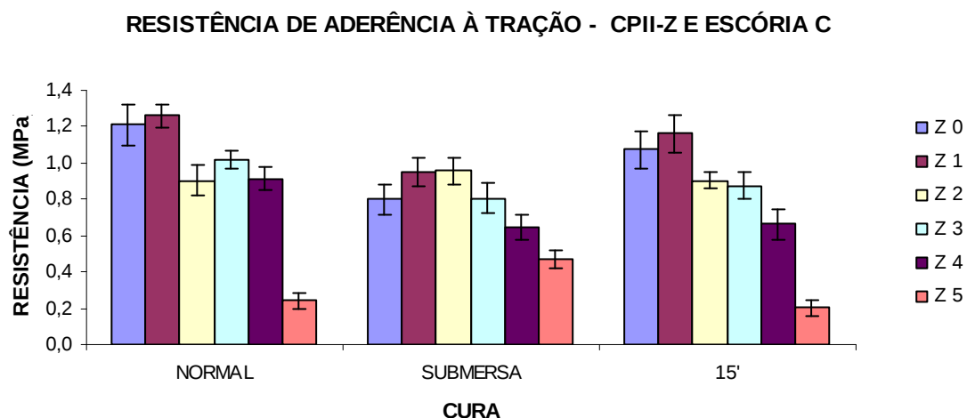
FIGURA 16. RESISTÊNCIA DE ADERÊNCIA À TRAÇÃO DAS COMPOSIÇÕES DE CII- Z E A ESCÓRIA C
