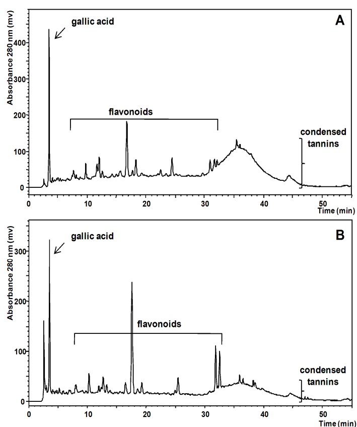
Figura 1. Perfil fitoquímico obtido em HPLC dos extratos metanólicos de D. elliptica (A) e D. nitida (B) (Kushima et al. , 2009).
